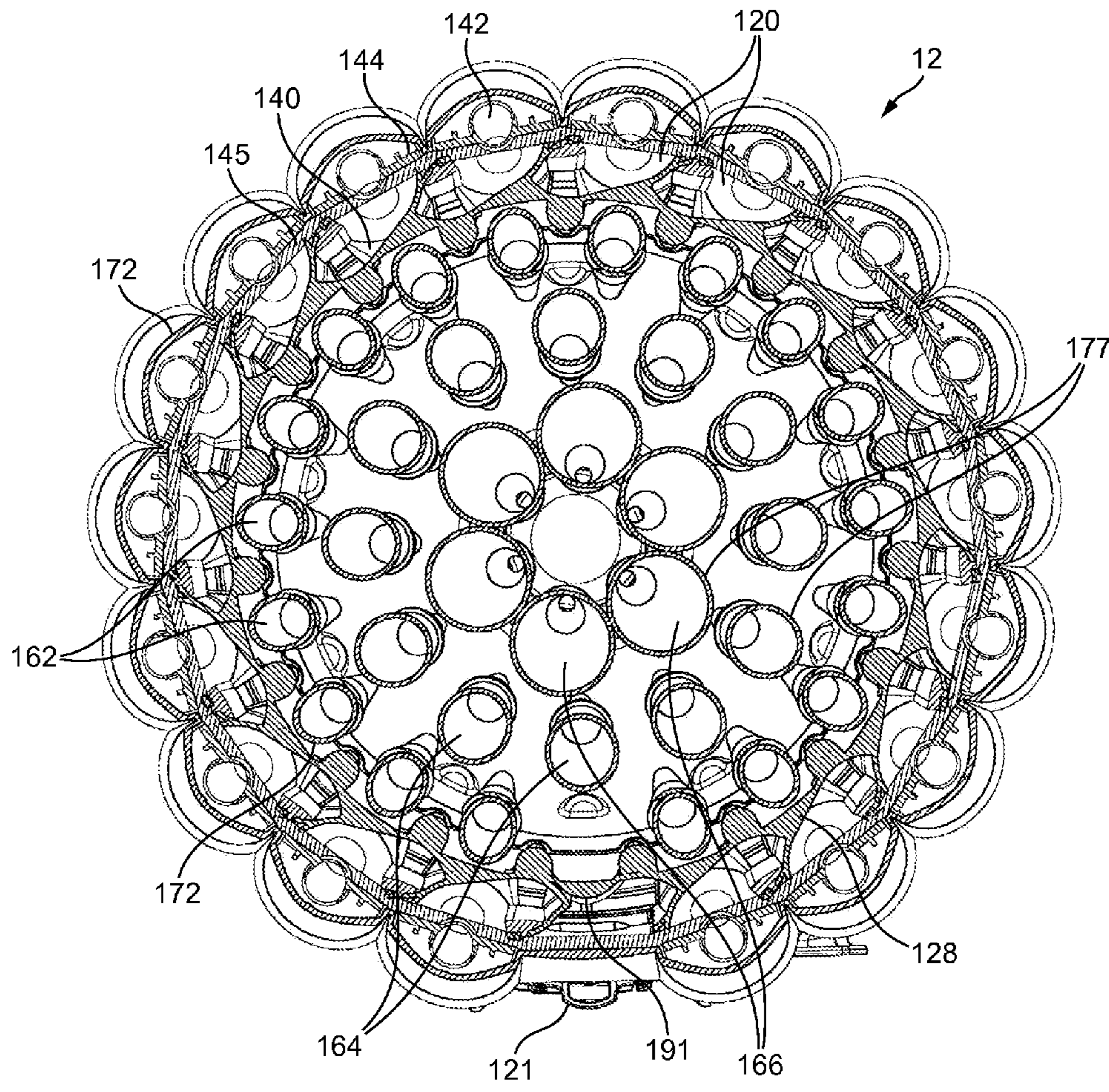
B - B FIG. 6(b)
