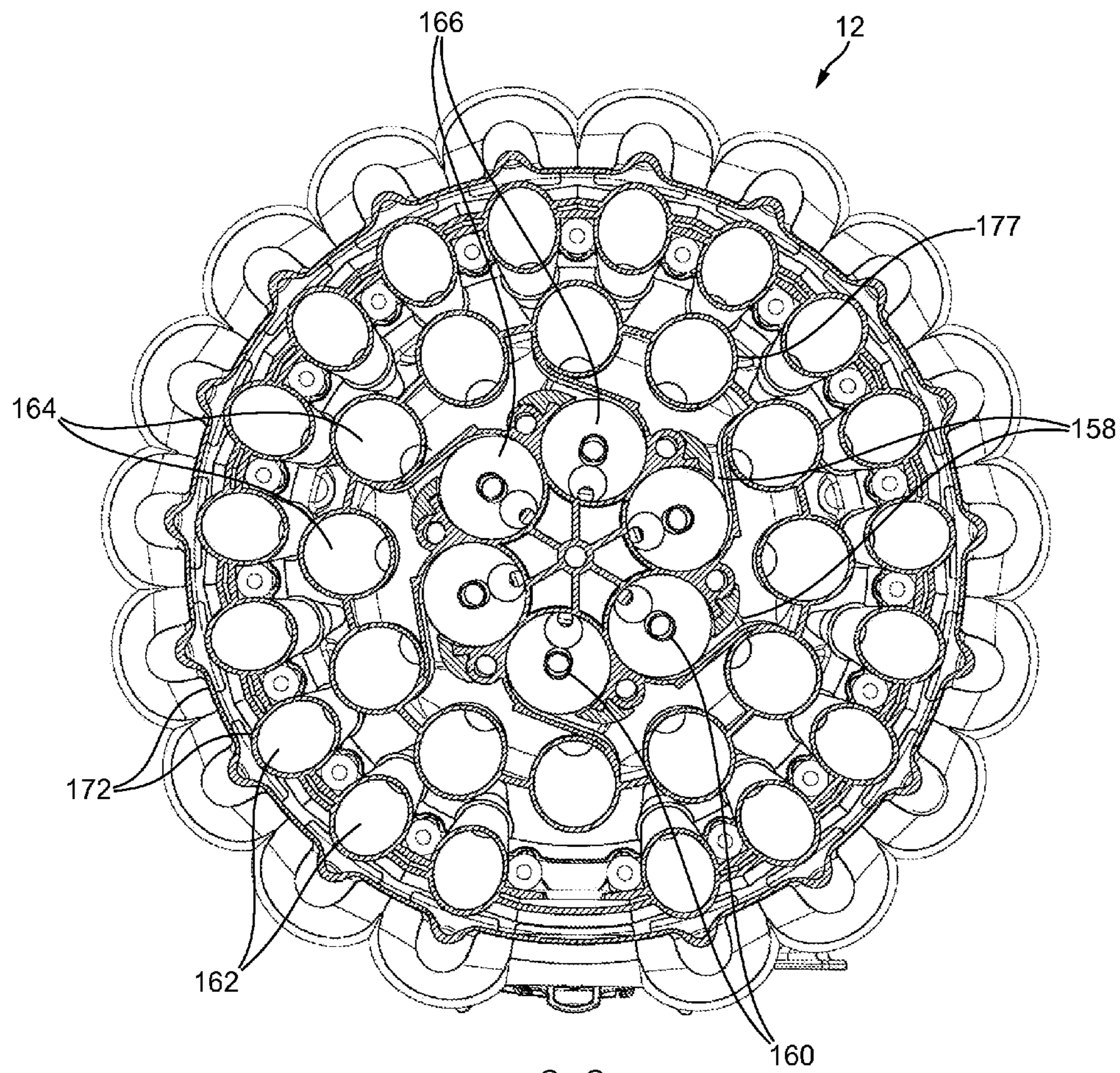
C - C FIG. 6(c)
