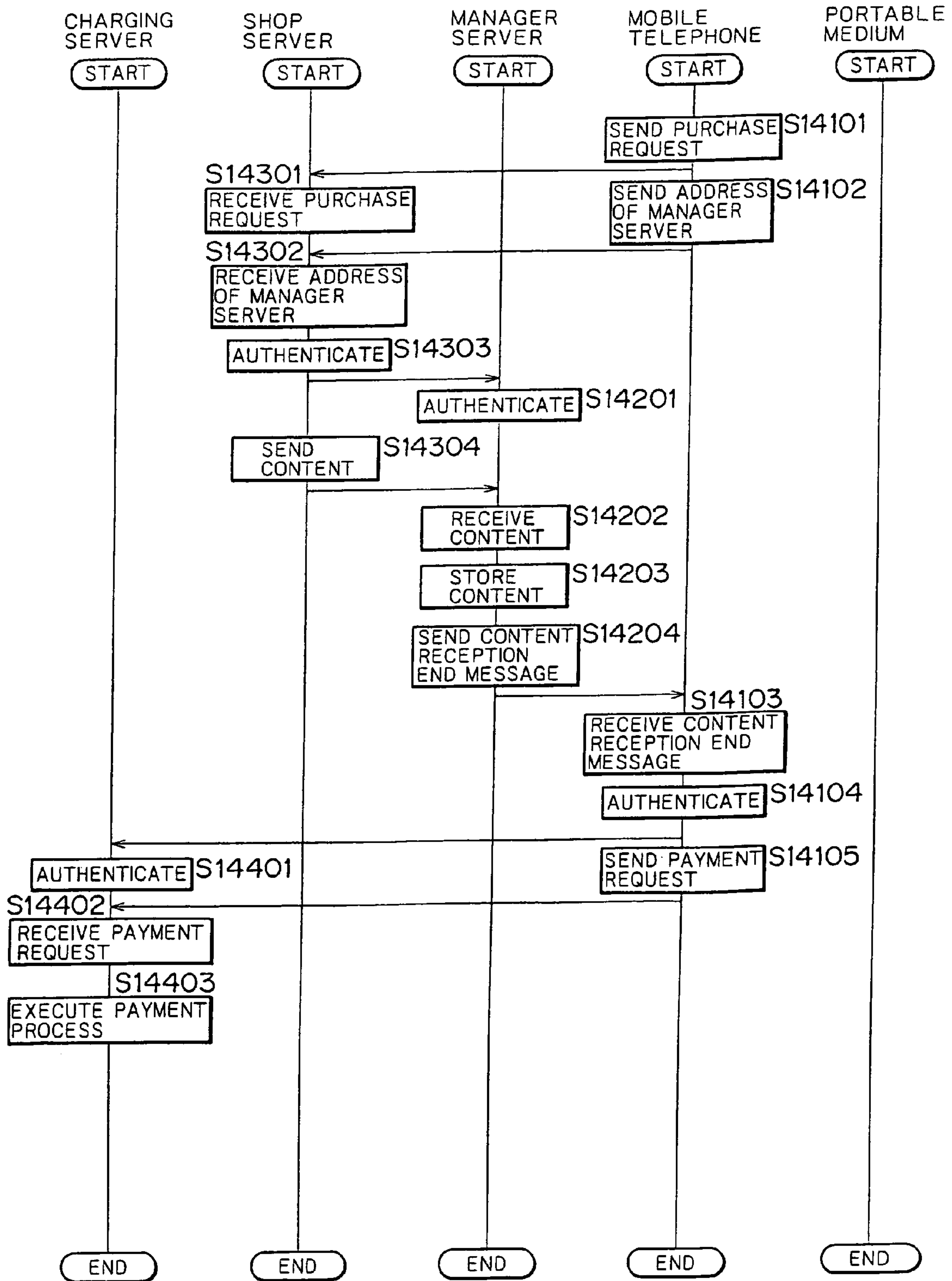
FIG. 39
