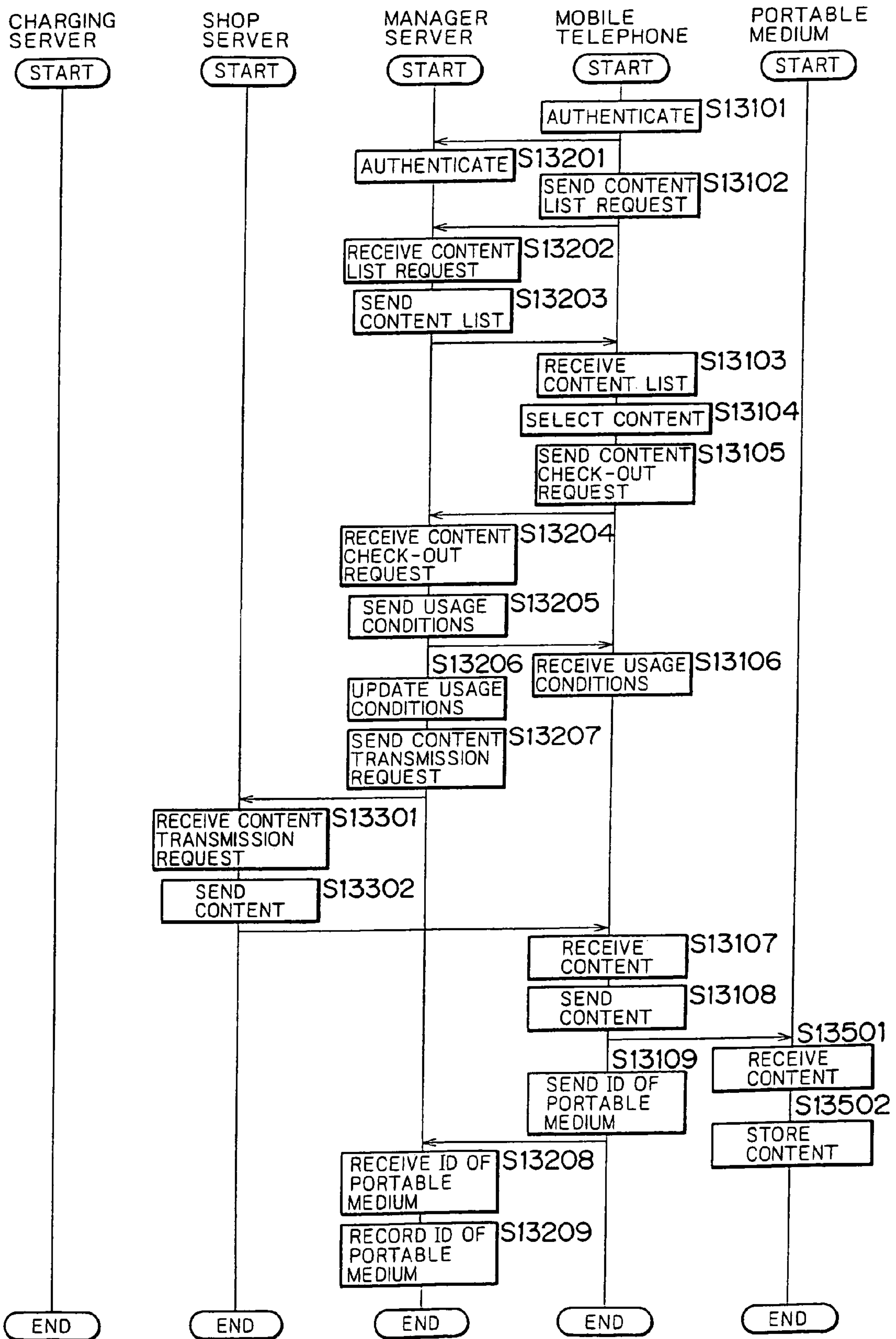
FIG. 37
