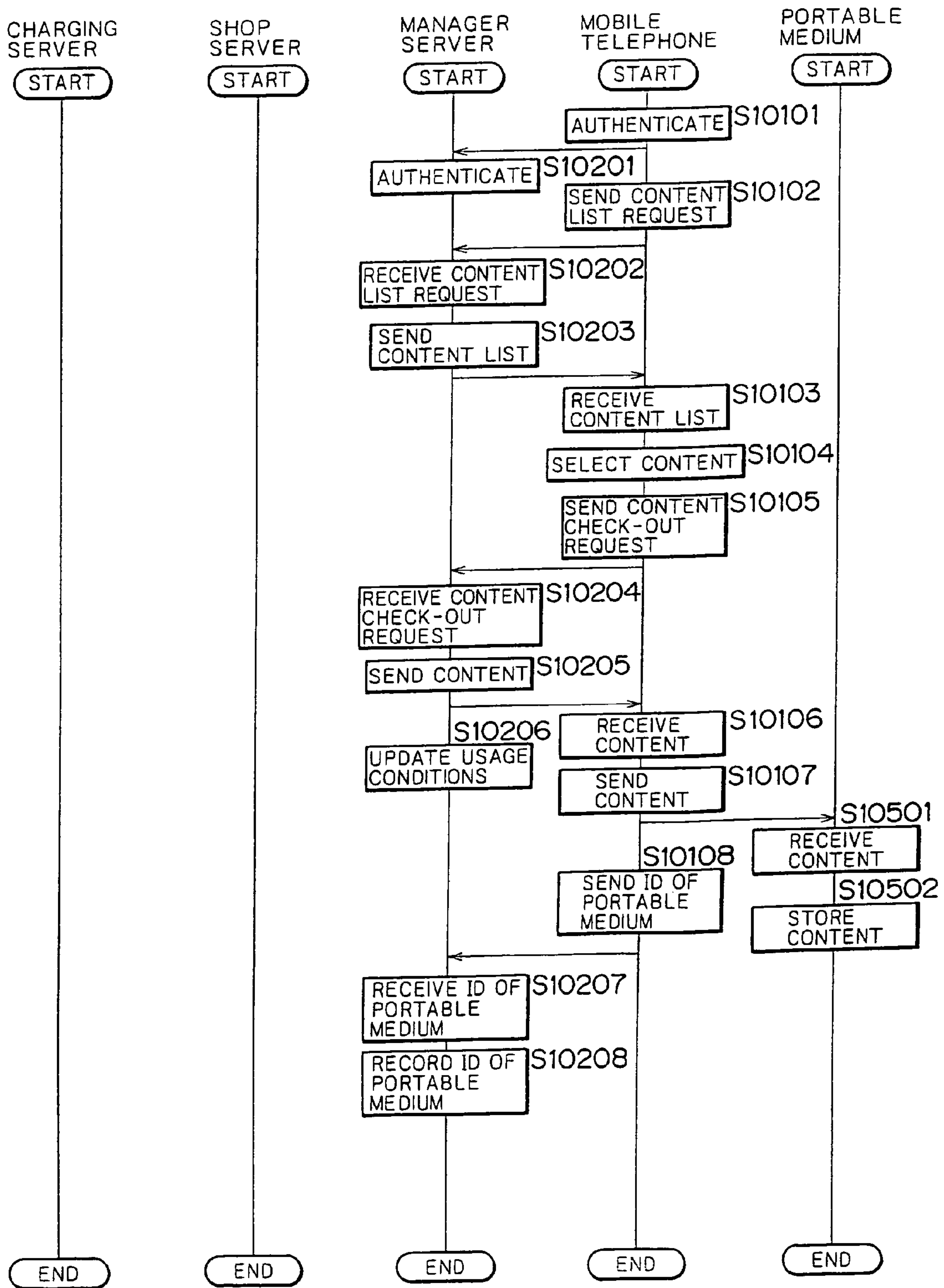
FIG. 32
