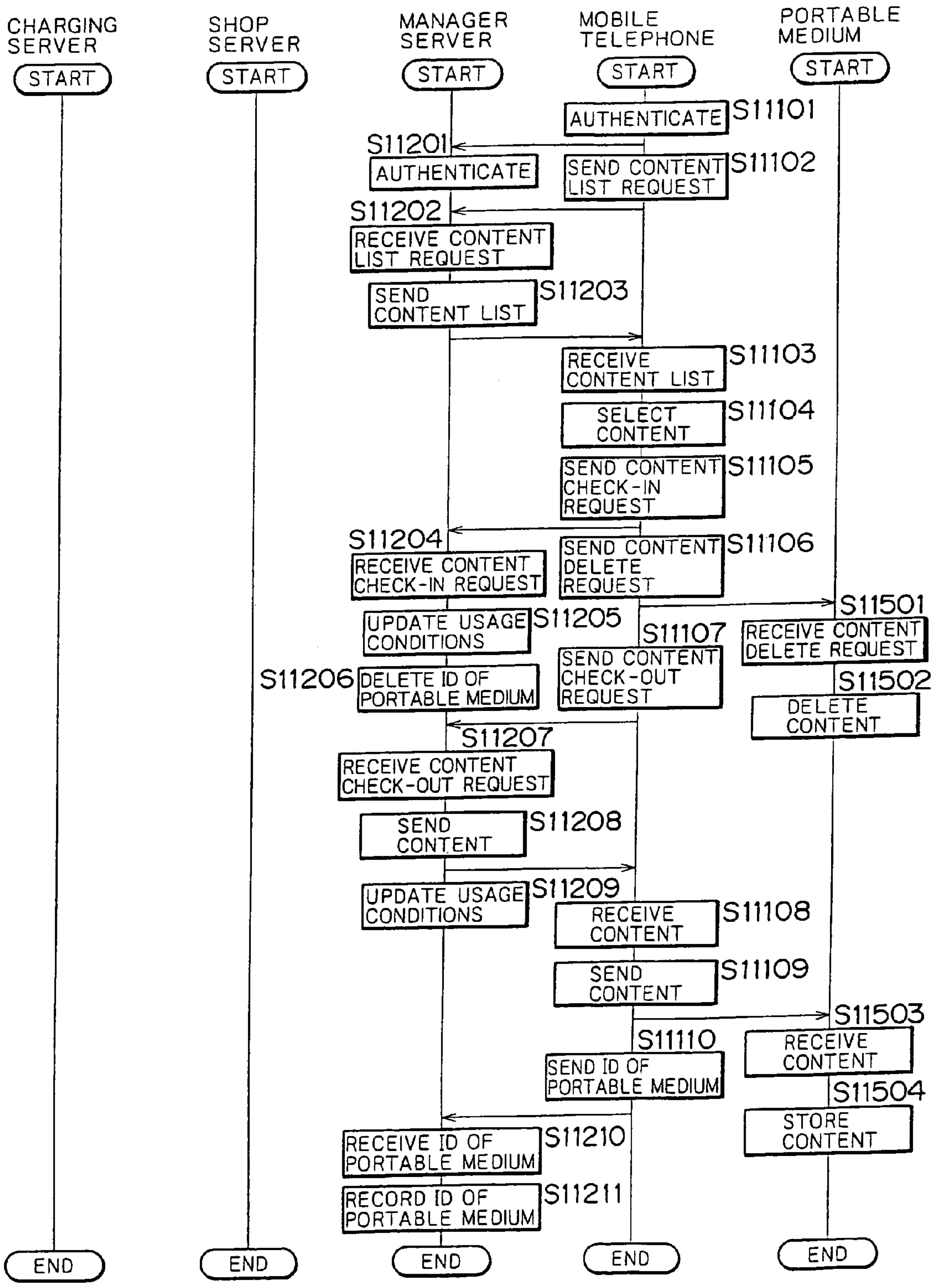
FIG. 33
