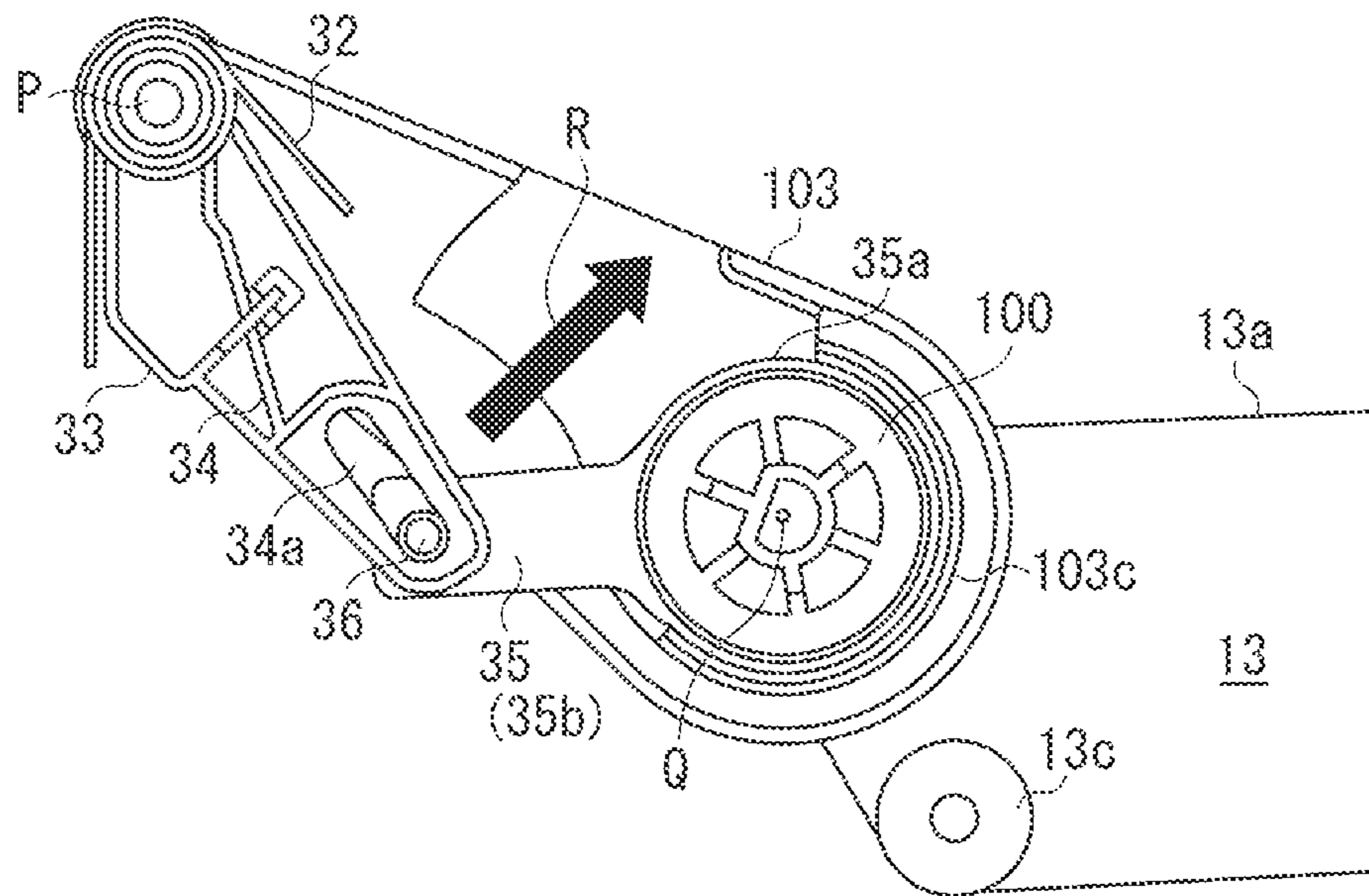
FIG. 9A DOOR OPENED STATE
