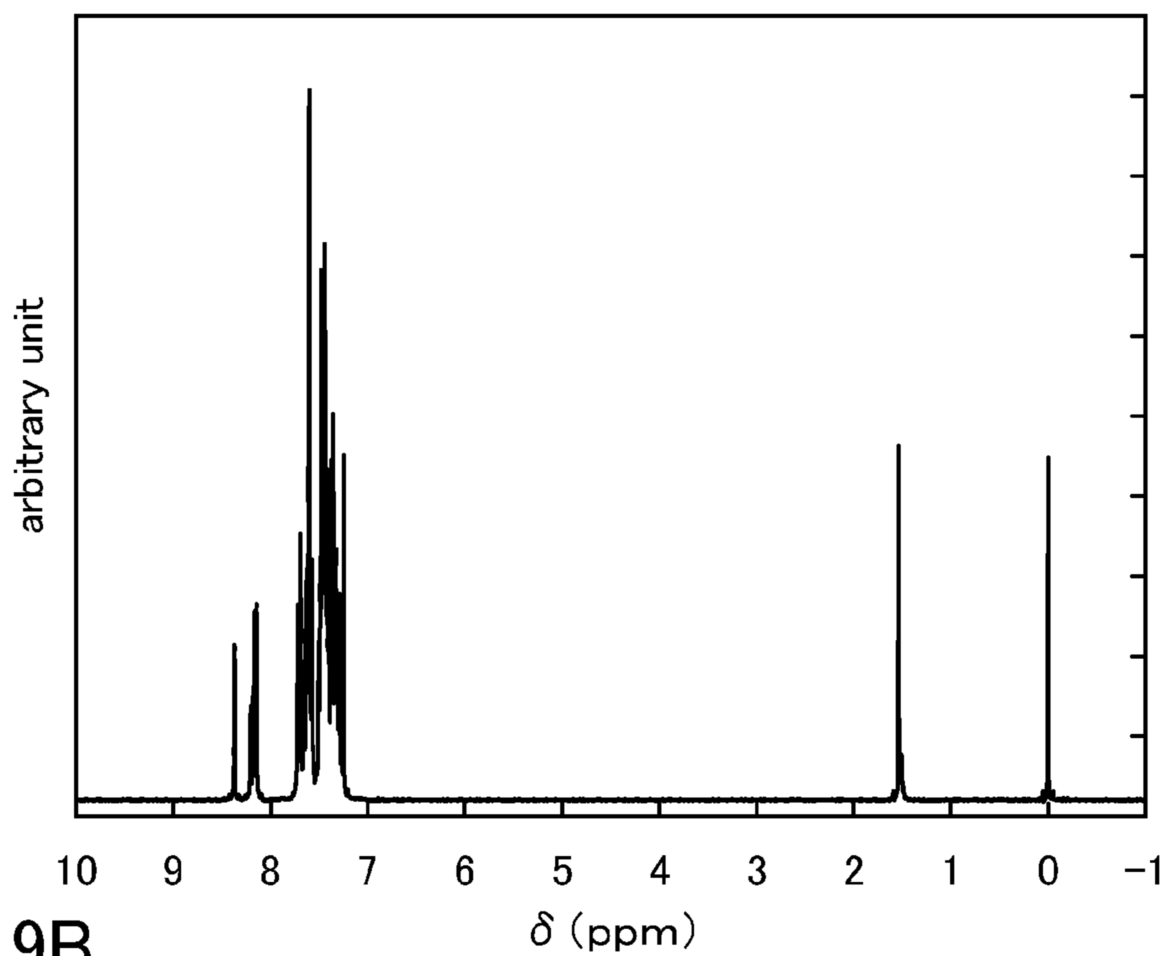
FIG. 19A
