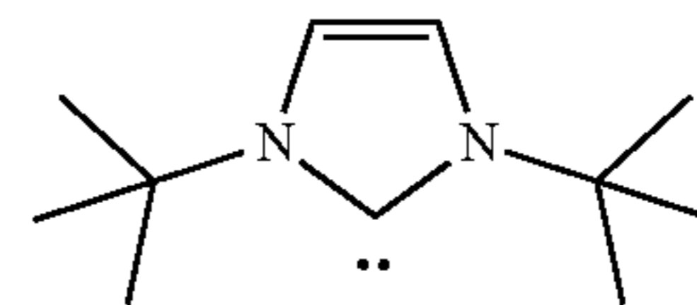
1,3-Di-t-butylimidazol-2-ylidene (Im-6)
