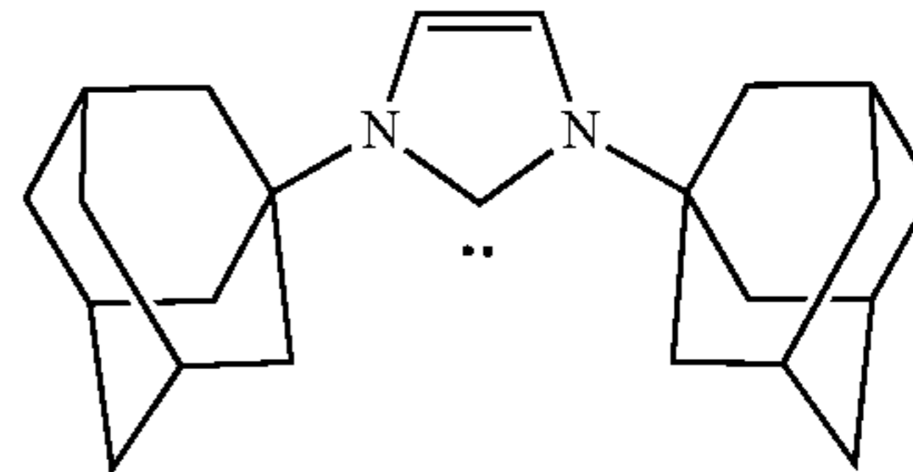
1,3-Bis(1-adamantyl)imidazol-2-ylidene (Im-4)
