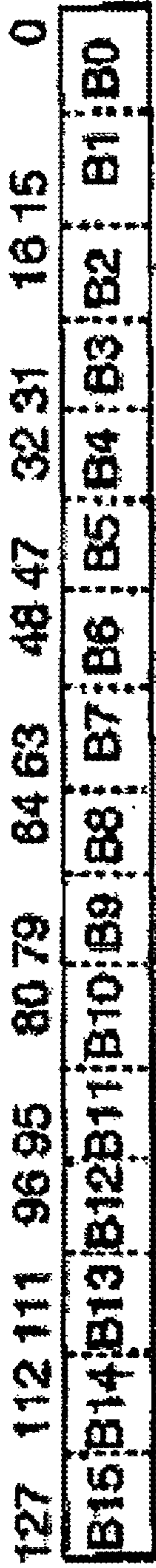
Packed Byte 421
