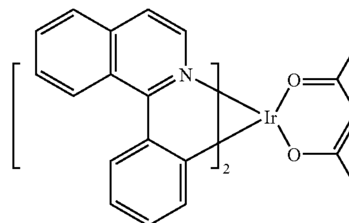
Ir(piq) 2 (acac)
