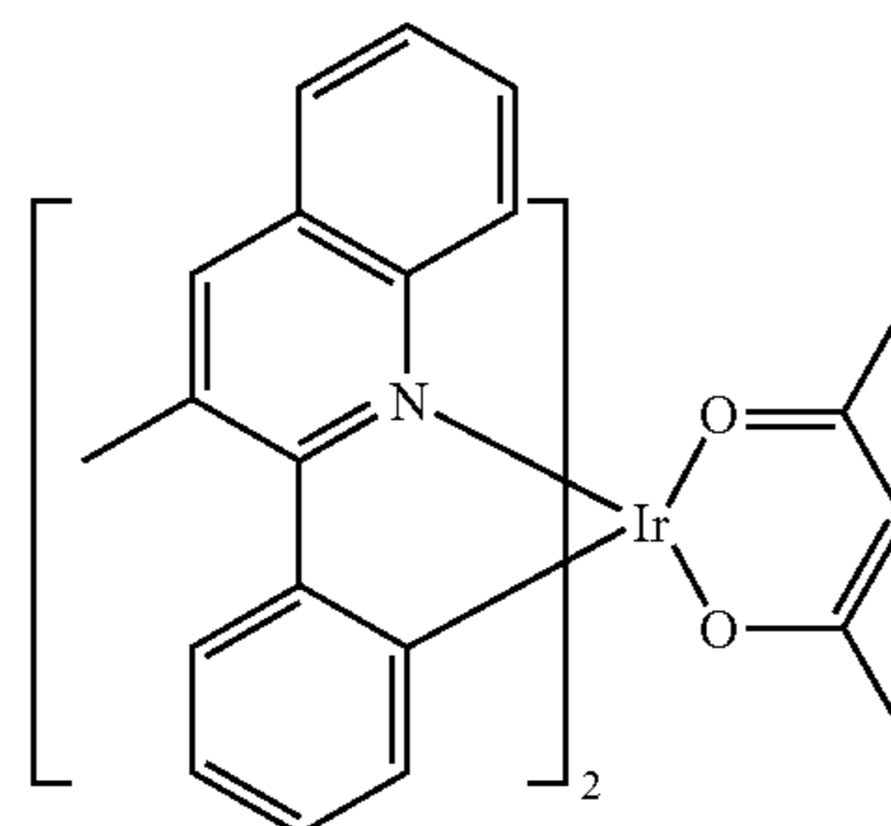
Ir(3-Mepq) 2 (acac)
