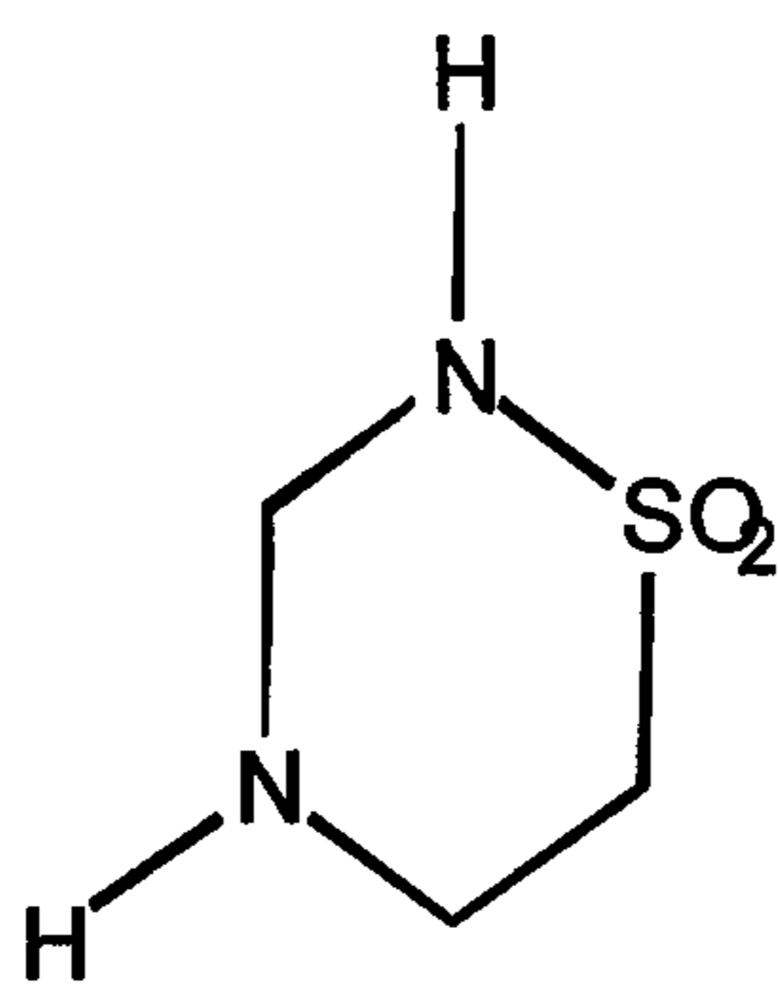
Taurultam
