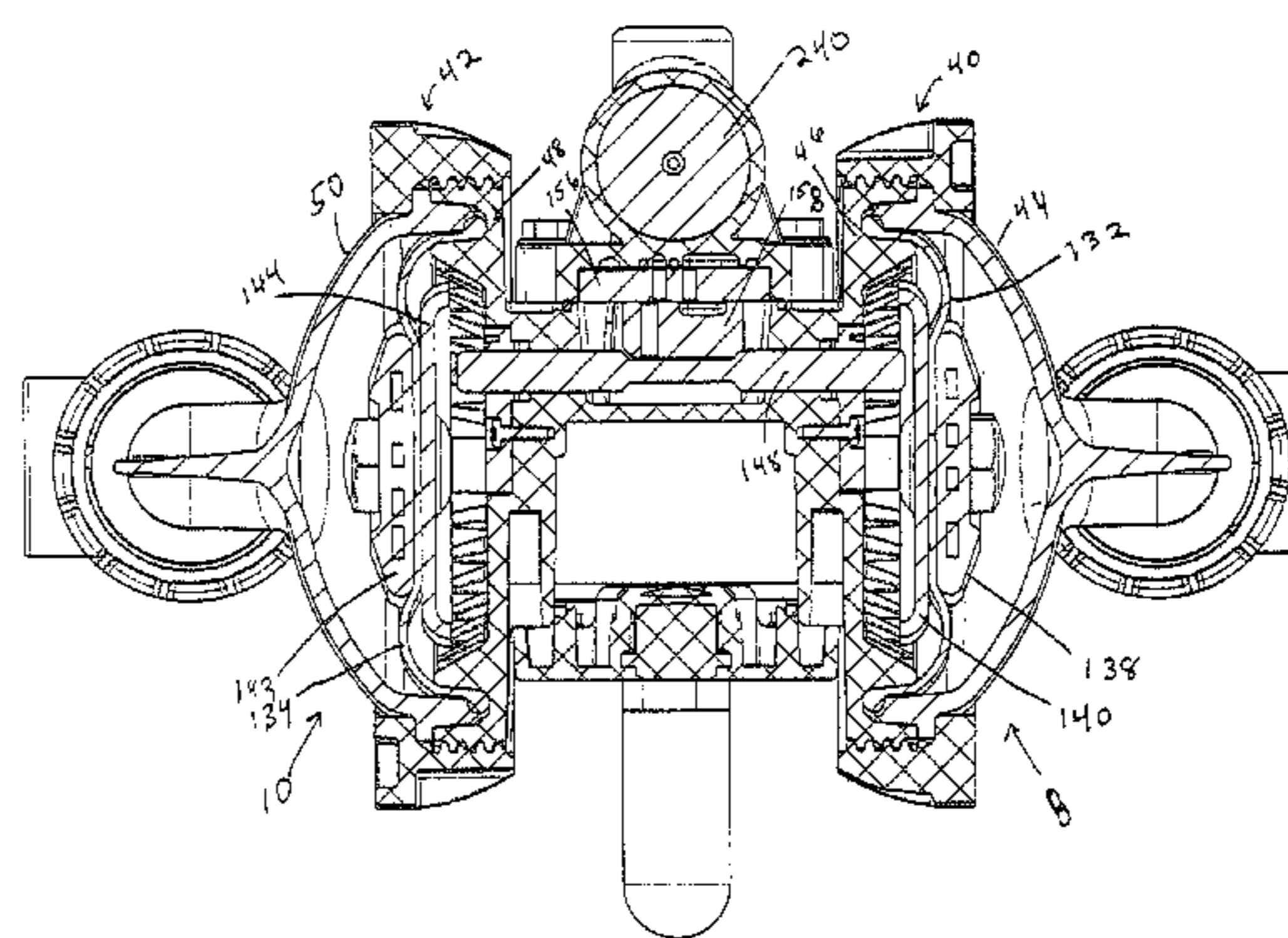
SECTION A-A
