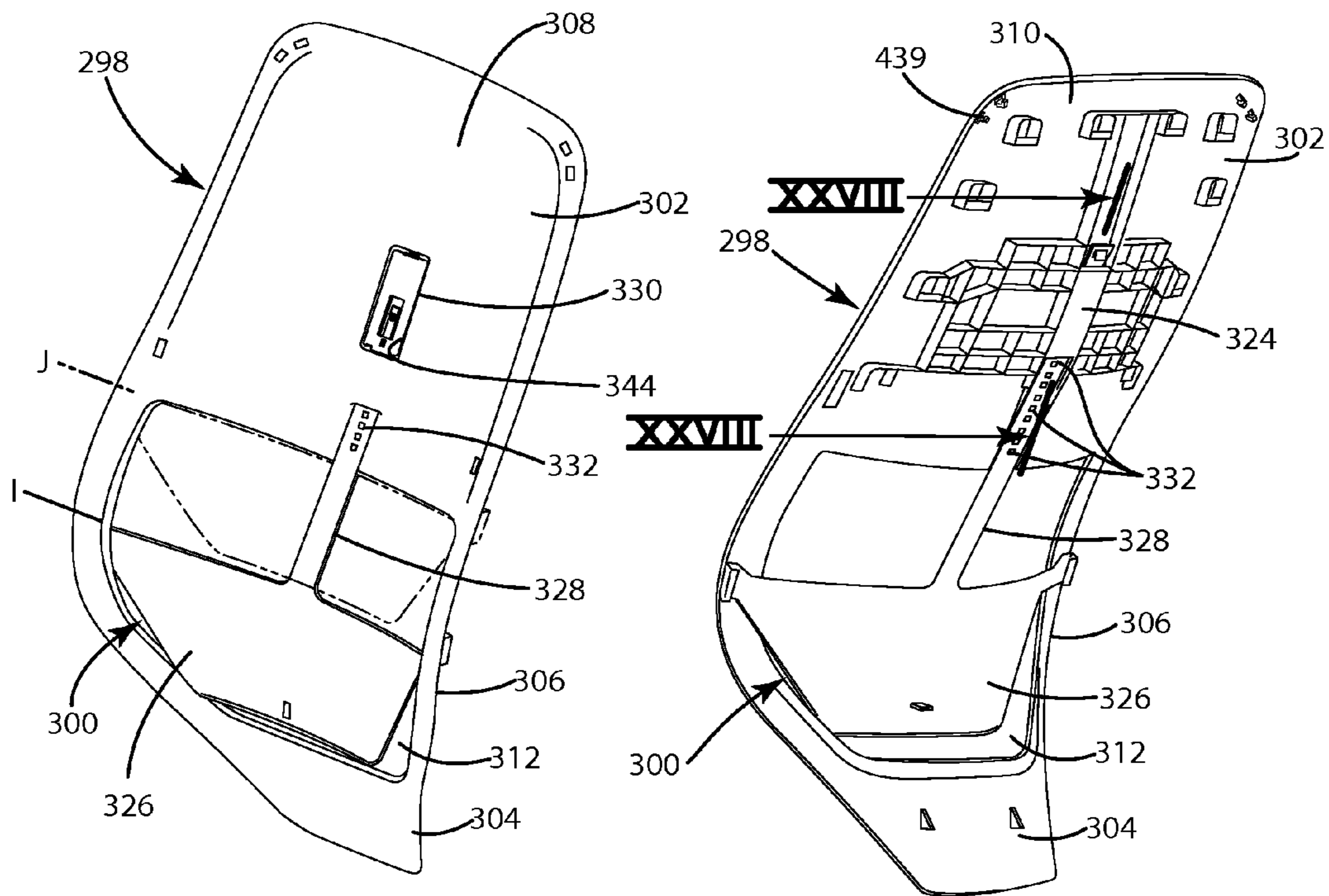
Fig. 26A
