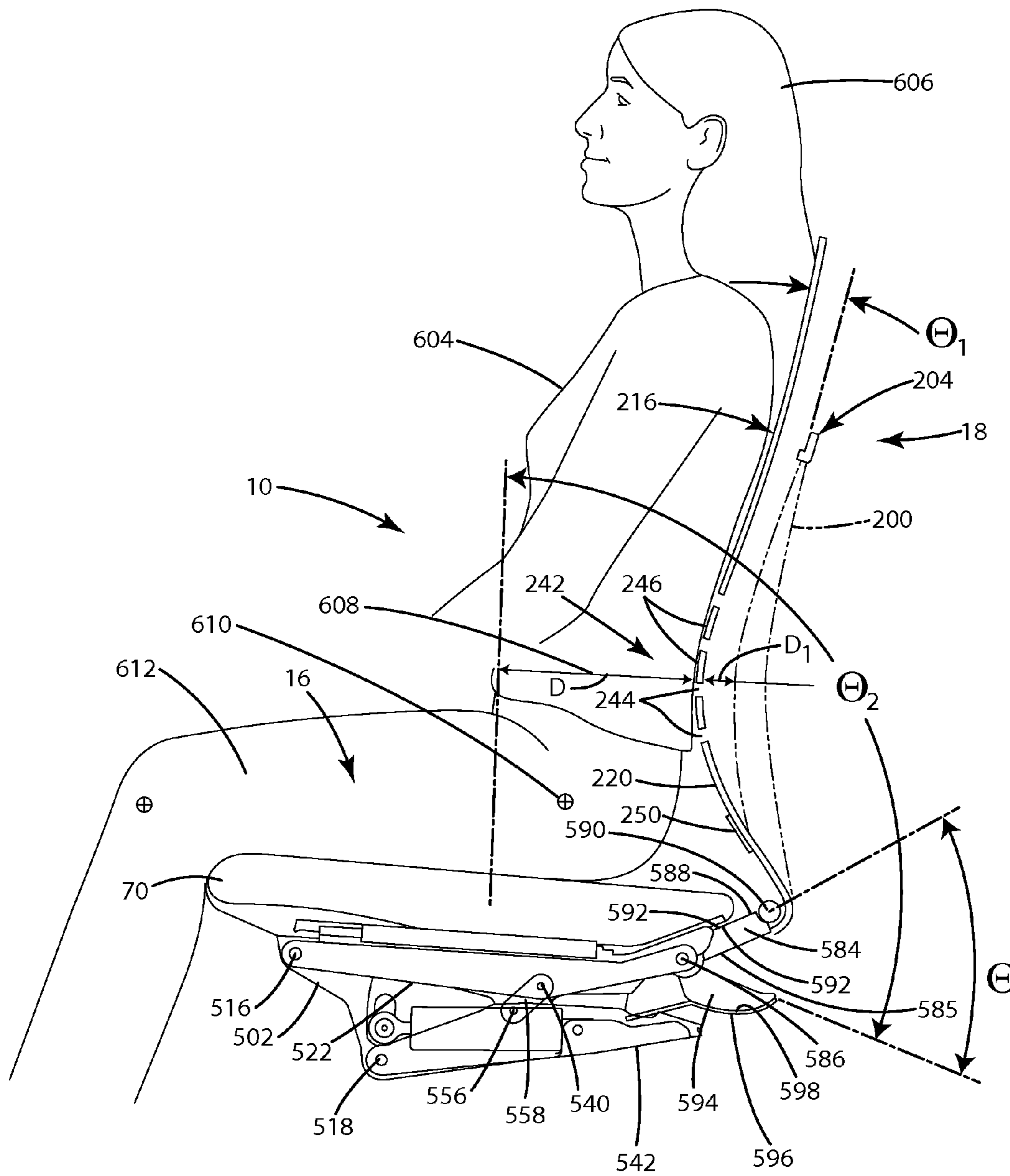
Fig. 49
