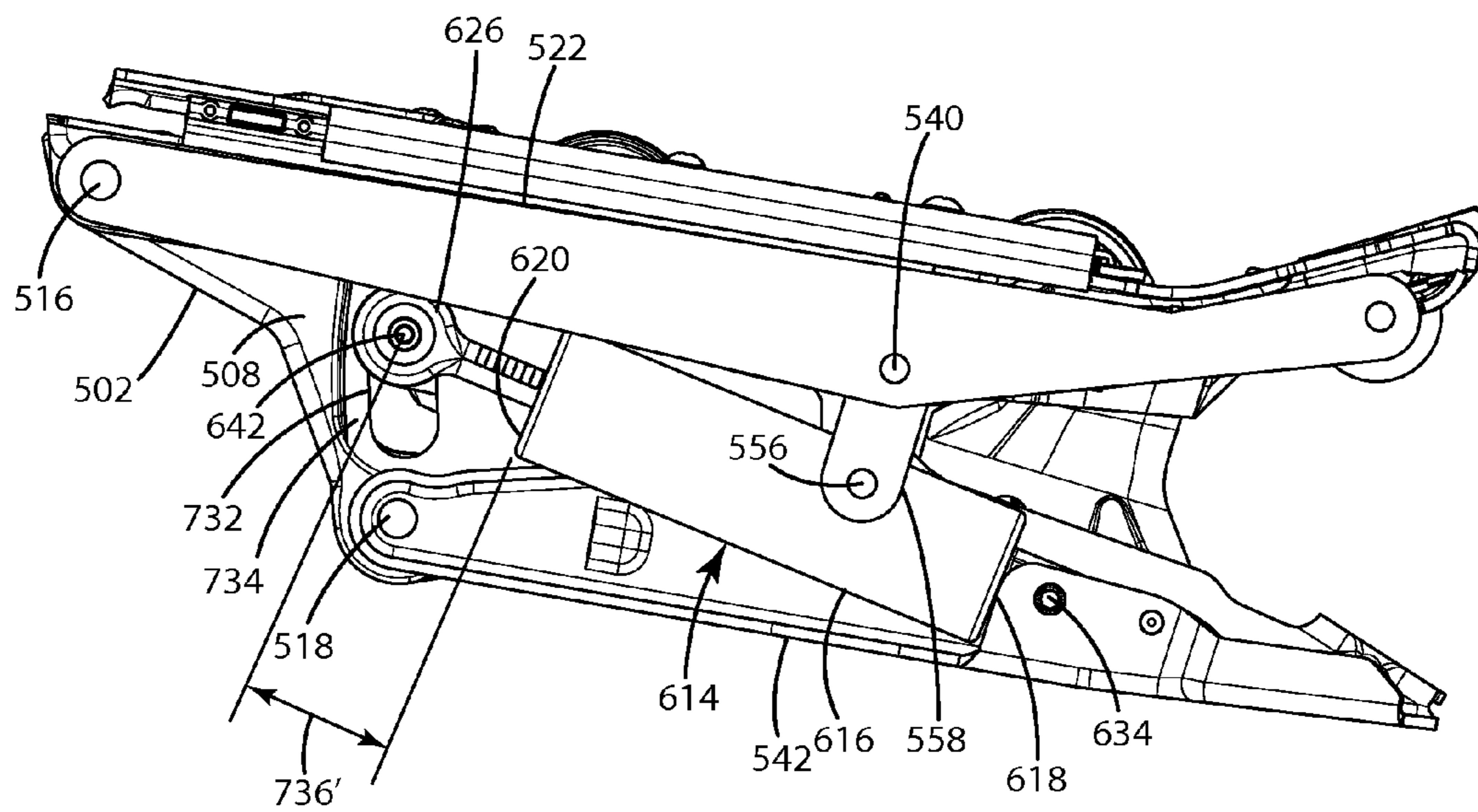
Fig. 58B
