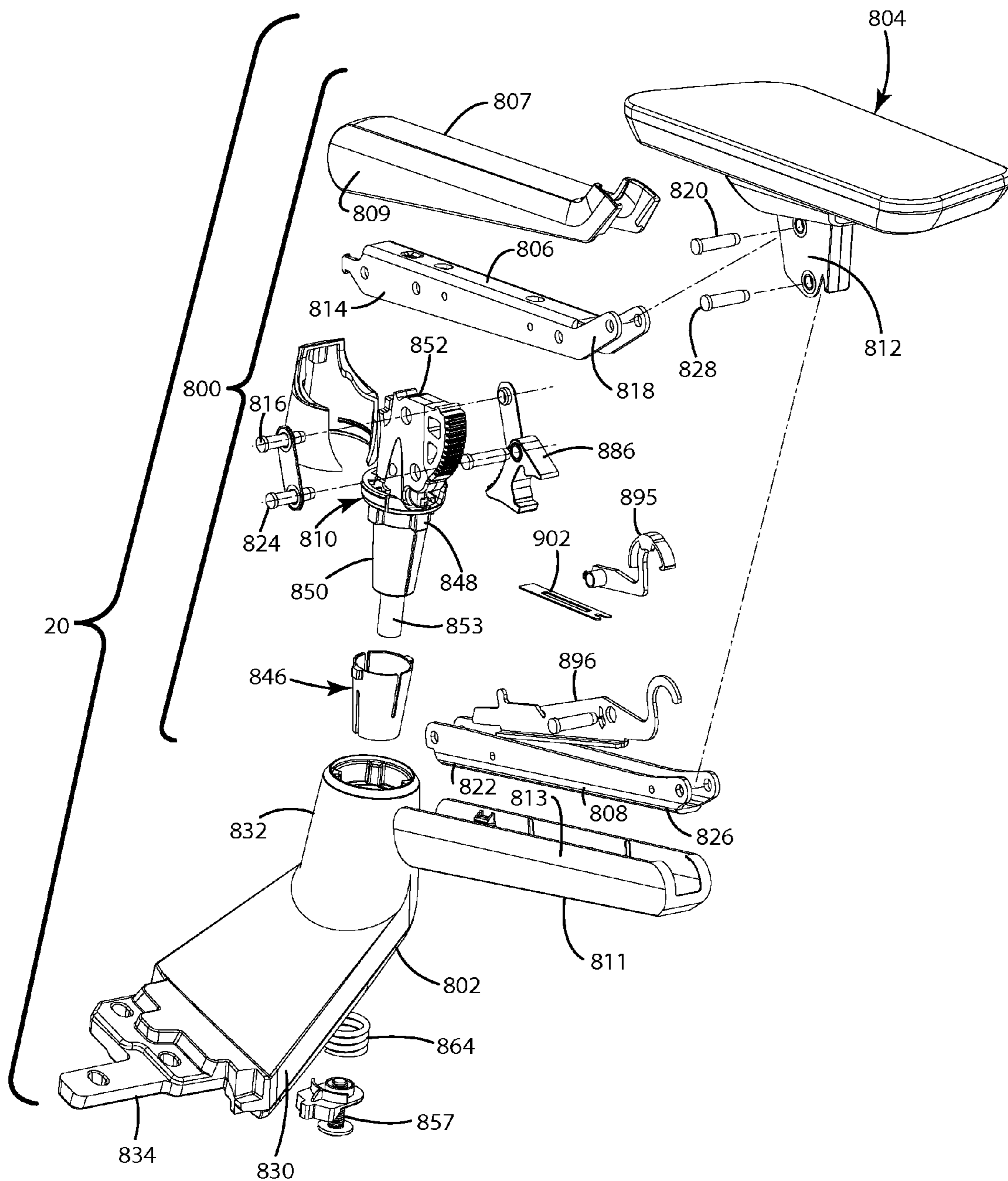
Fig. 69
