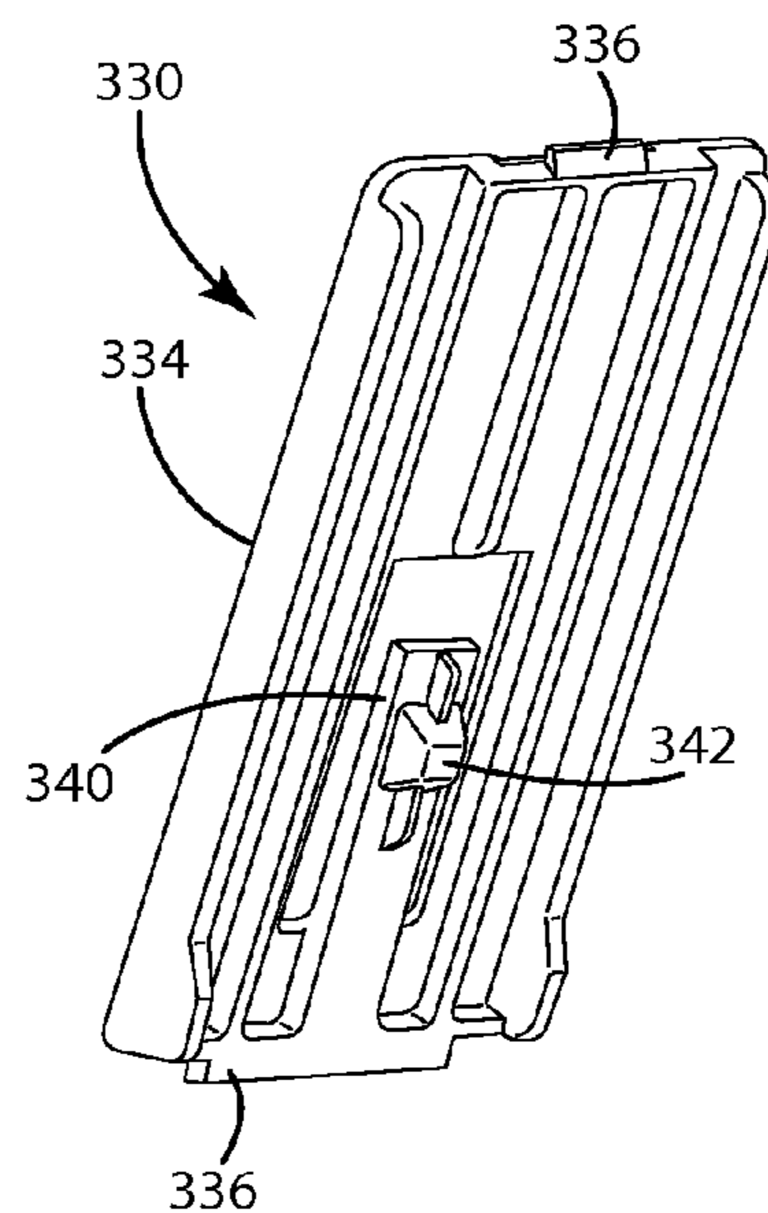
Fig. 27B
