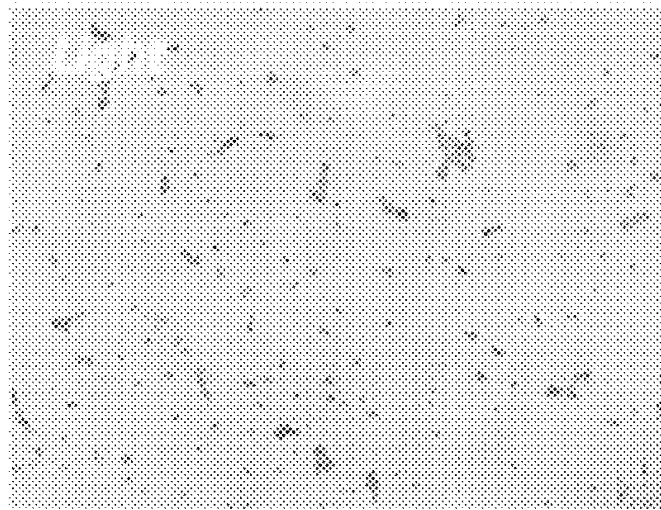
S. aureus
