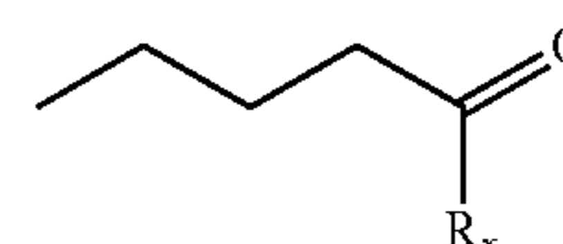
(5:Ald)
