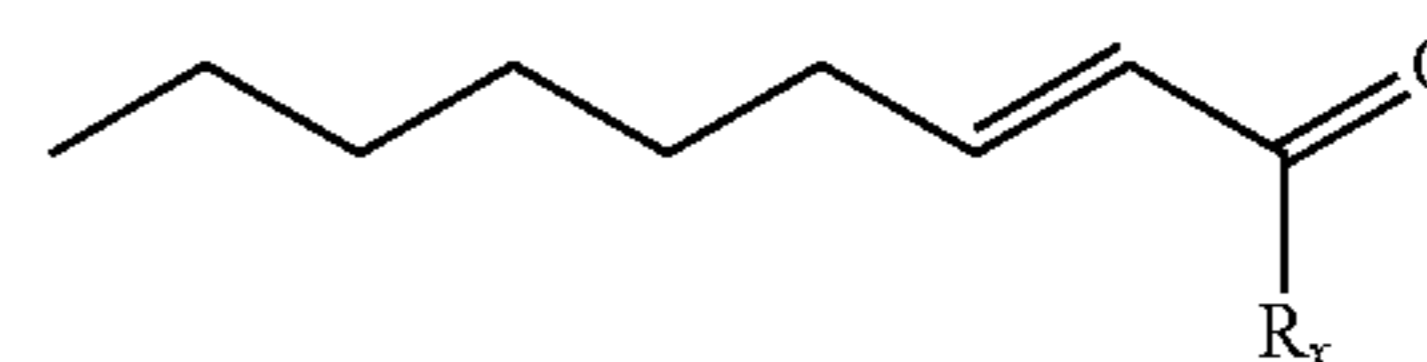
(E2-9:Ald)
