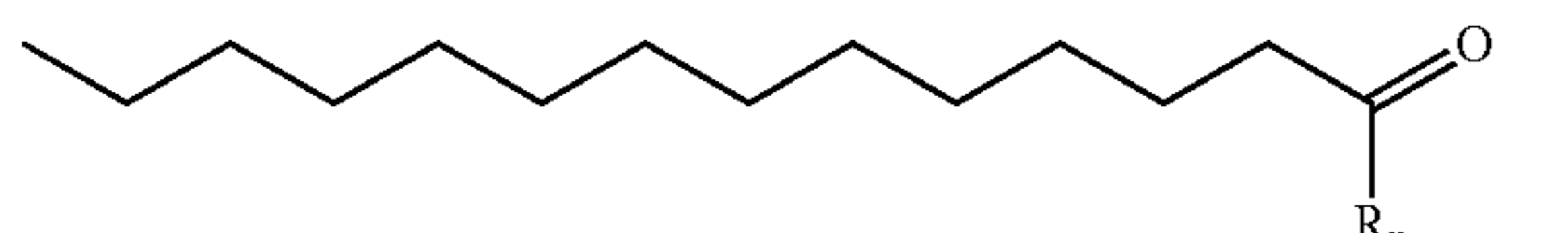
(14:Ald)
