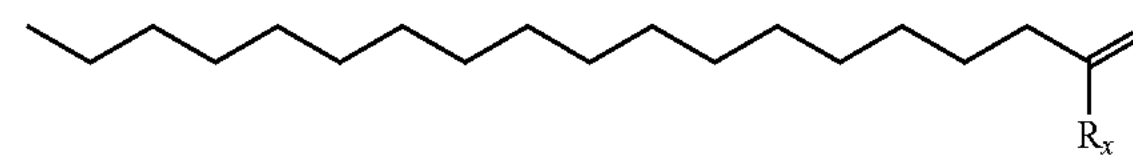
(18:Ald)
