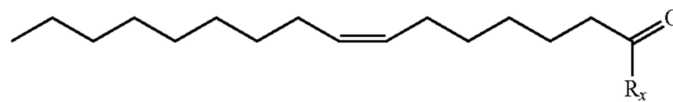
(Z7-16:Ald)
