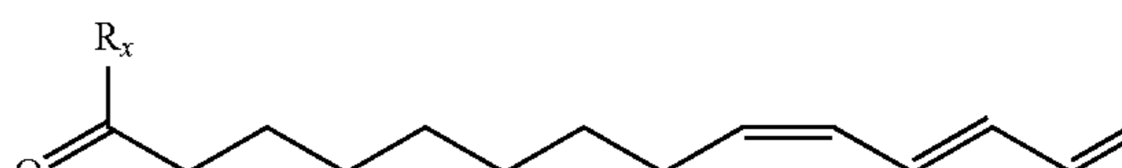
(Z9,E11,13-14:Ald)
