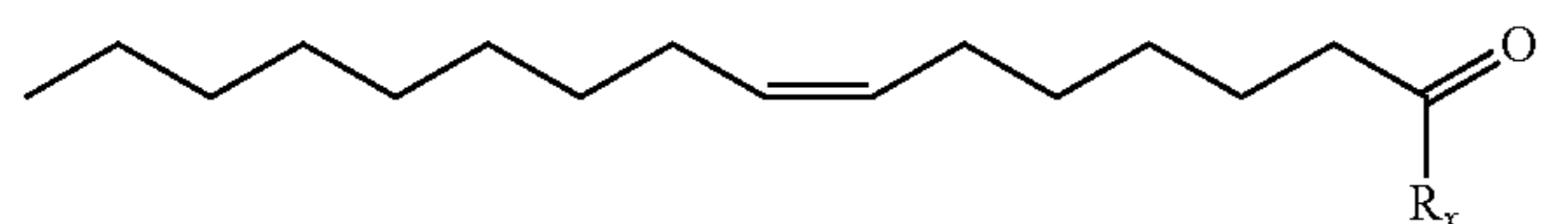
(Z7-16:Ald)
