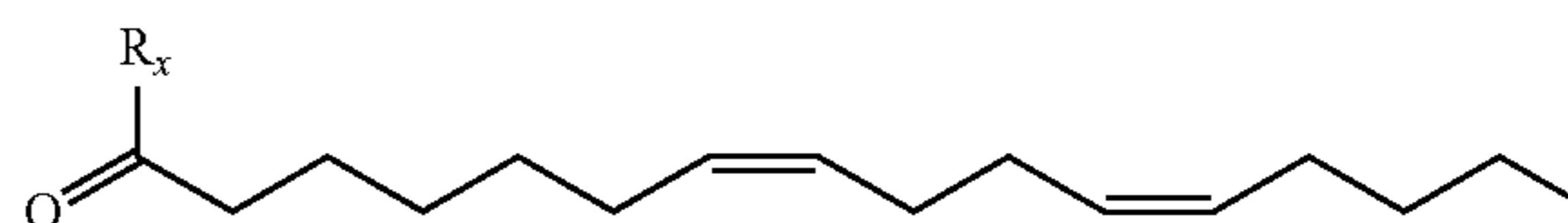
(Z7,Z11-16:Ald)
