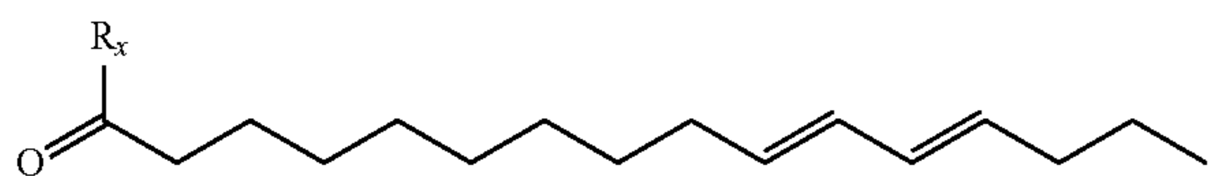
(E10, E12-16:Ald)
