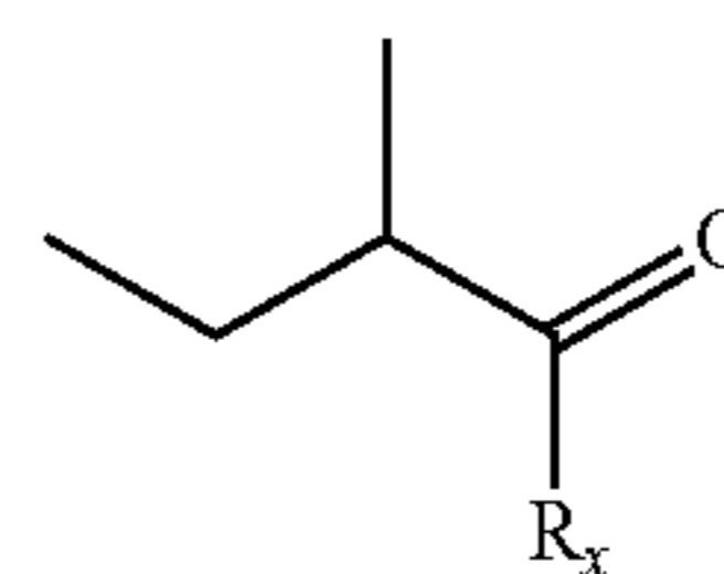
(2-Me-4:Ald)
