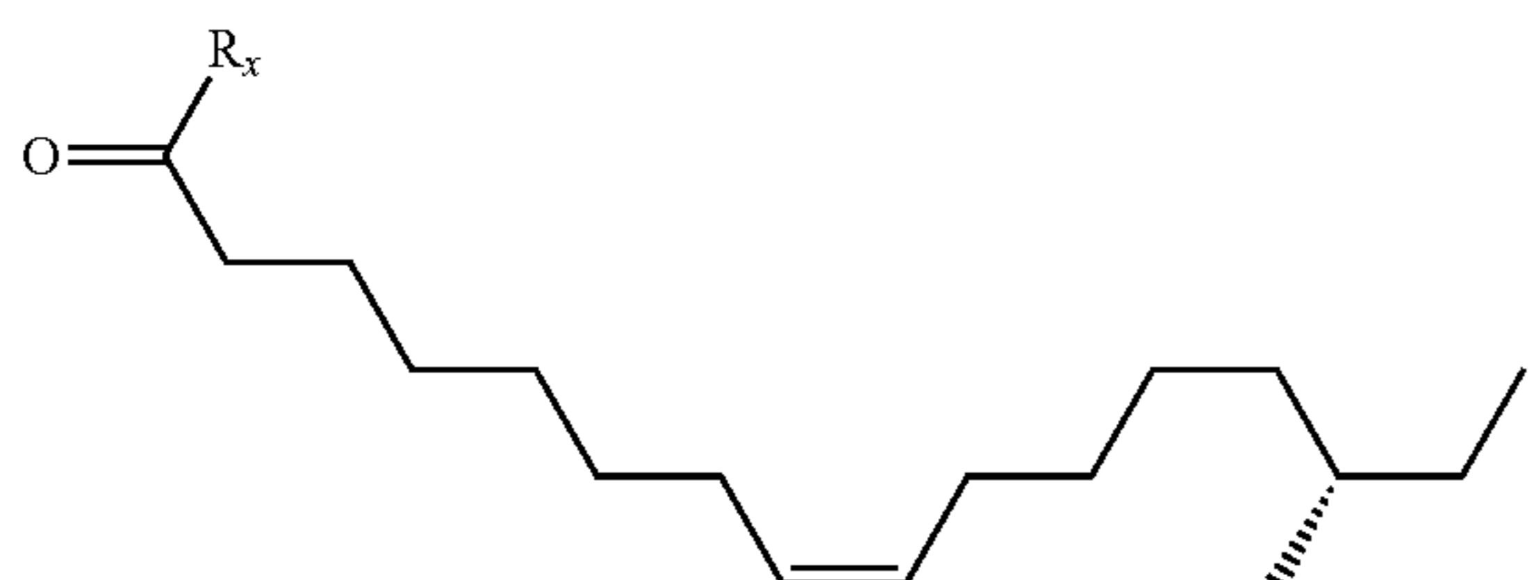
(R,Z-trogodermal)
