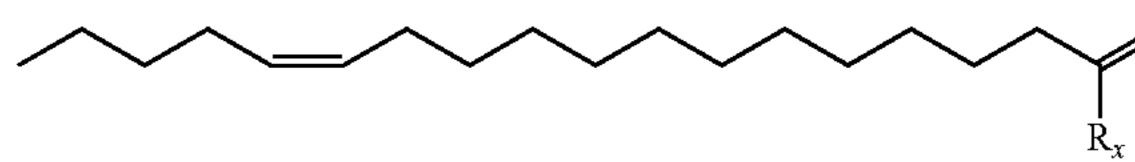
(Z13-18:Ald)
