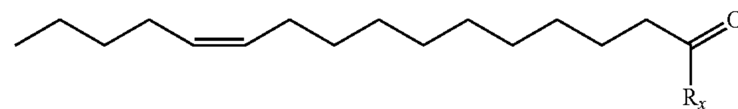
(Z11-16:Ald)
