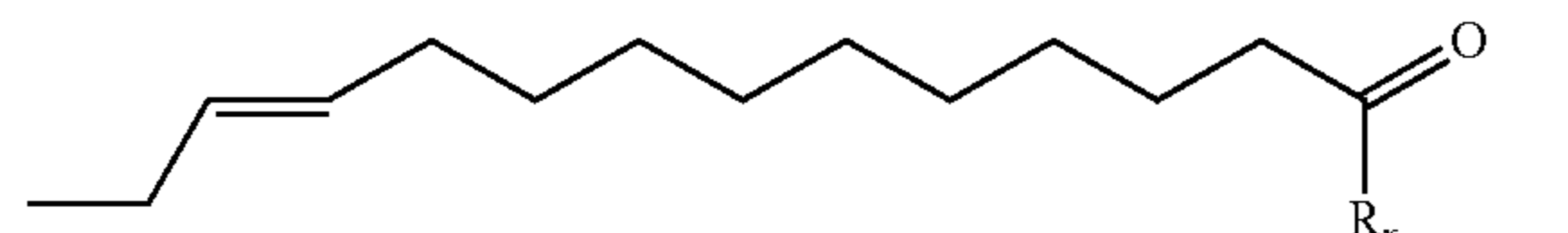
(E11-14:Ald)
