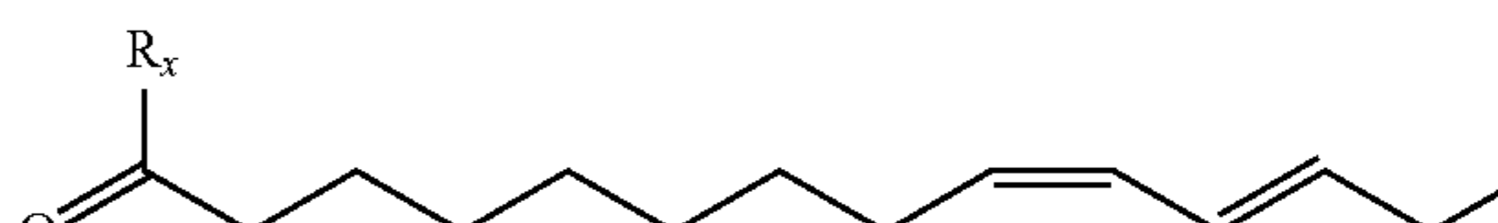
(Z9,E11-14:Ald)
