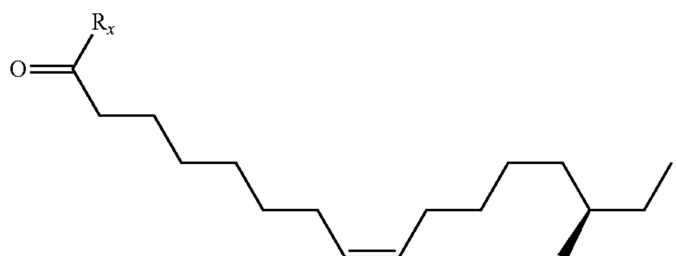
(S,Z-trogodermal)
