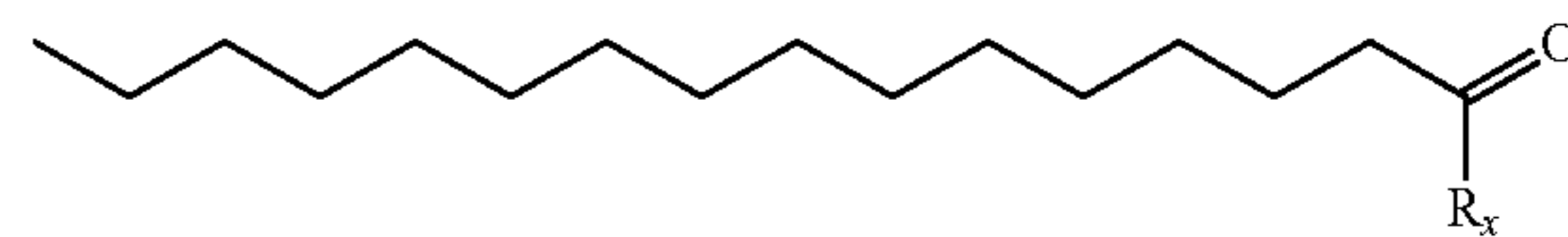
(16:Ald)
