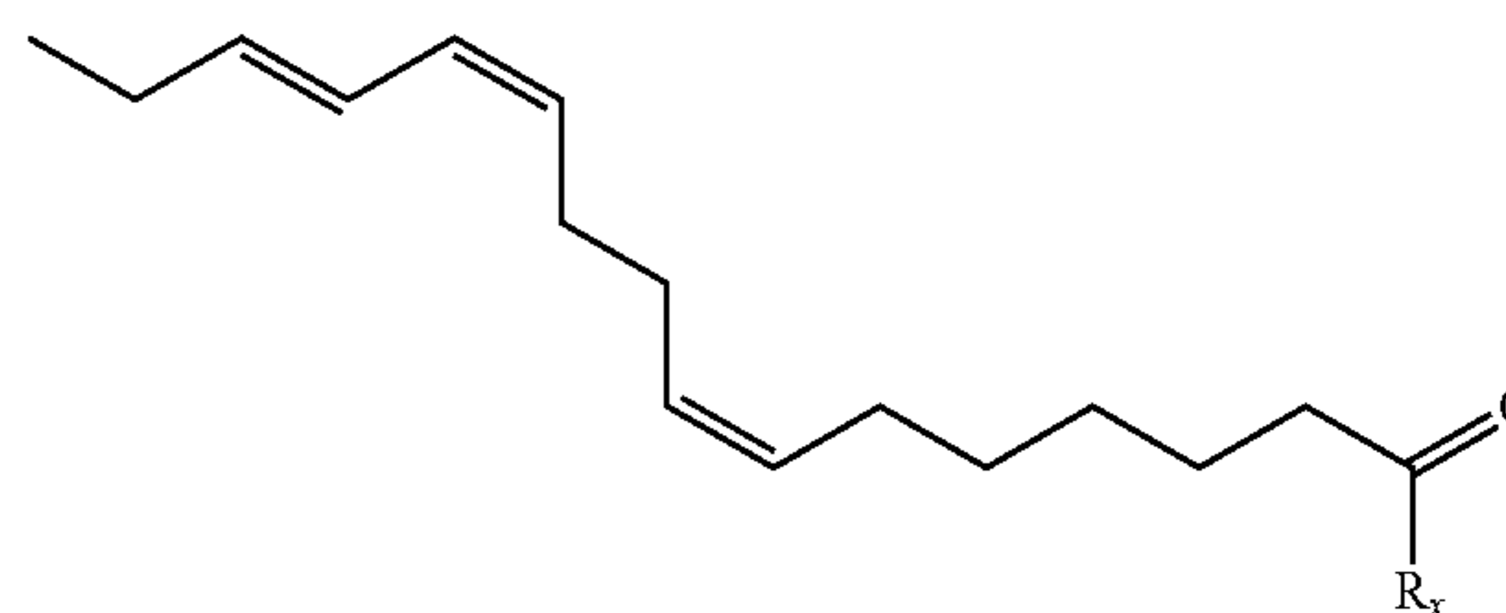
(Z7,Z11,E13-16:Ald)
