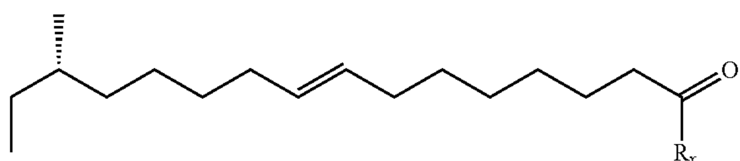
(R,E-trogodermal)
