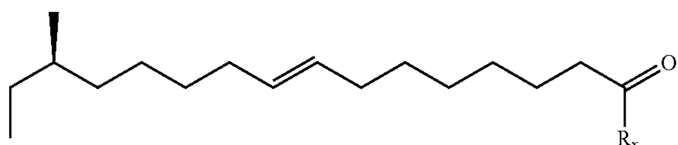
(S,E-trogodermal)
