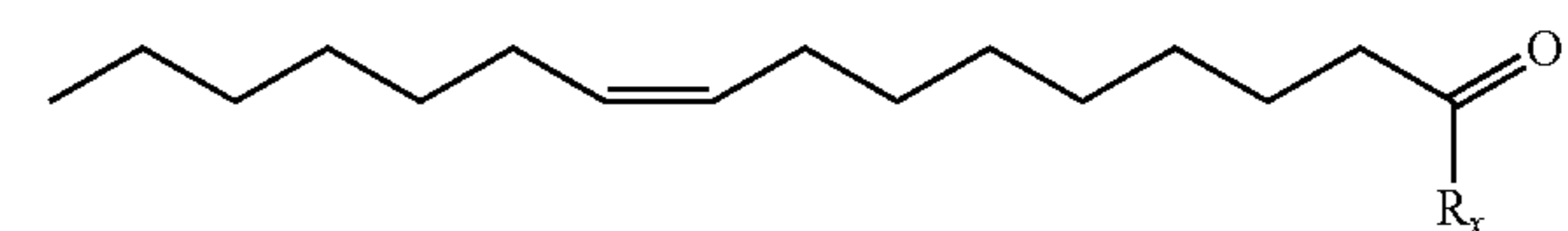
(Z9-16:Ald)
