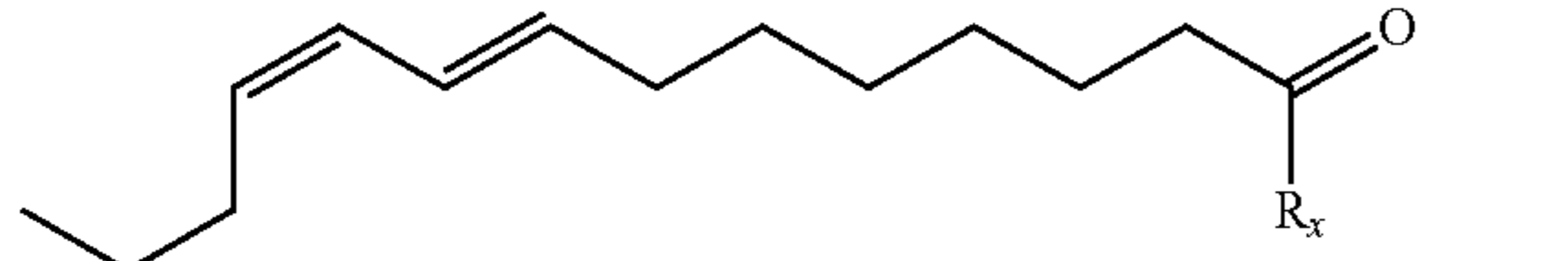
(E8,Z10-14:Ald)
