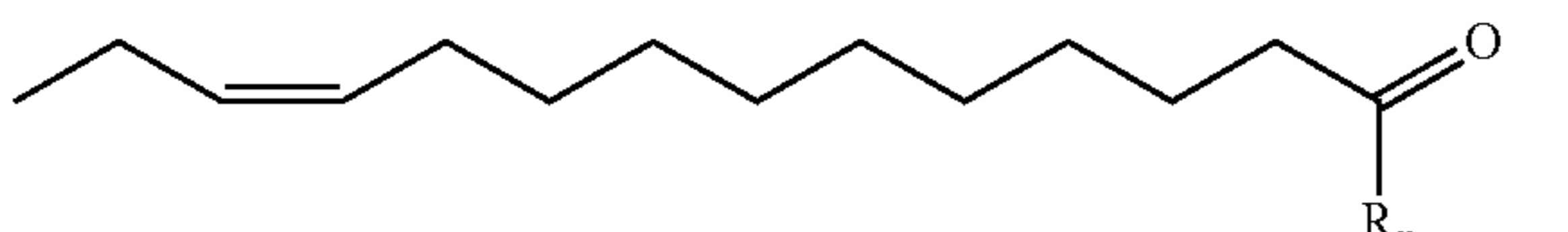
(Z11-14:Ald)
