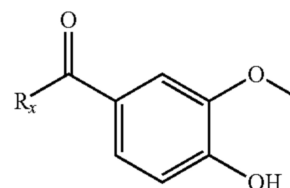
(vanillin)
