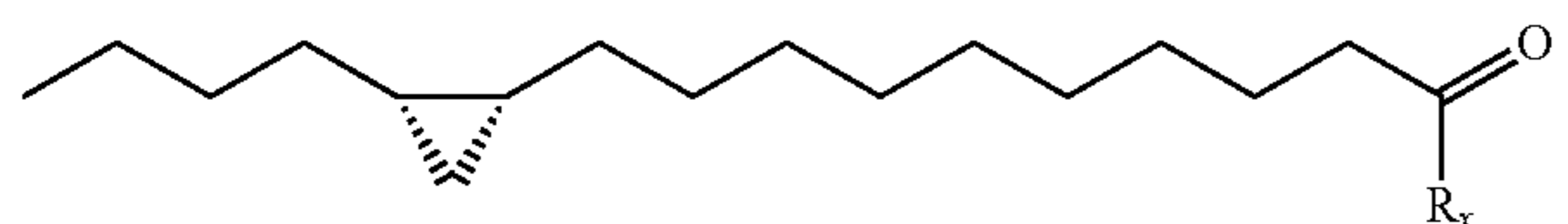
(E10, E12-16:Ald)
