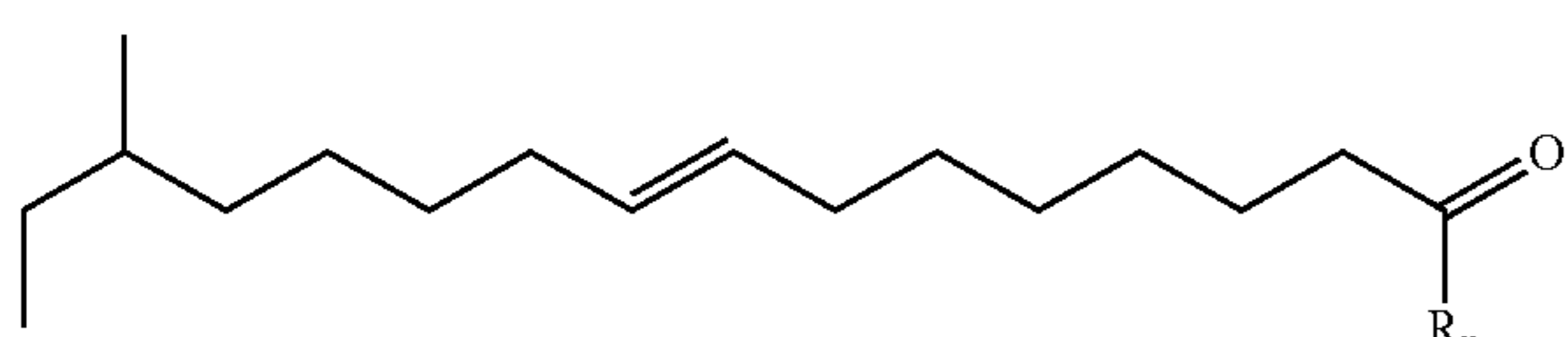
(E-trogodermal)
