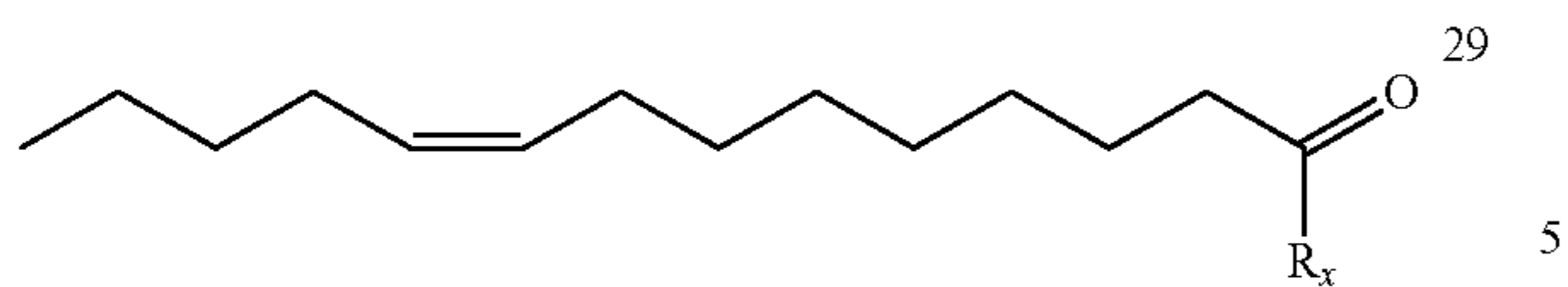
(Z9-14:Ald)
