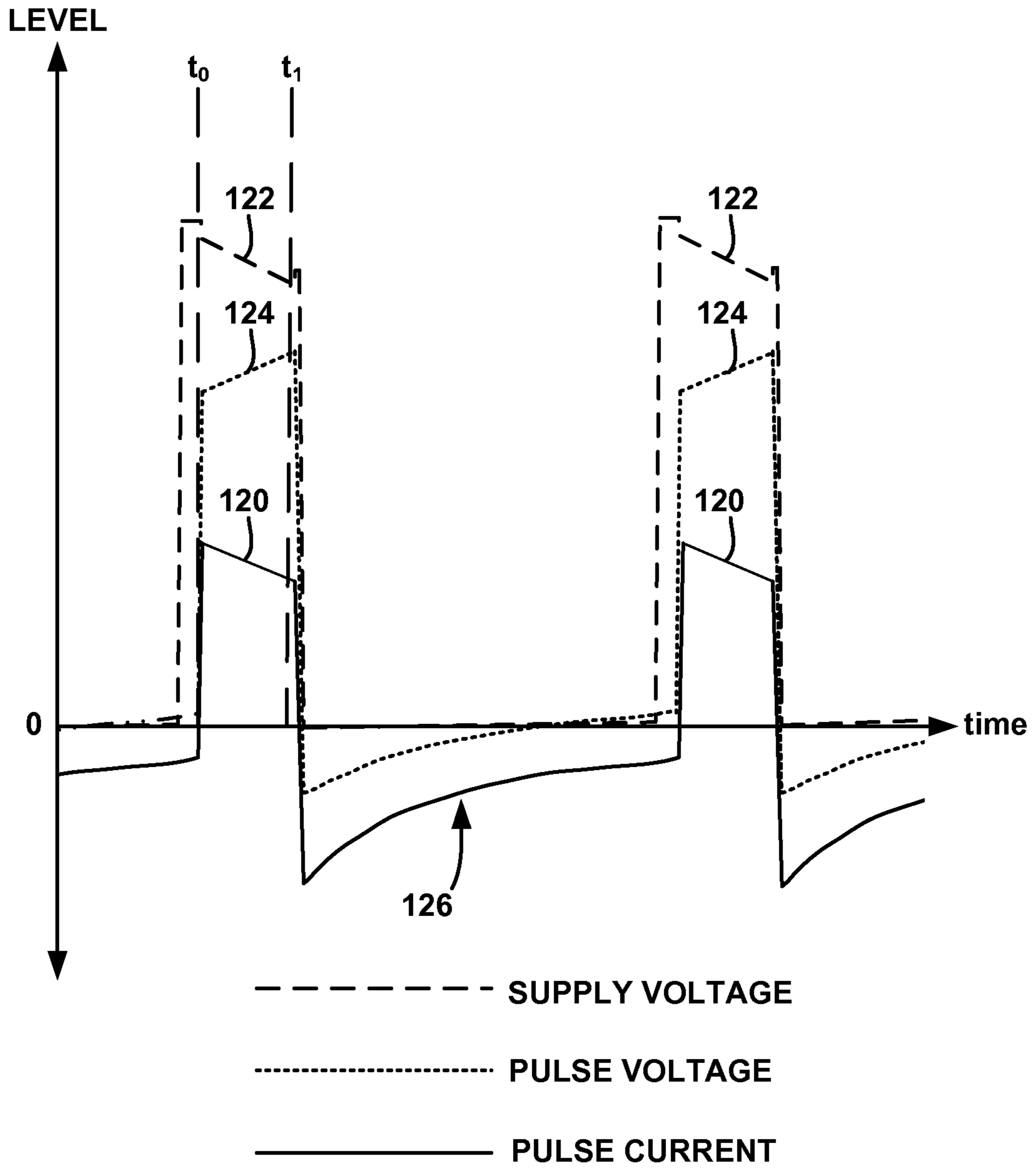
FIG. 7A
