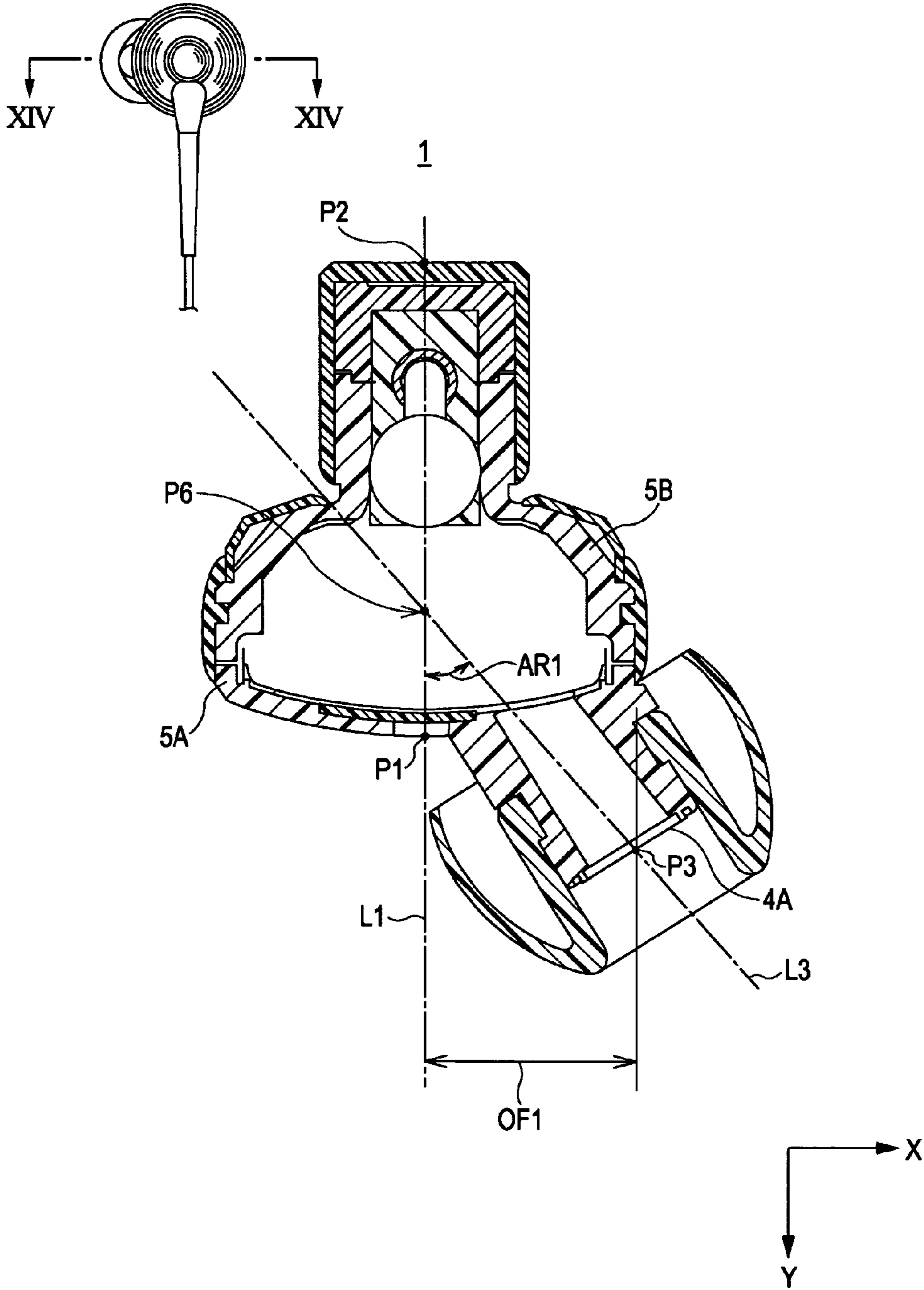
FIG. 14
