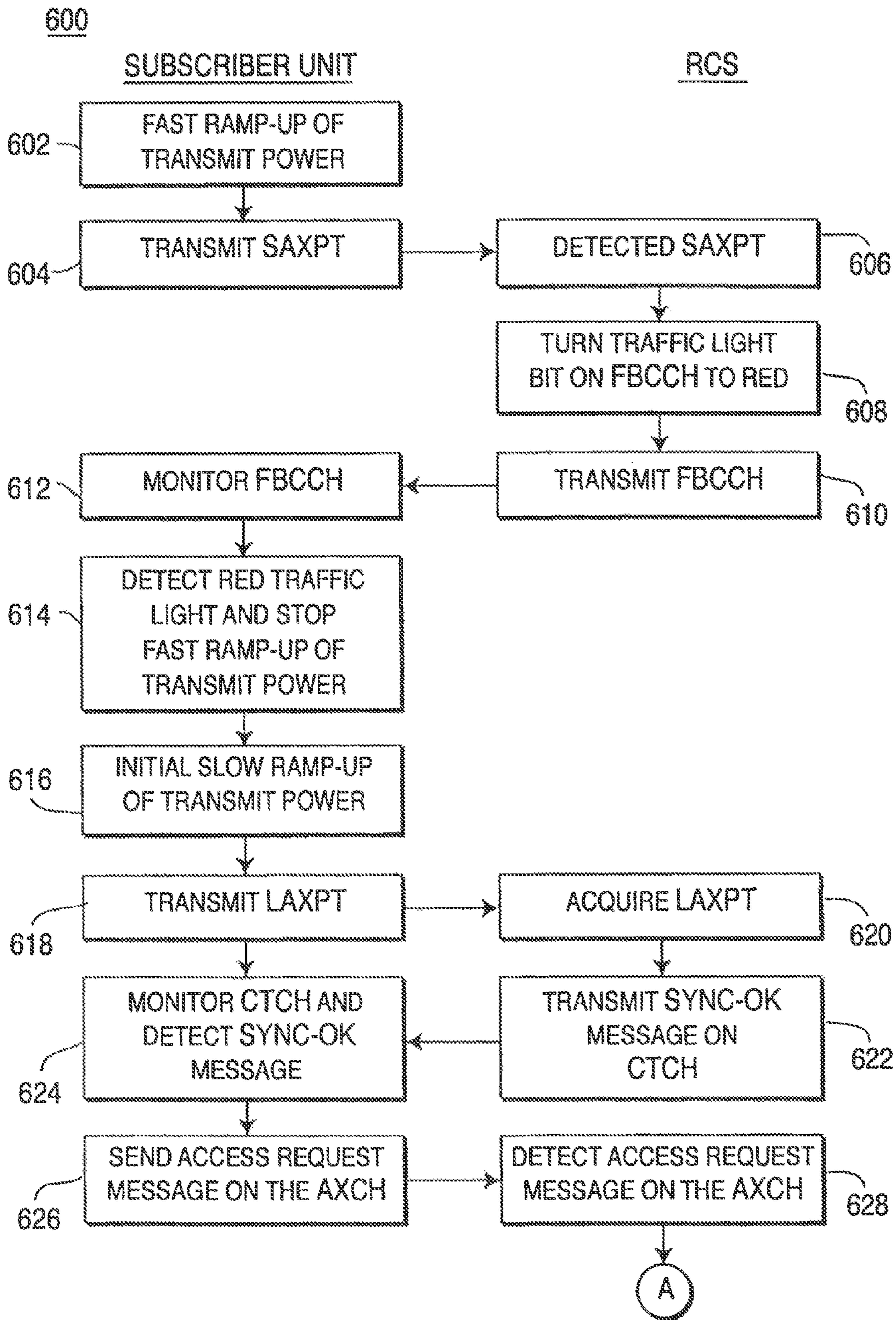
FIG. 6A
