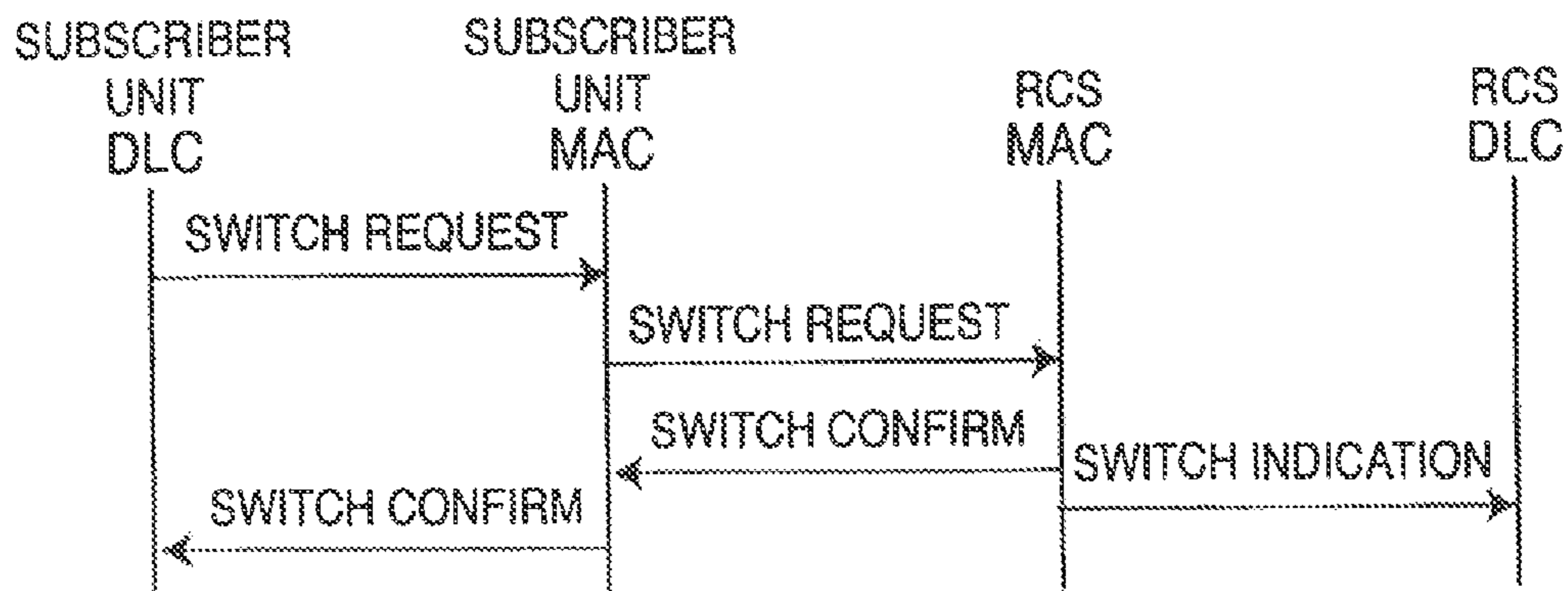
FIG. 8A
