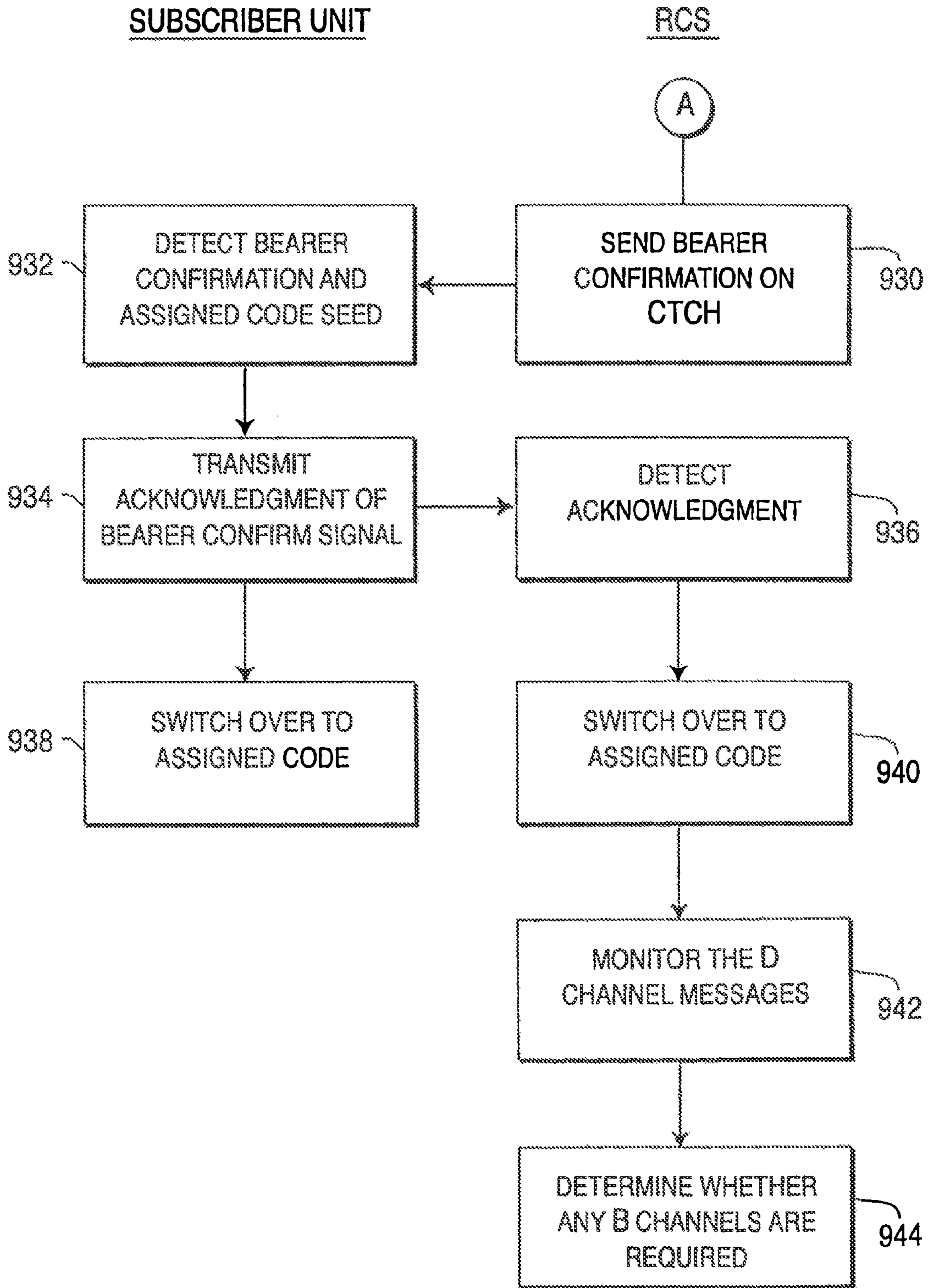
FIG. 9B
