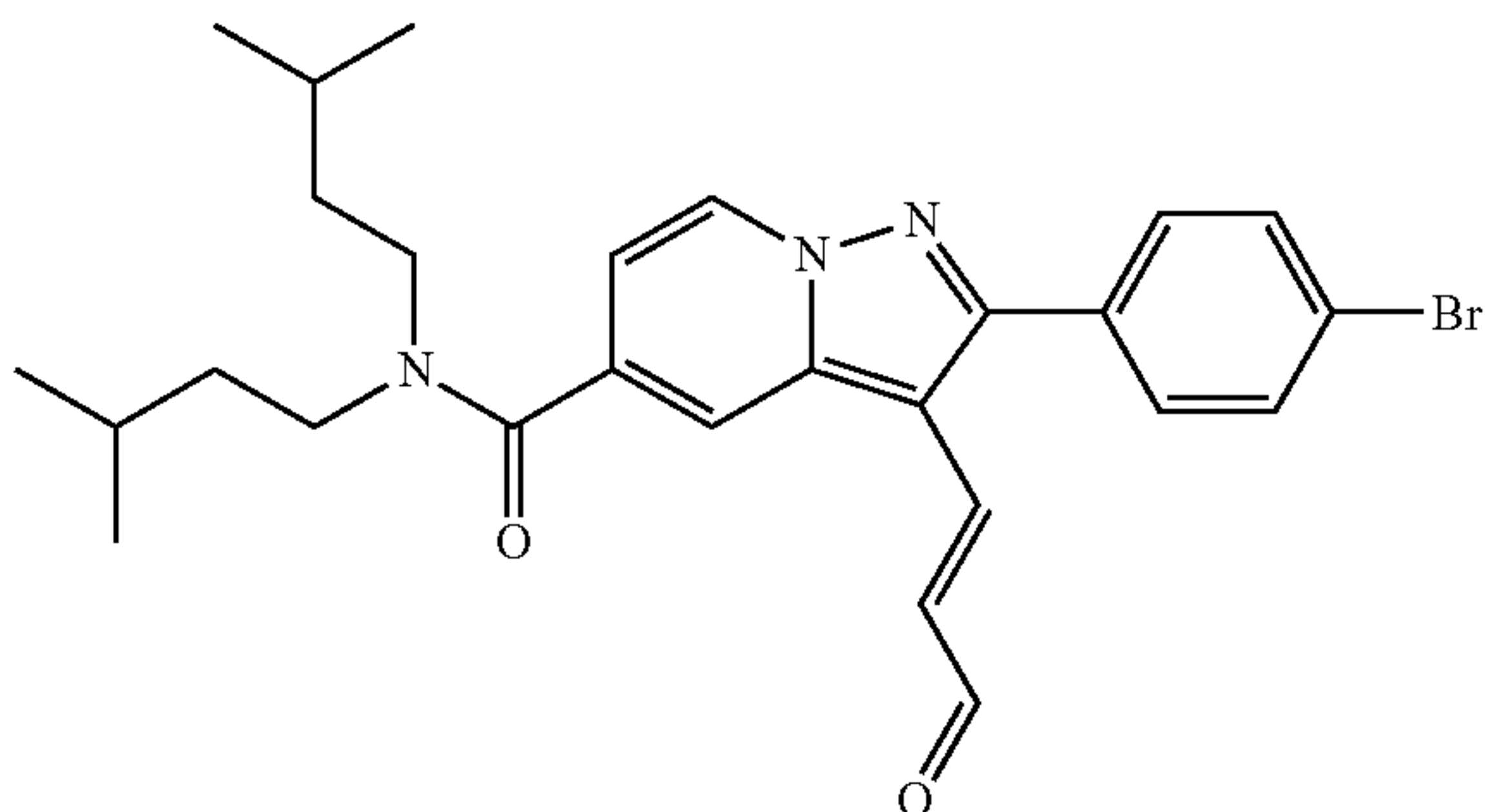
(E)-2-(4-Bromophenyl)-N,N-diisopentyl-3-(3-oxoprop-1-en-1-yl)pyrazolo[1,5-a]pyridine-5-carboxamide
