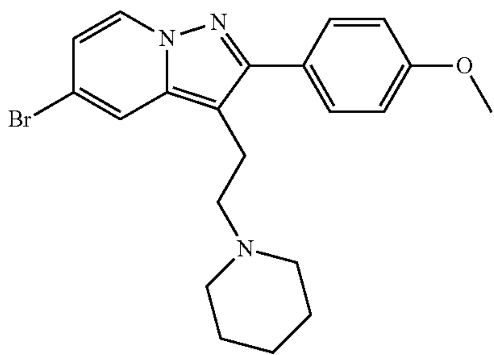
5-bromo-2-(4-methoxyphenyl)-3-(2-(piperidin-1-yl)ethyl)pyrazolo[1,5-a]pyridine
