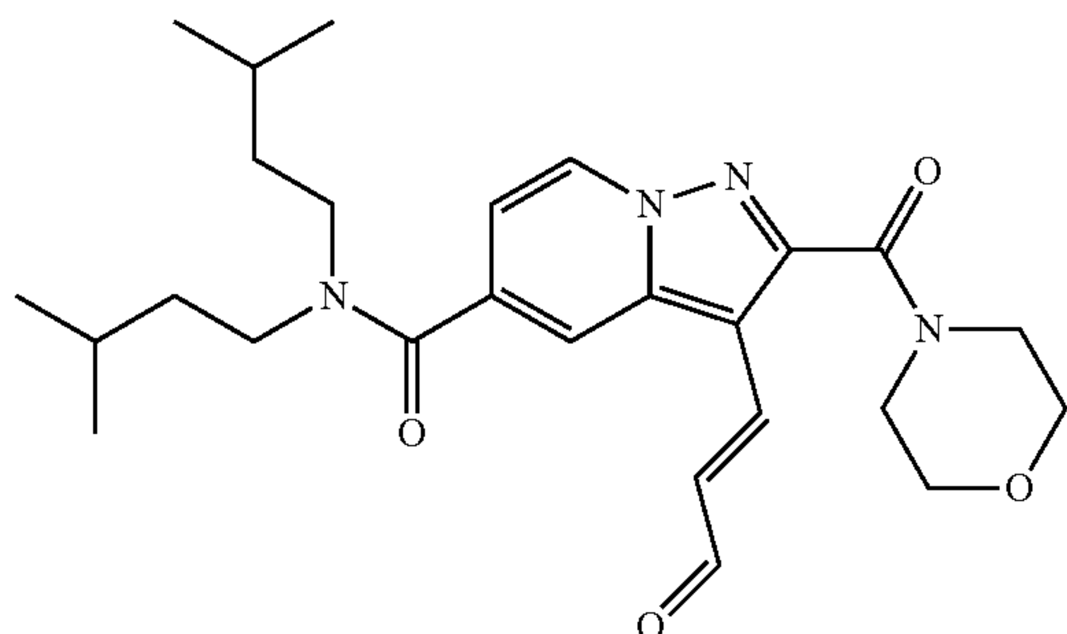
(E)-N,N-diisopentyl-2-(morpholine-4-carbonyl)-3-(3-oxoprop-1-en-1-yl)pyrazolo[1,5-a]pyridine-5-carboxamide
