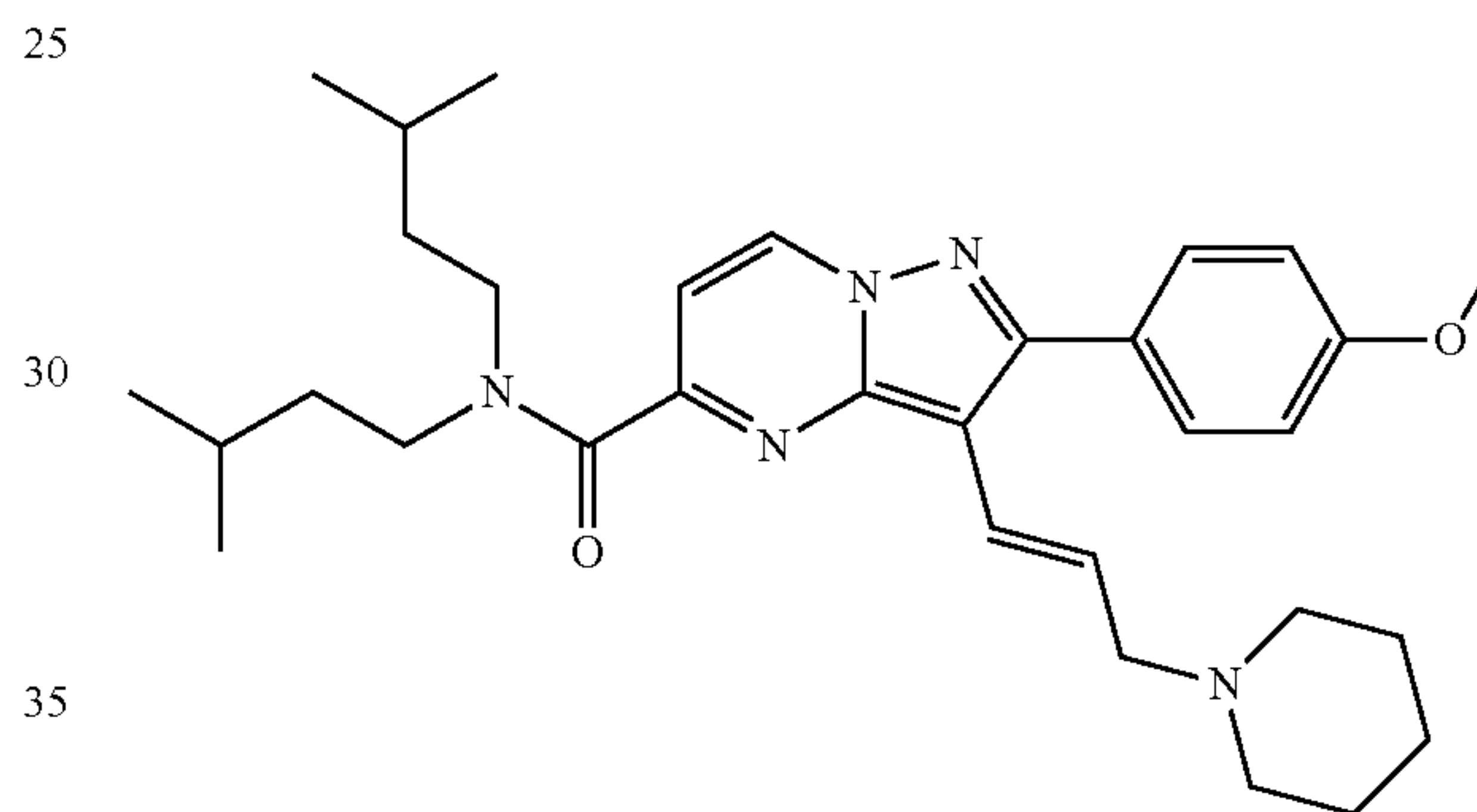
(E)-N,N-Diisopentyl-2-(4-methoxyphenyl)-3-(3-(piperidin-1-yl)prop-1-en-1-yl)pyrazolo[1,5-a]pyrimidine-5-carboxamide
