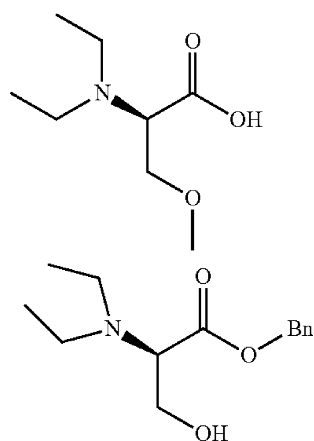
Cap-75, step a
