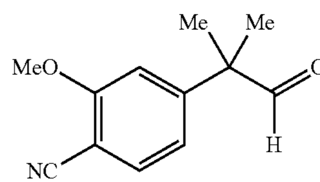
4-(1,1-dimethyl-2-oxoethyl)-2-(methoxy)benzointrile
