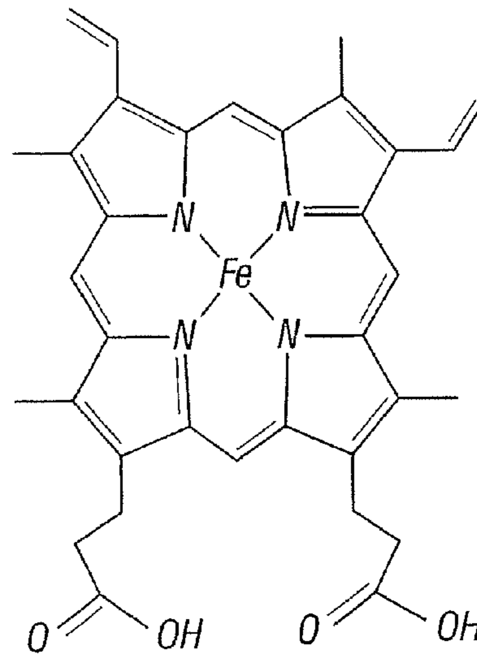
Haem b (C00032) Protoporphyrin IX
