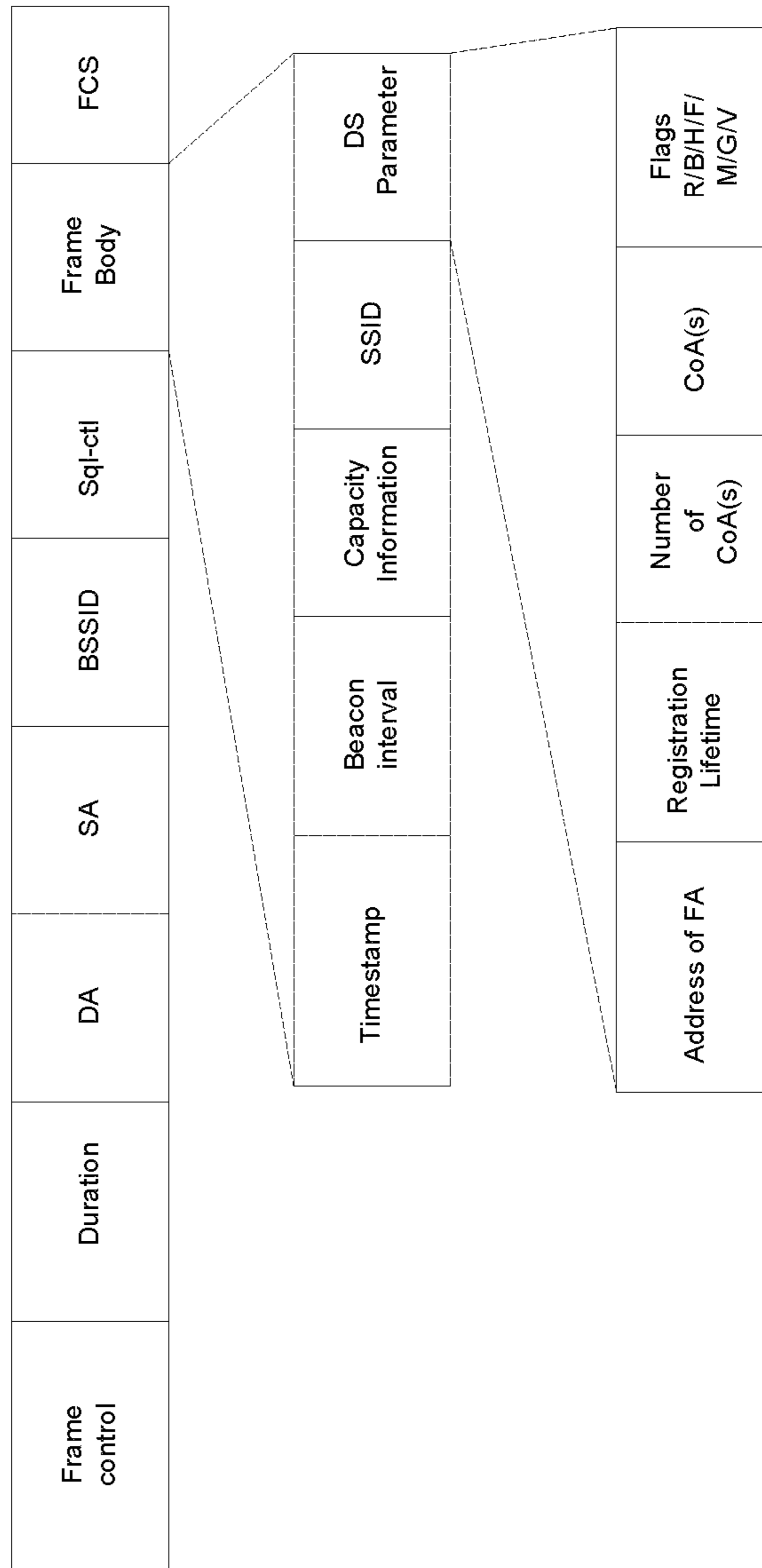
FIG. 4A
