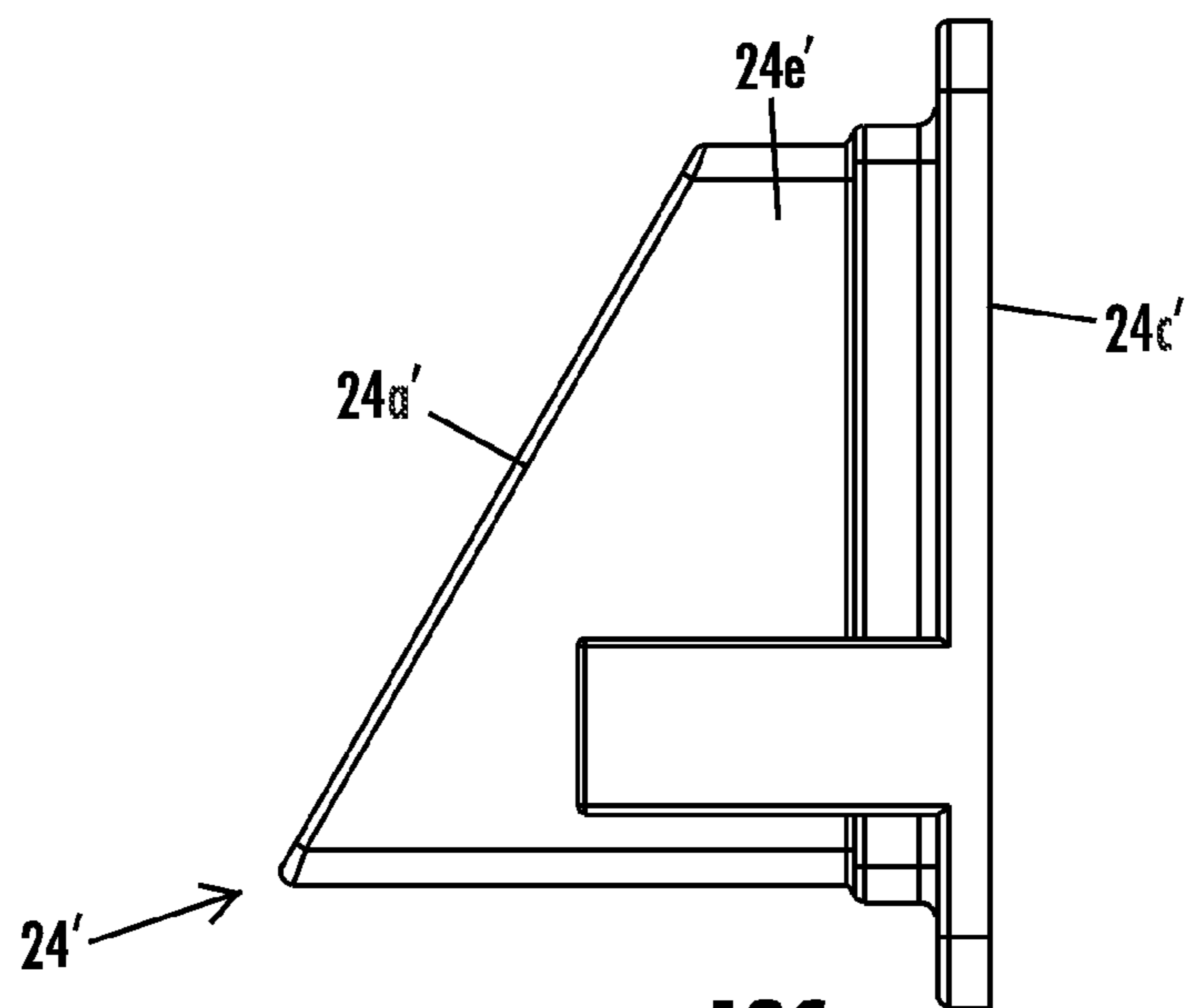
FIG. 12C
