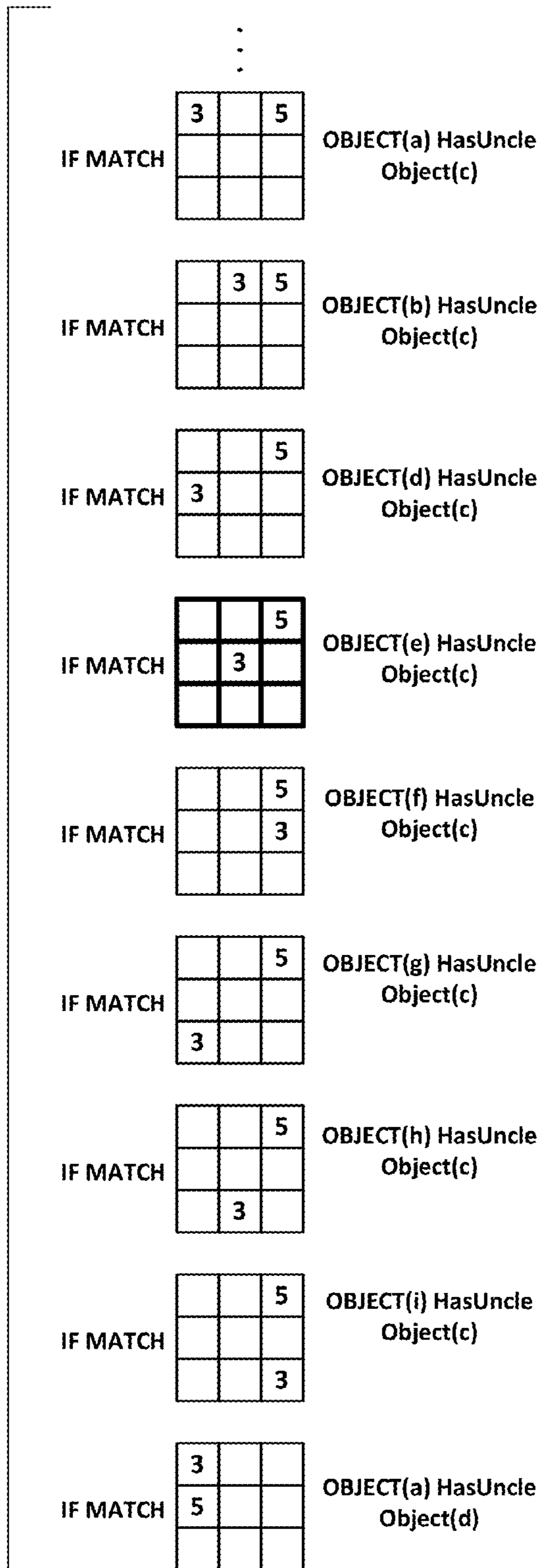
FIG. 26 – PREDICATE TEMPLATES
