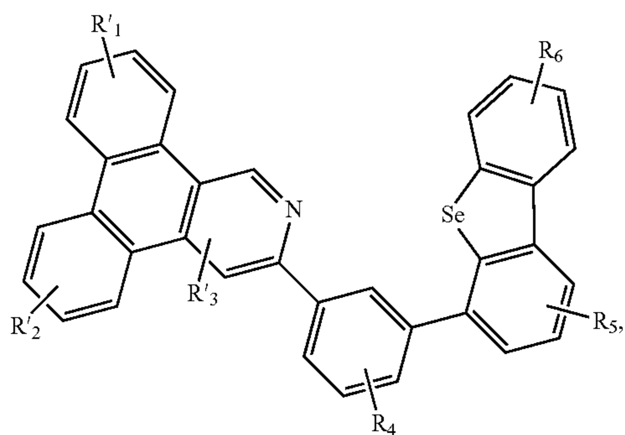
Compound 6G
