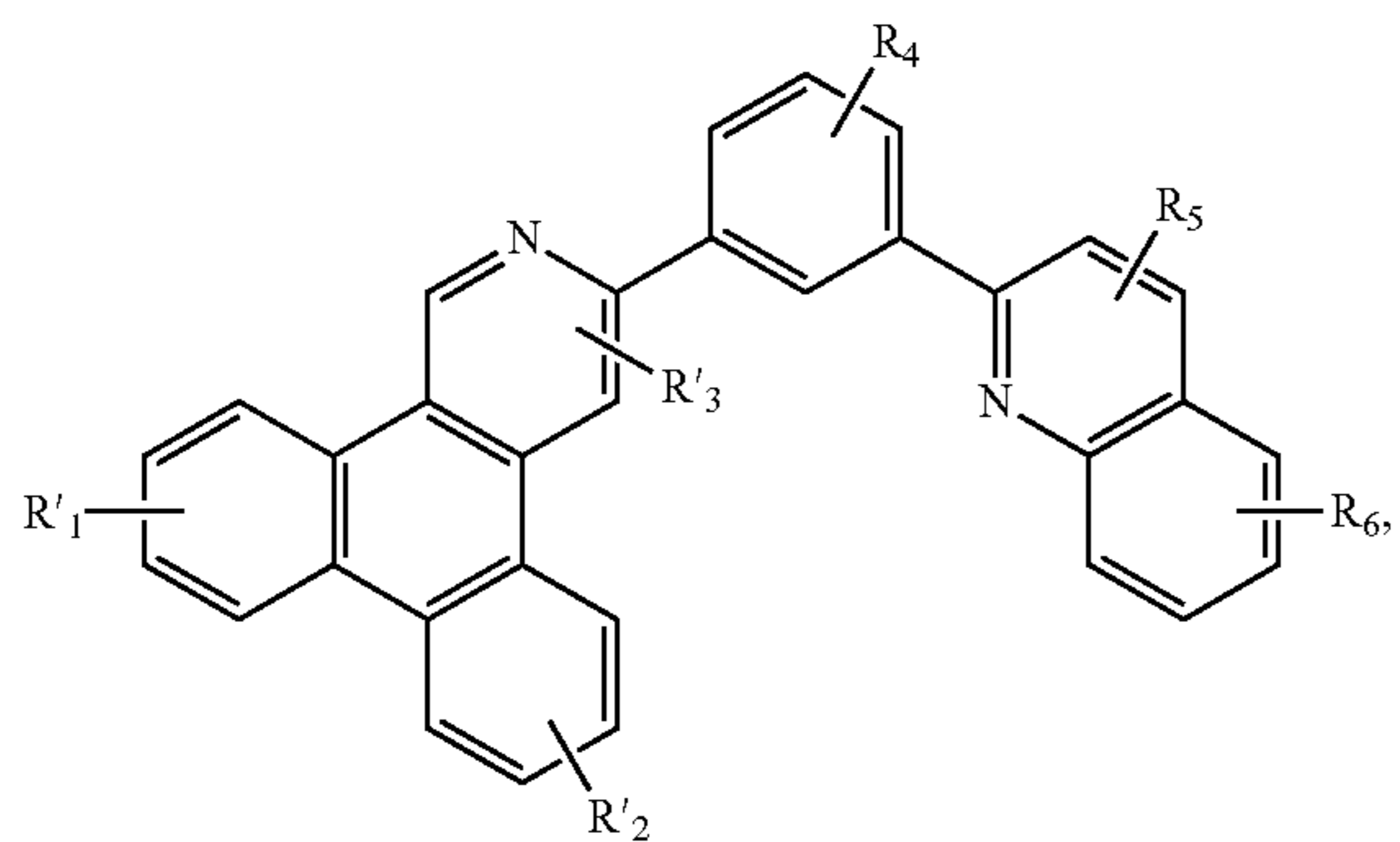
Compound 6G
