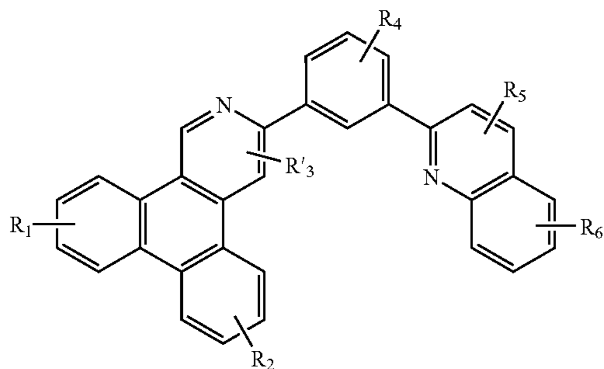
Compound 6G
