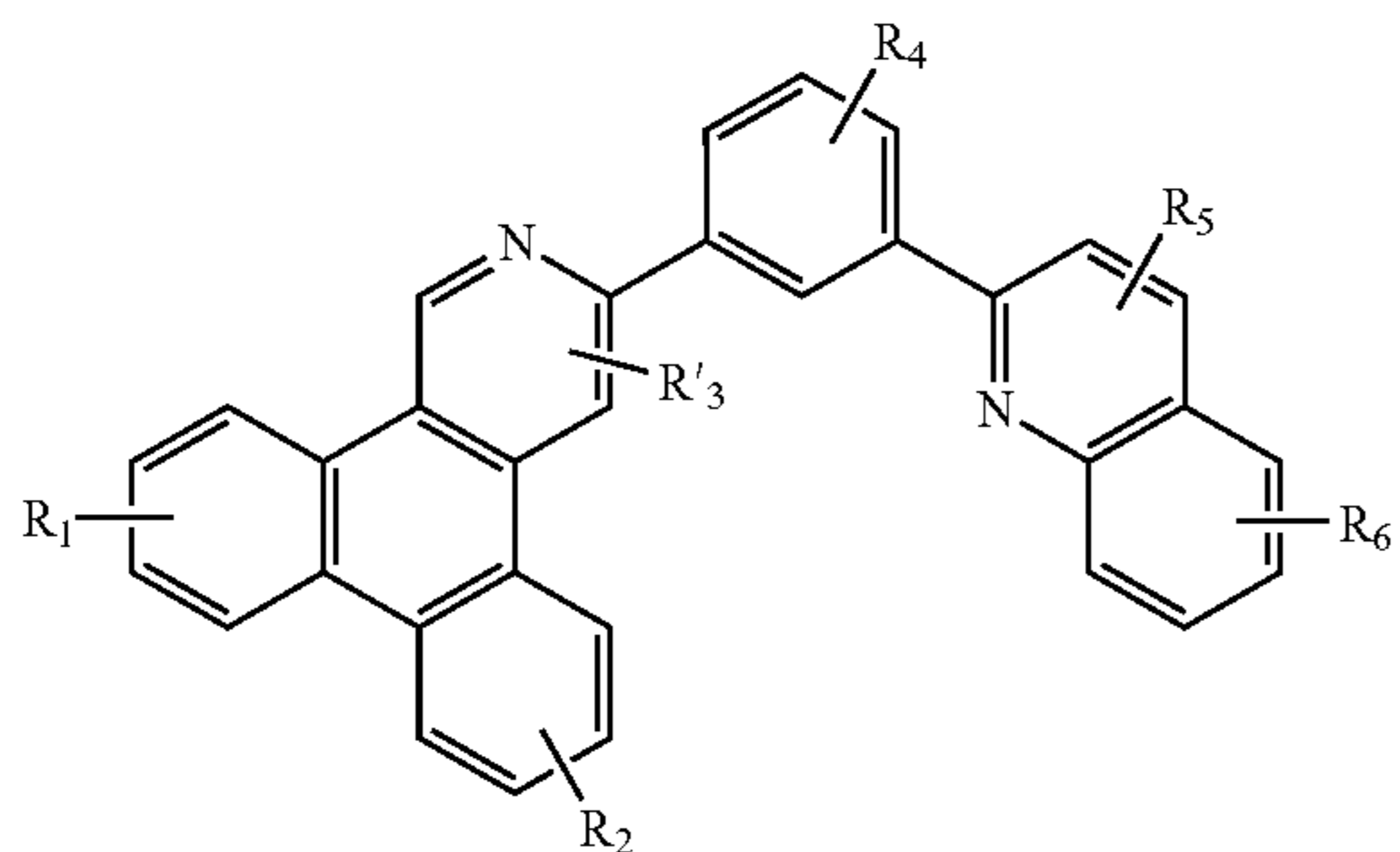
Compound 6G
