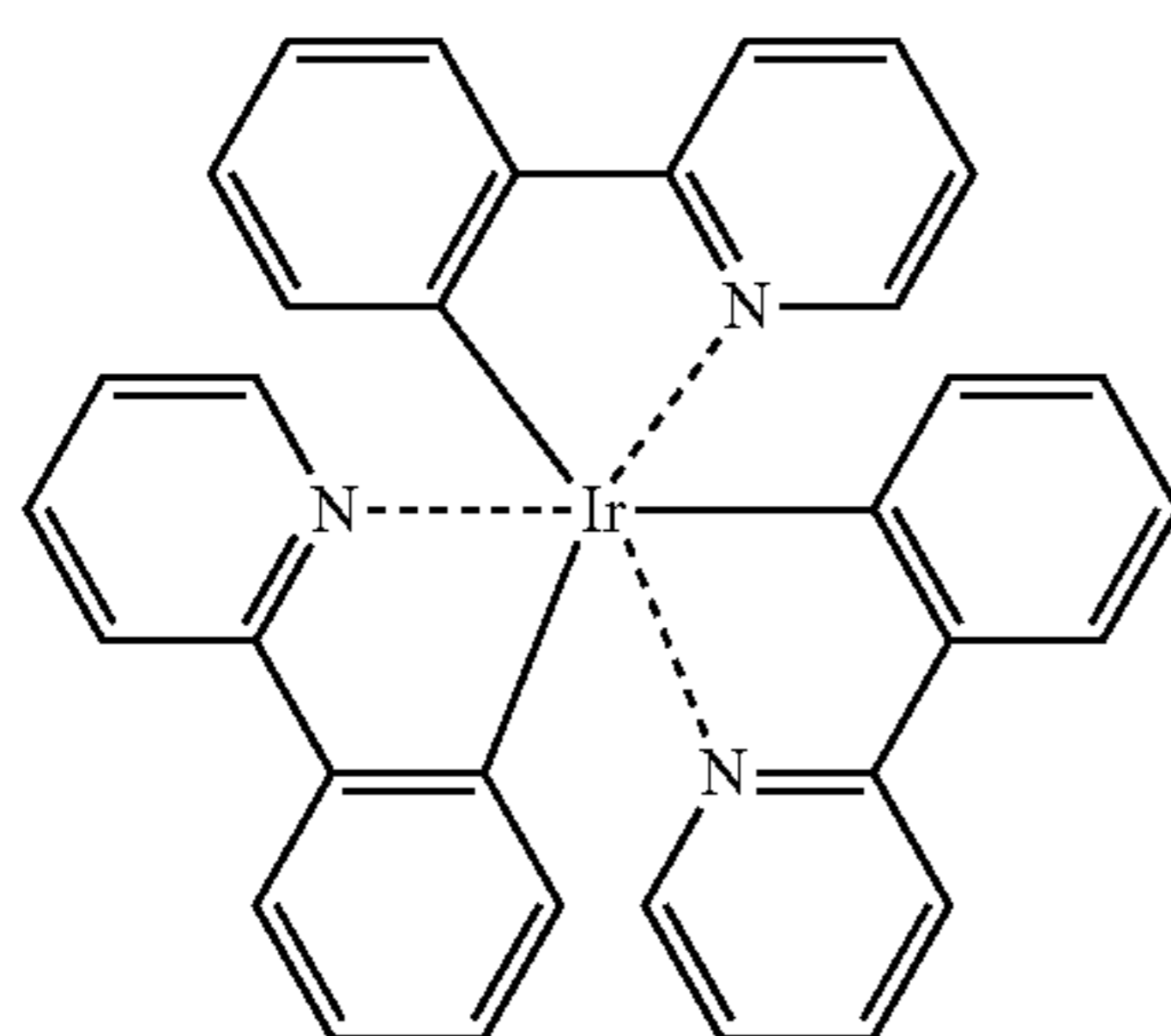
Ir(ppy) 3
