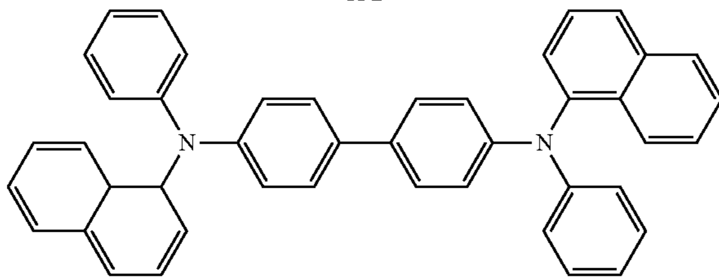
\alpha -NPD
