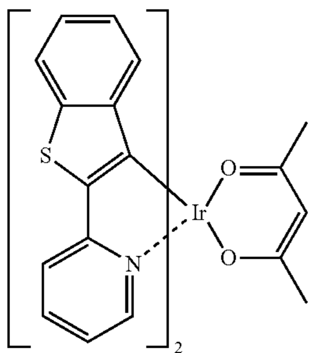
Btp 2 Ir(acac)
