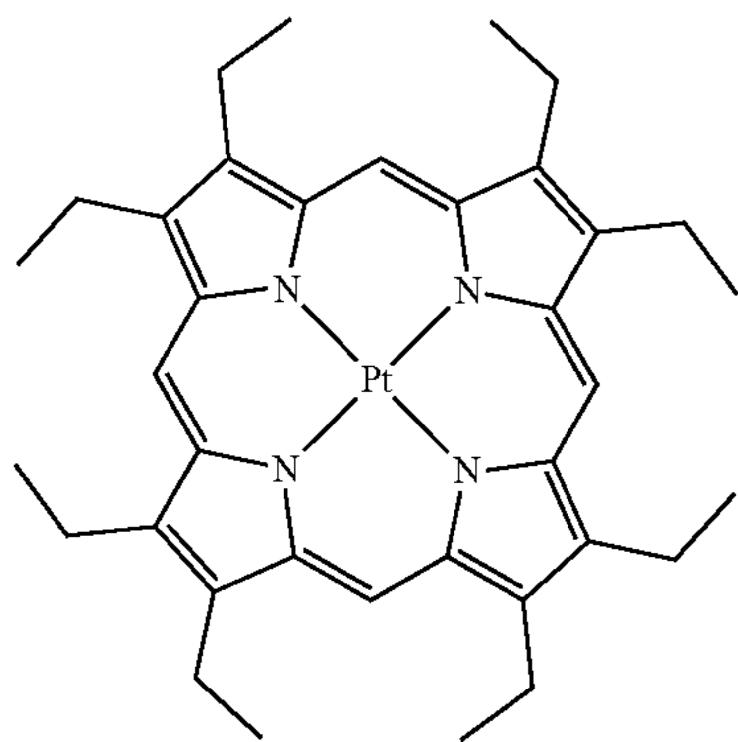
PtOEP
