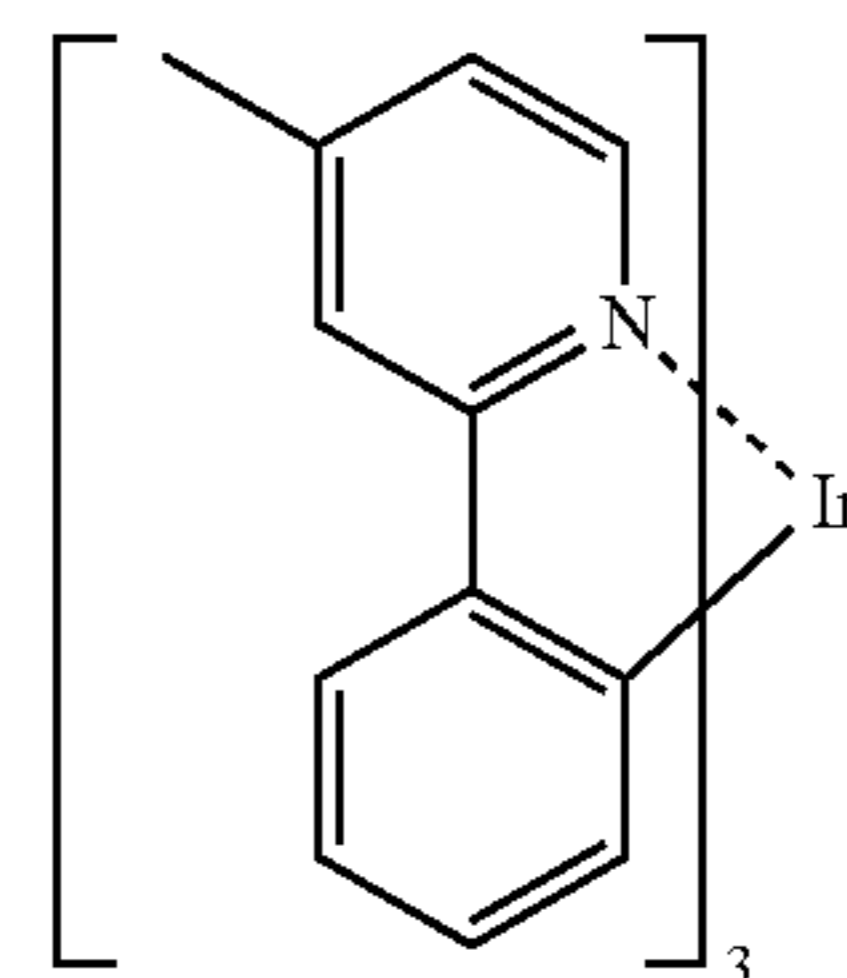
Ir(mpyp) 3
