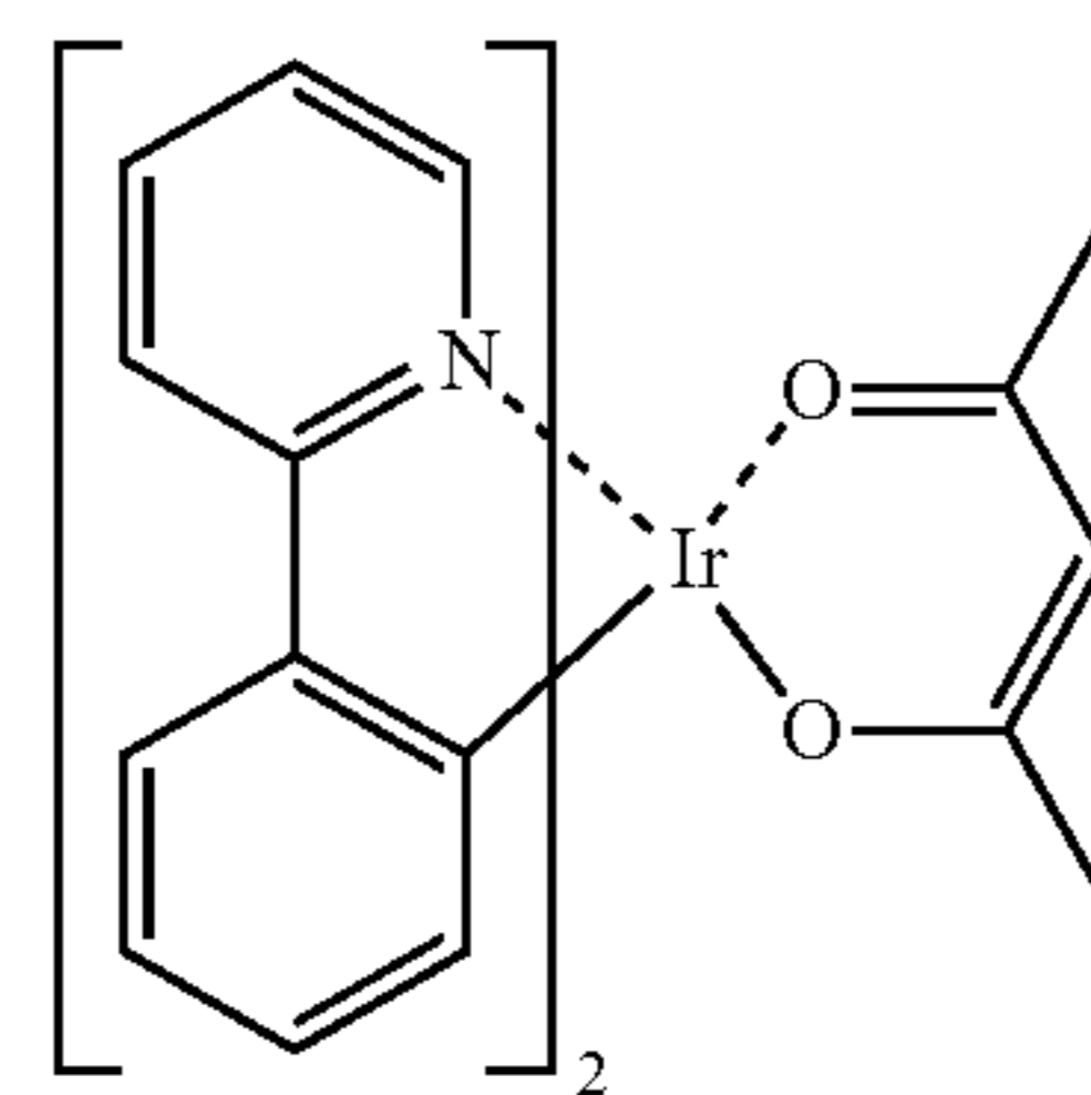
Ir(ppy) 2 (acac)
