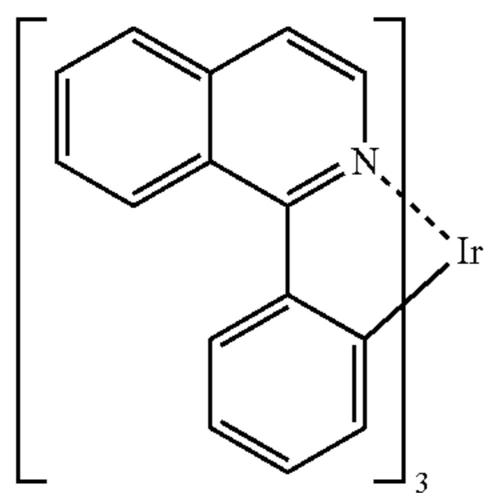
Ir(piq) 3
