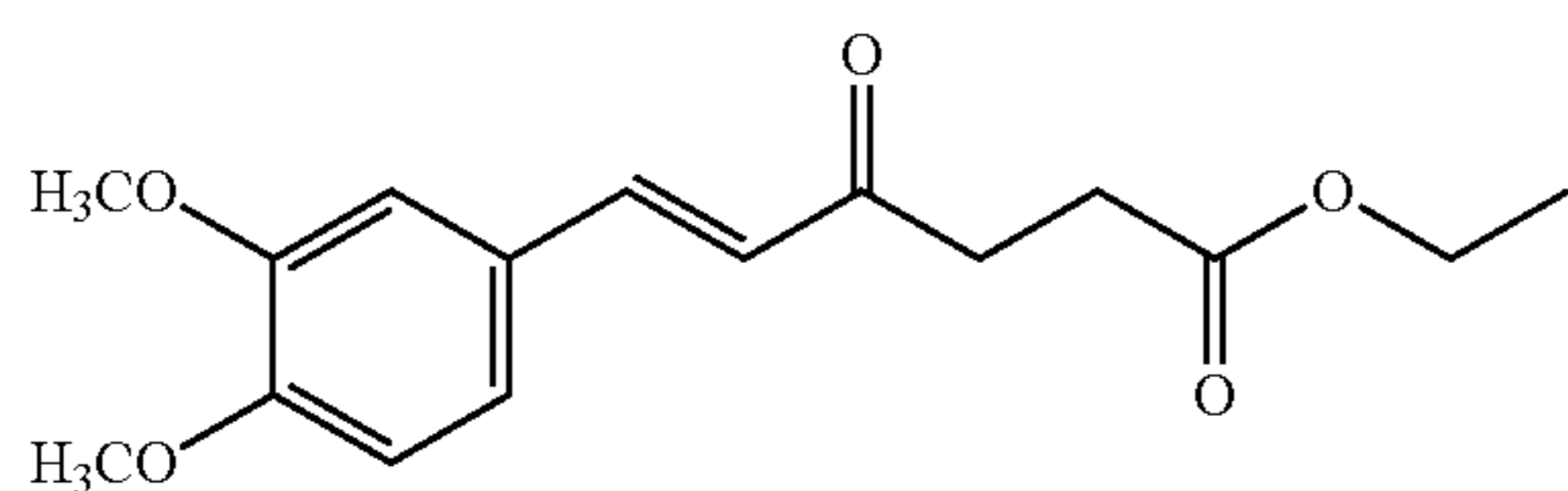
Monomer-6
