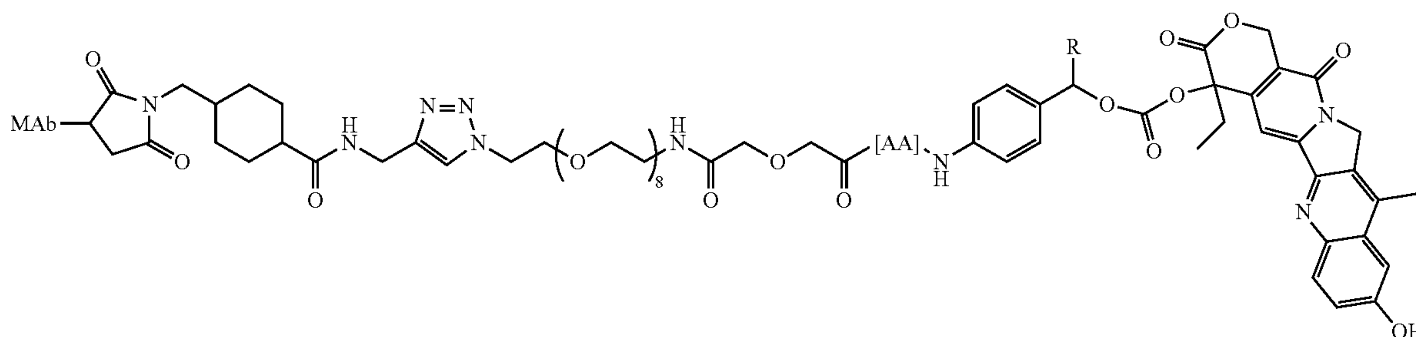
MAb-CLX-SN-38
