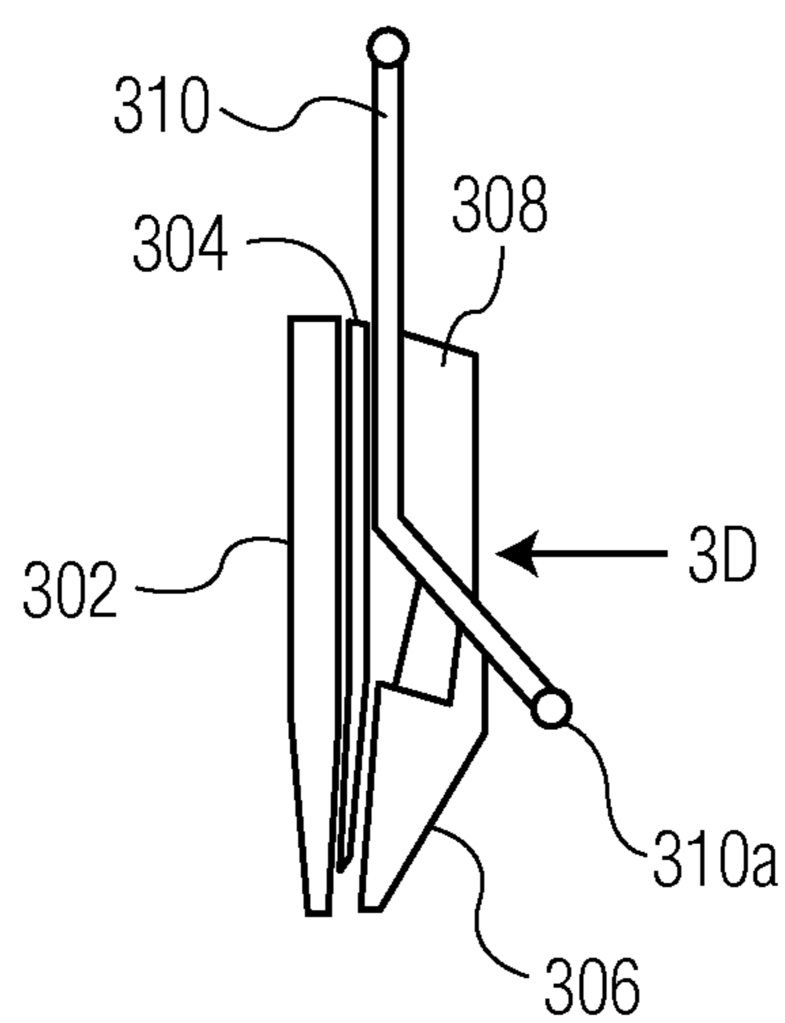
FIG. 3C
