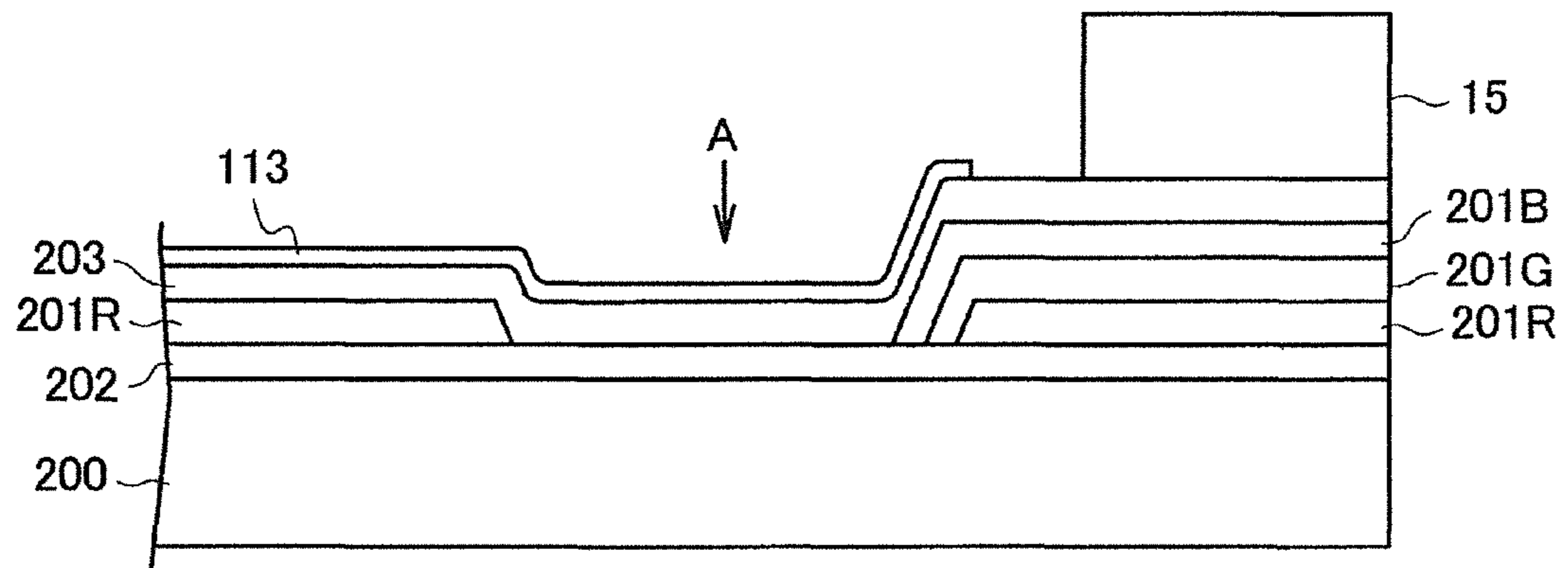
FIG. 10
