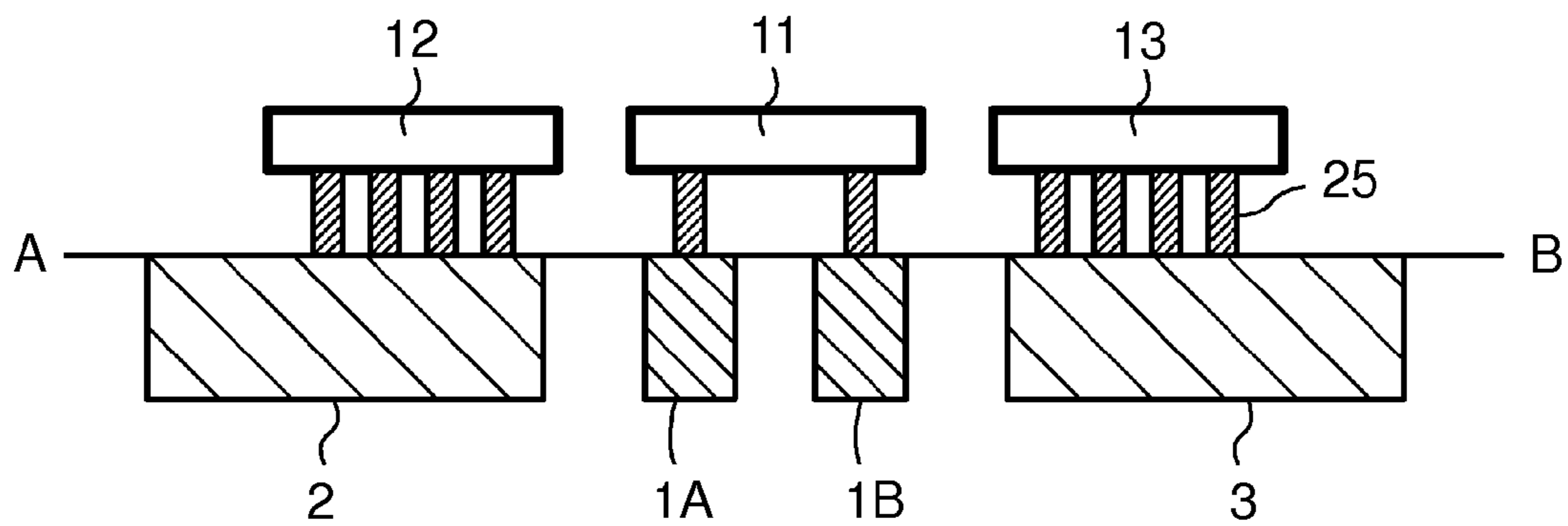
FIG. 8B
