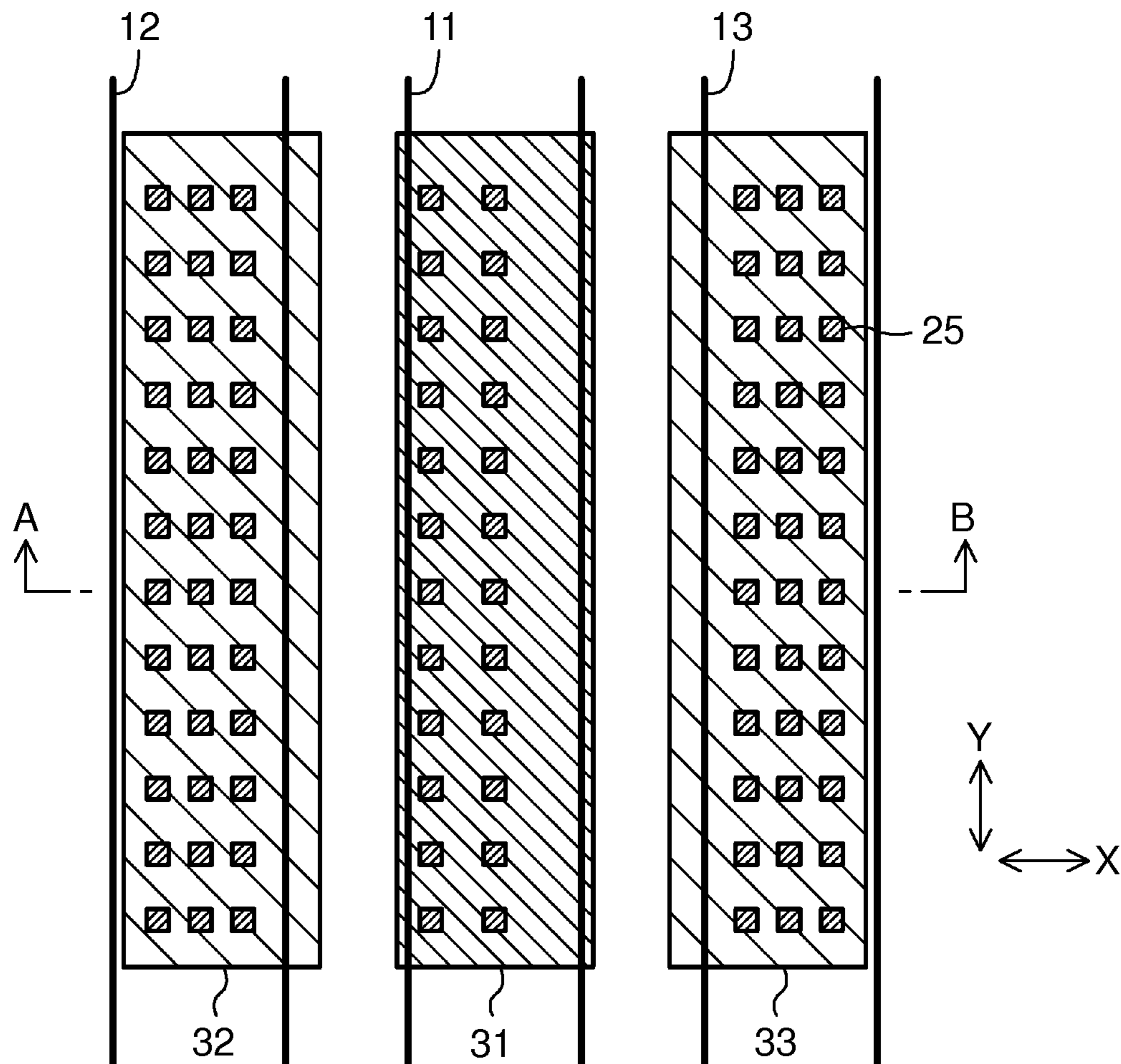
FIG. 13A
