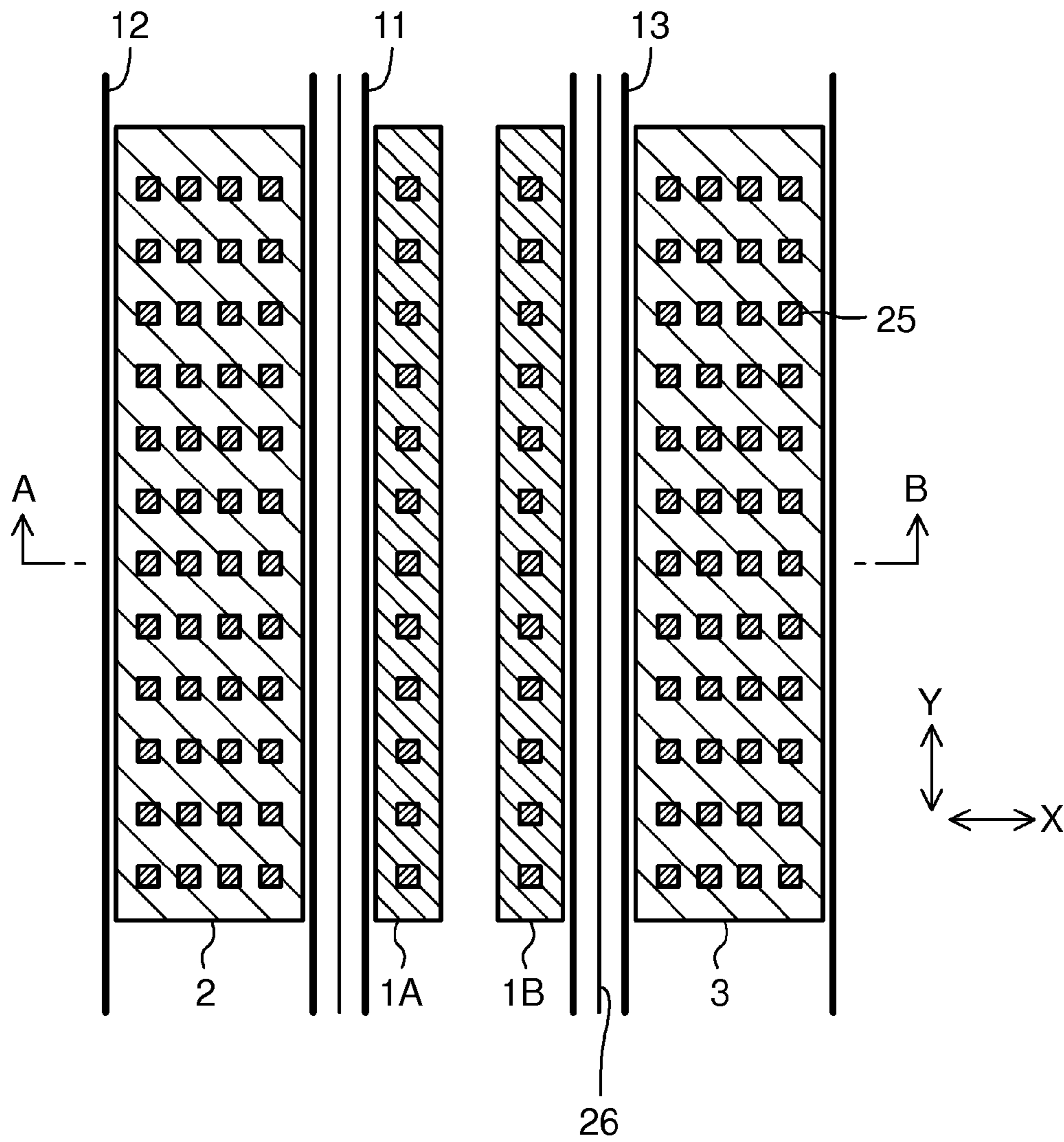
FIG. 4A
