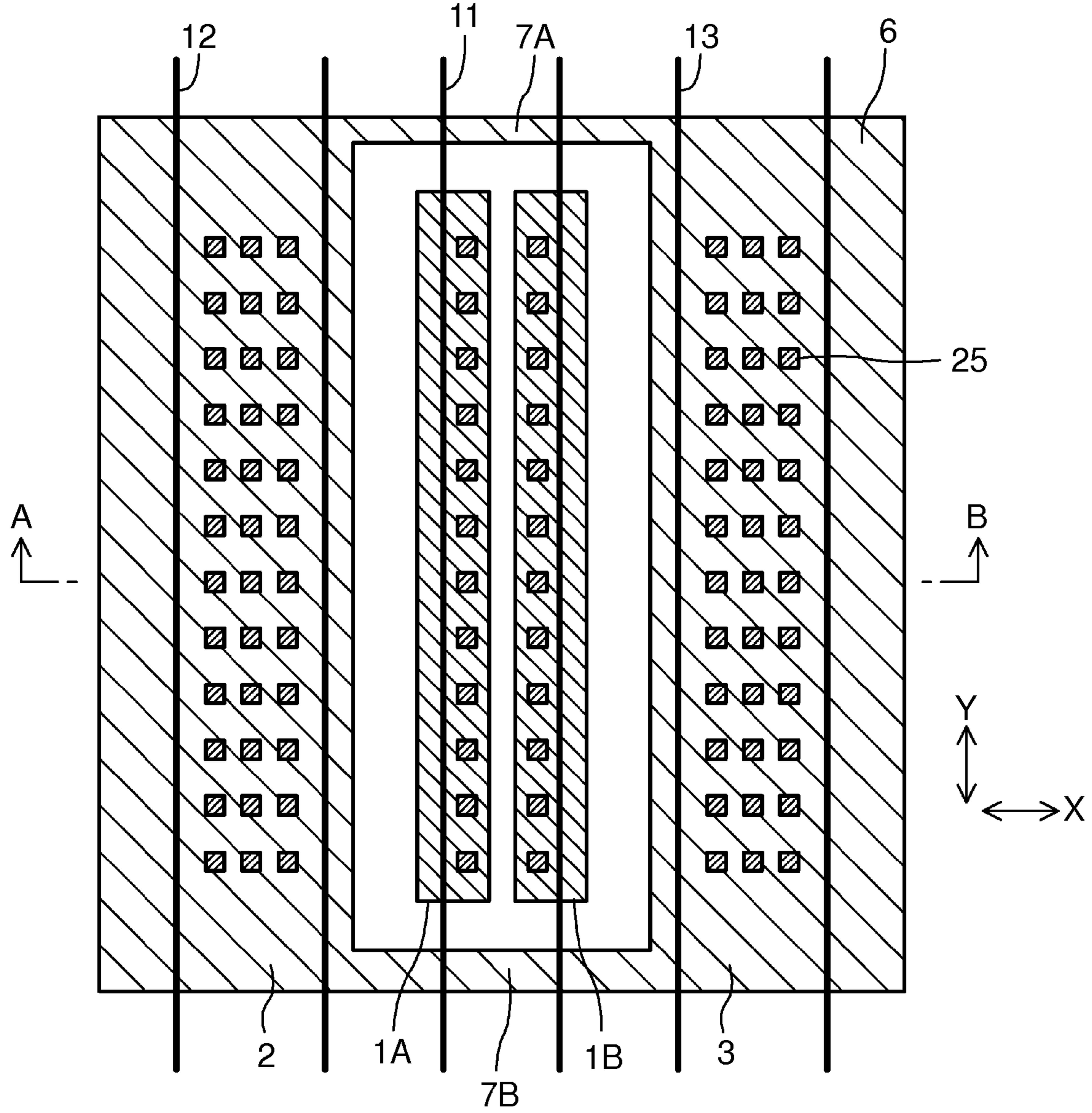
FIG. 9A
