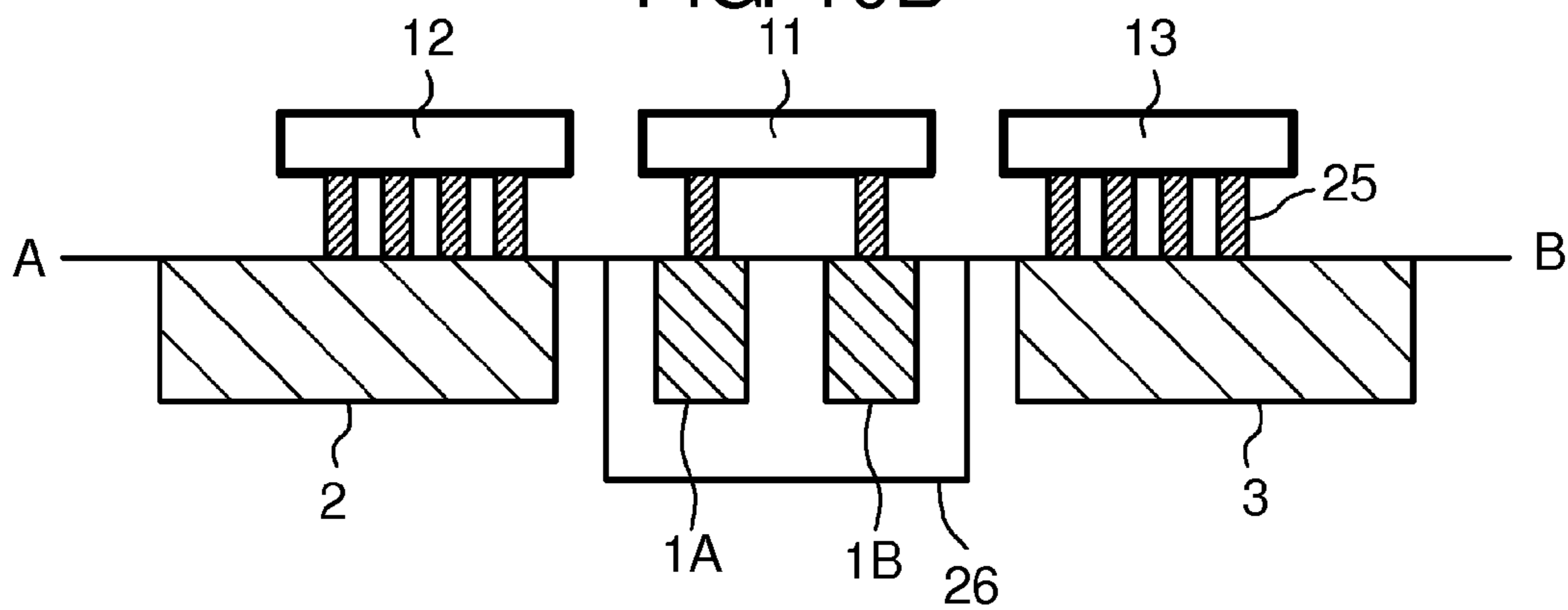
FIG. 10B
