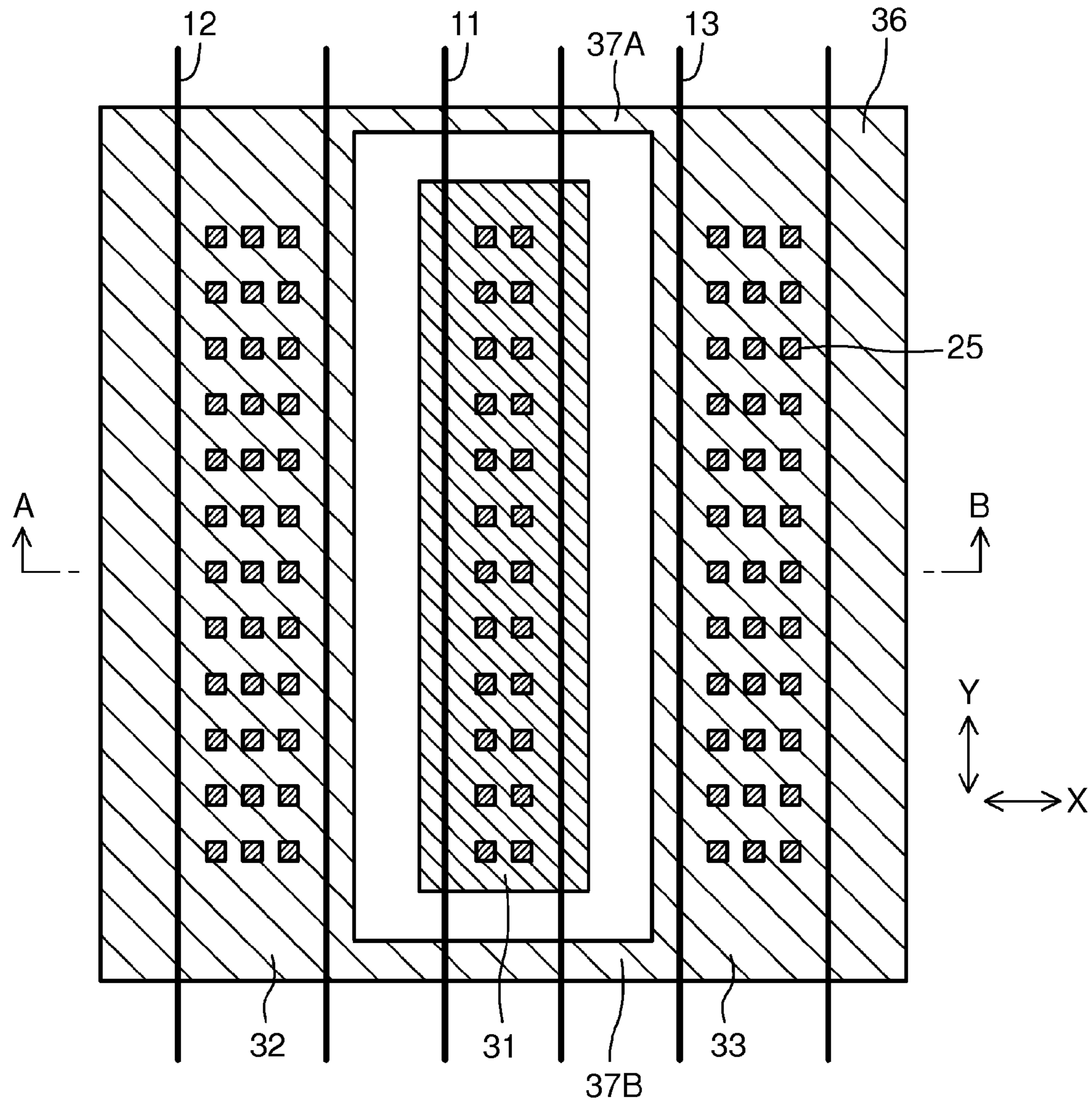
FIG. 14A
