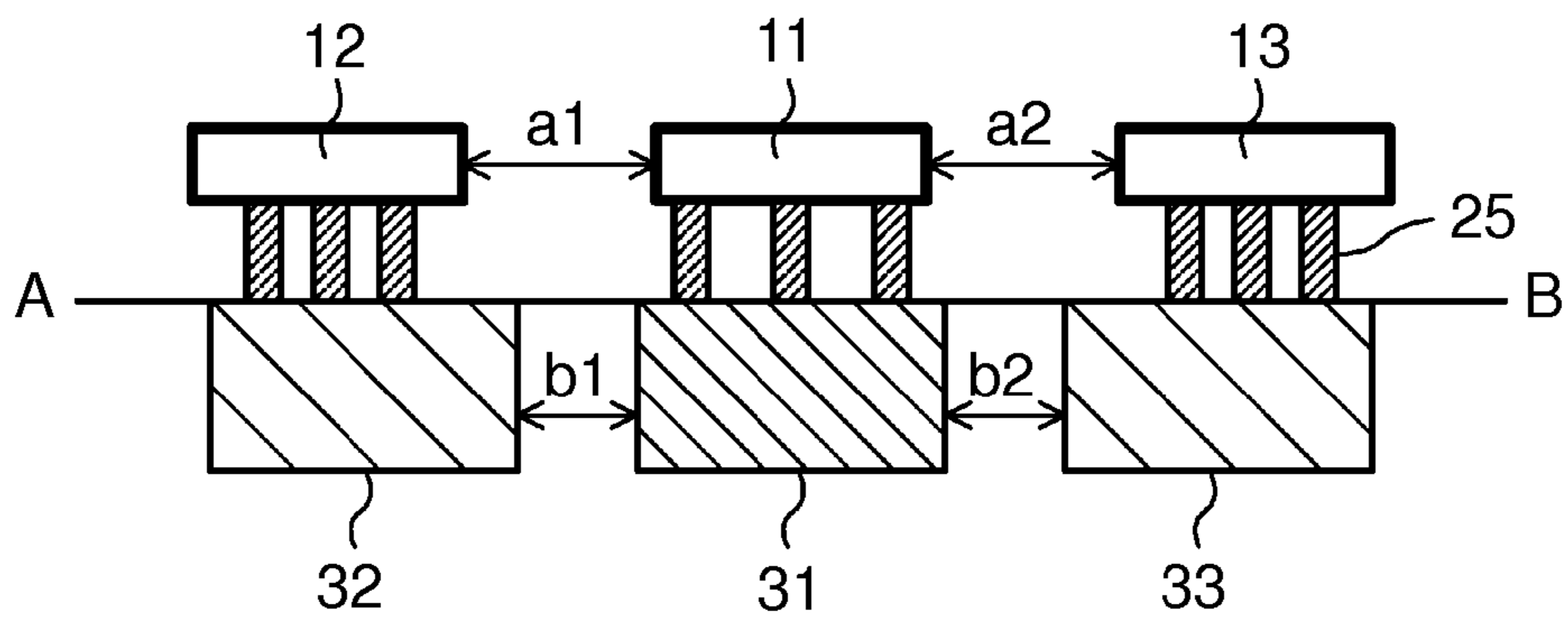
FIG. 12B
