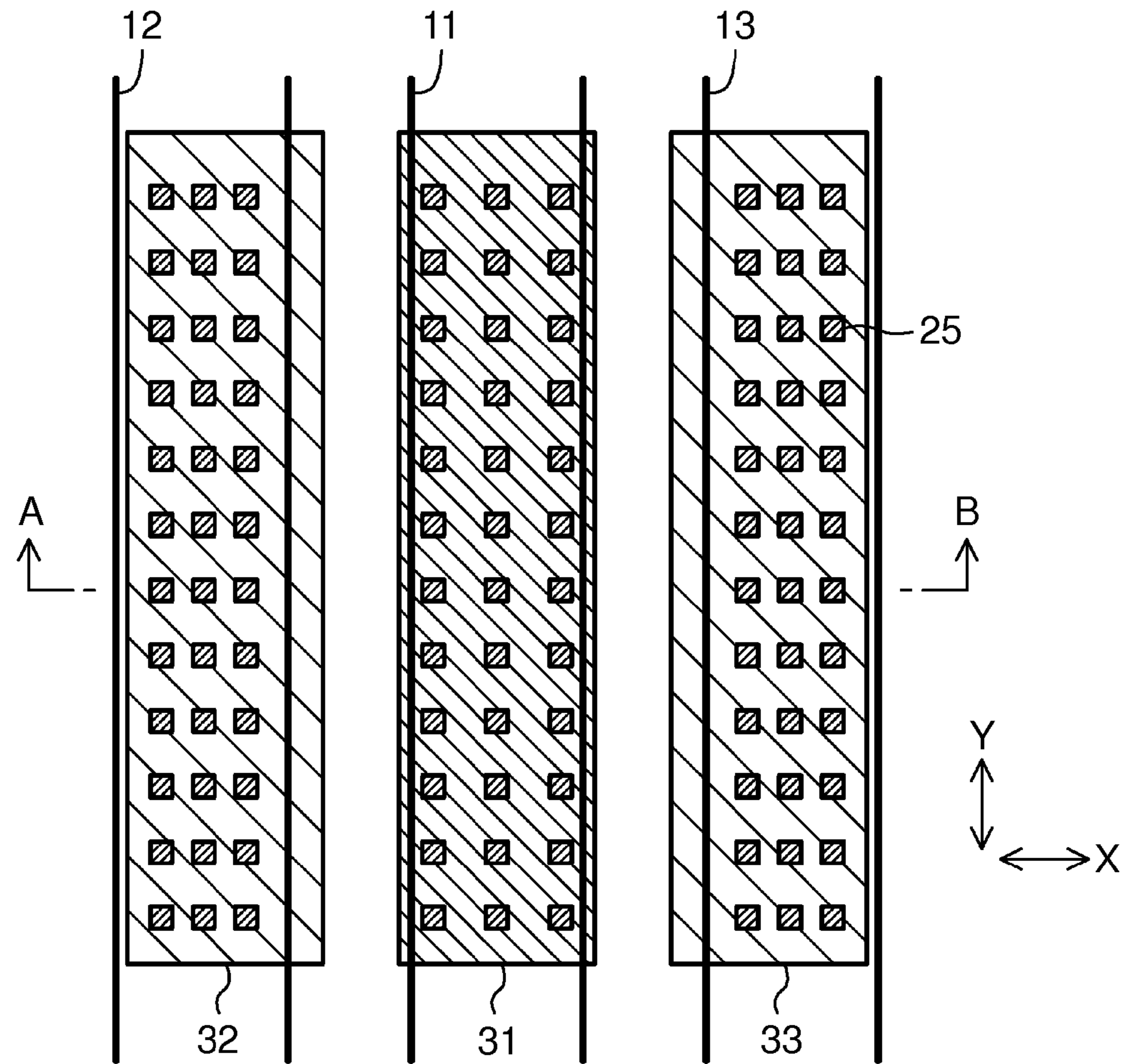
FIG. 12A
