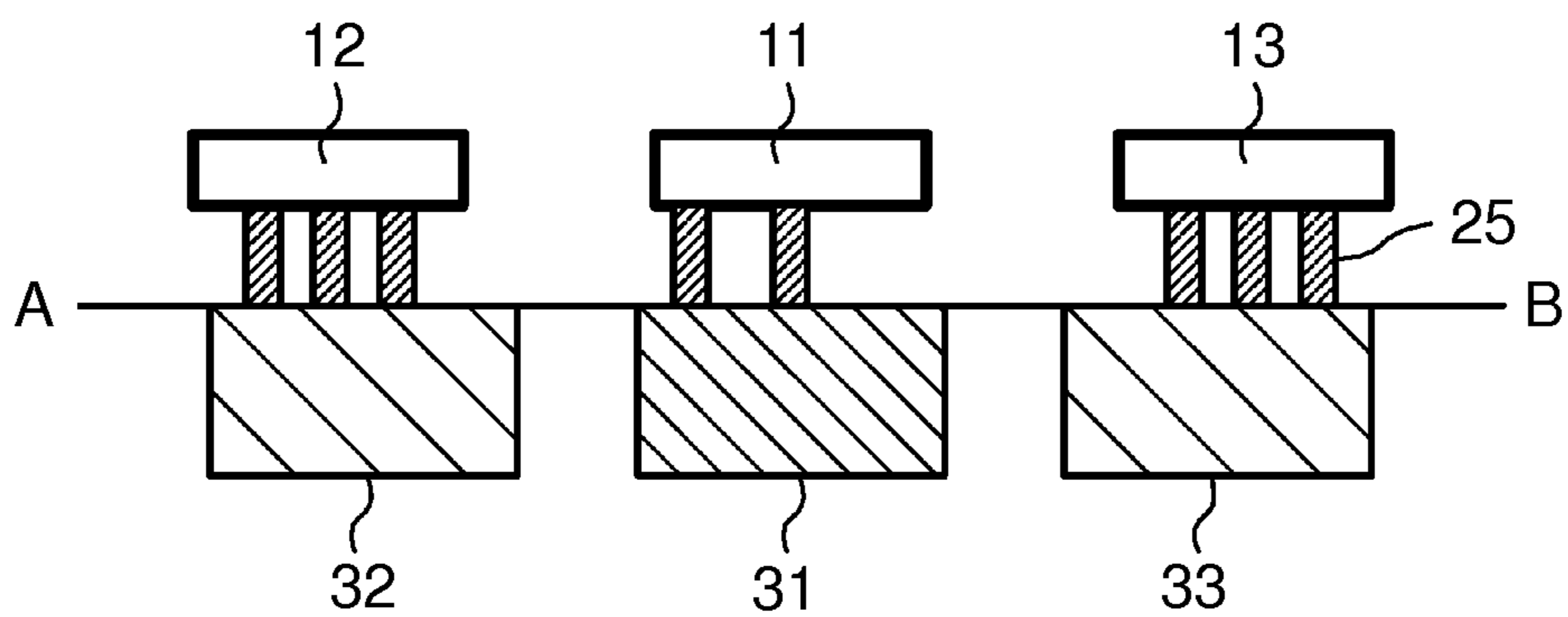
FIG. 13B
