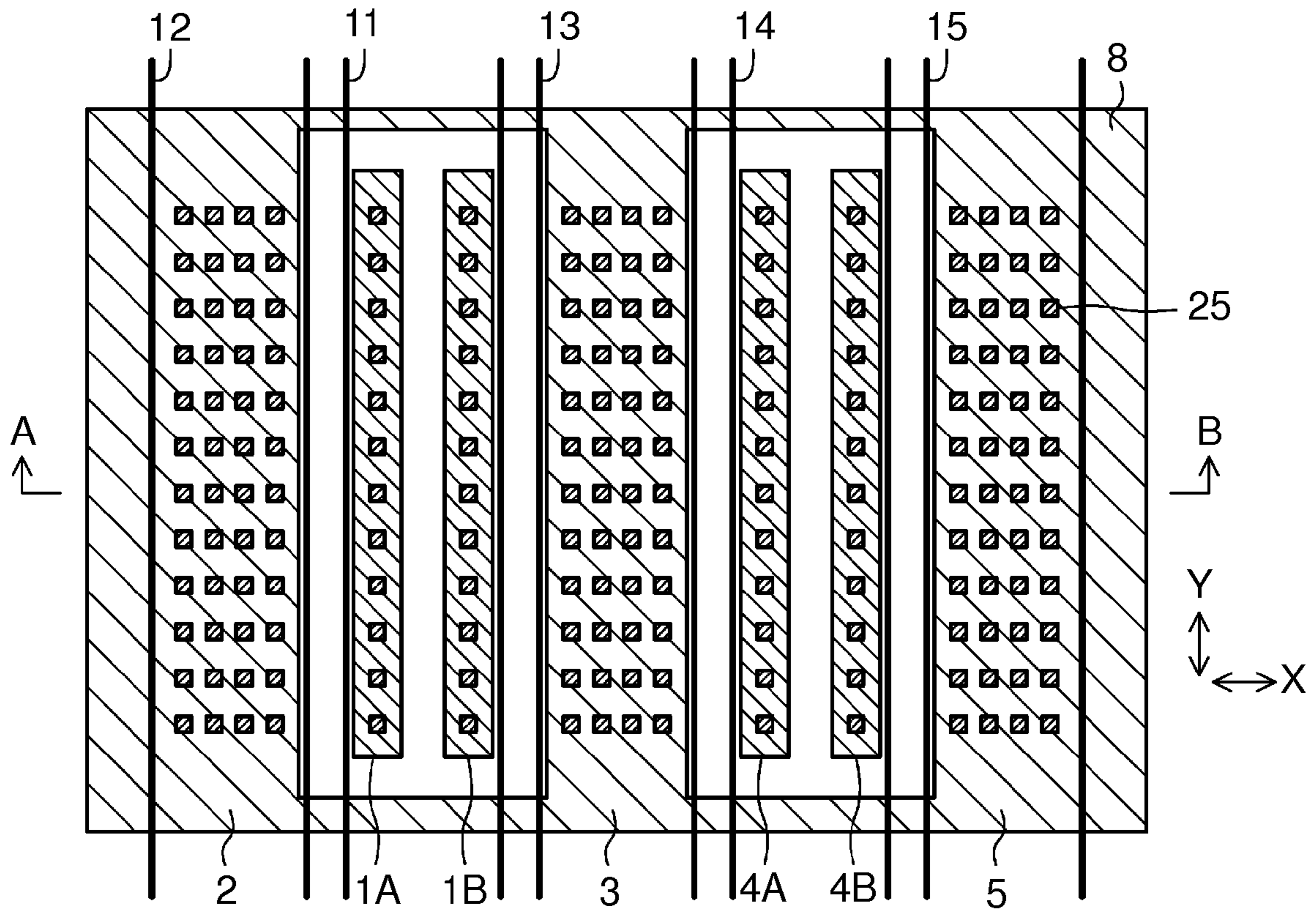
FIG. 11A
