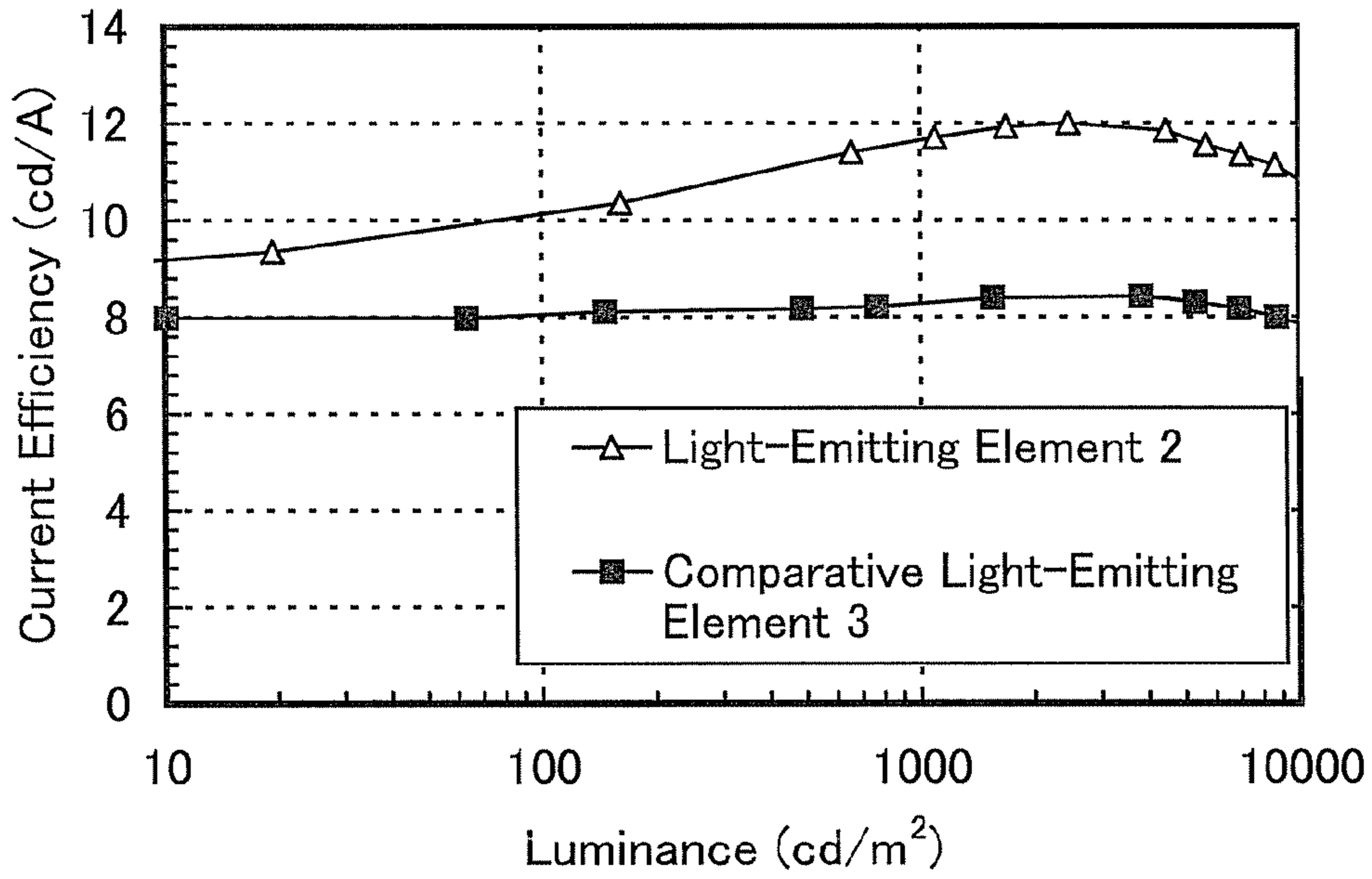
FIG. 20
