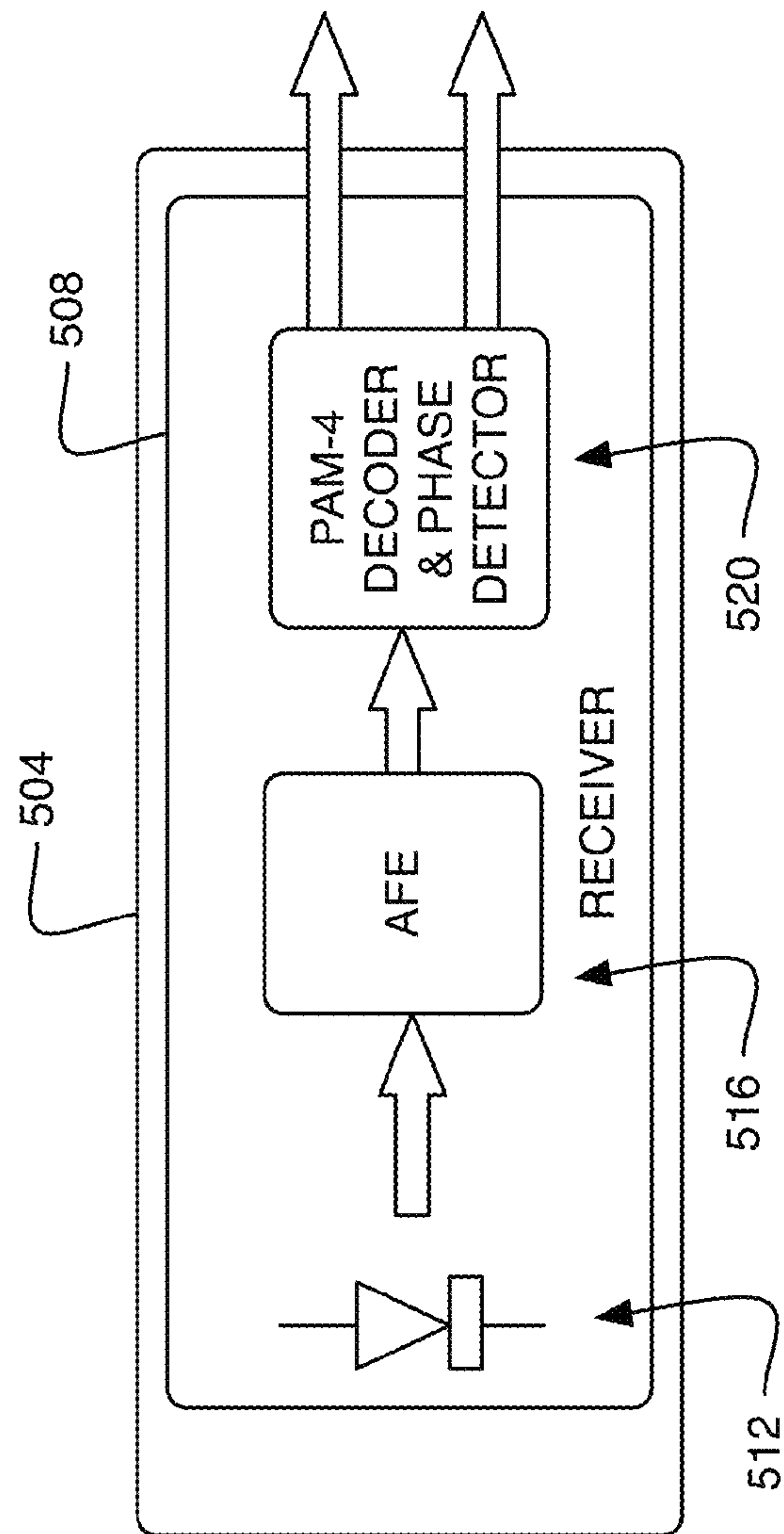
FIG. 5
