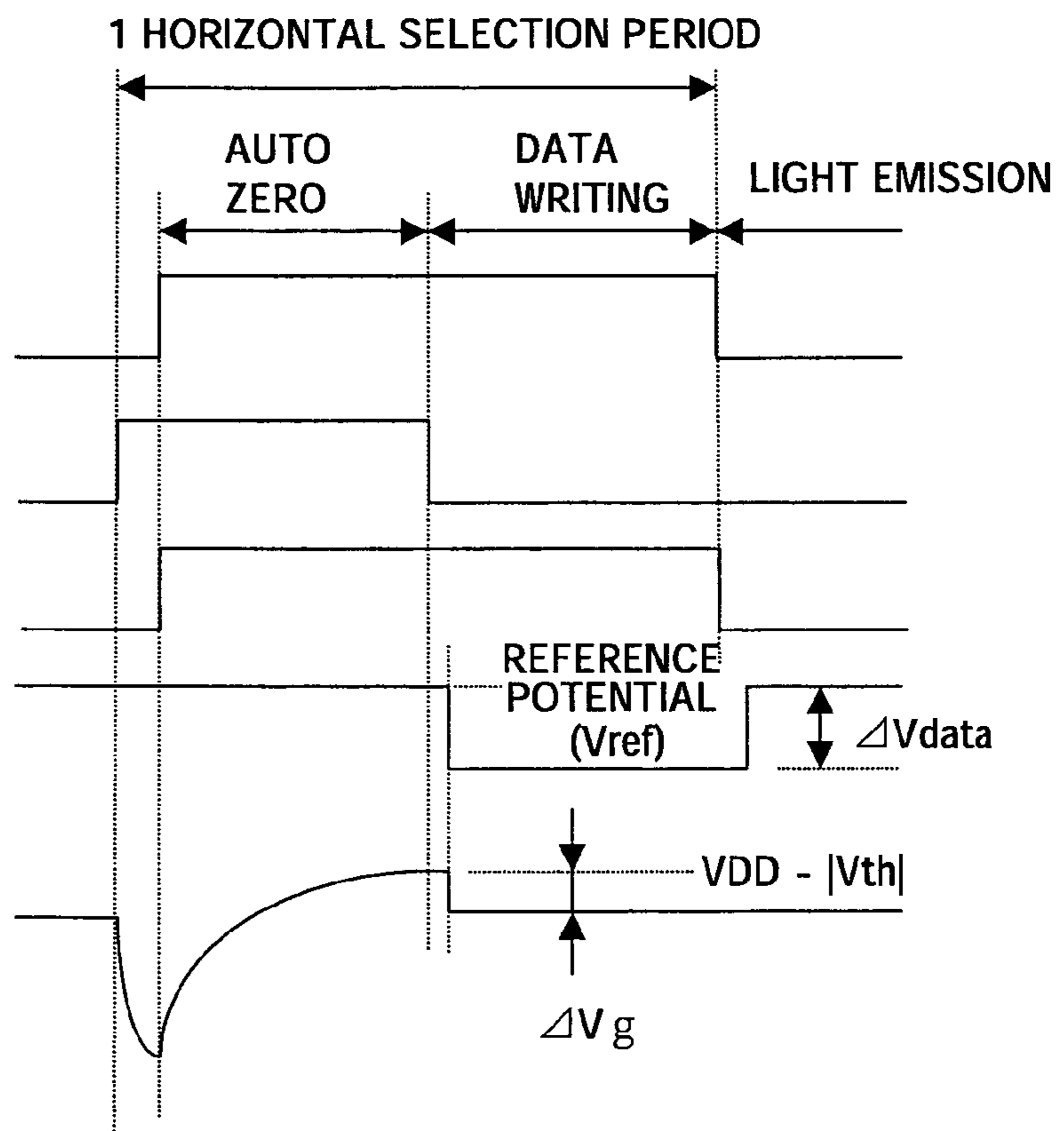
FIG. 4E V_g (TFT21)
