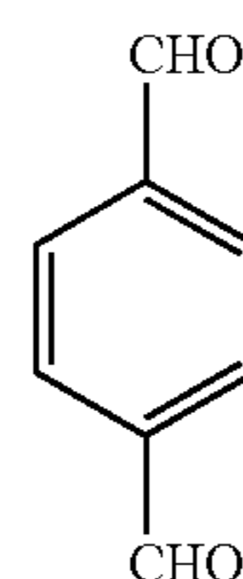
p-Benzylidialdehyde
