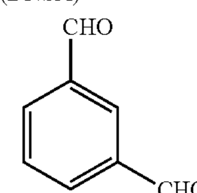
m-Benzylidialdehyde
