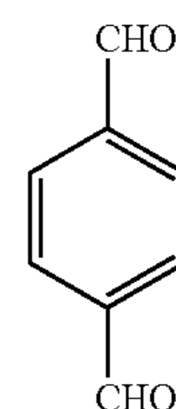
p-Benzylidialdehyde
