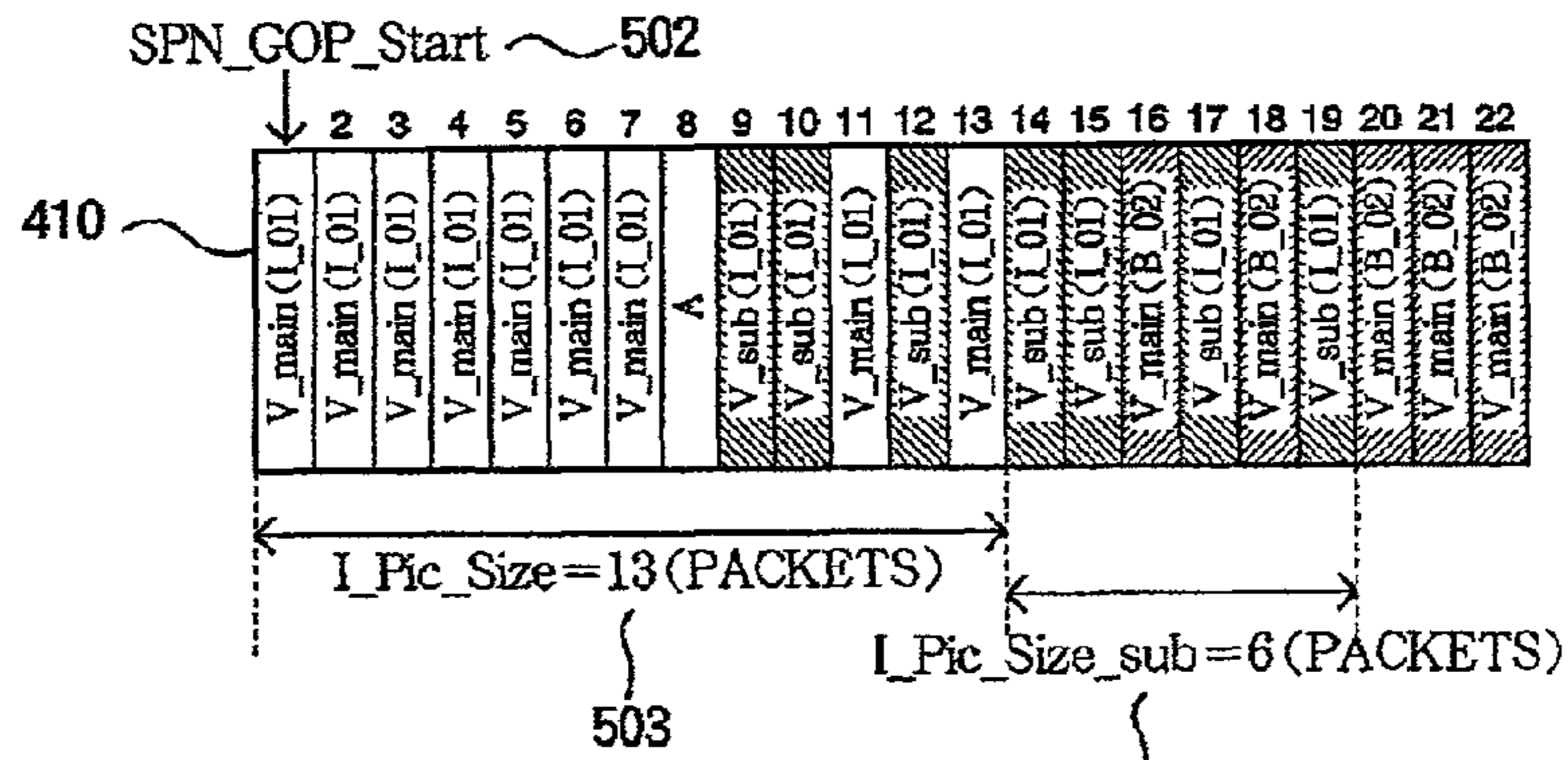
FIG. 15 (B)
