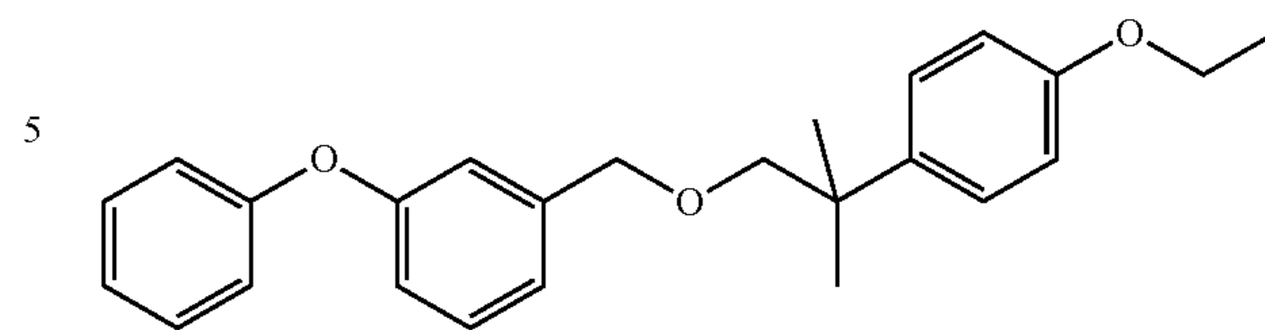
Ethofenprox
