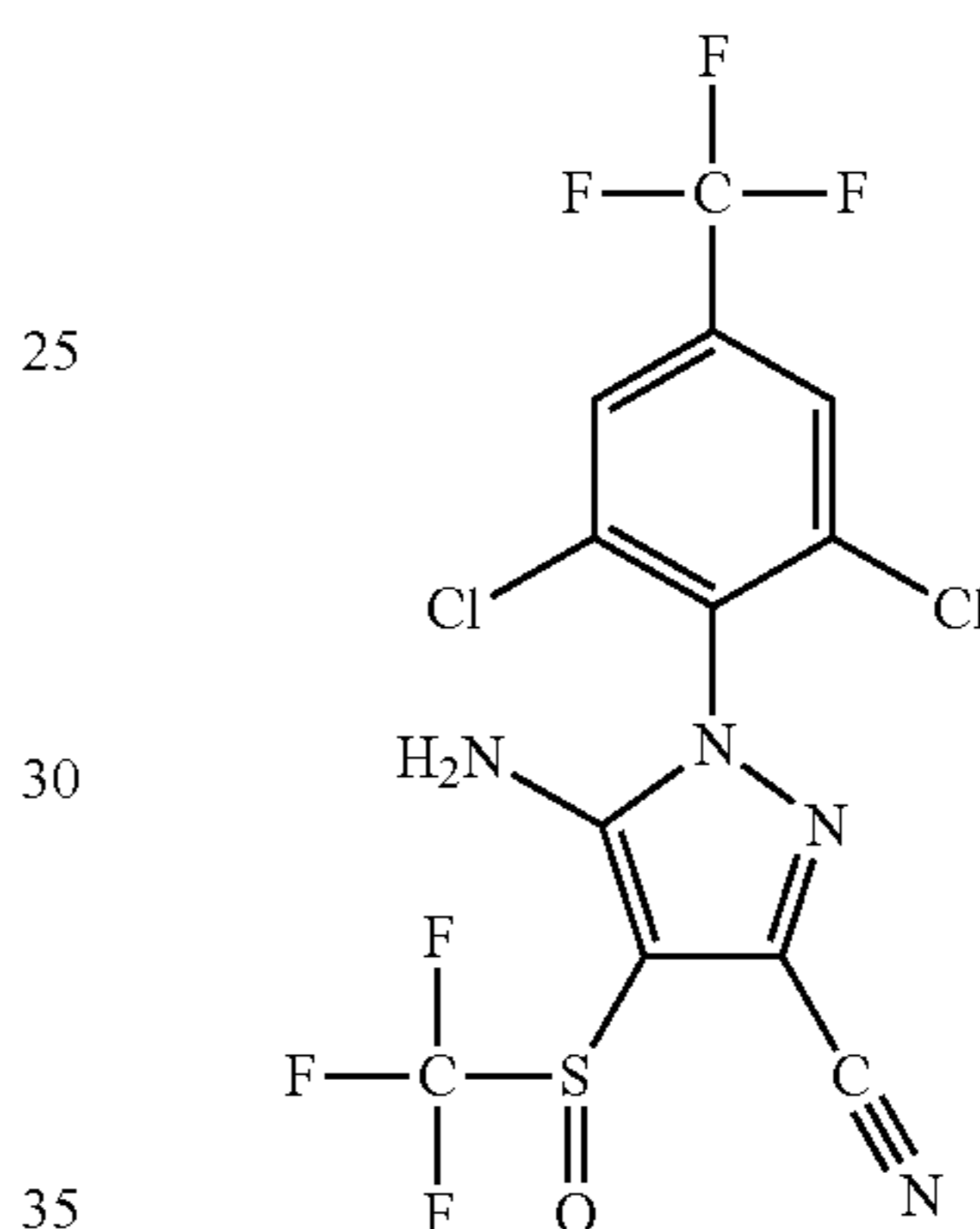
Fipronil
