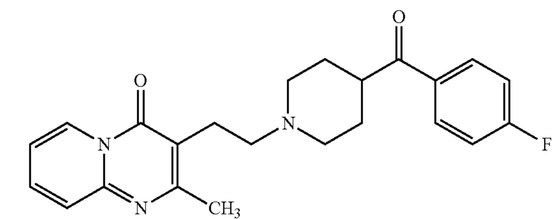
(pirenperone)
