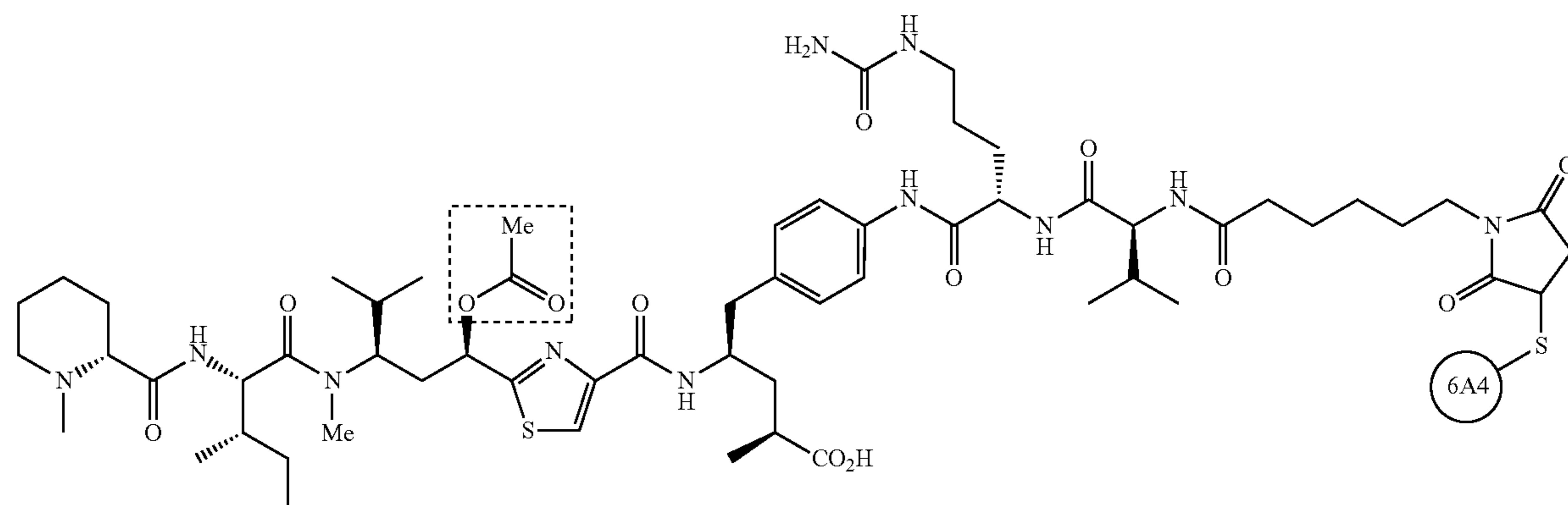
Conjugate B
