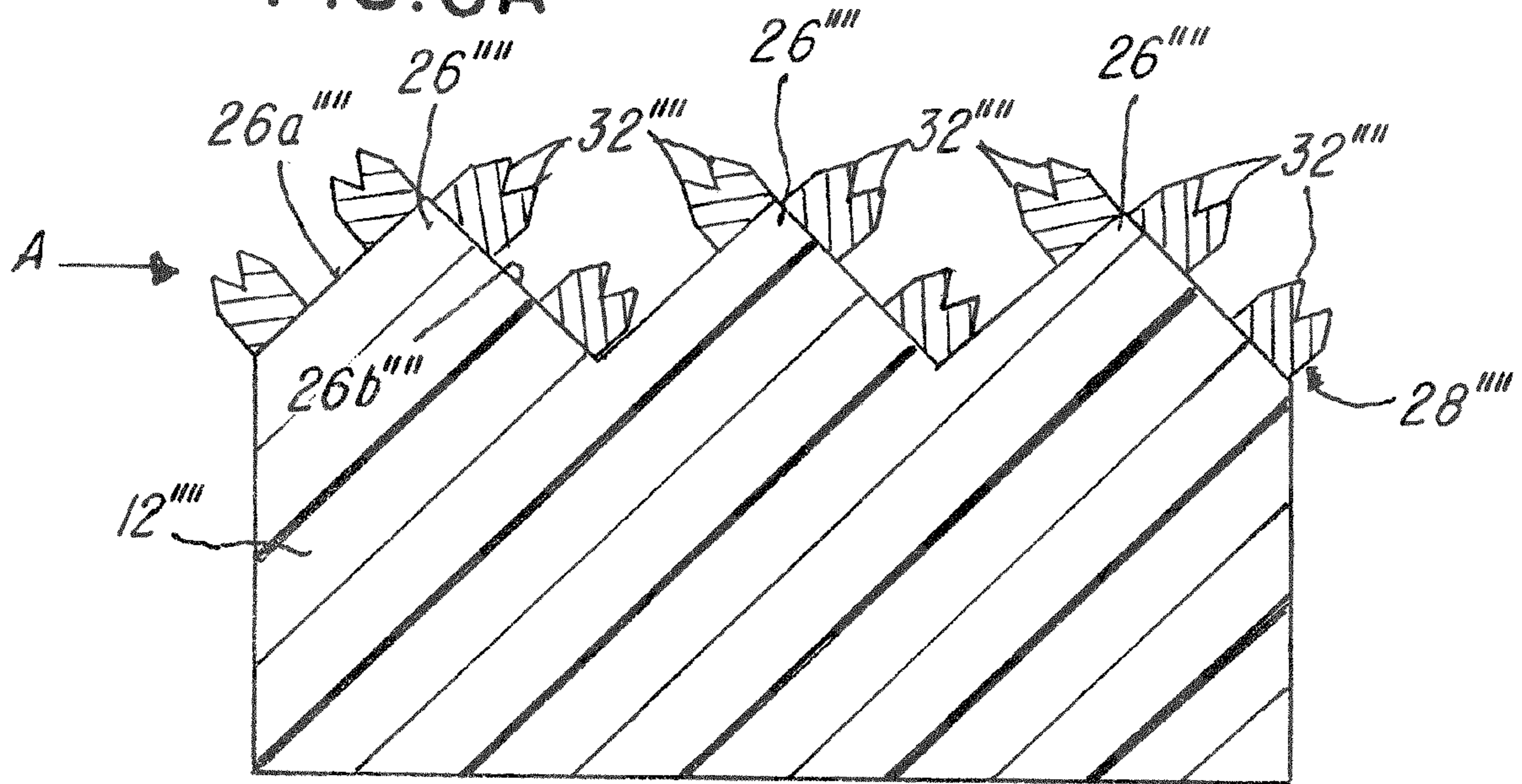
FIG. 6A
