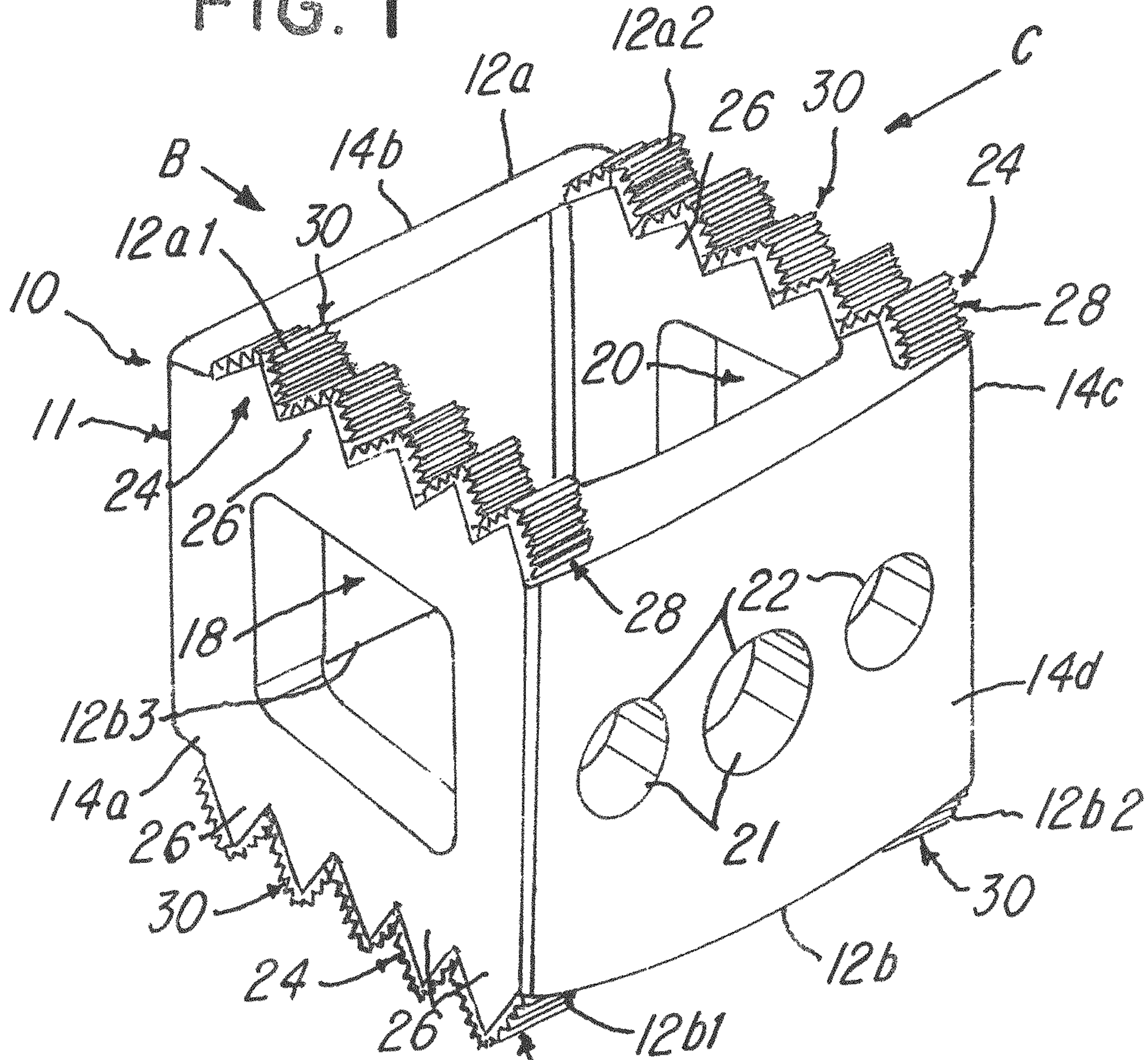
FIG. 1A
