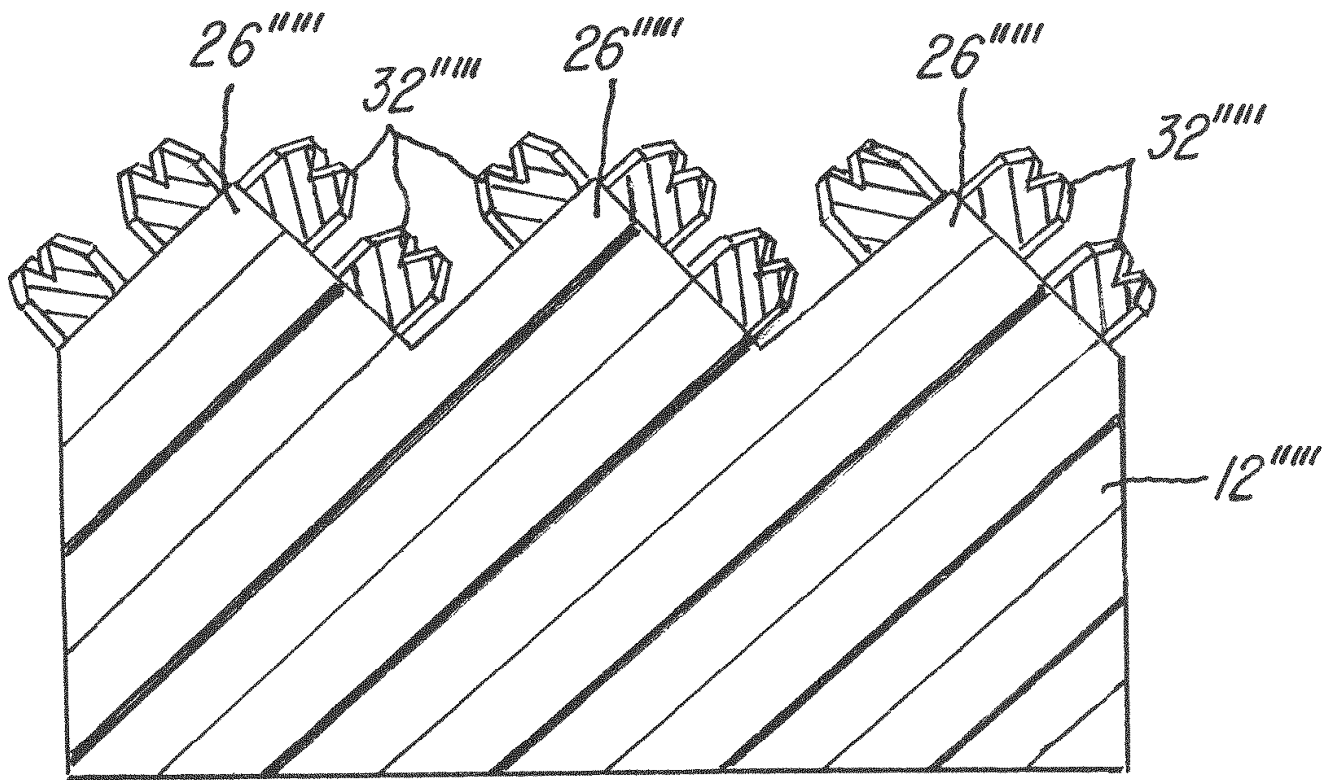
FIG. 8A
