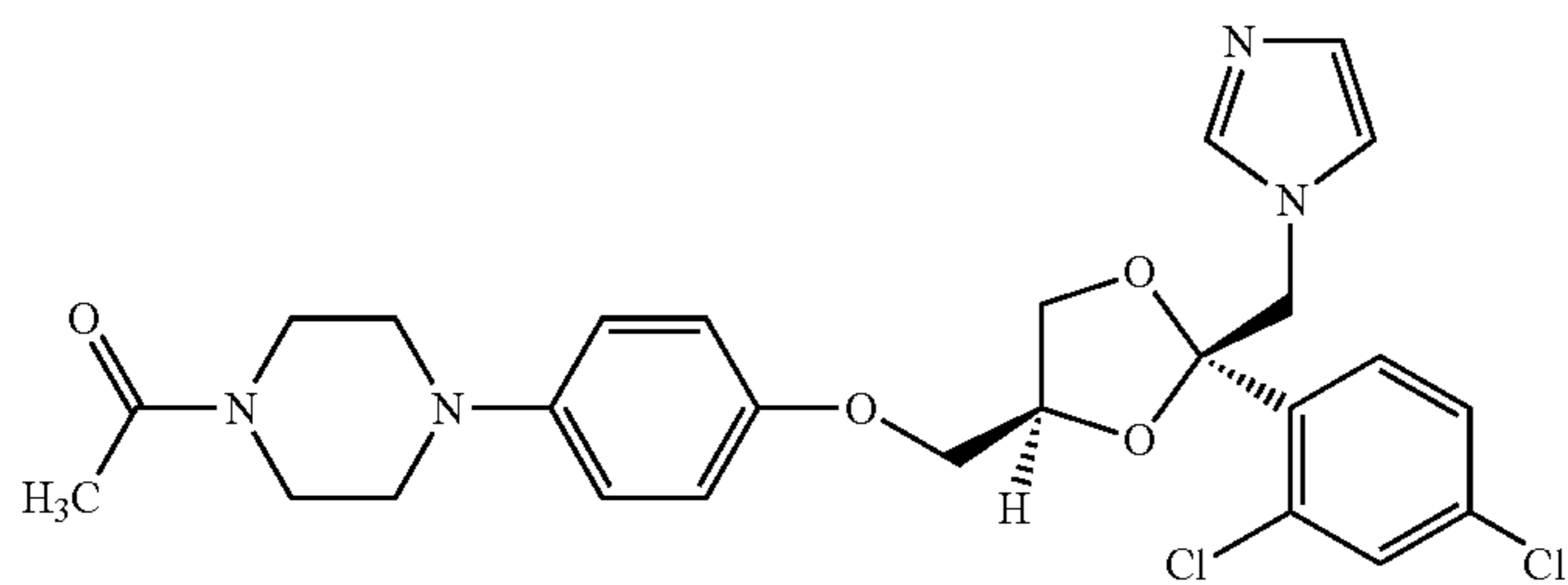
Ketoconazole
