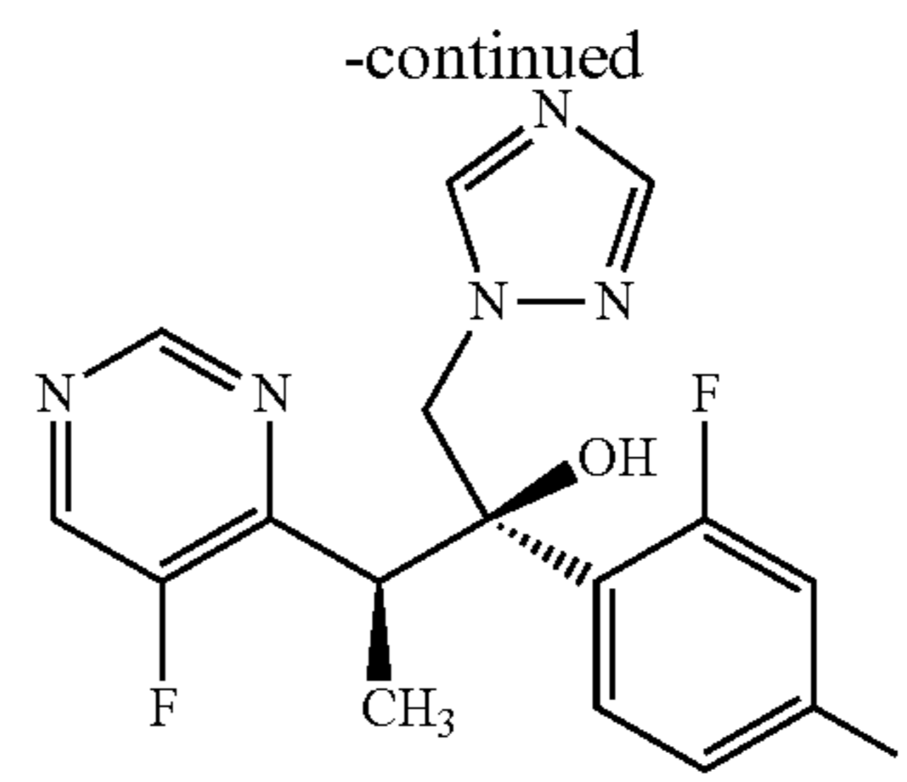
Voriconazole
