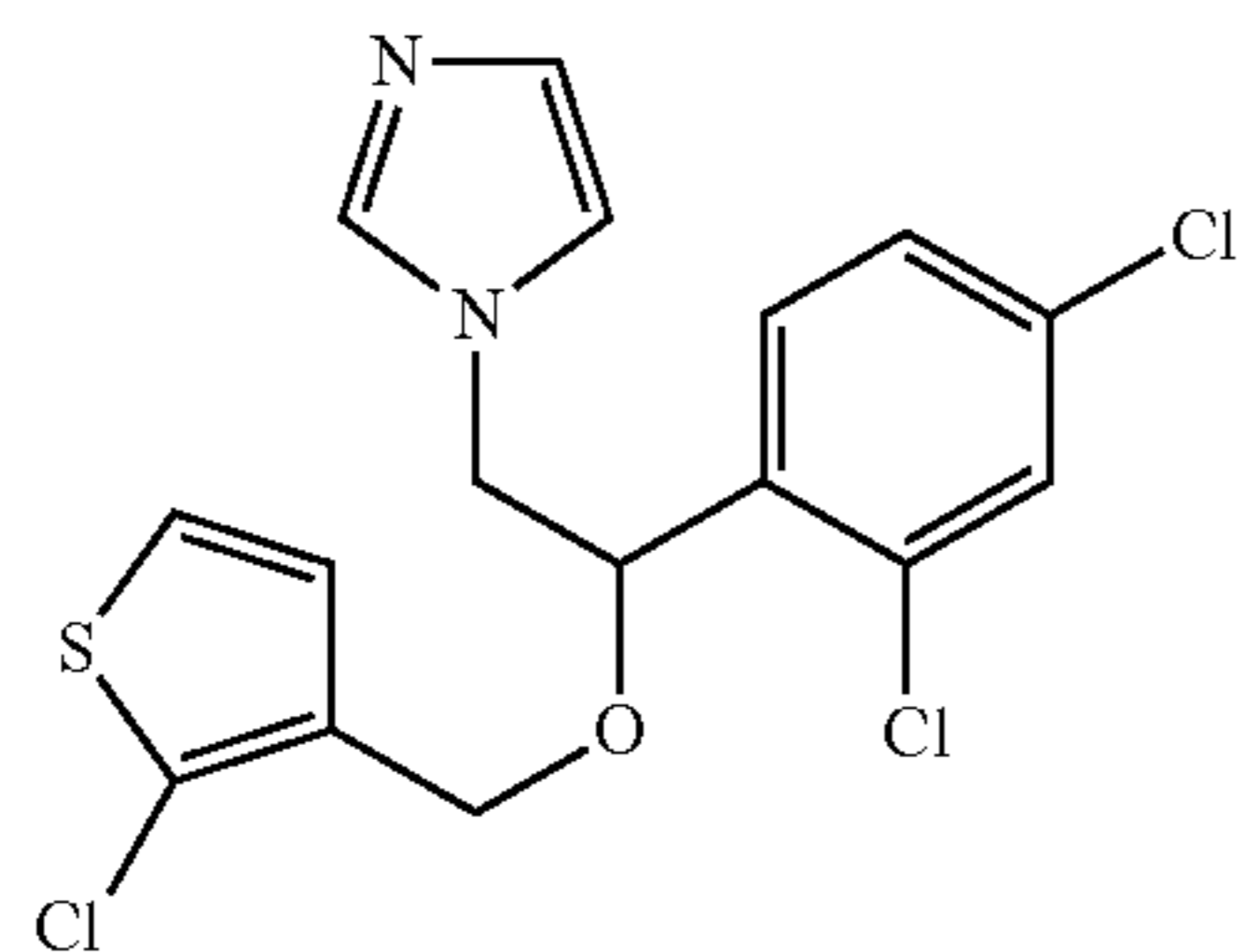
Tioconazole
