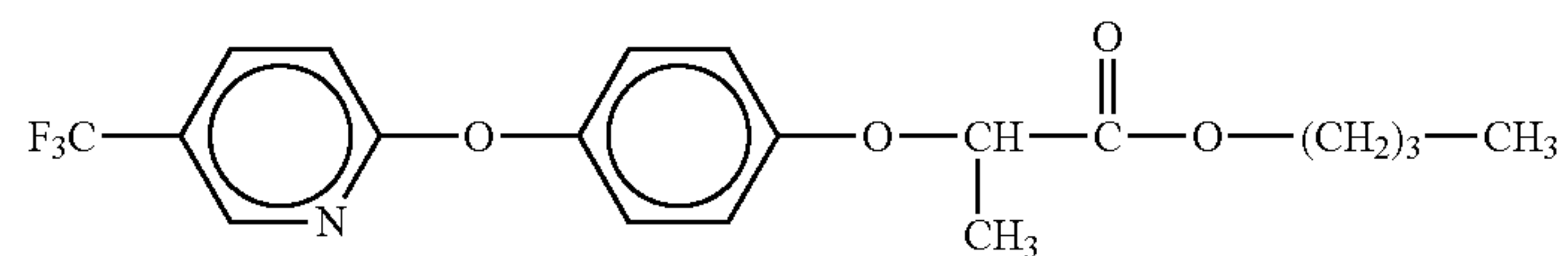
Fluazifop-P-butyl
