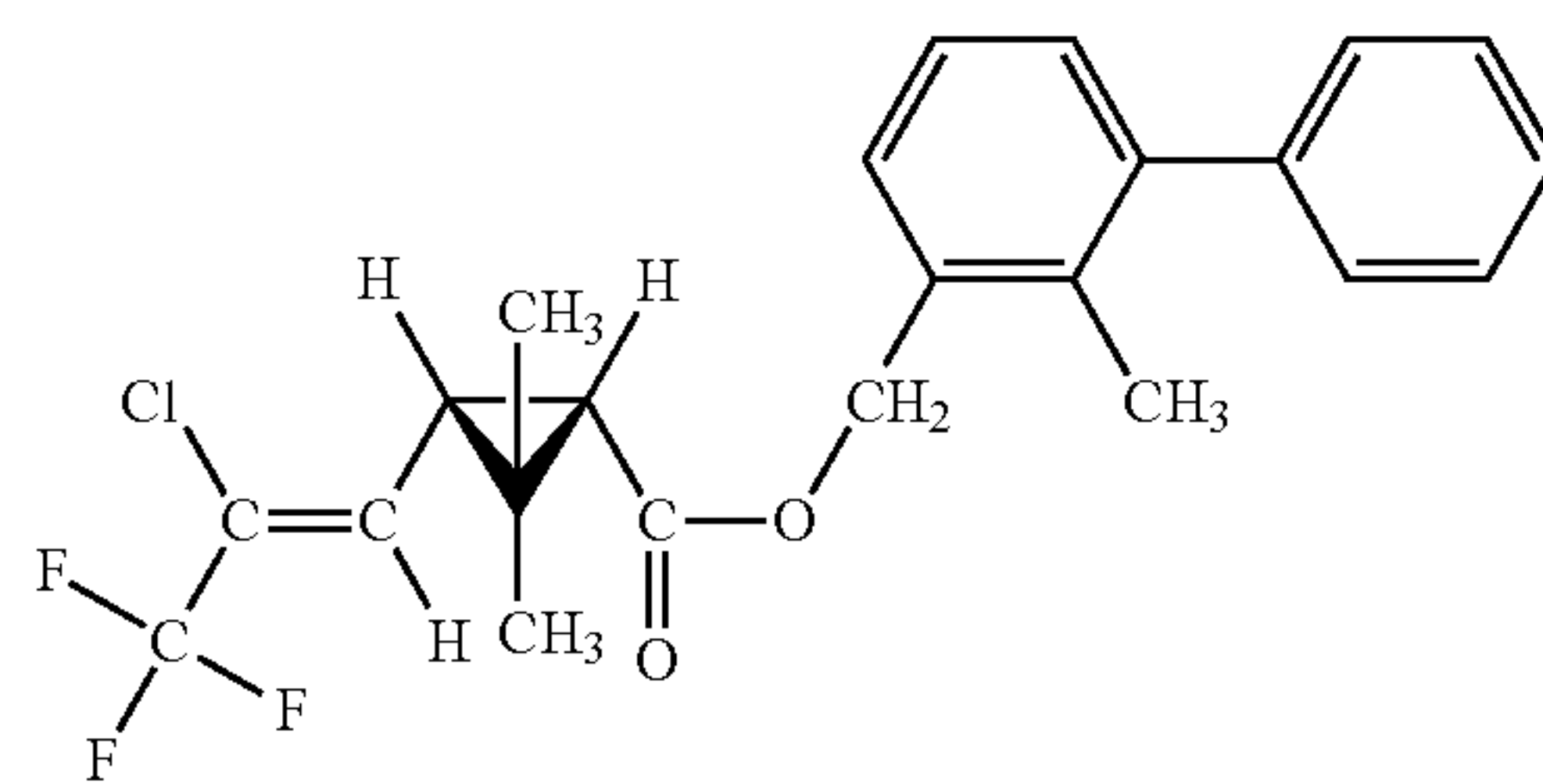
(Z)-(1S)-cis-acid
