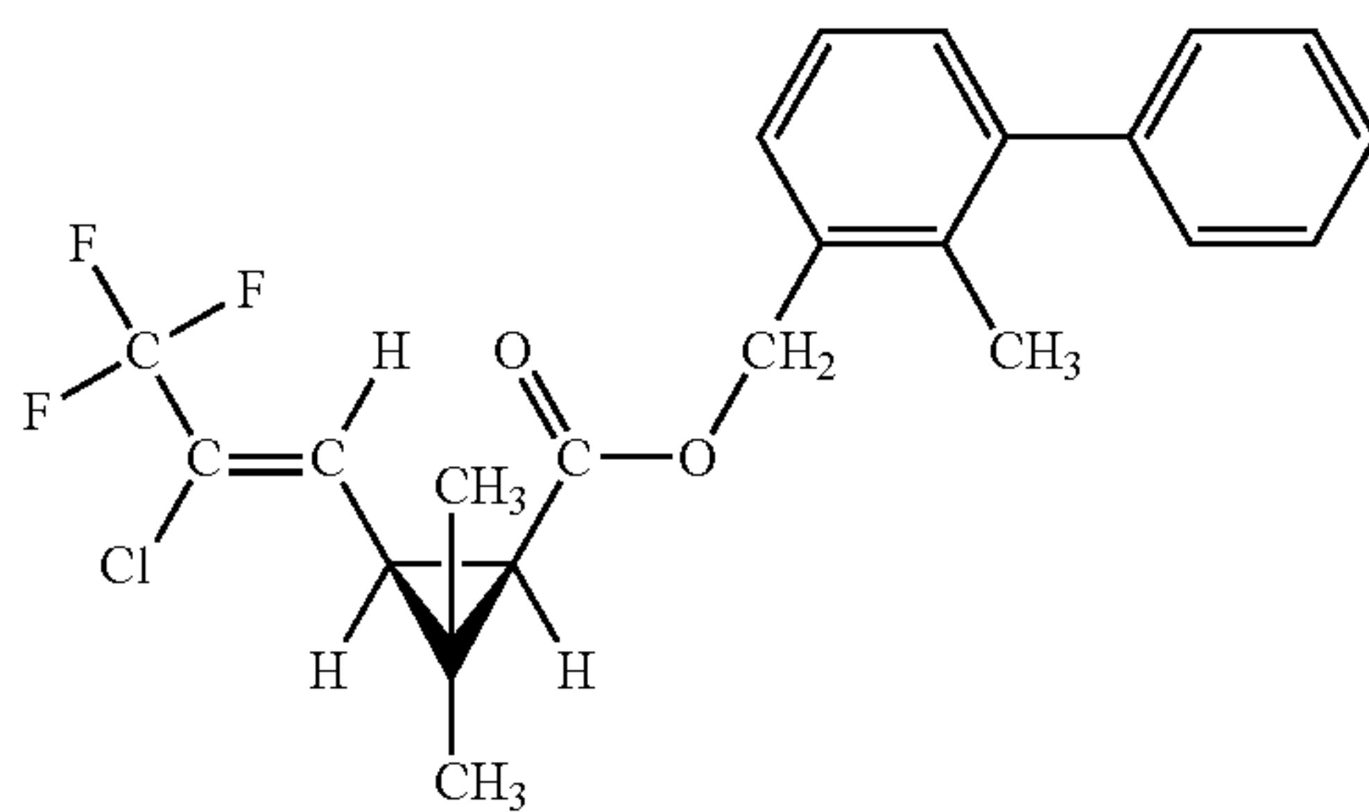
(Z)-(1R)-cis-acid
