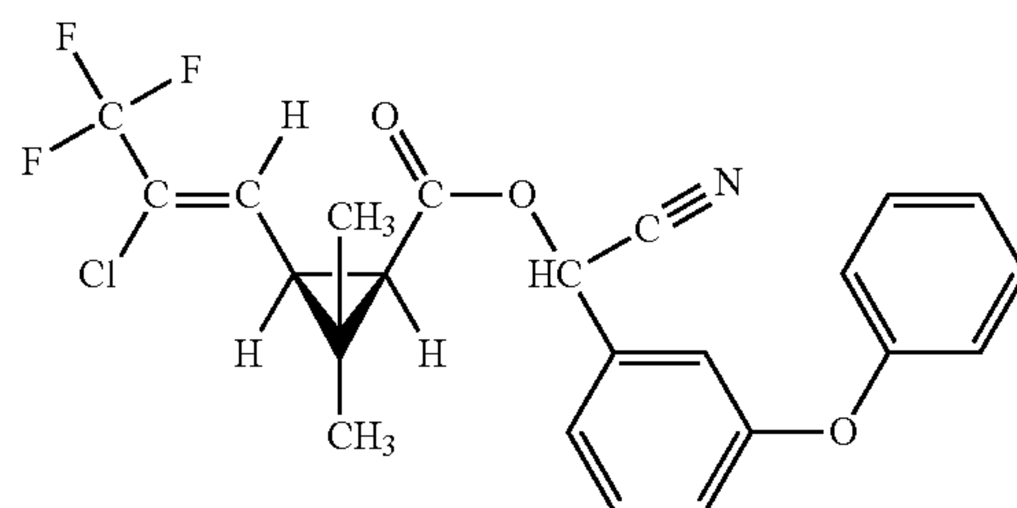
(Z)-(1R)-cis-acid
