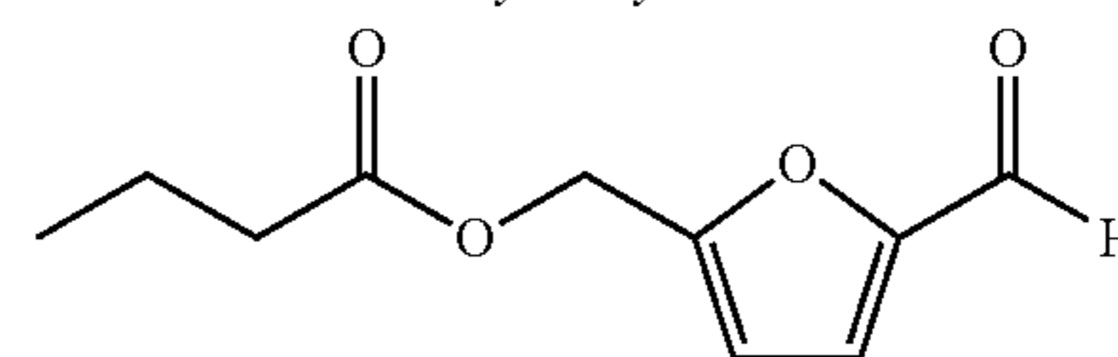
5-butyroxymethylfurfural
