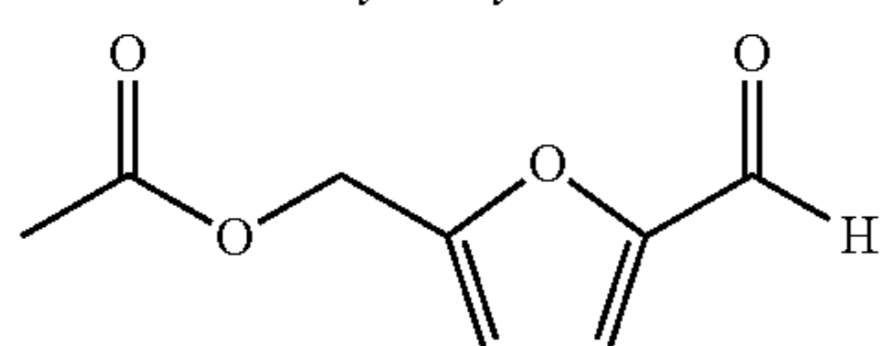
5-acetoxymethylfurfural
