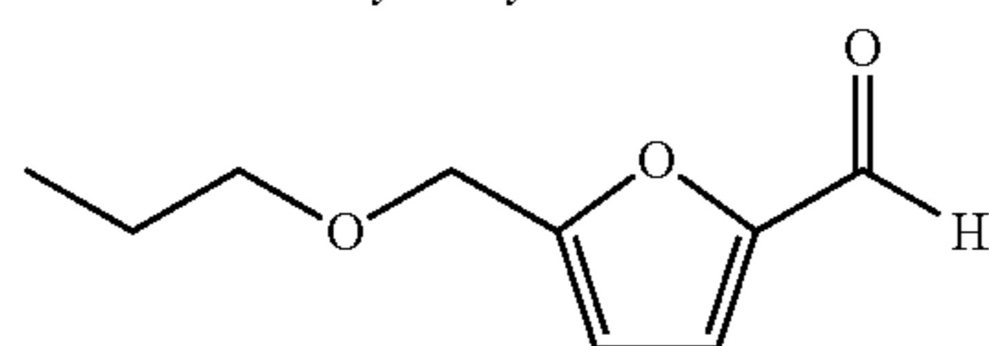
5-propoxymethylfurfural
