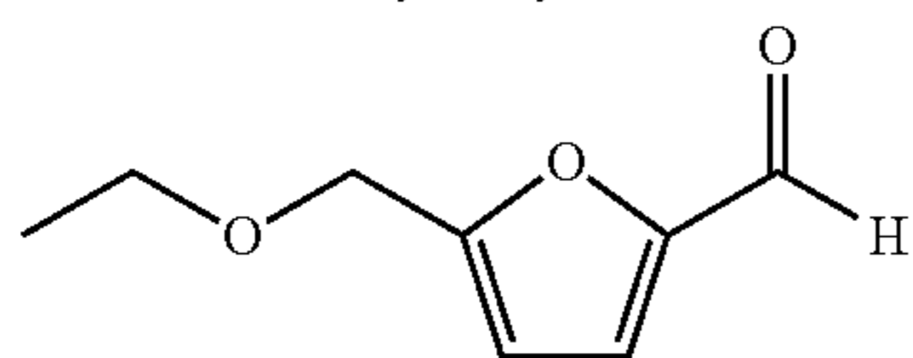
5-ethoxymethylfurfural
