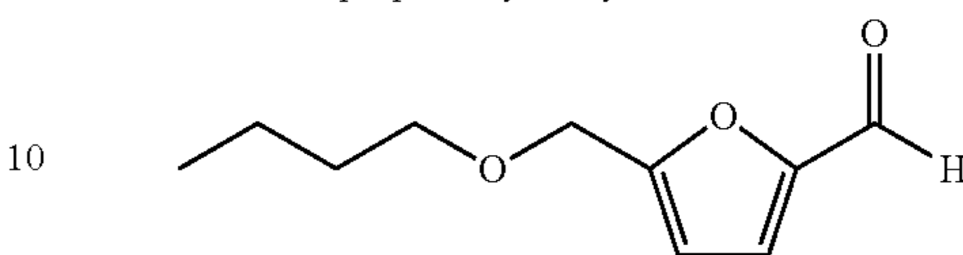
5-butoxymethylfurfural
