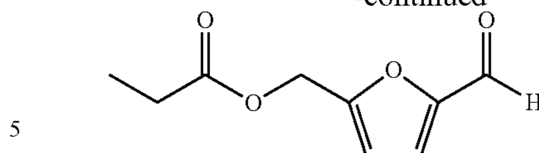
5-propionoxymethylfurfural
