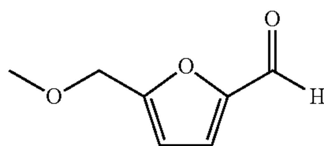
5-methoxymethylfurfural
