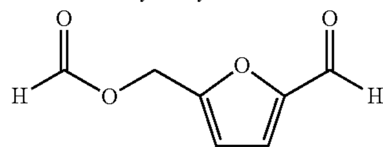
5-formoxymethylfurfural
