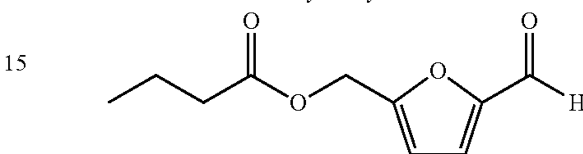
5-butyroxymethylfurfural
