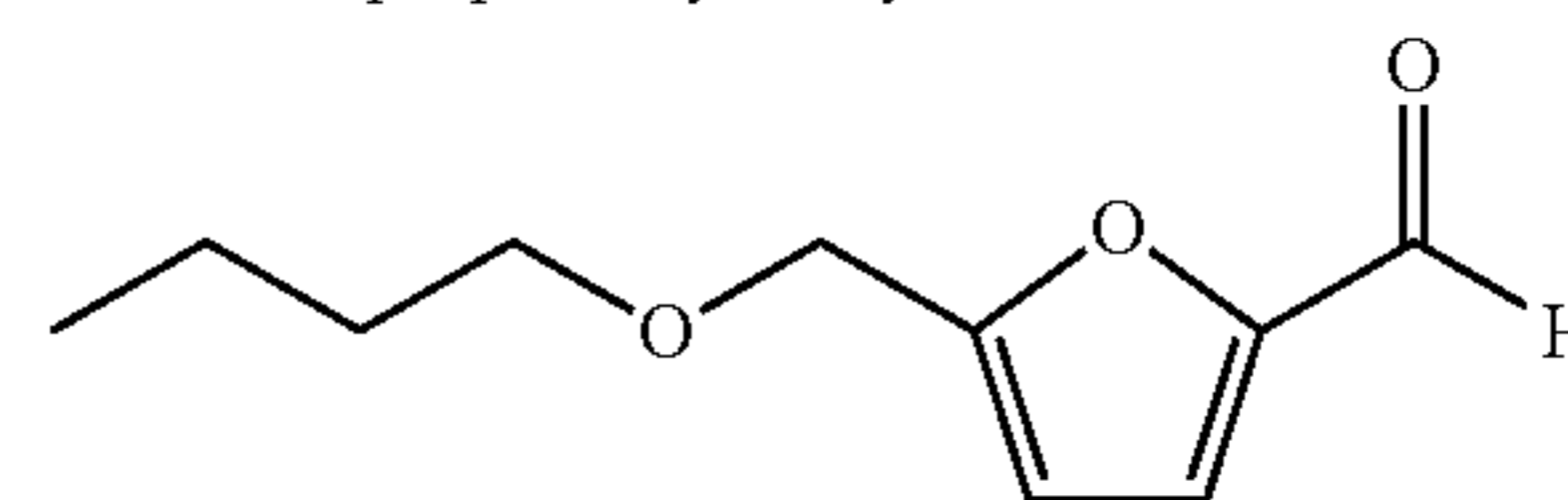
5-butoxymethylfurfural
