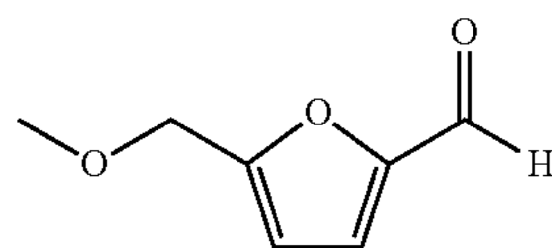
5-methoxymethylfurfural
