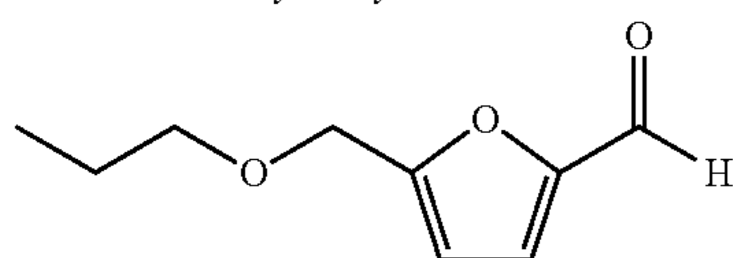
5-propoxymethylfurfural
