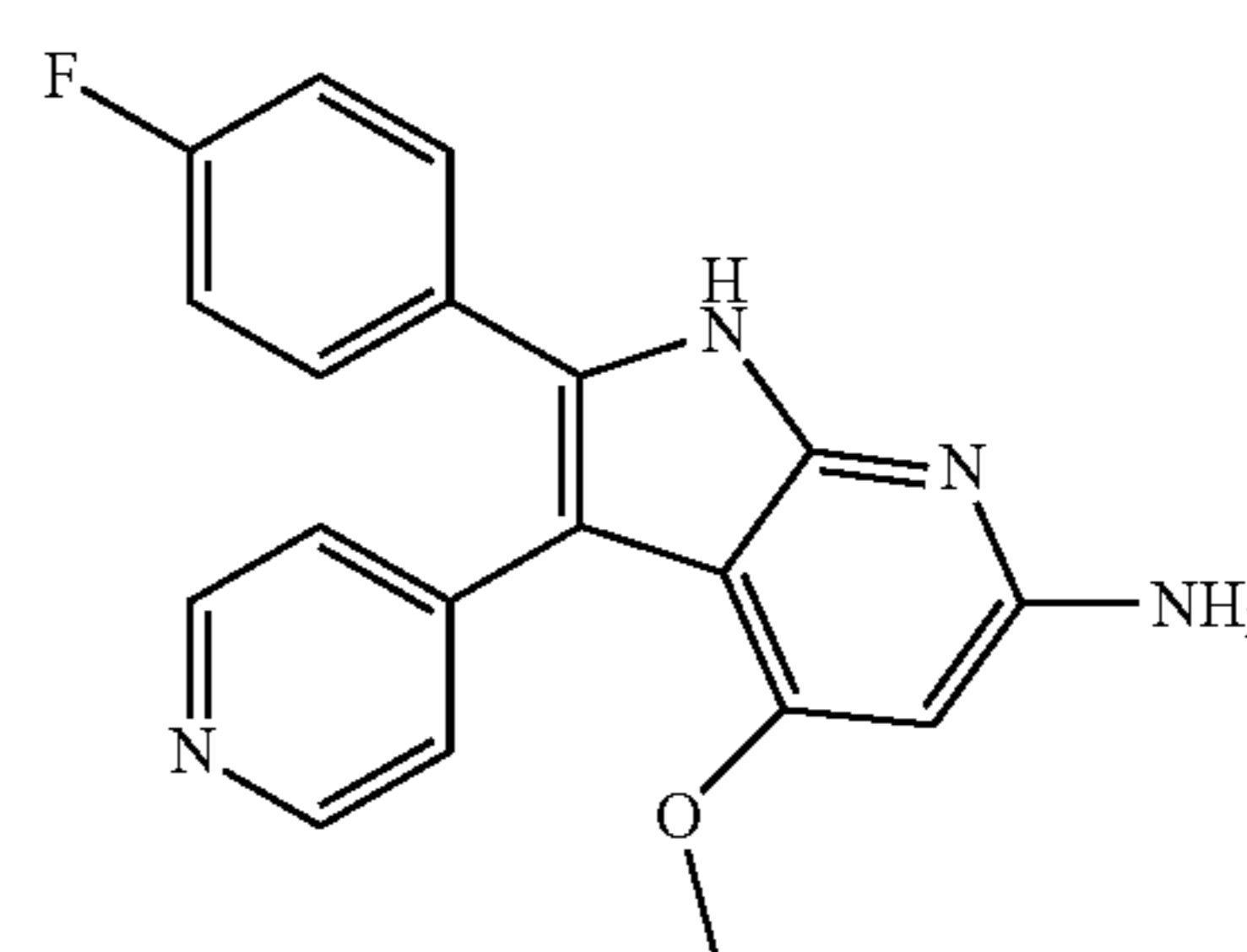
RWJ 68354
