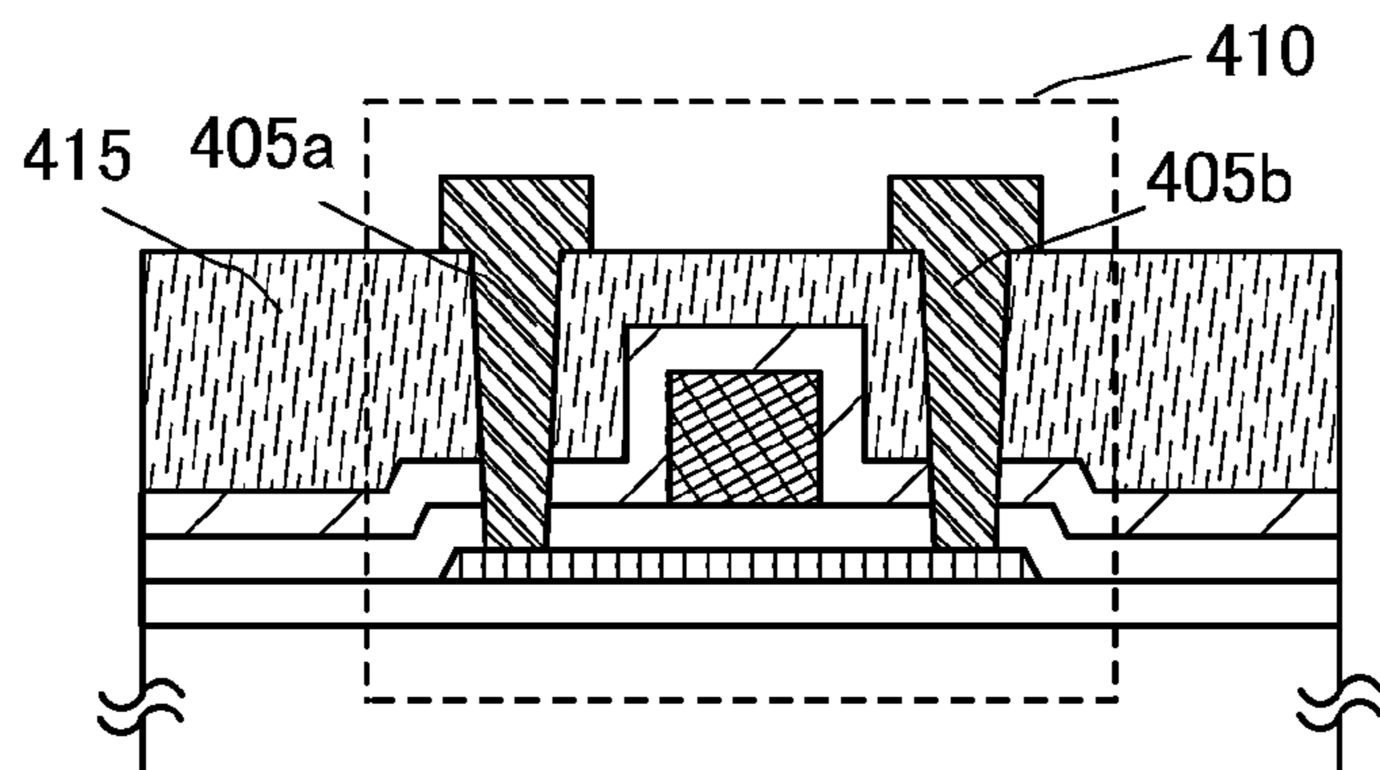
FIG. 4E
