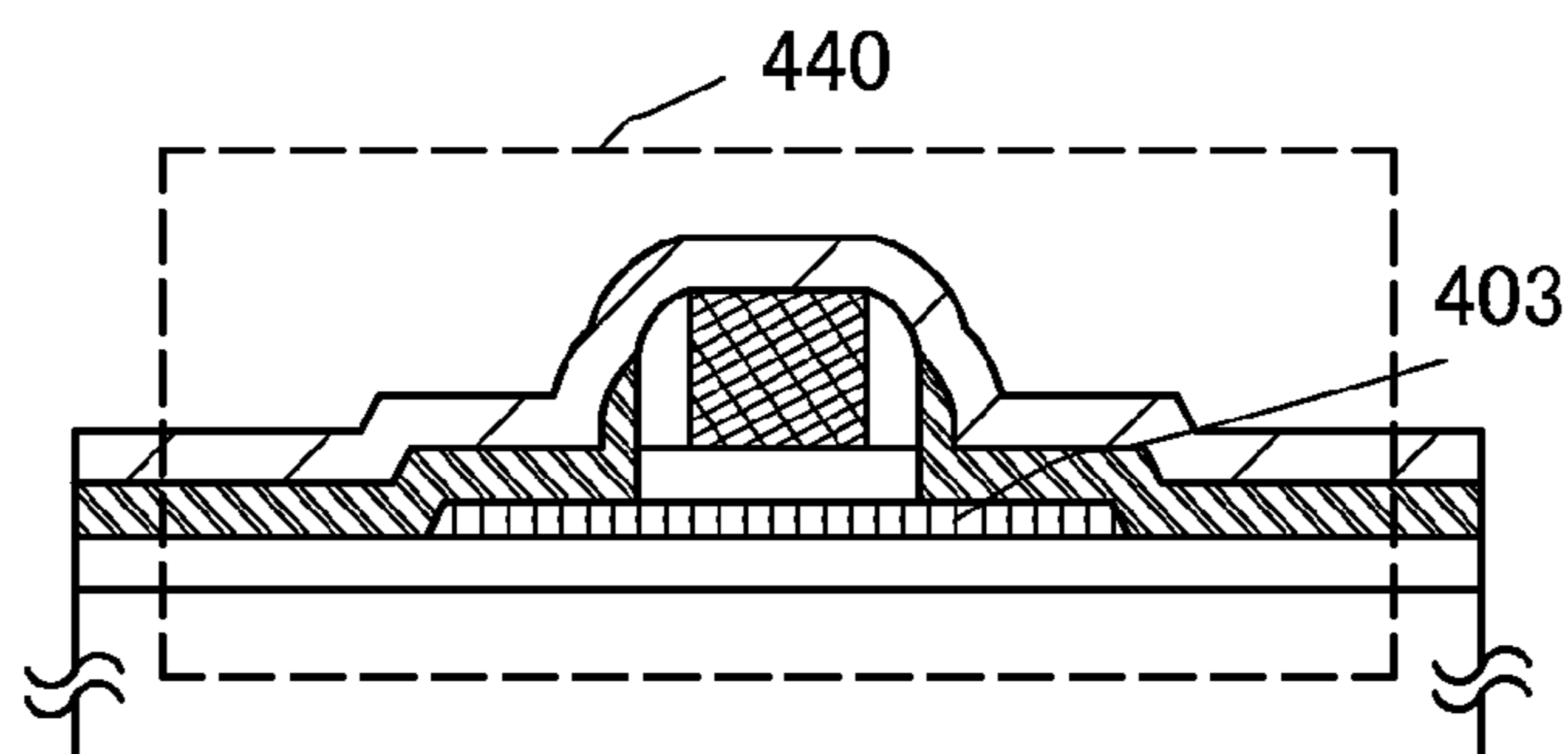
FIG. 2F
