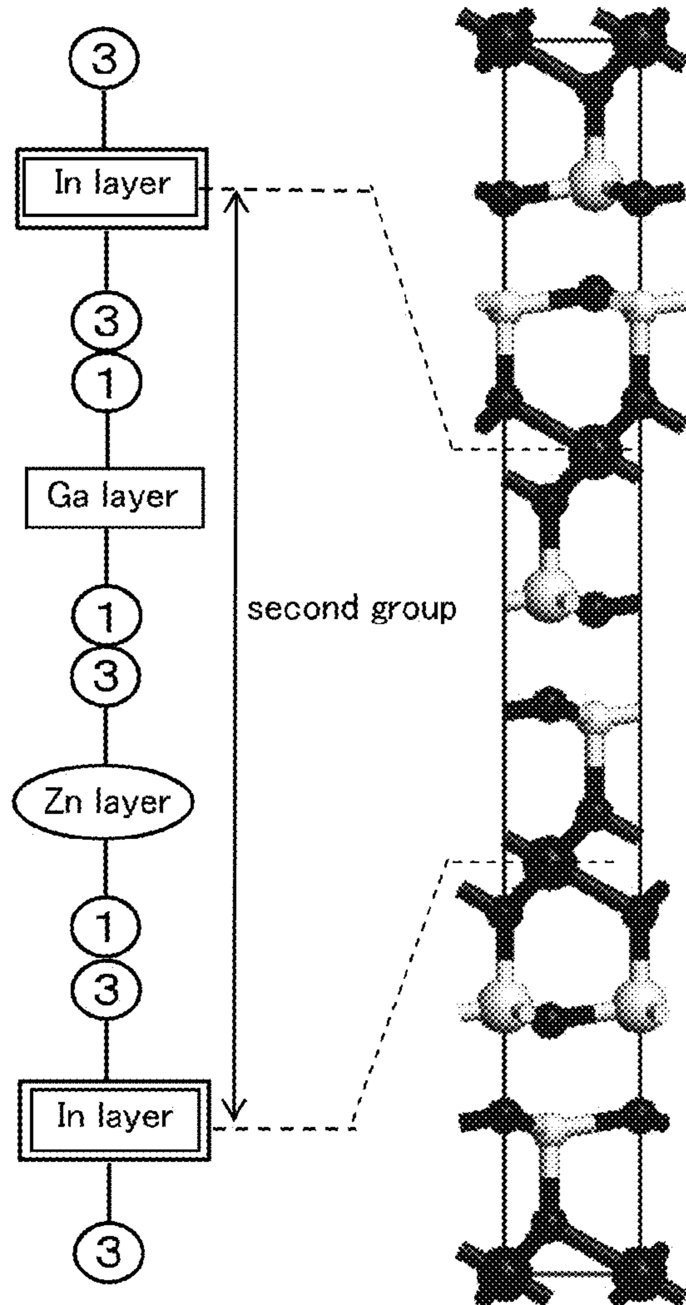
FIG. 28A
