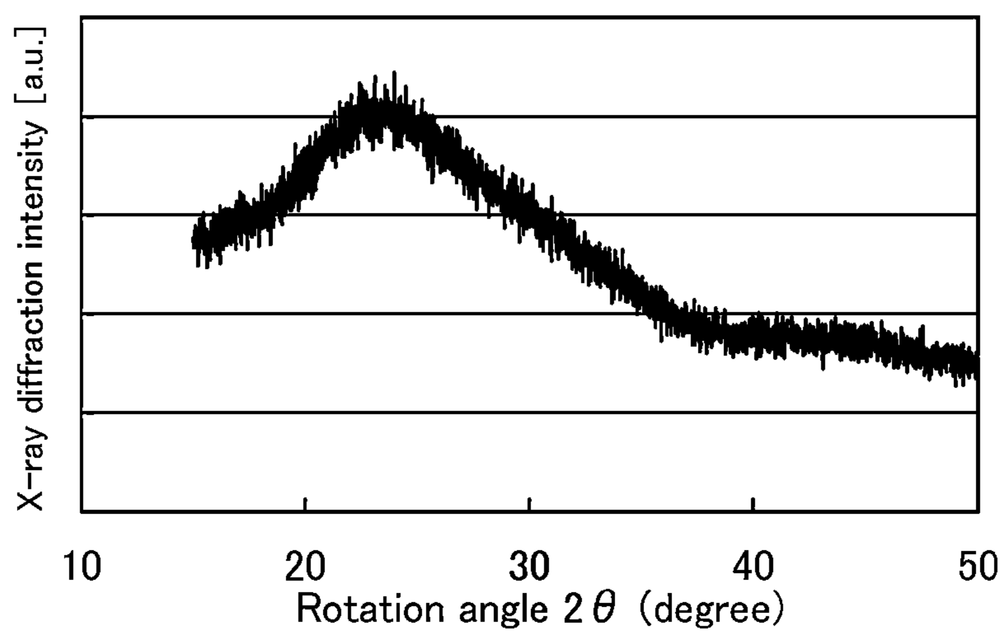
FIG. 13C
