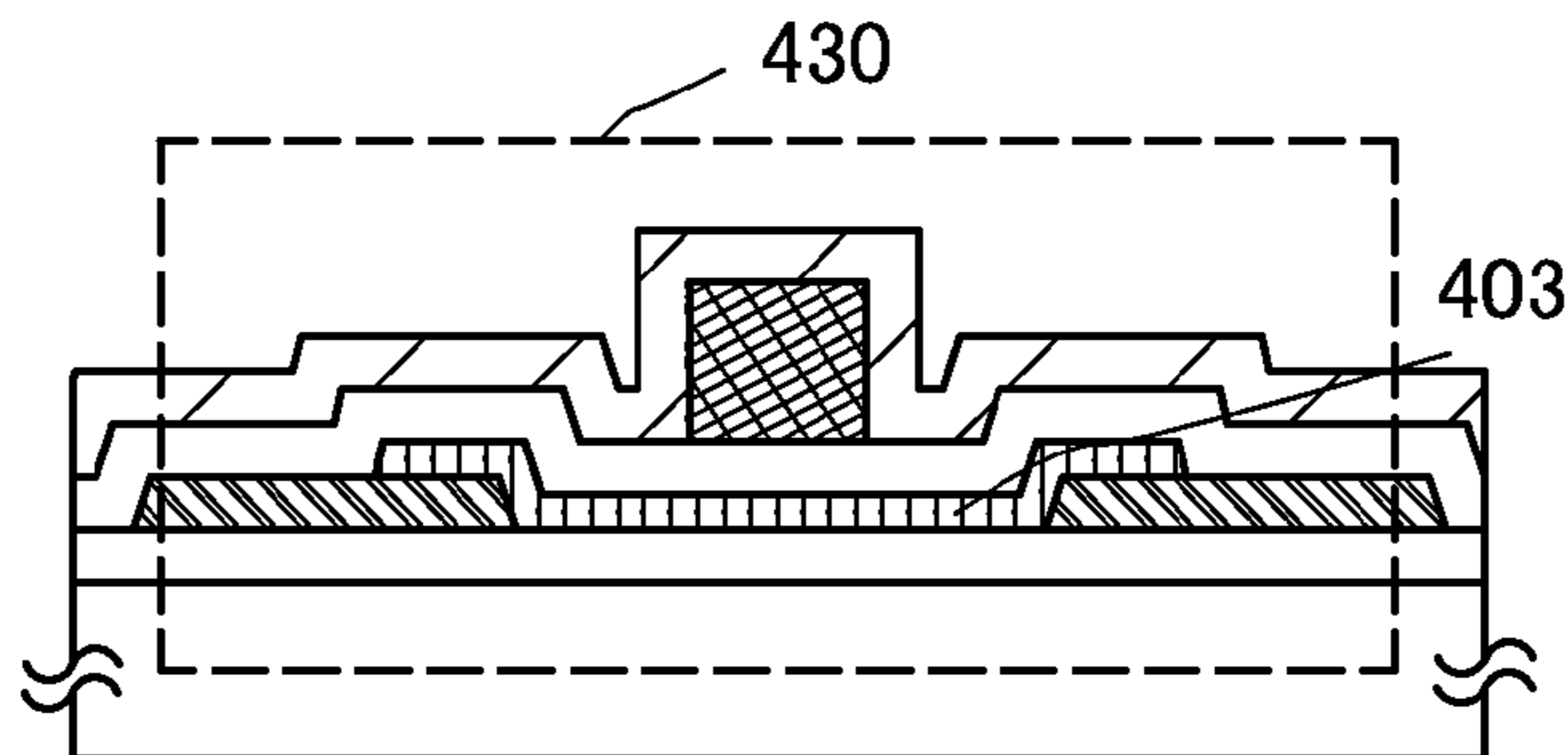
FIG. 5F
