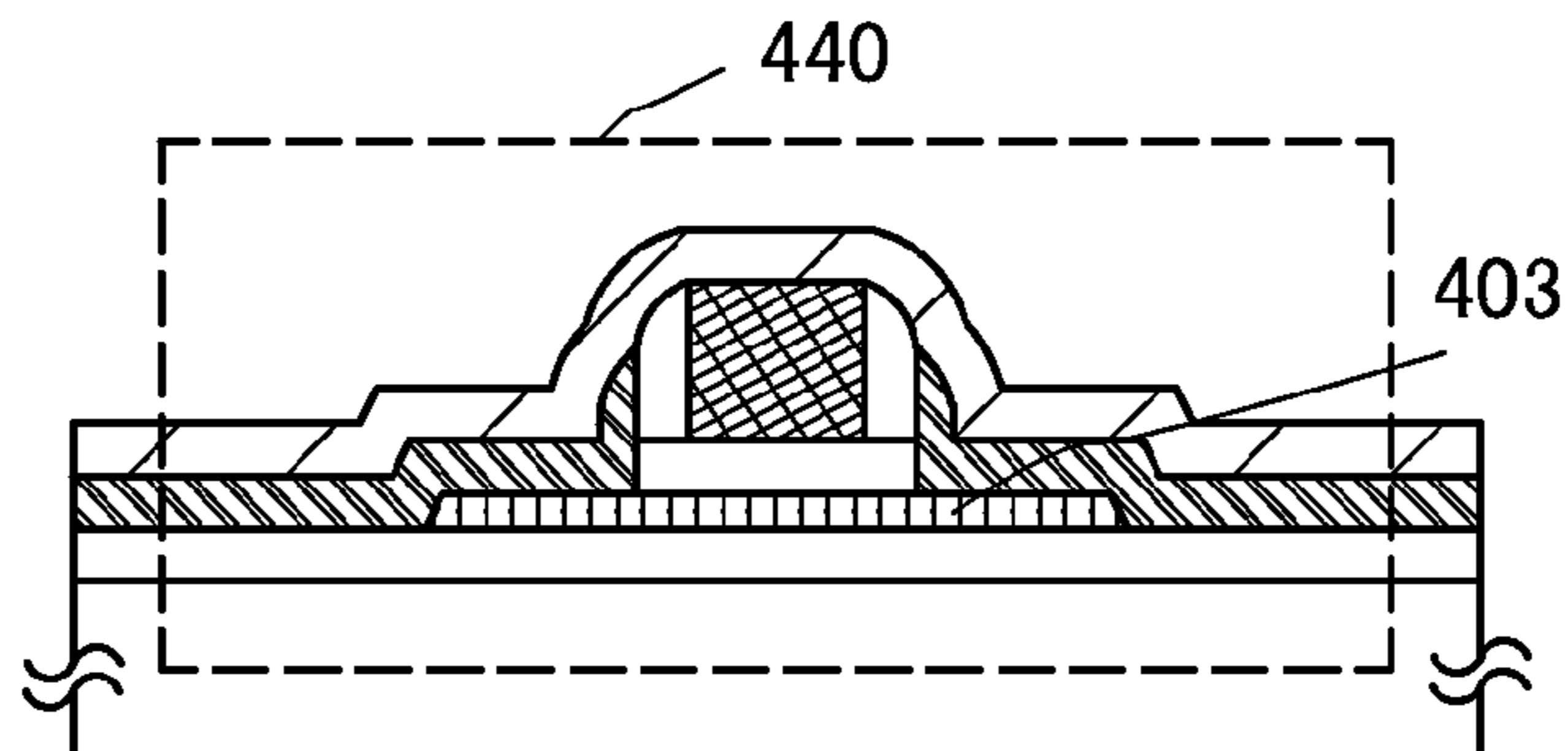
FIG. 1F
