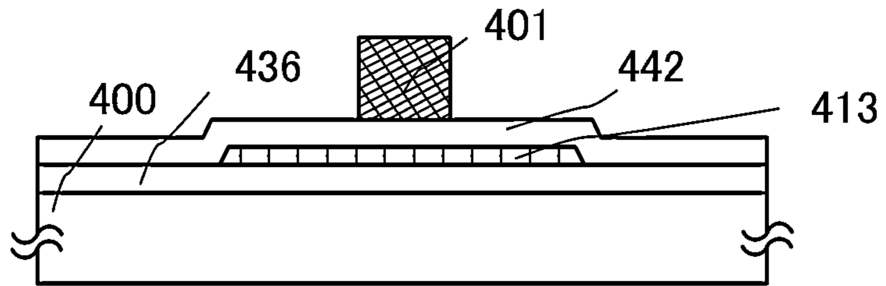
FIG. 3A
