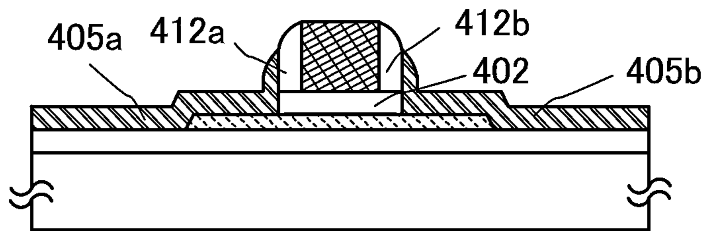
FIG. 3C
