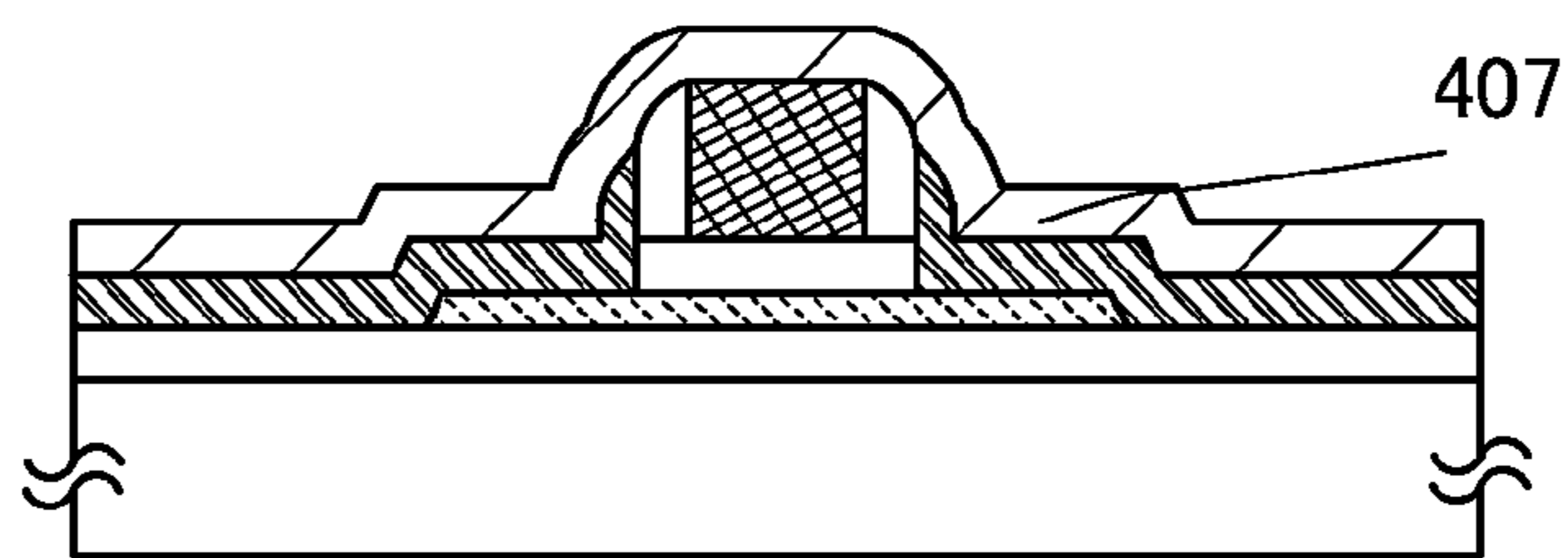
FIG. 1E
