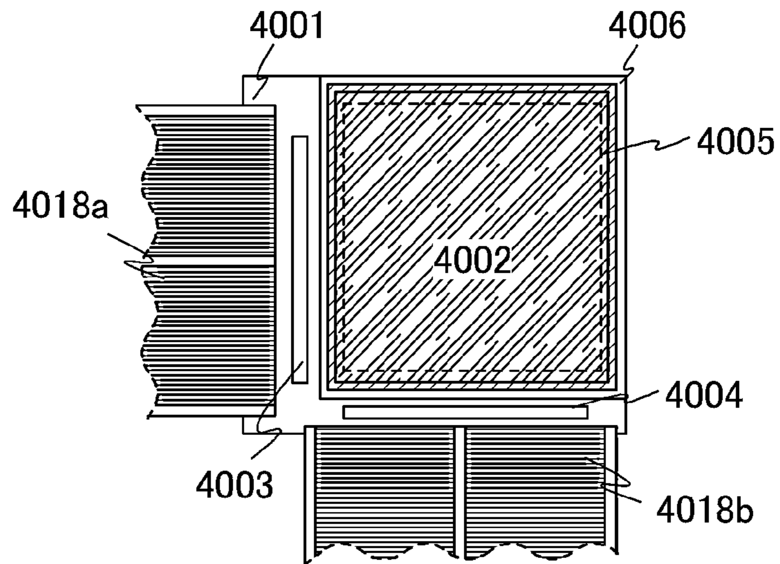
FIG. 20B
