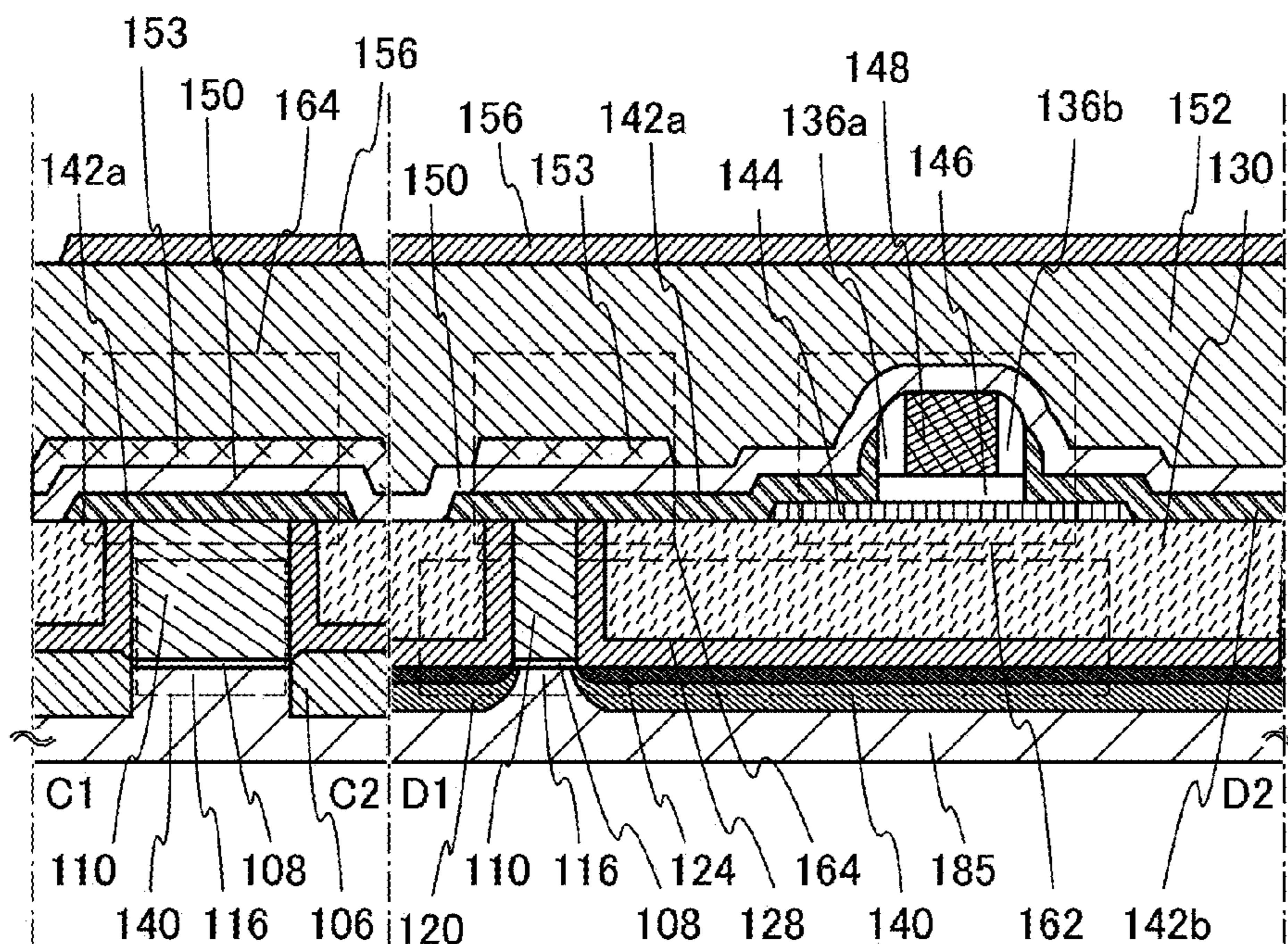
FIG. 19A
