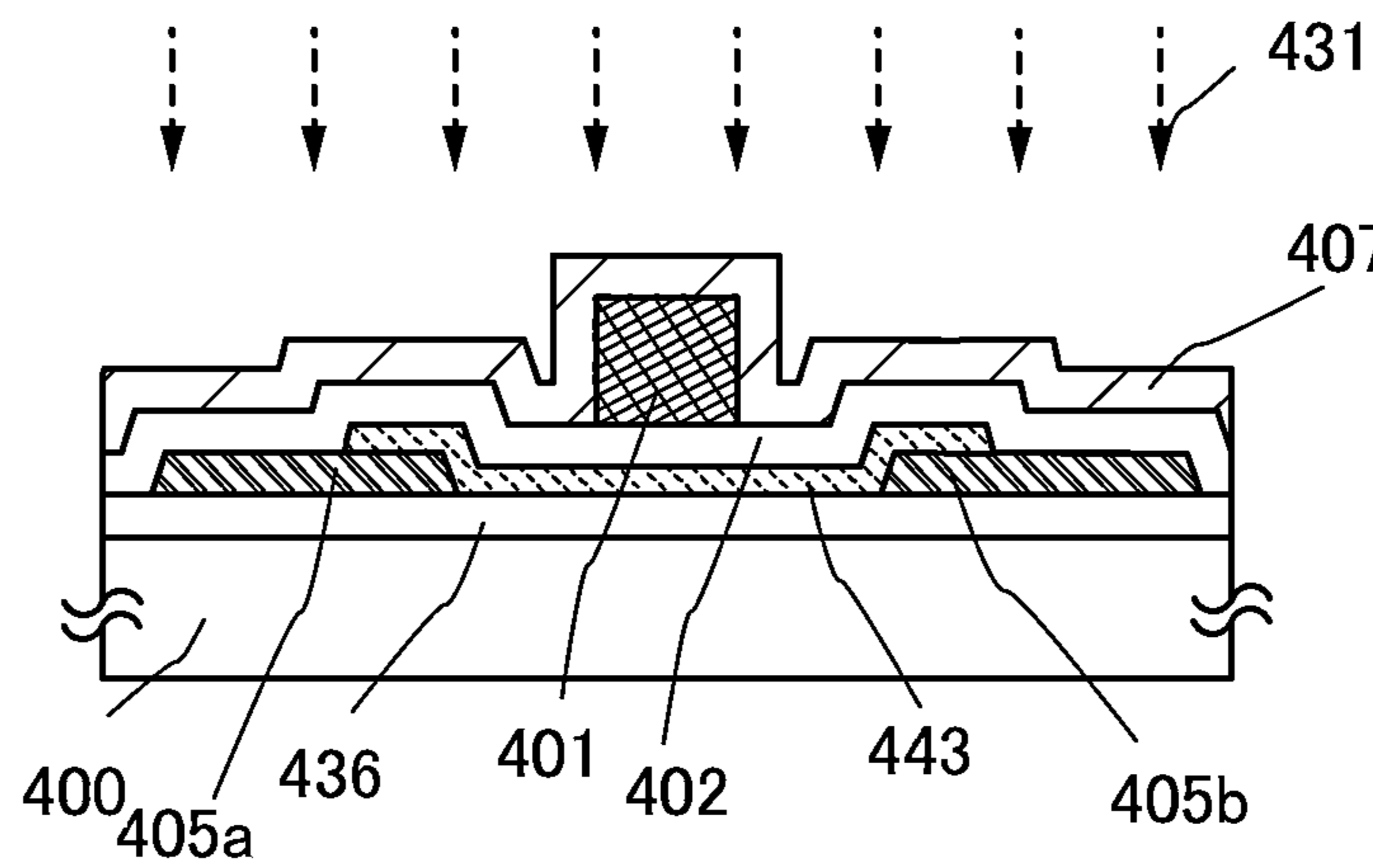
FIG. 6C
