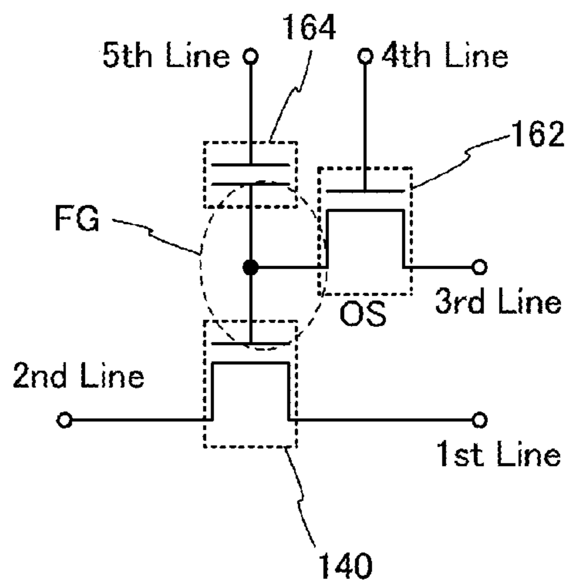
FIG. 19C
