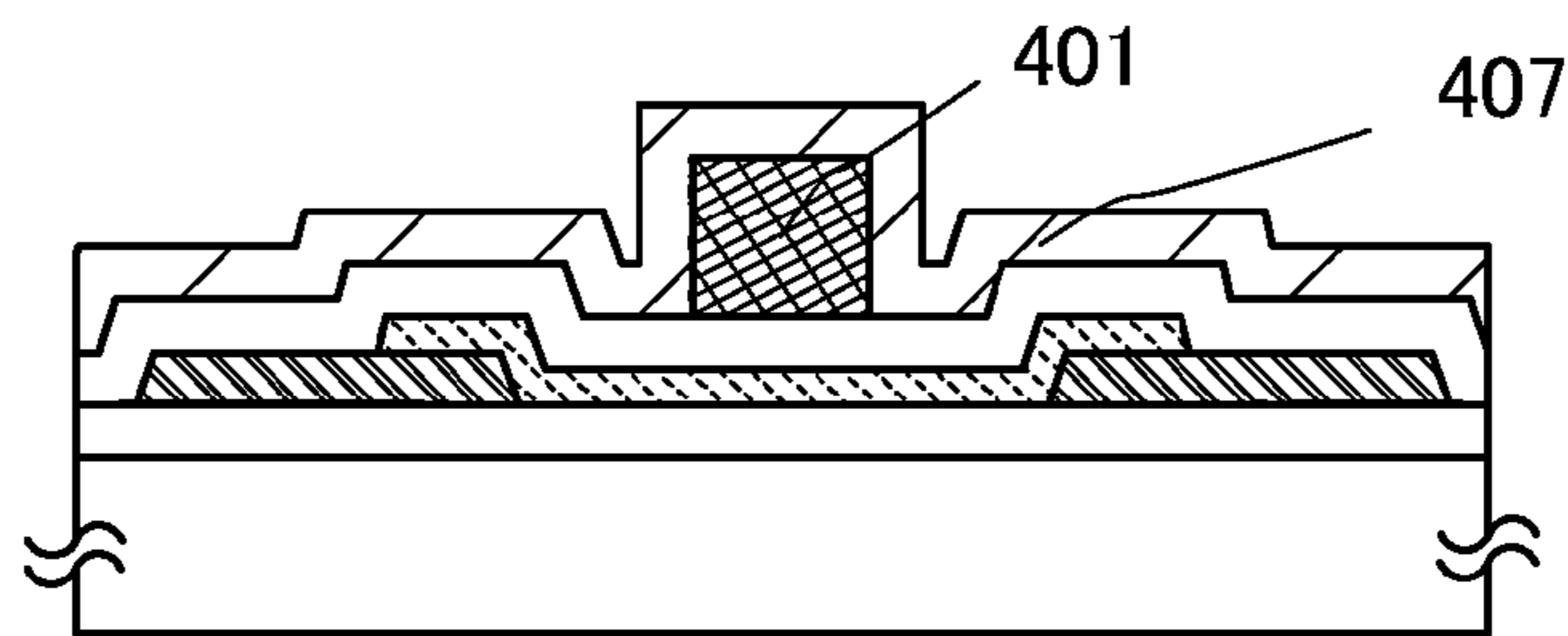
FIG. 5E
