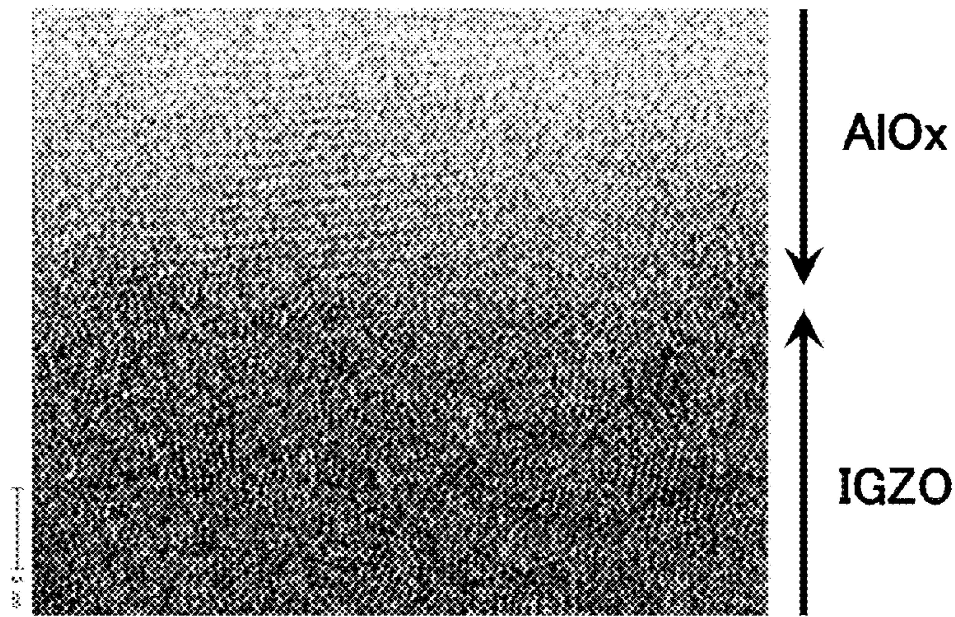
FIG. 16B
