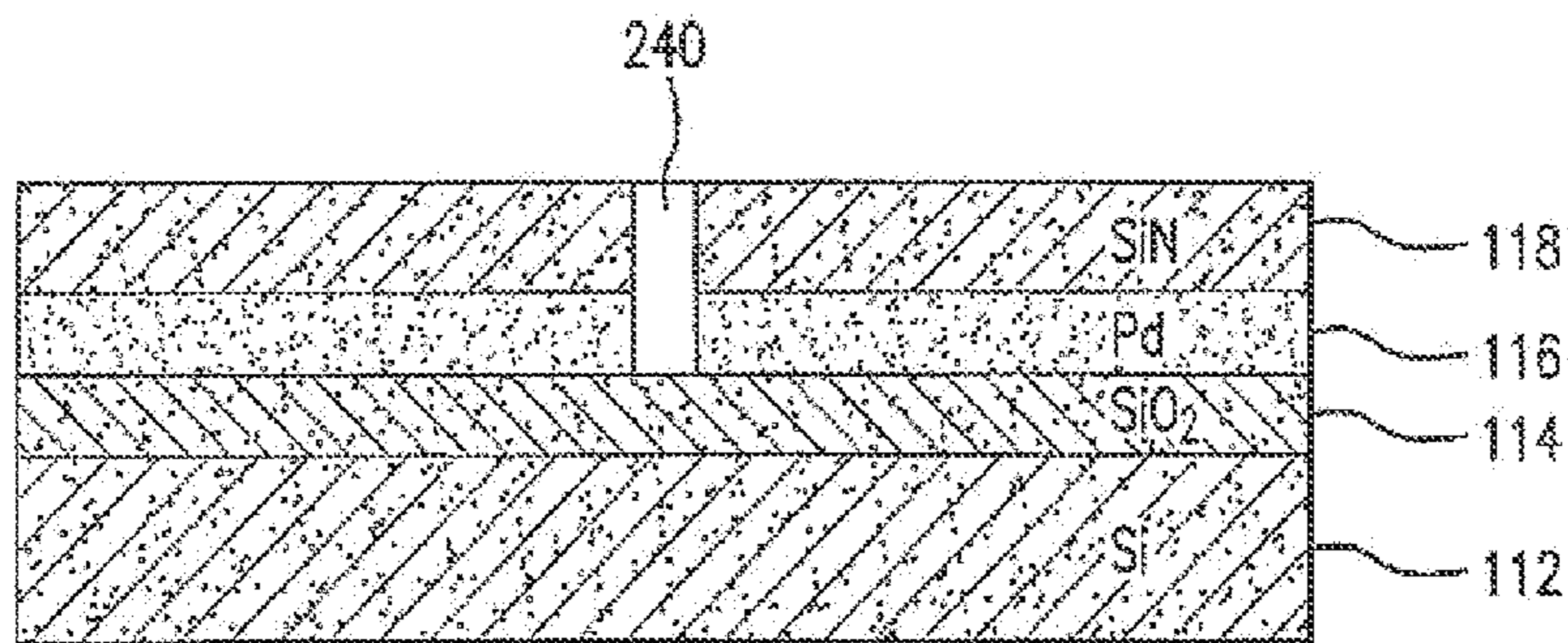
Etch Back FIG.2E
