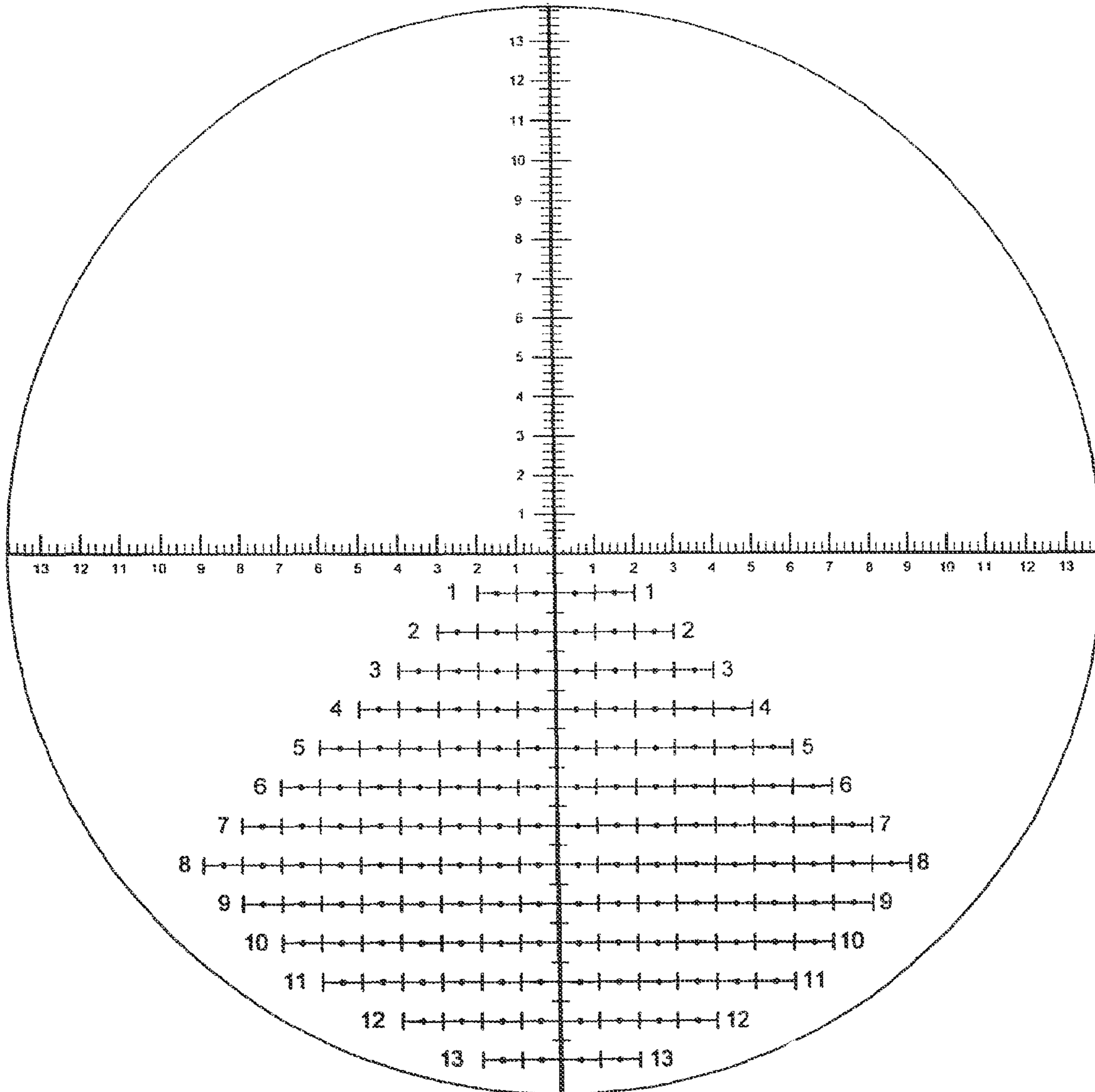
FIG. 26
