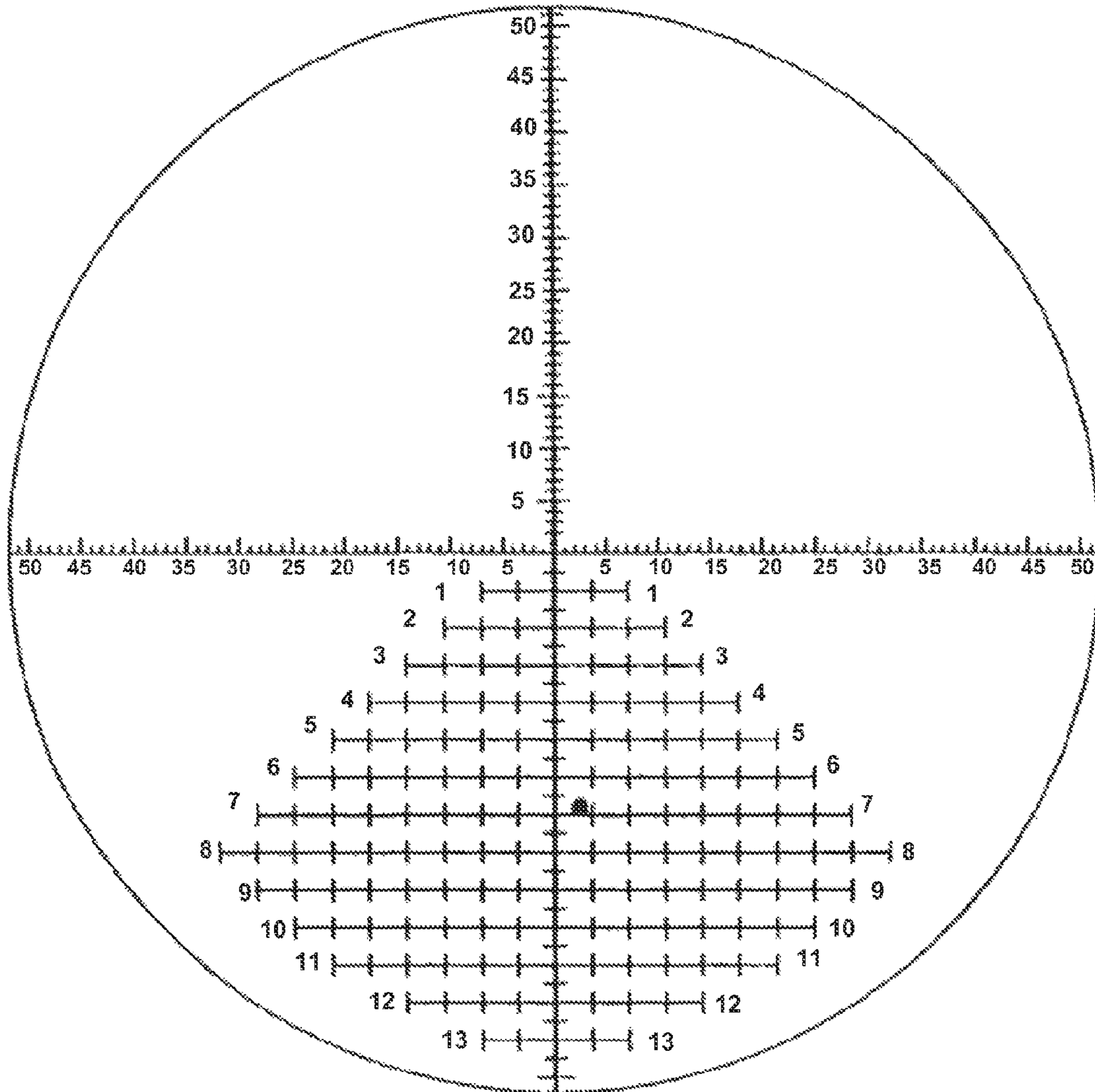
FIG. 19A
