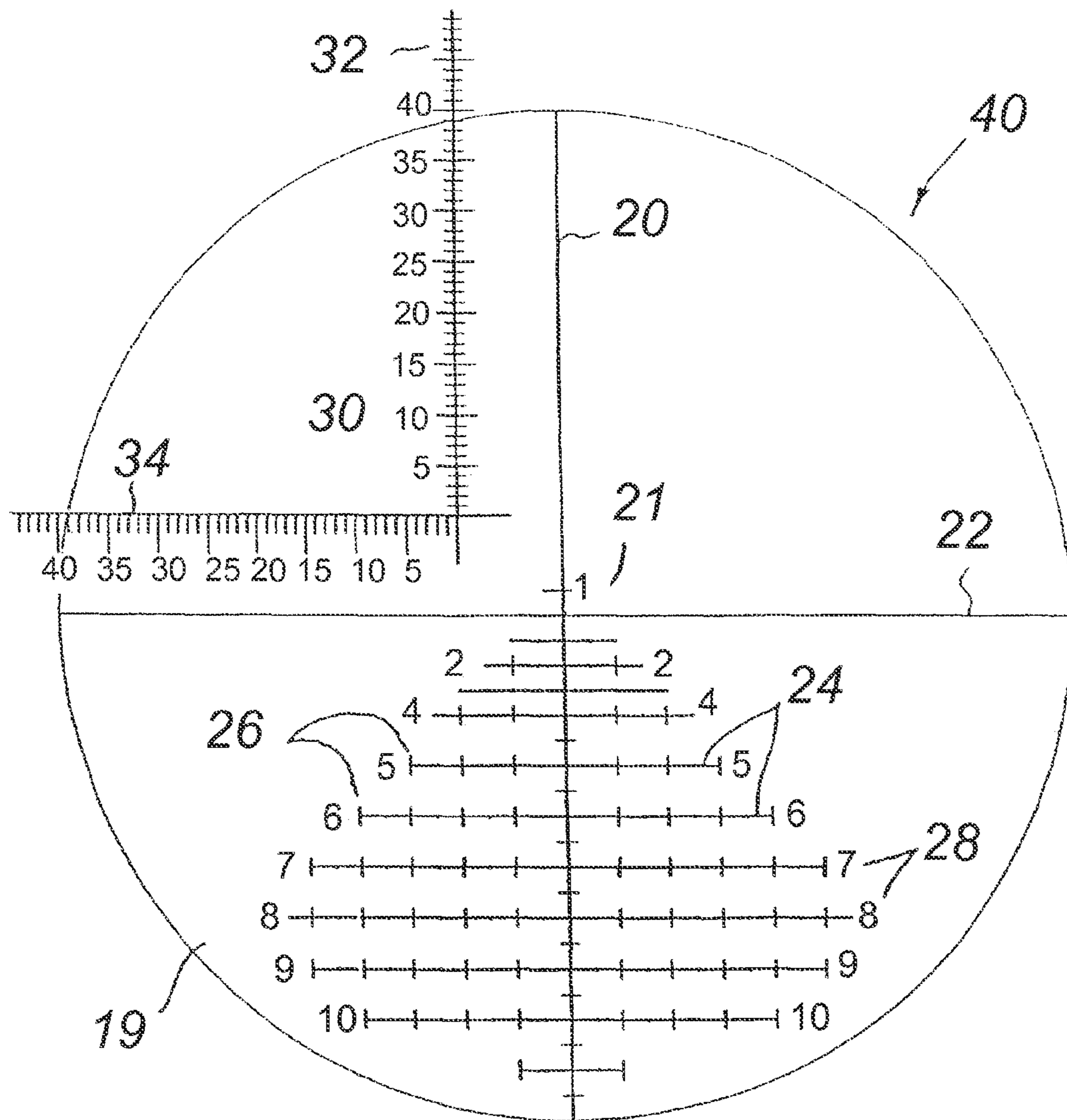
FIG. 10
