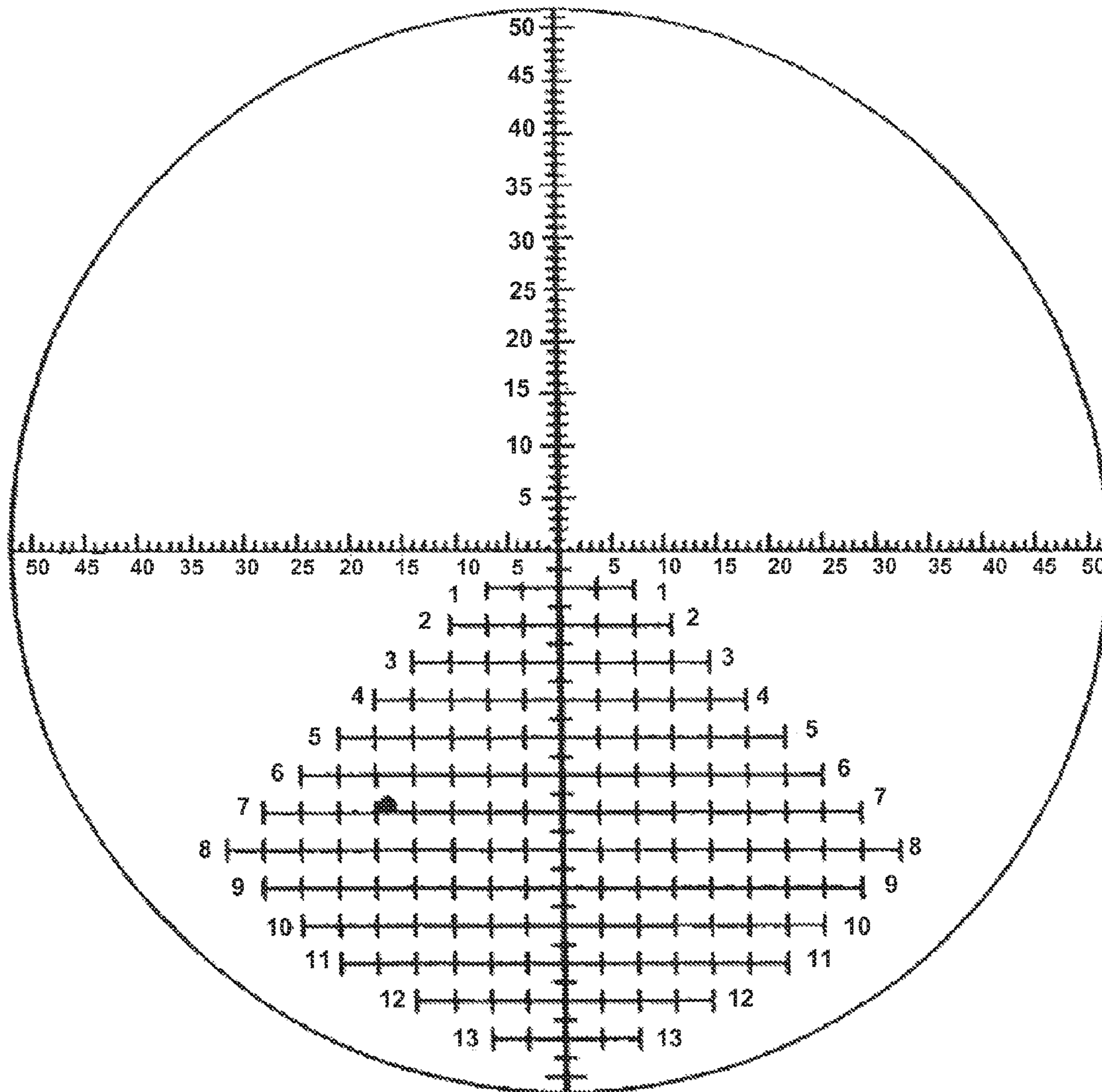
FIG. 19B
