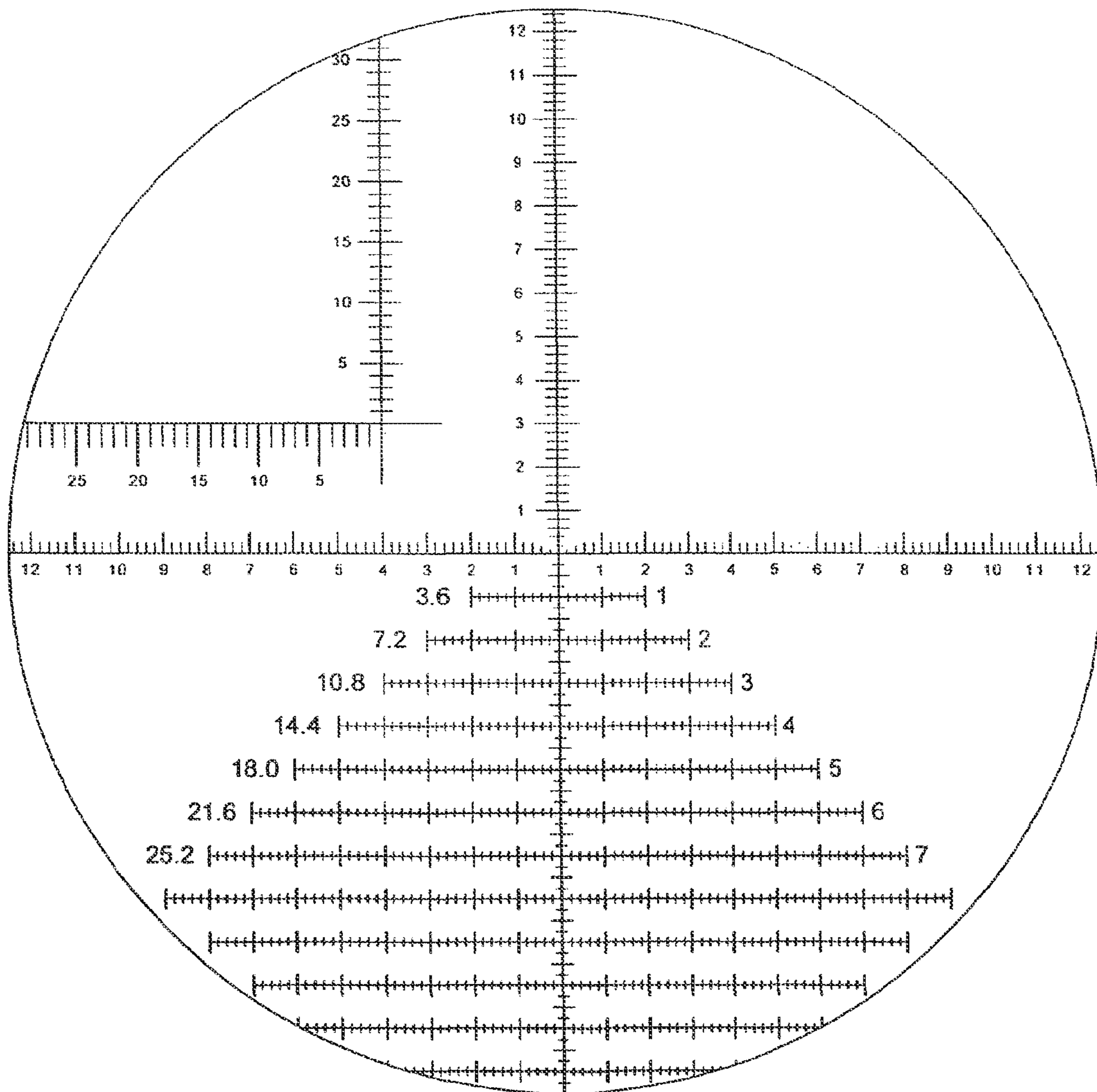
FIG. 22
