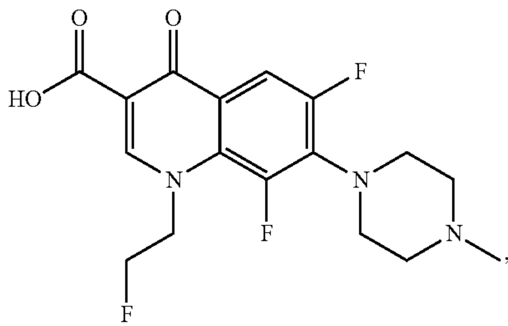
Fleroxacin
