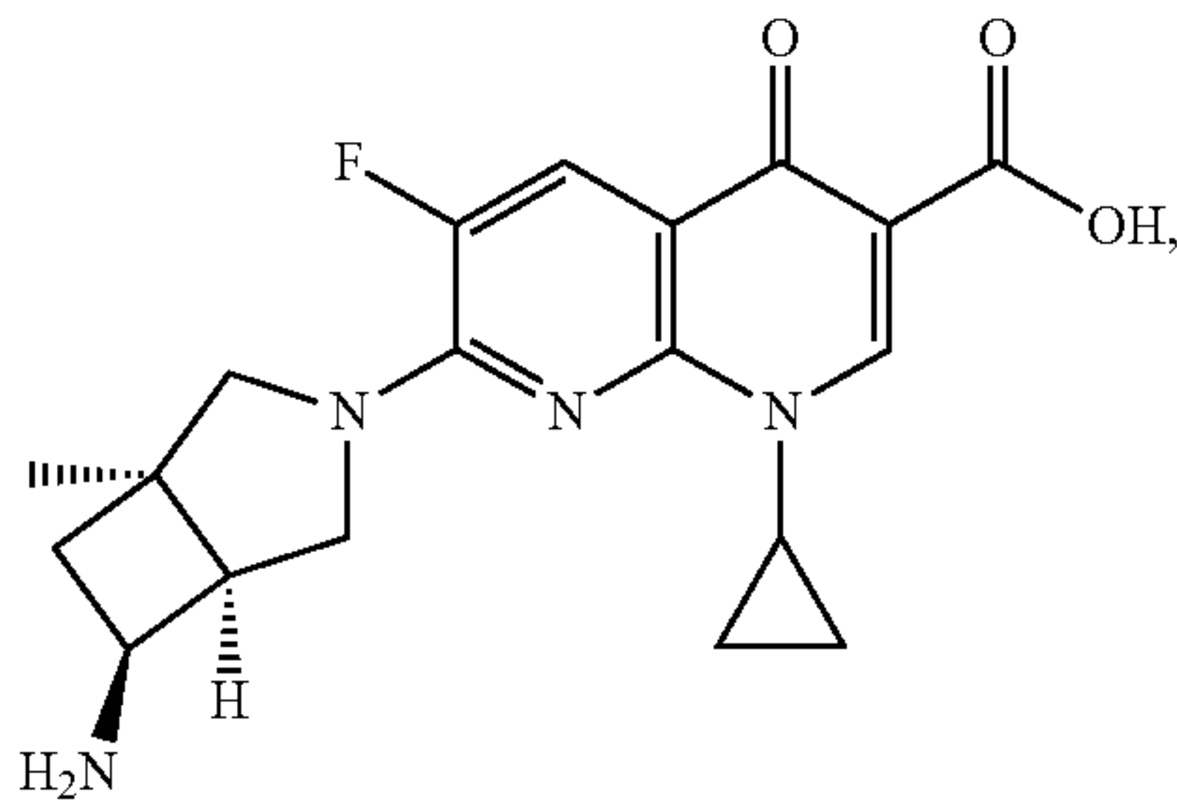
Ecenofloxacin
