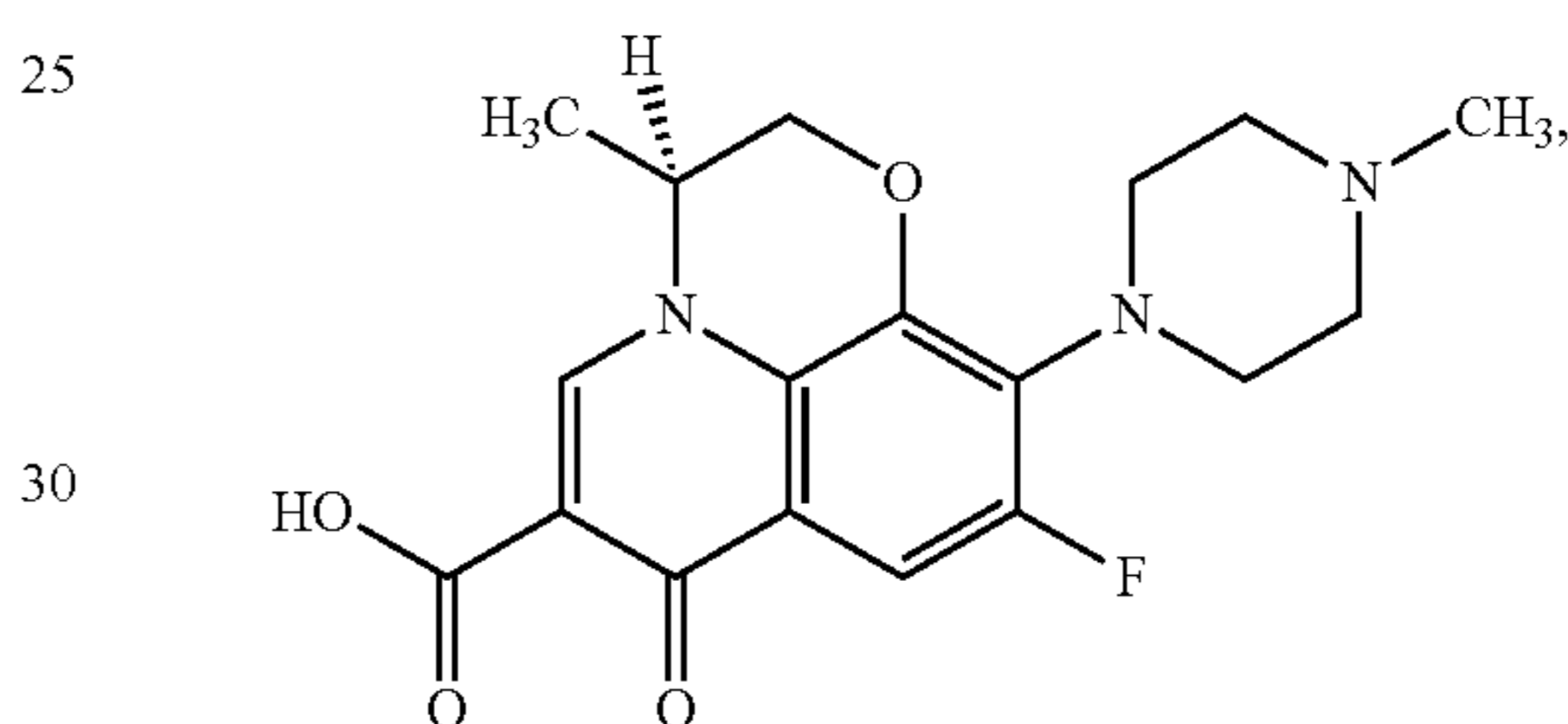
Levofloxacina
