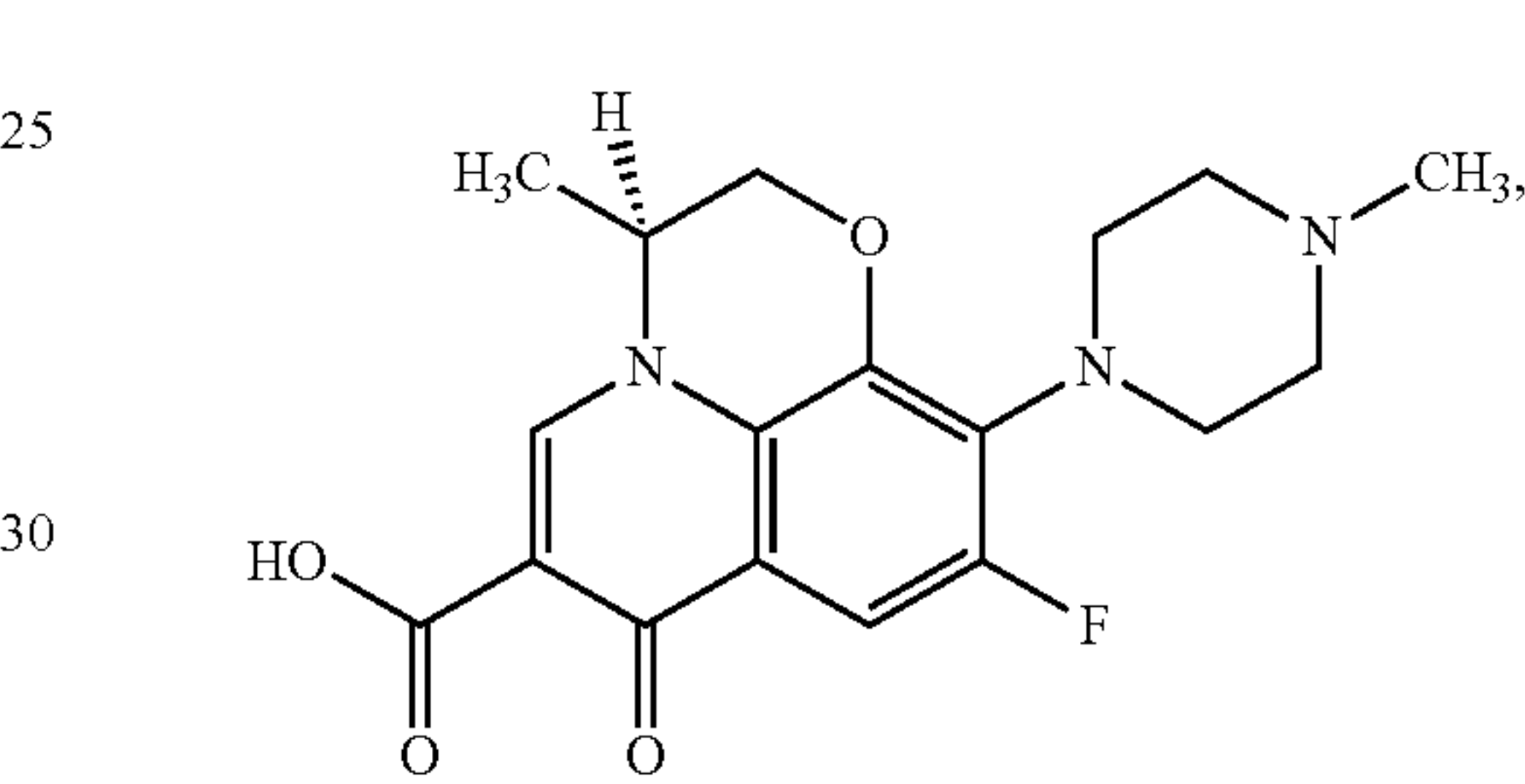
Levofloxacin
