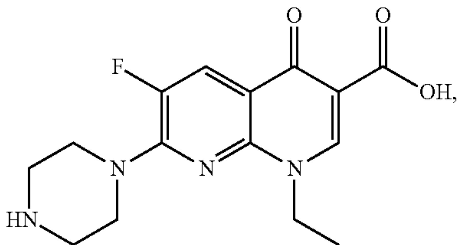
Enoxacin
