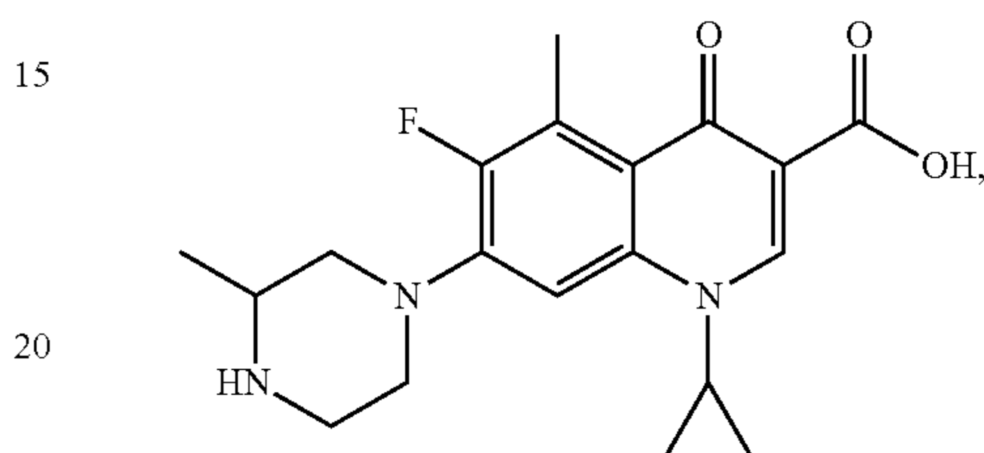
Grepafloxacina
