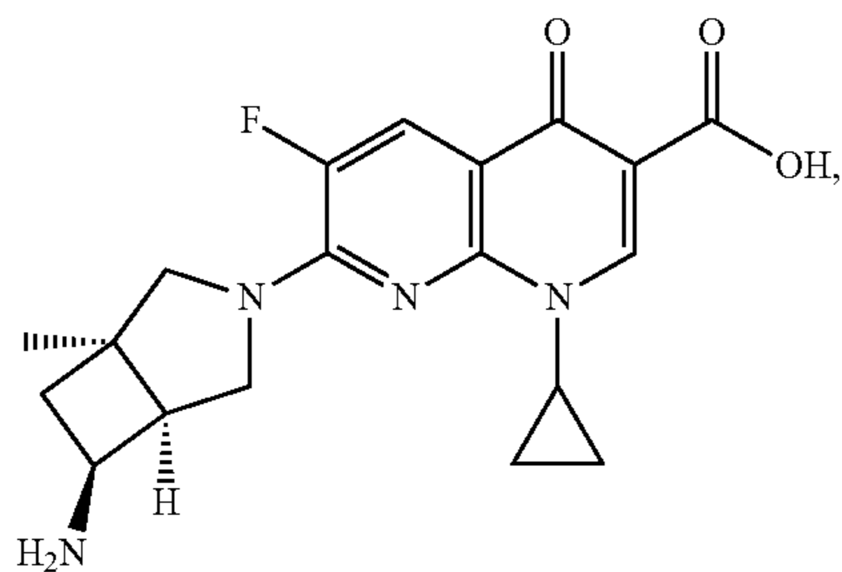
Ecenofloxacin
