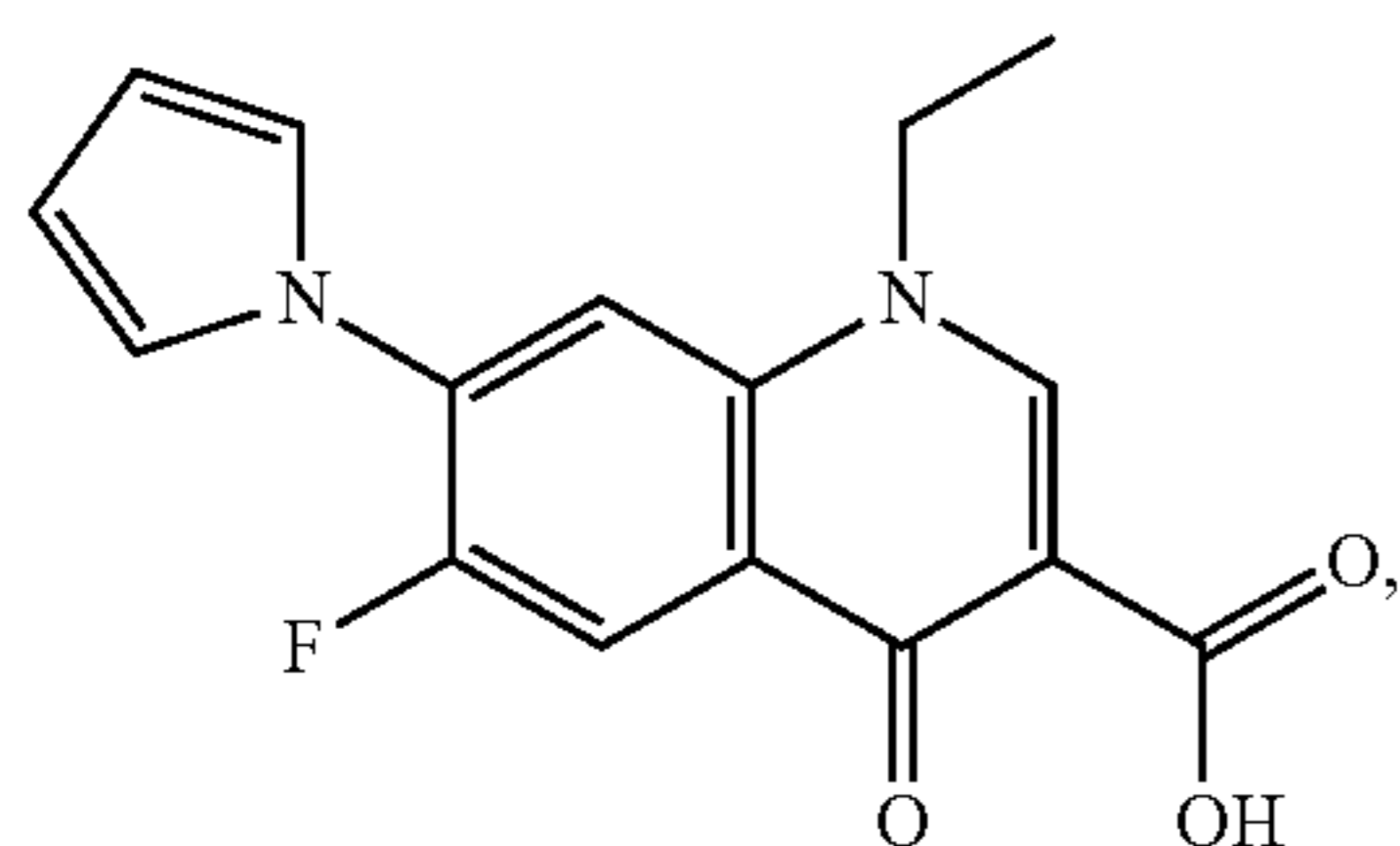
Irloxacin
