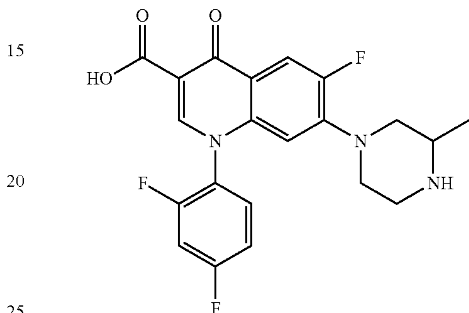
Temafloxacin
