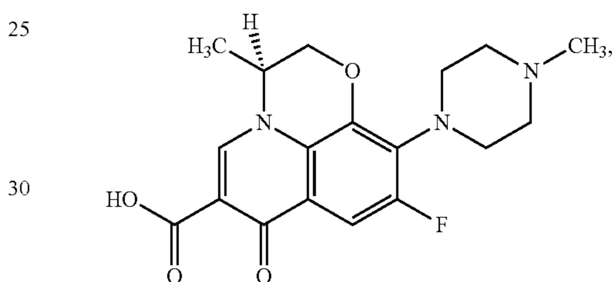
Levofloxacina
