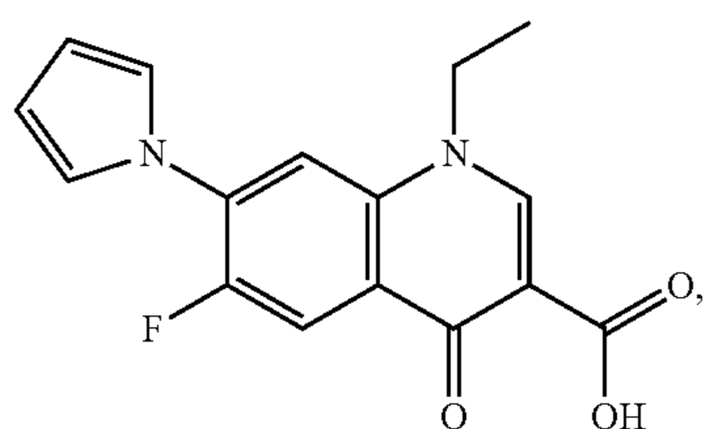
Irloxacin
