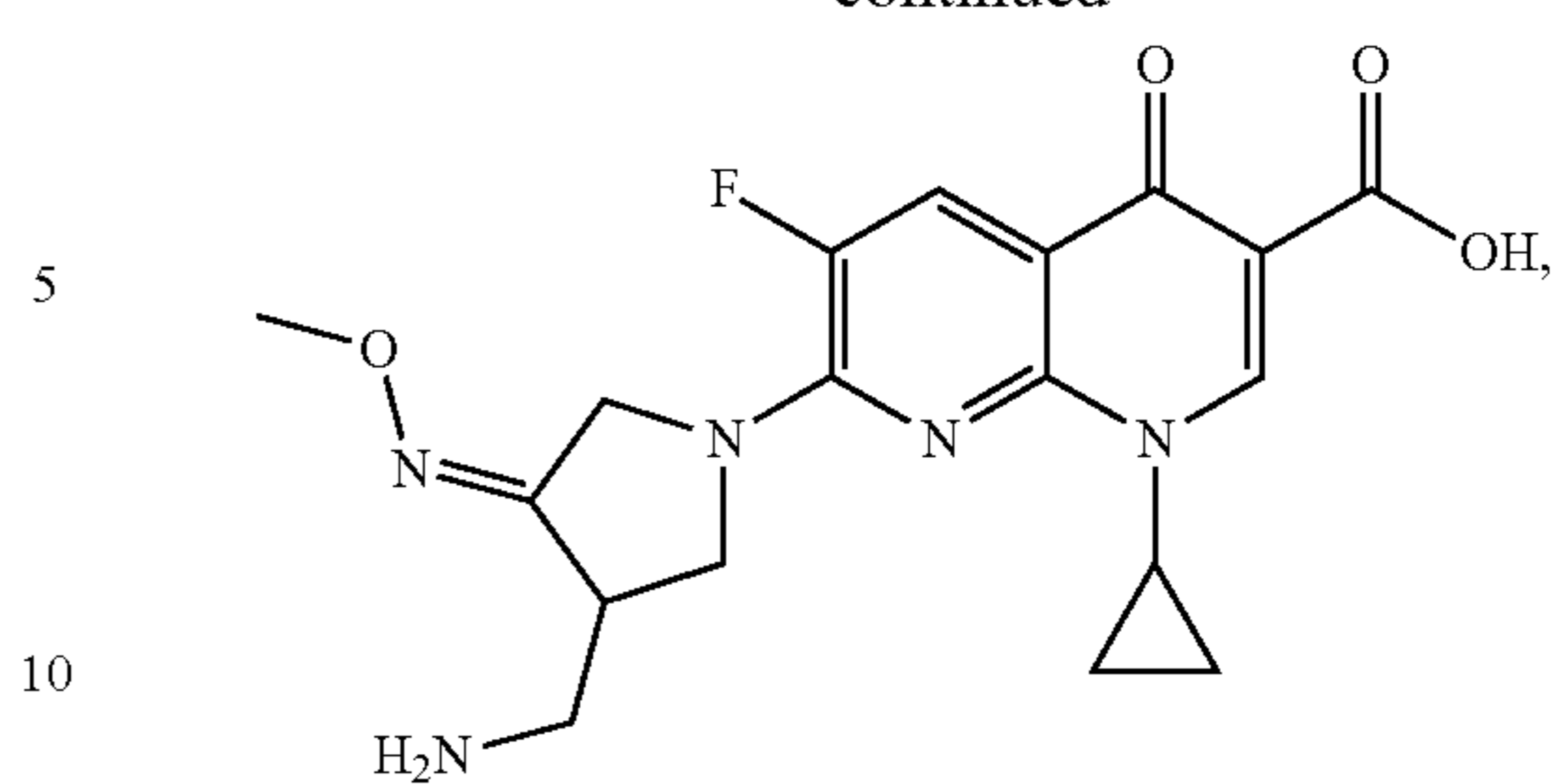
Gemifloxacina
