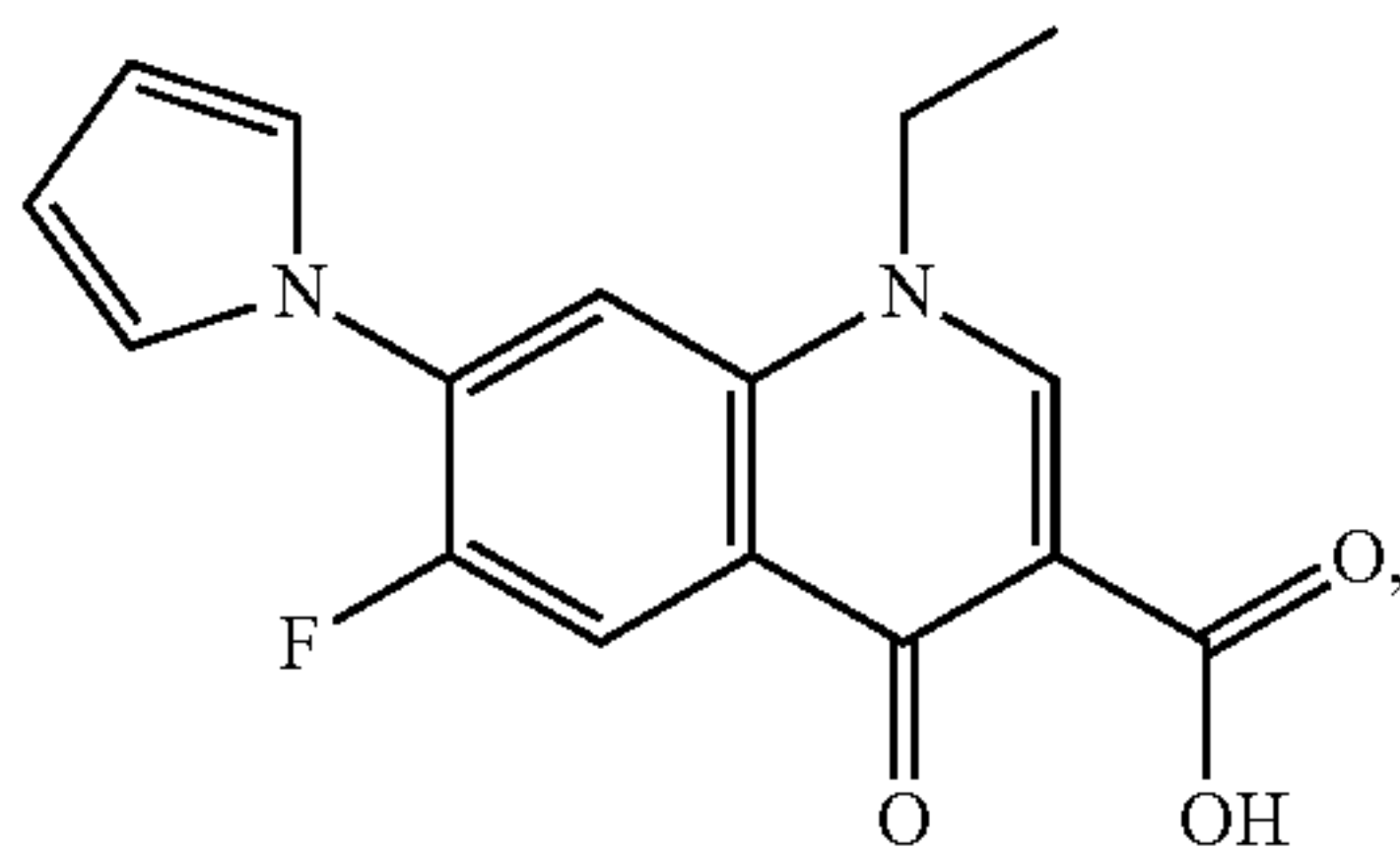
Irloxacin
