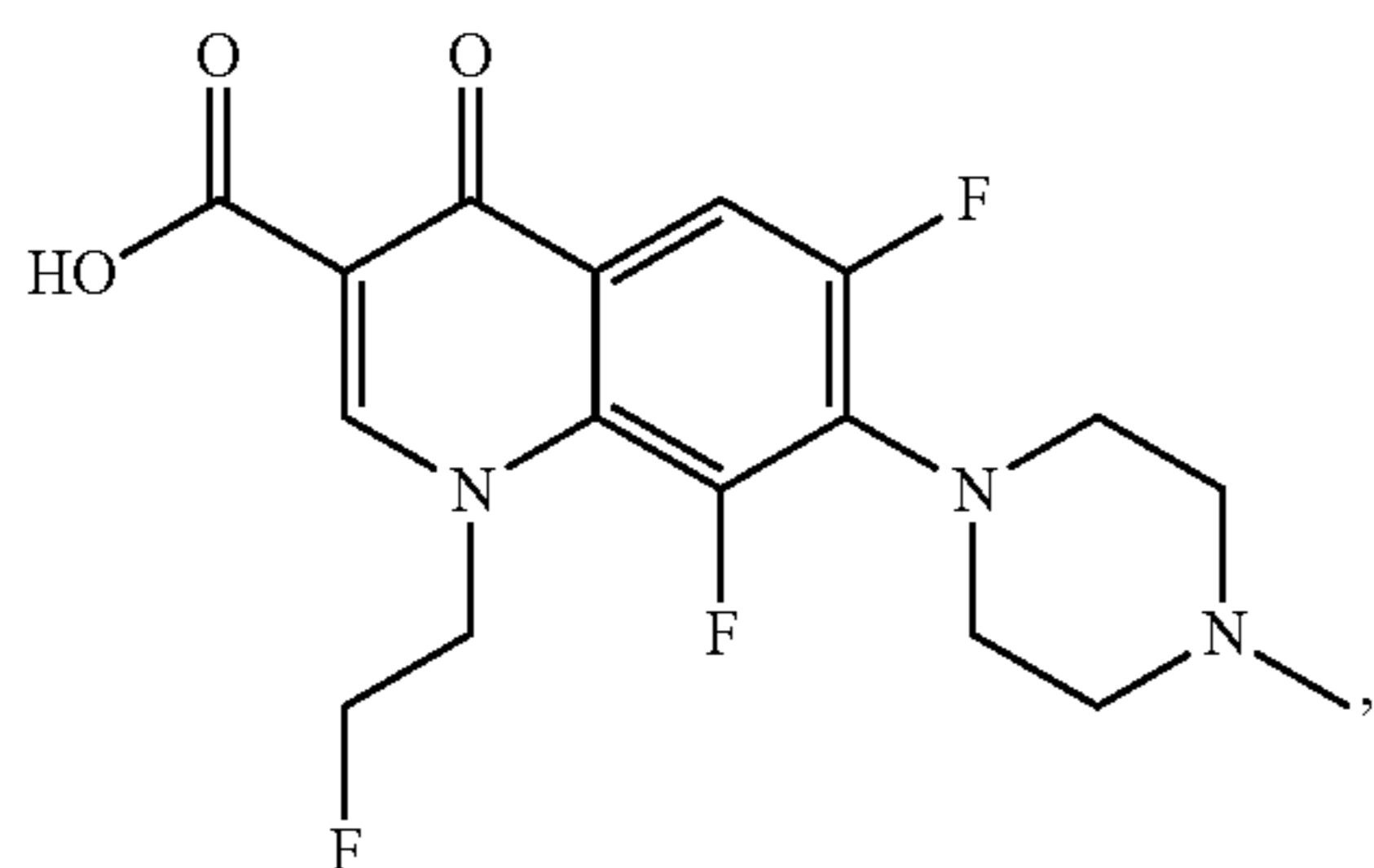
Fleroxacin
