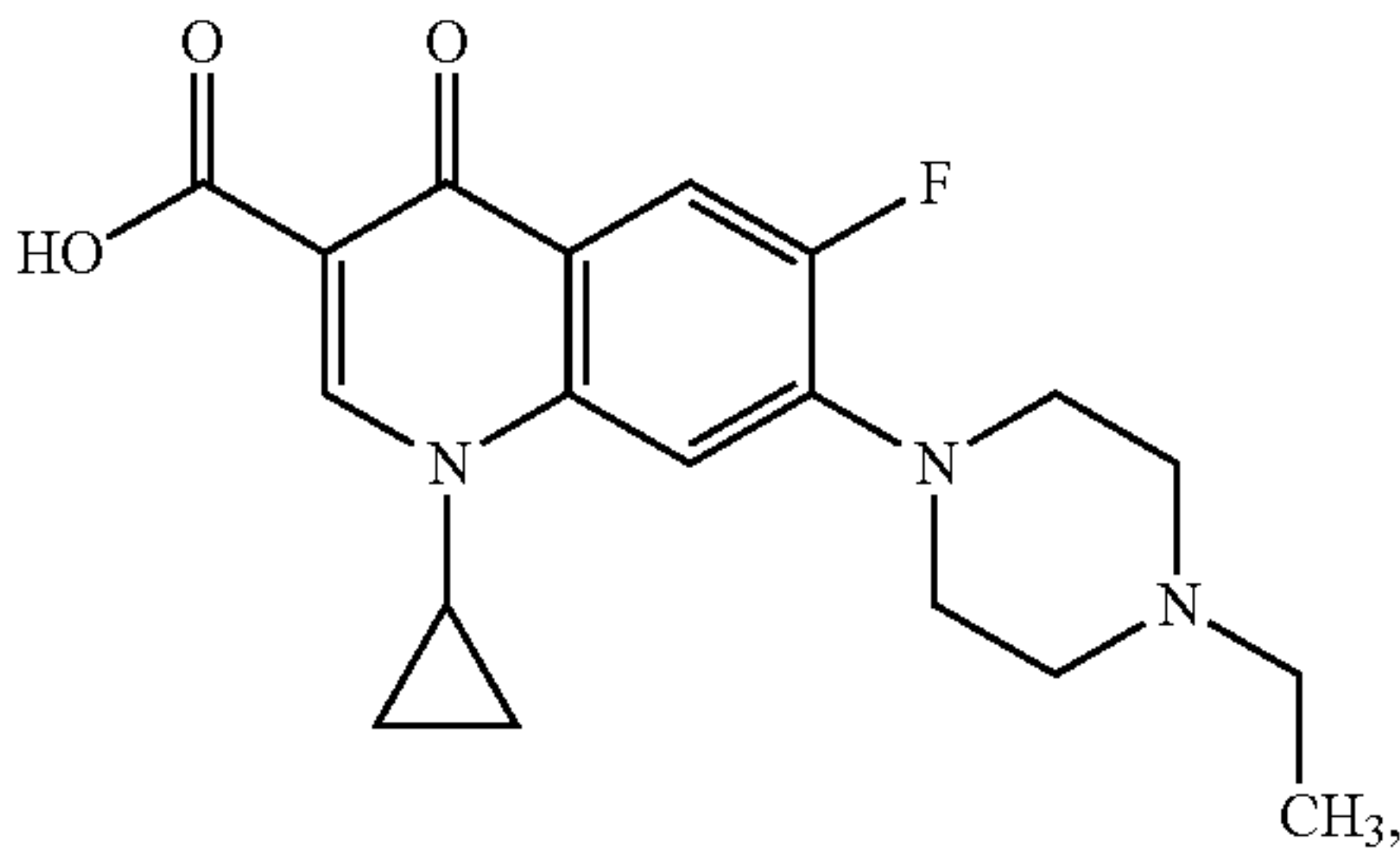
Enoxacin
