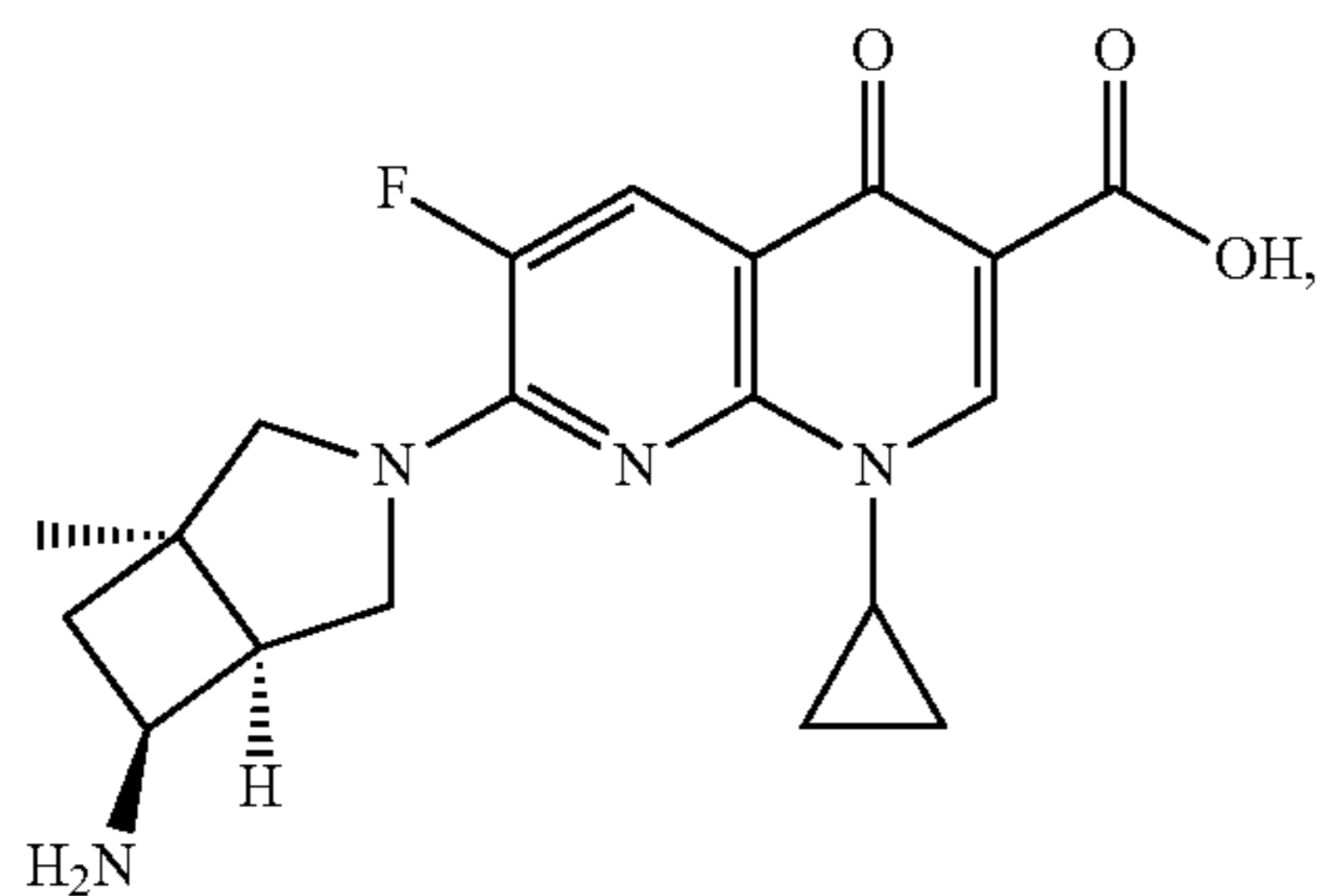
Ecenofloxacin
