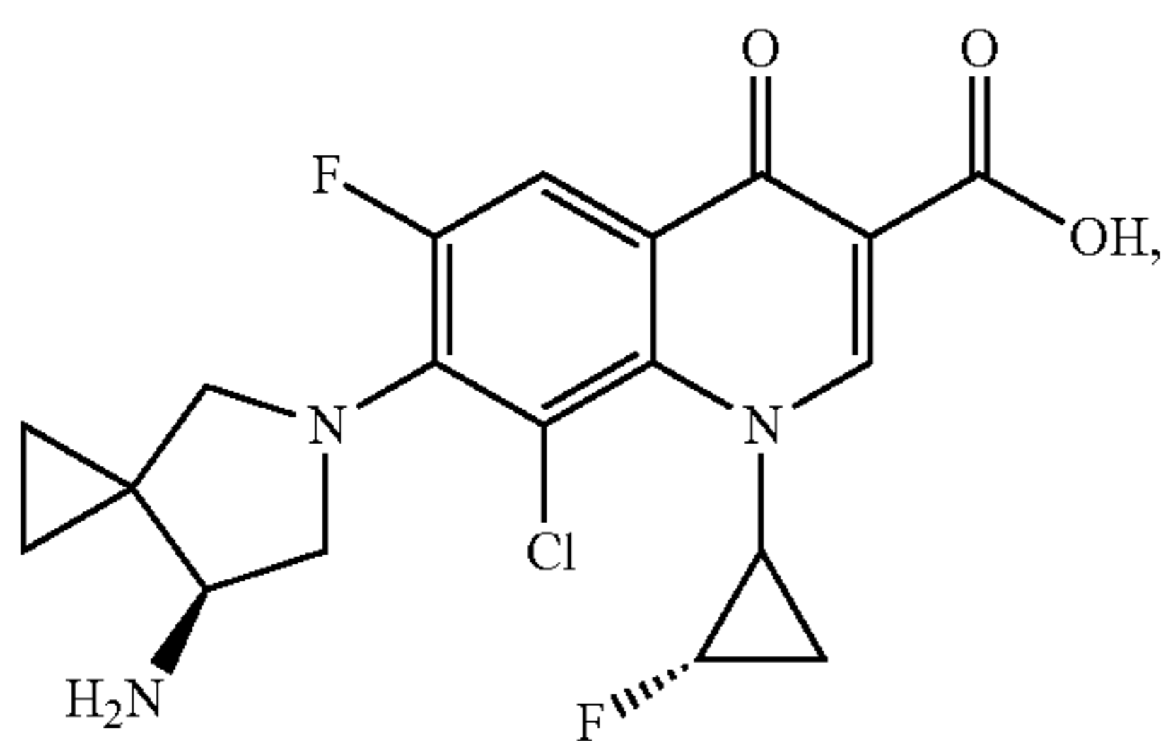
Sitafloxacin
