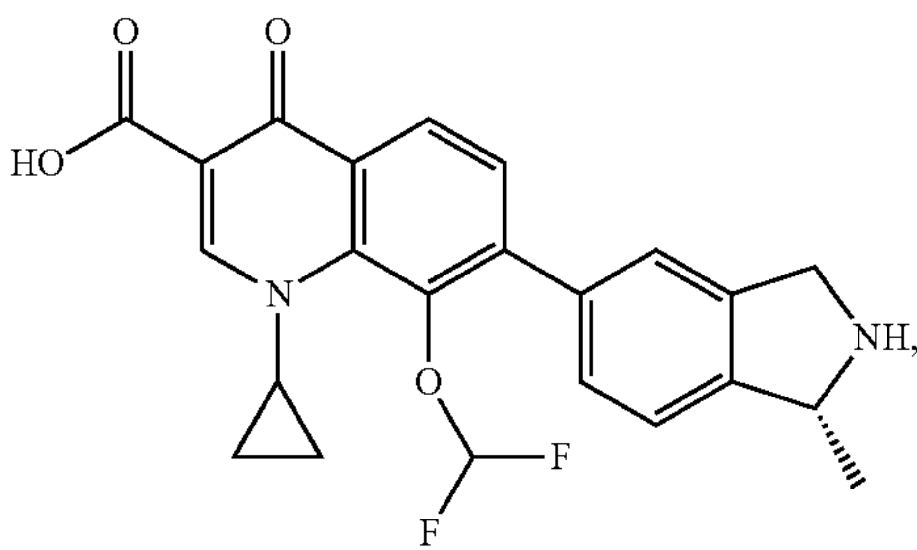
Garenoxacin
