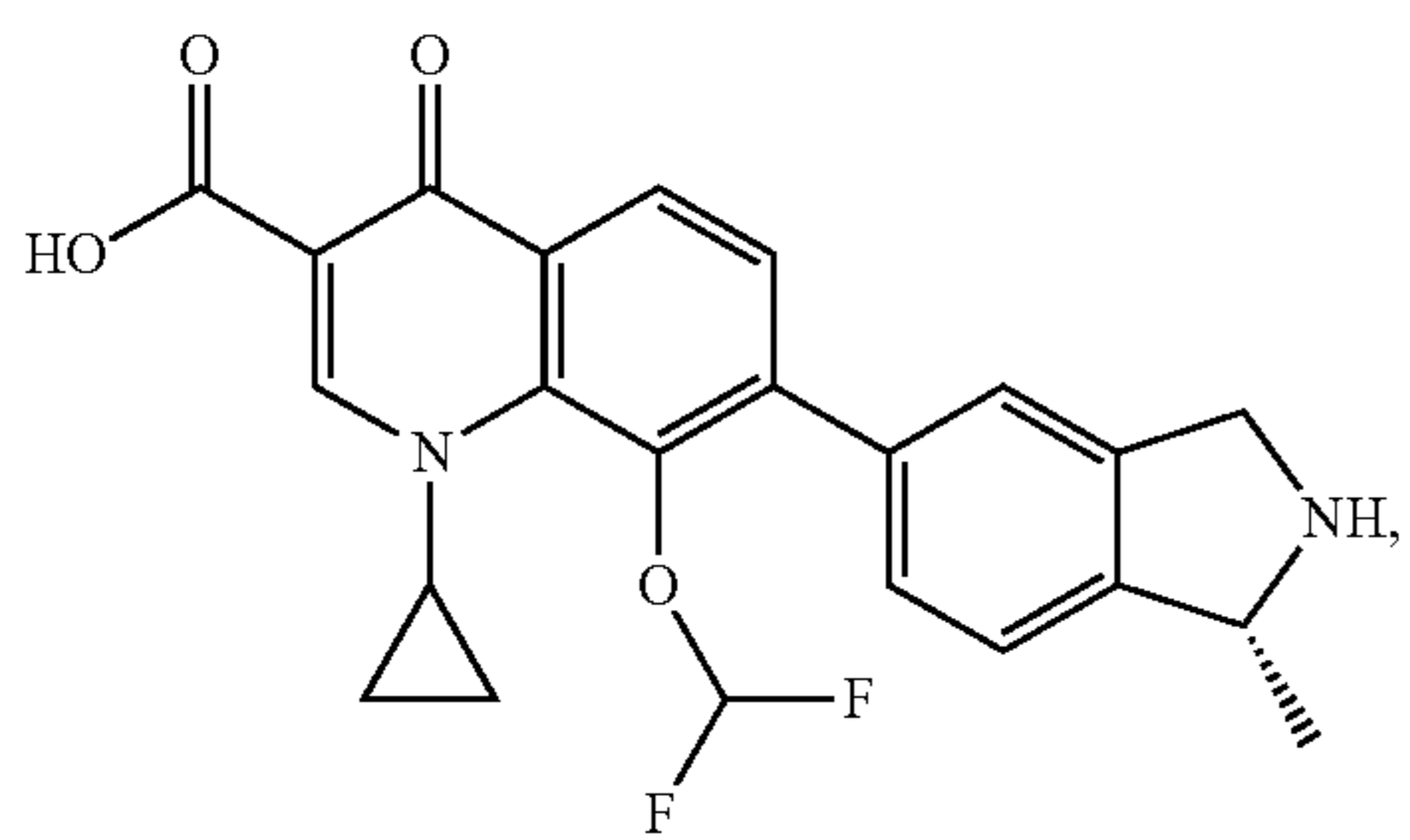
Garenoxacin
