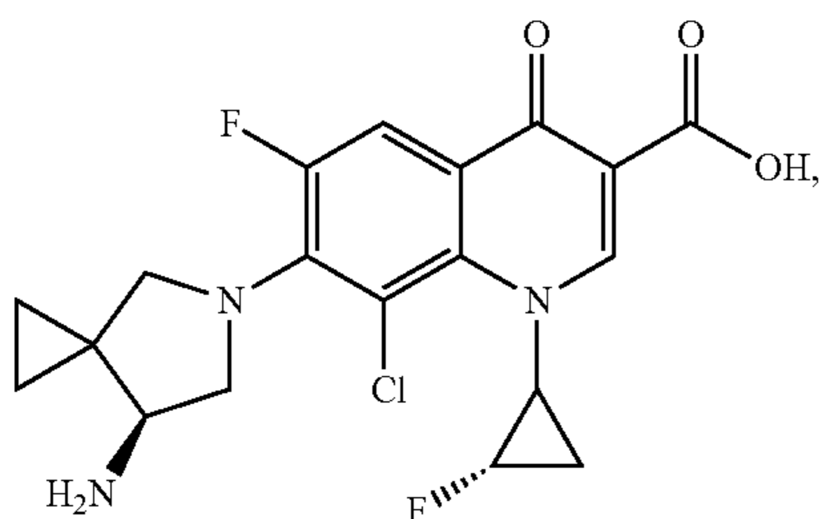
Sitafloxacin
