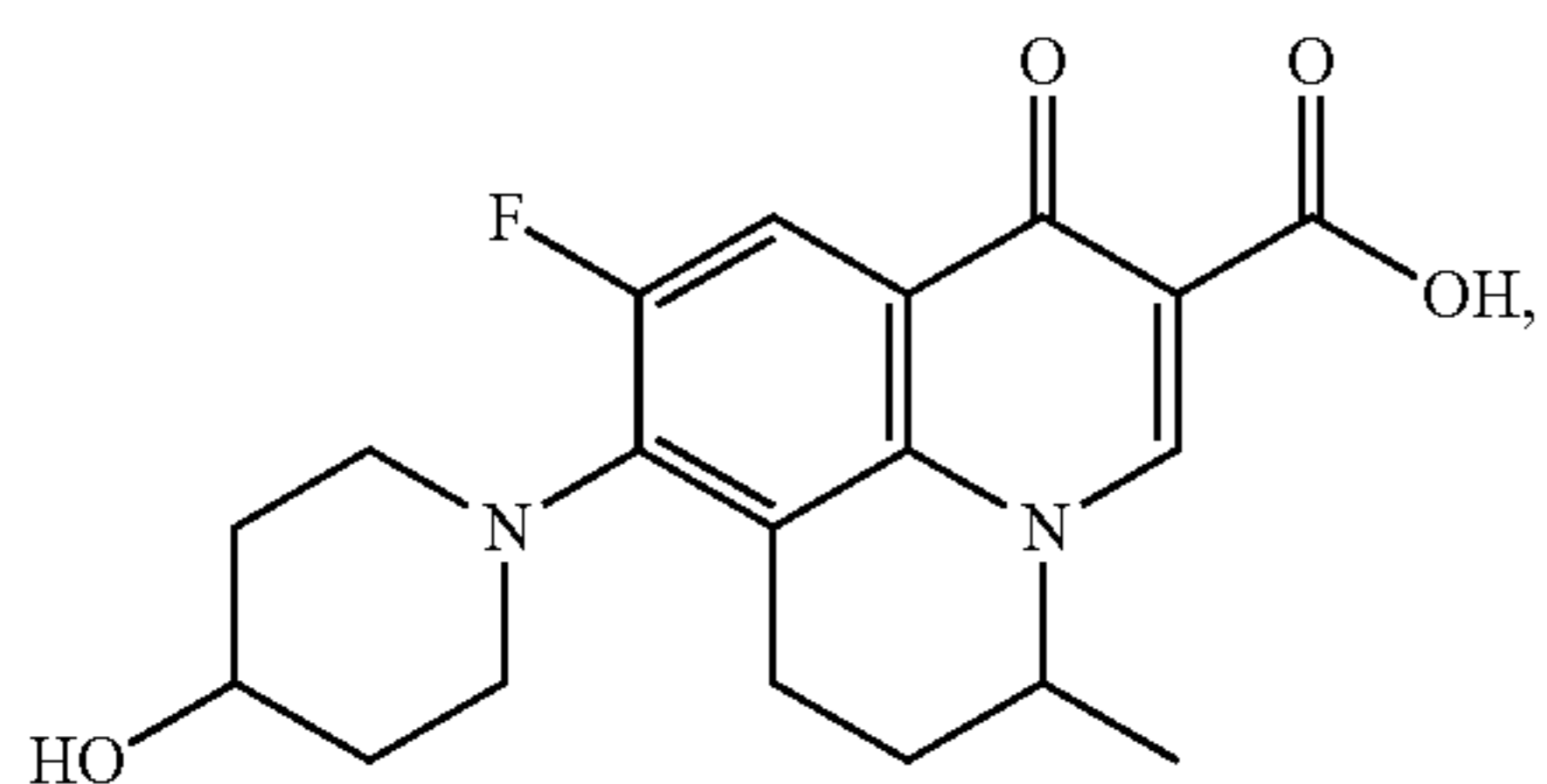
Nadifloxacin
