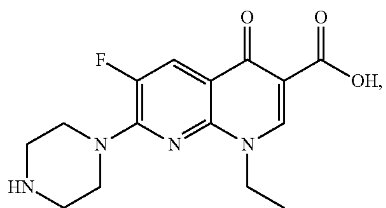
Enoxacin
