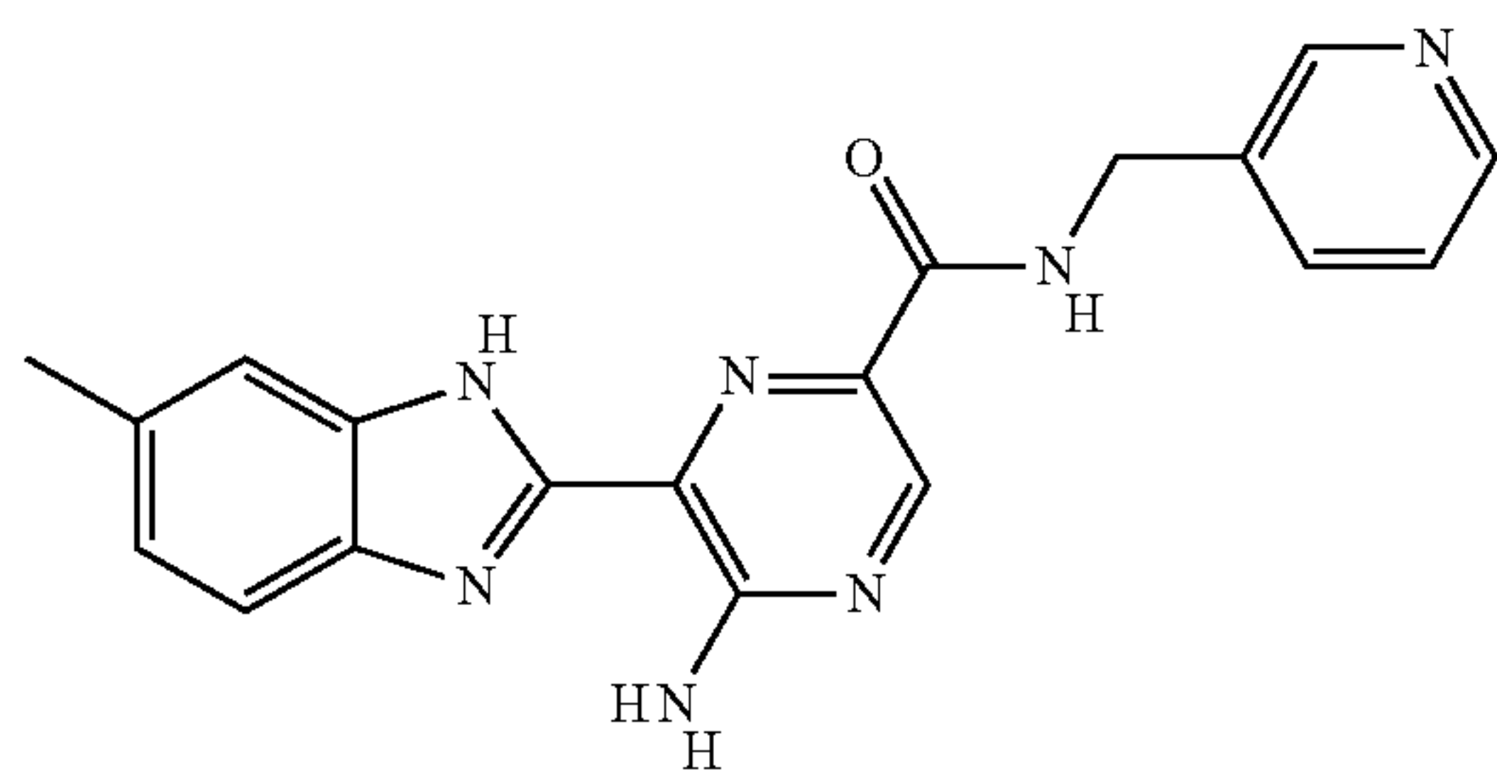
II-70
