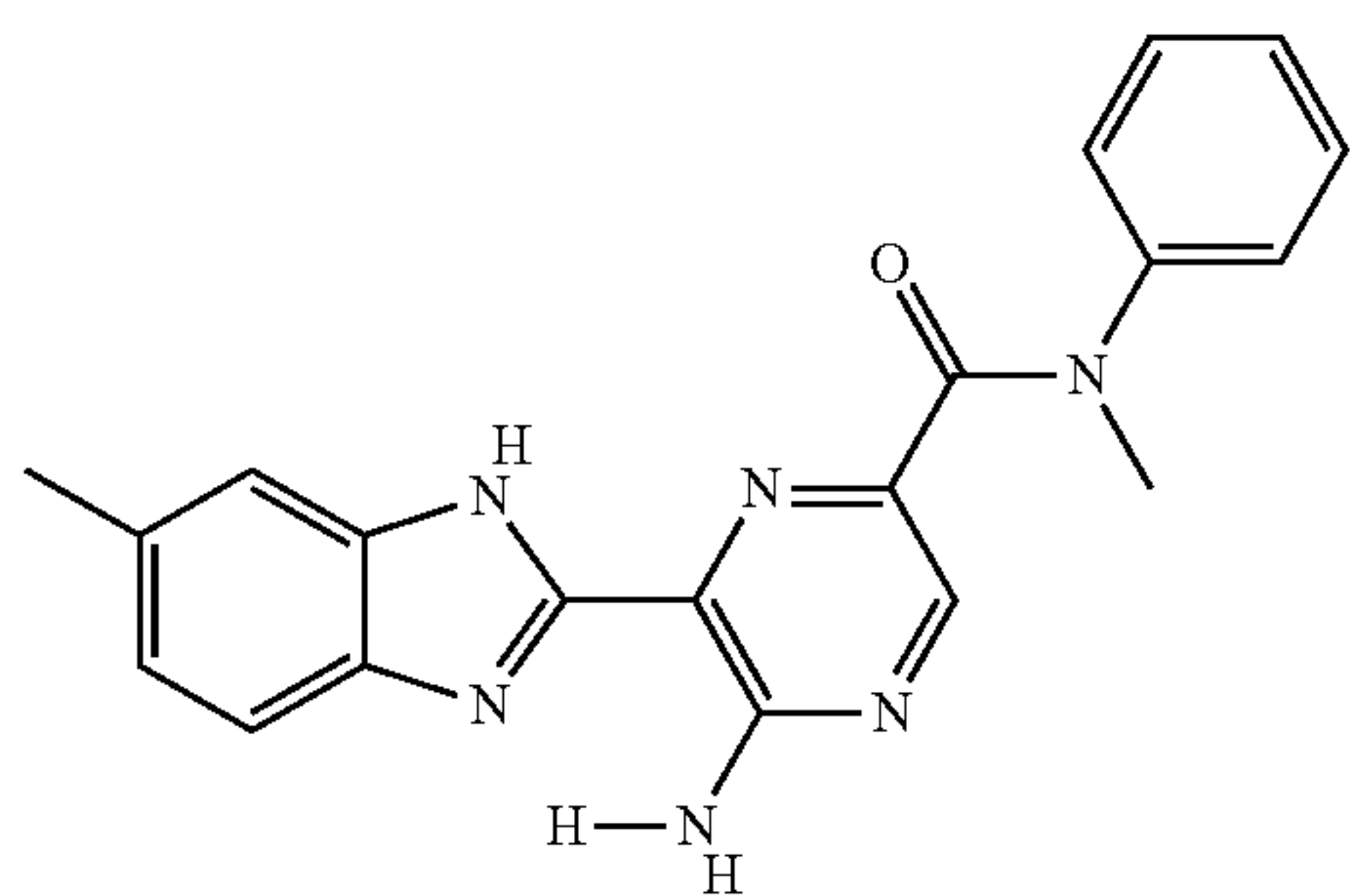
II-44
