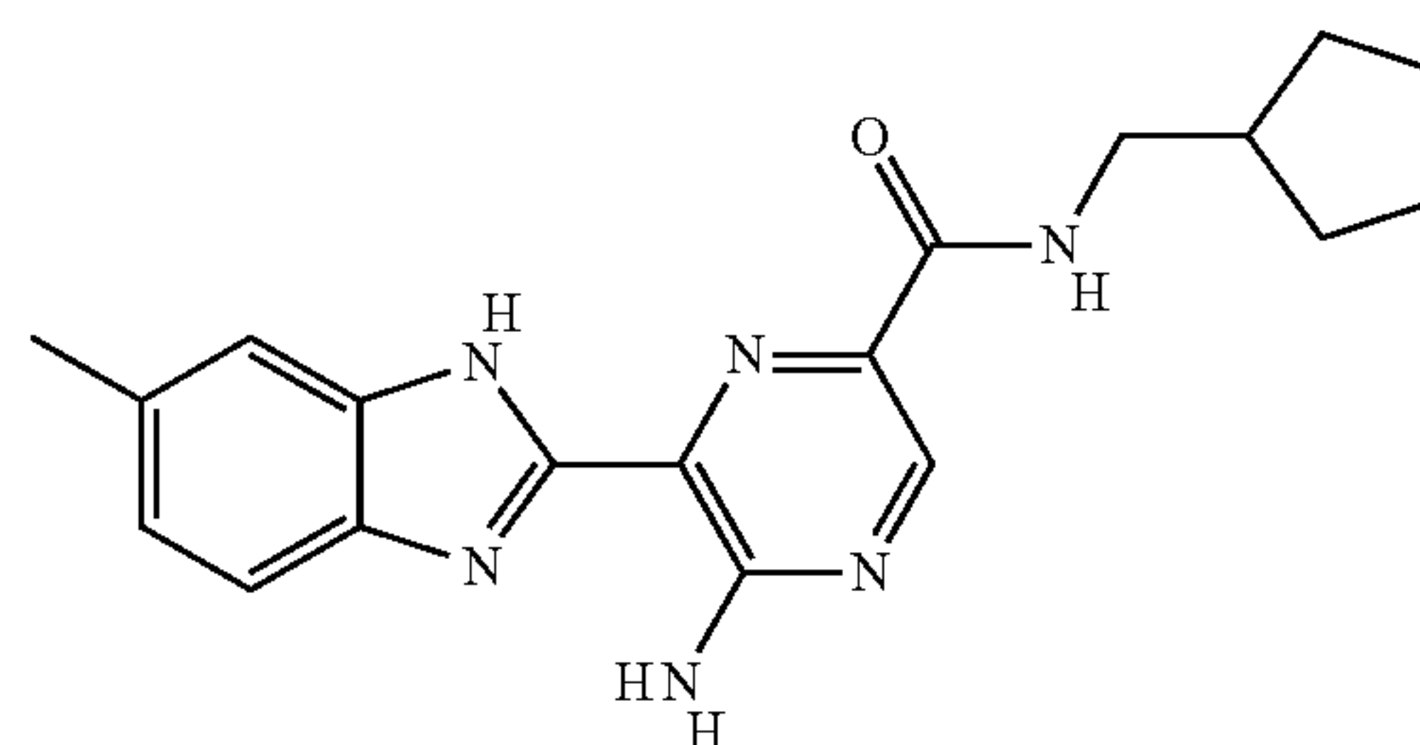
II-49
