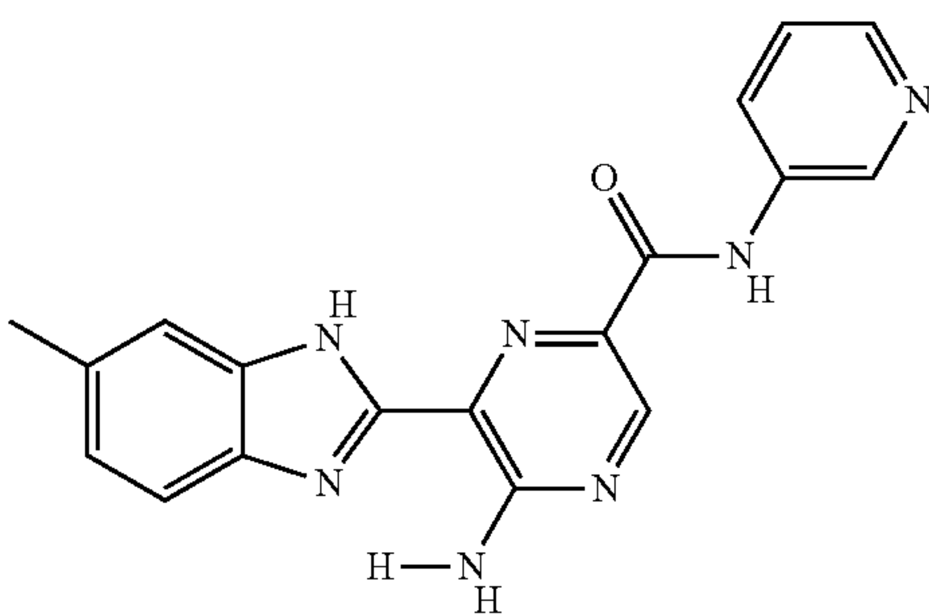
II-42
