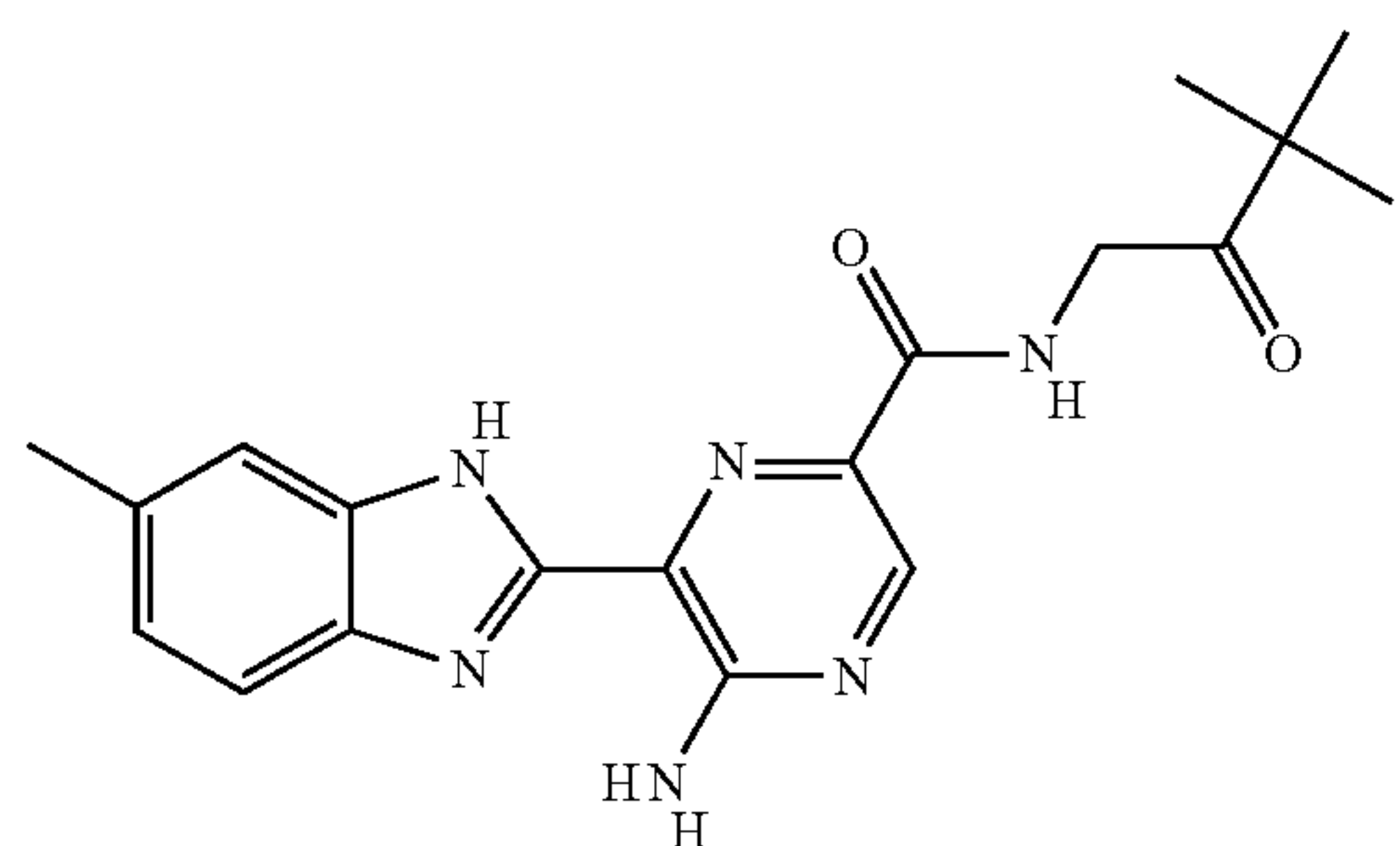
II-62
