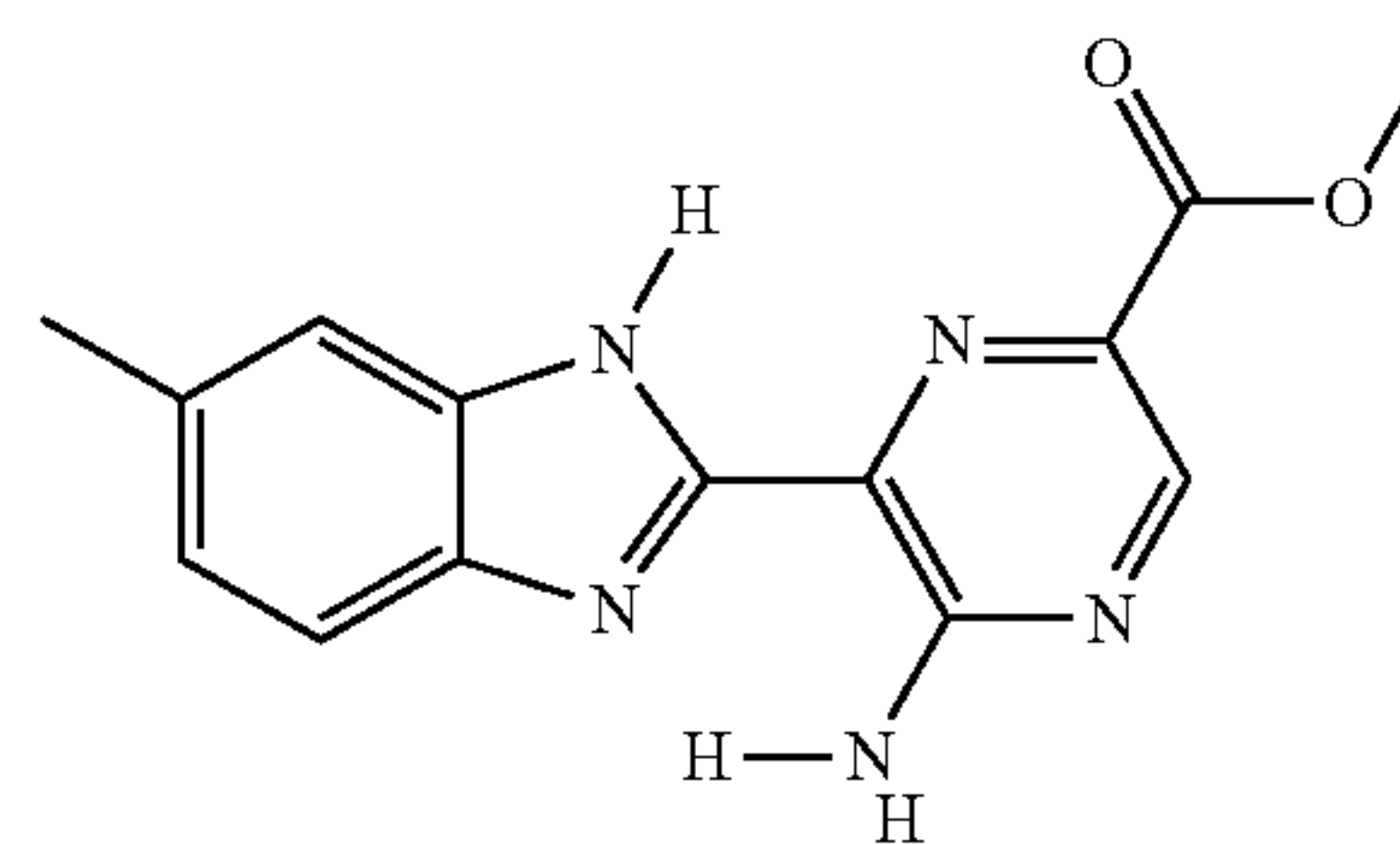
II-47
