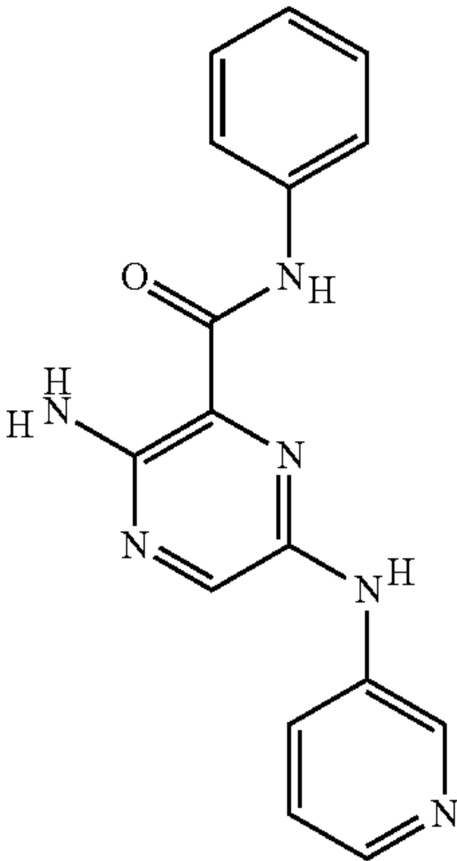
II-4
