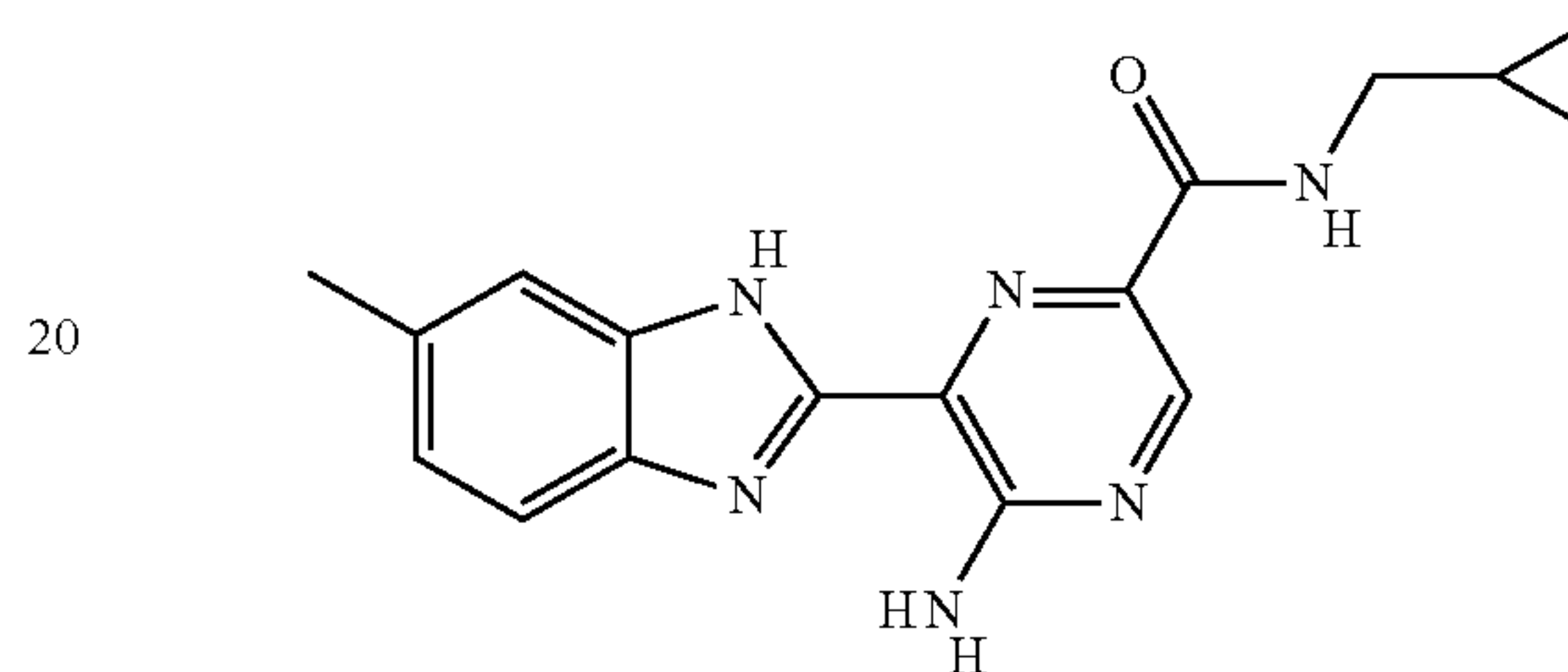
II-56
