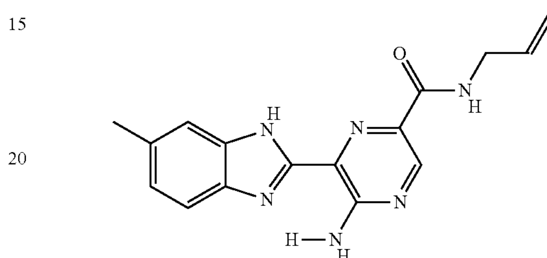
II-66
