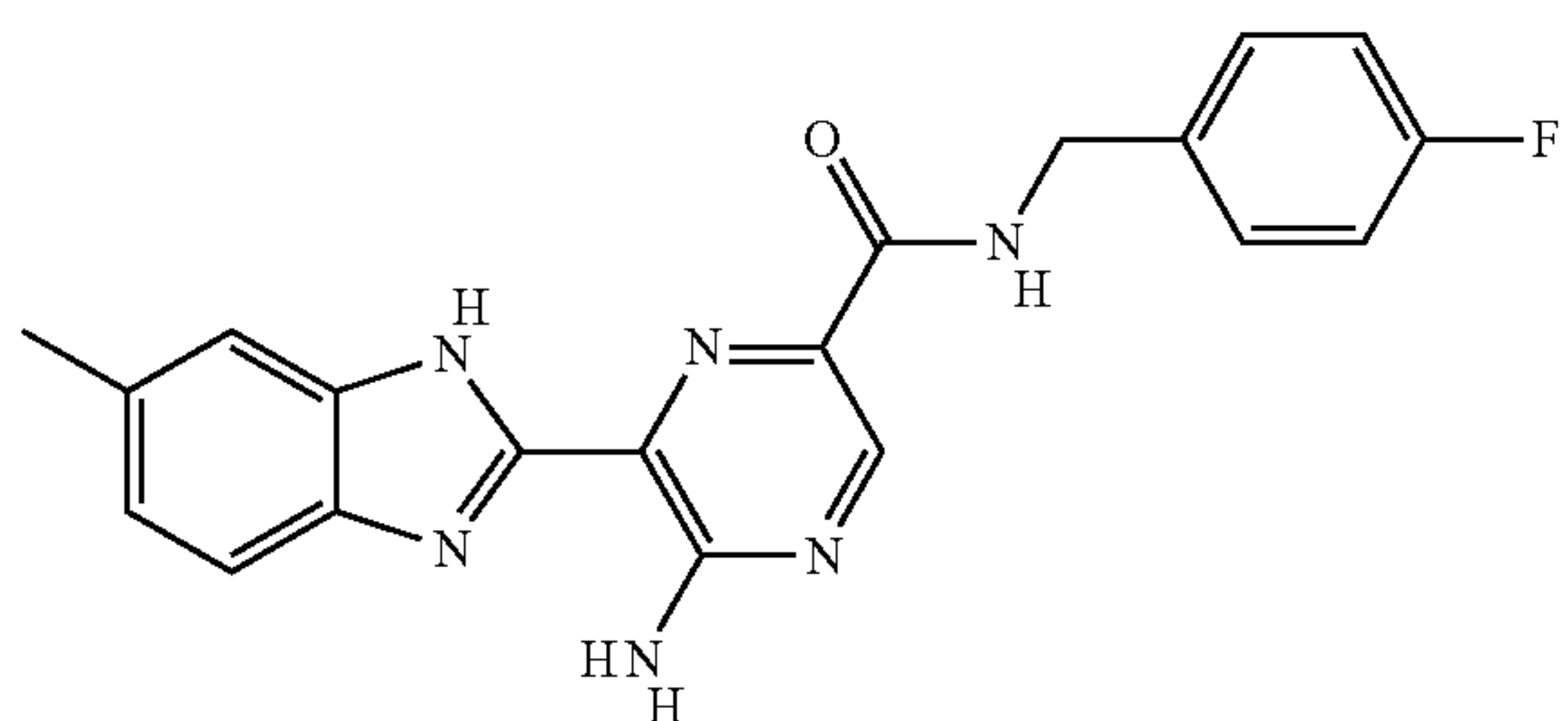
II-64
