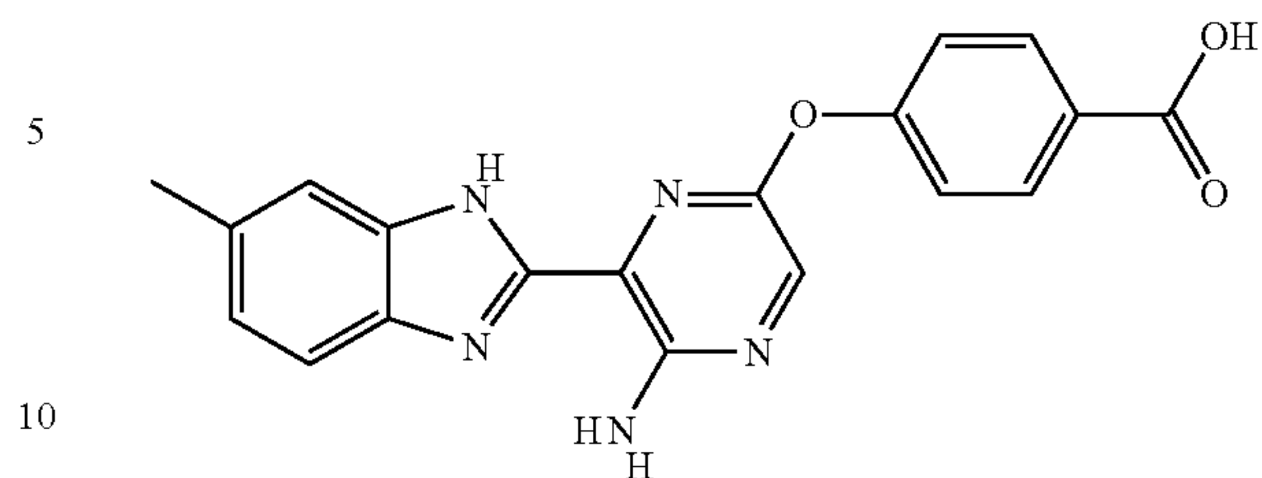
II-26
