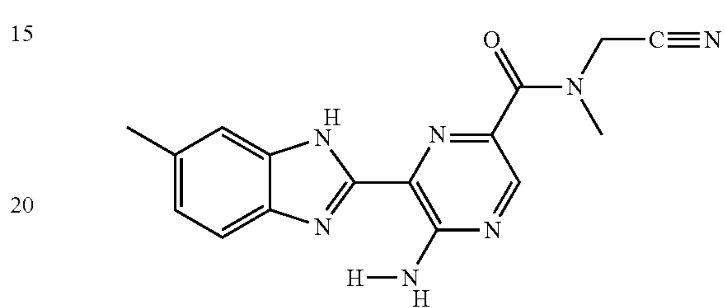
II-76
