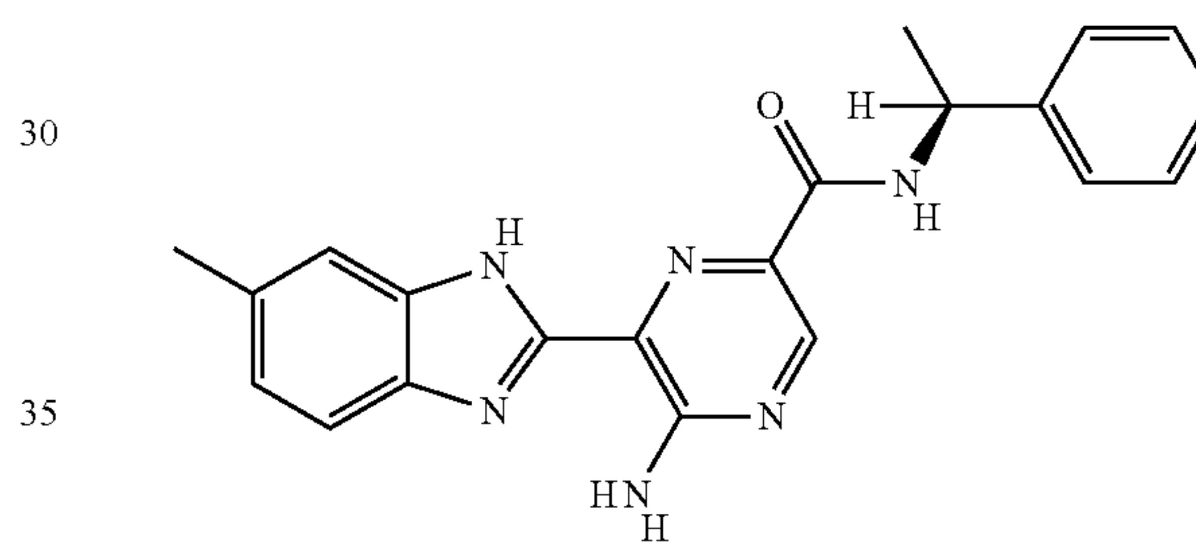
II-57
