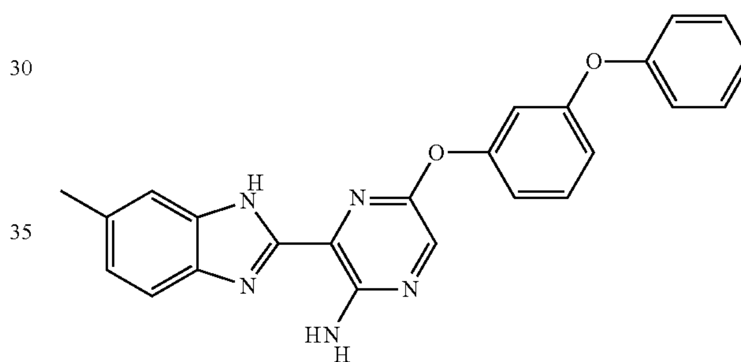
II-28
