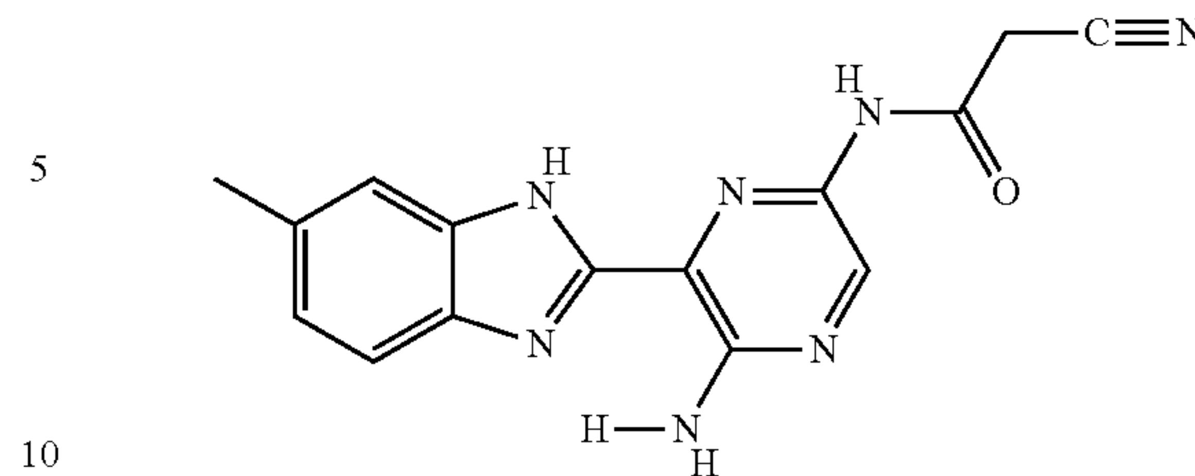
II-92
