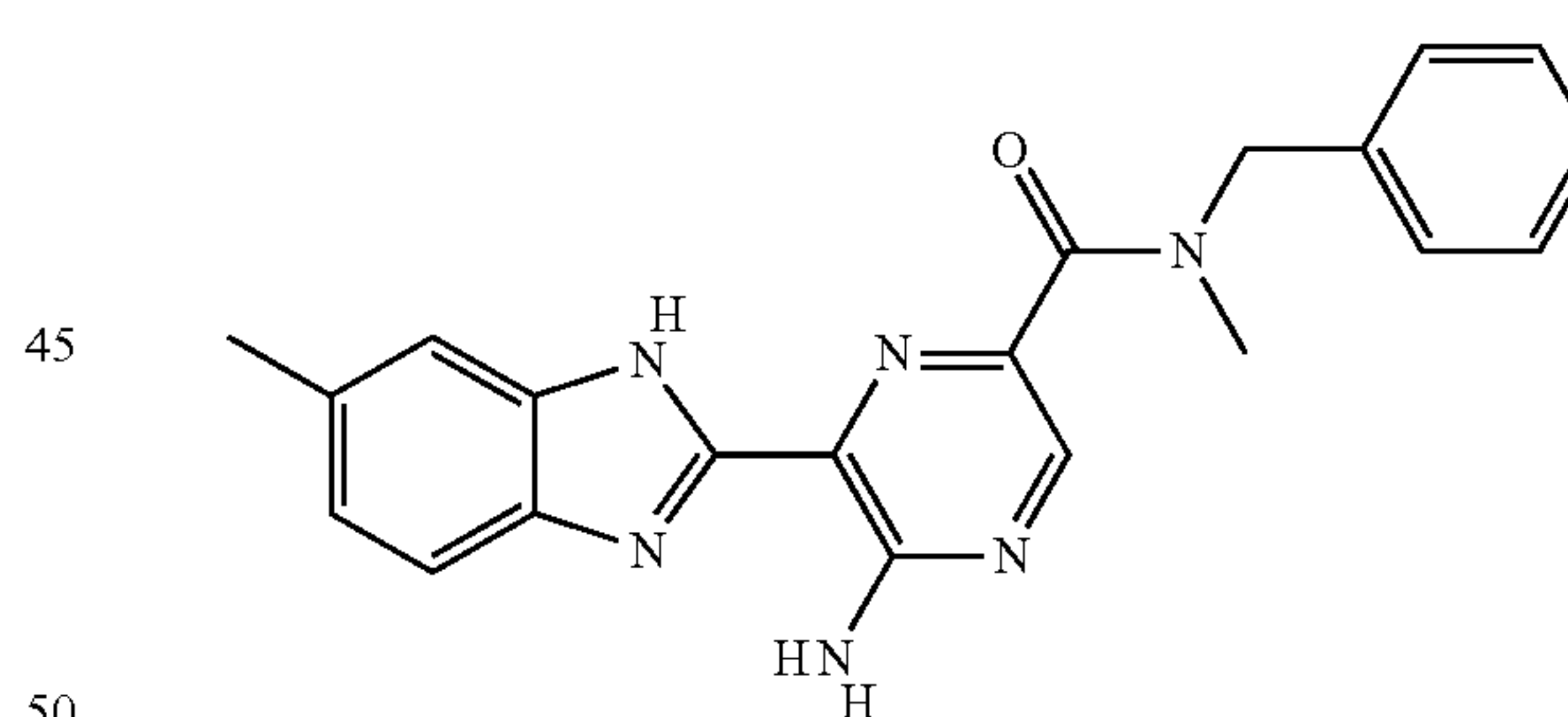
II-58
