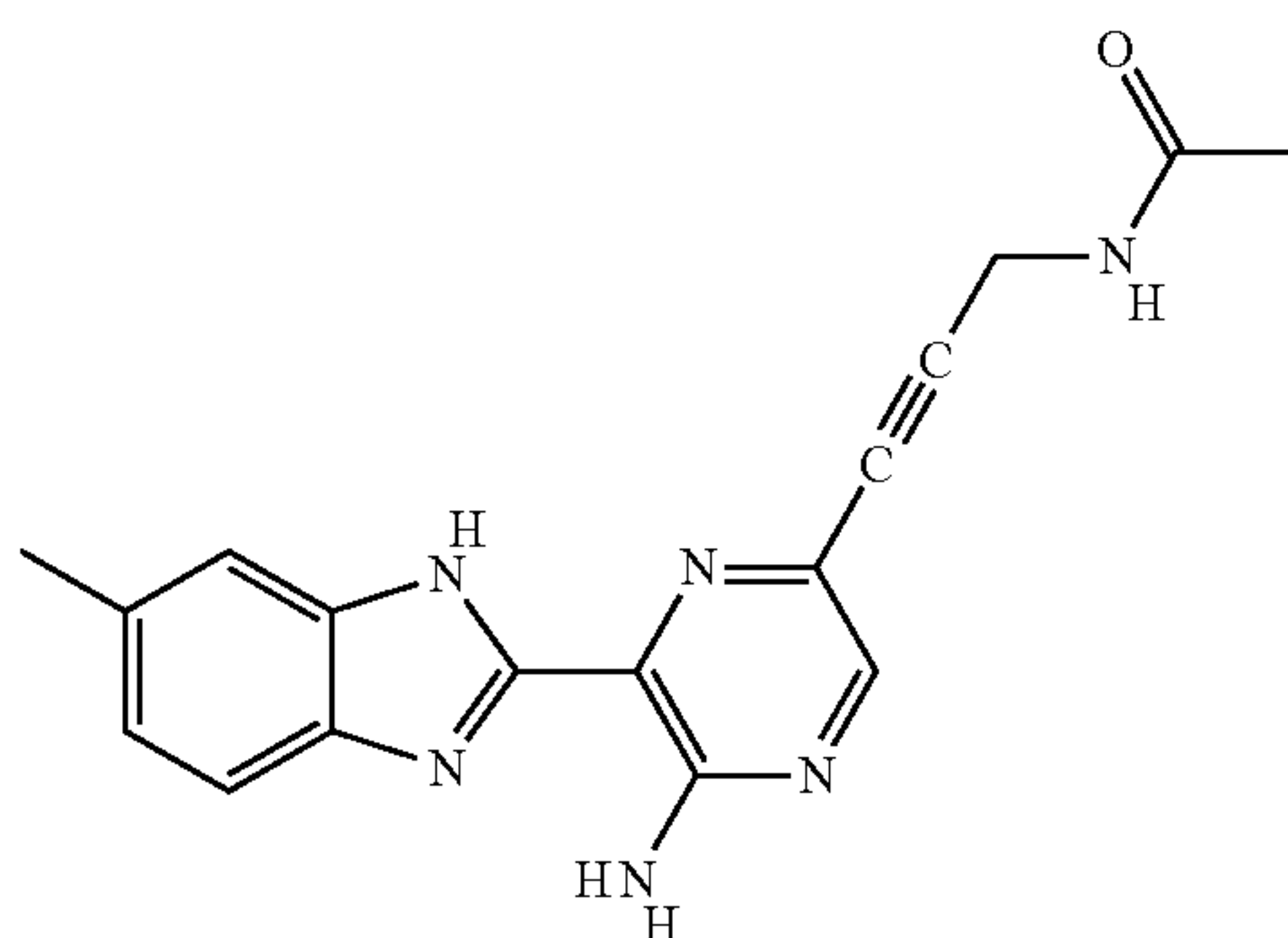
II-88
