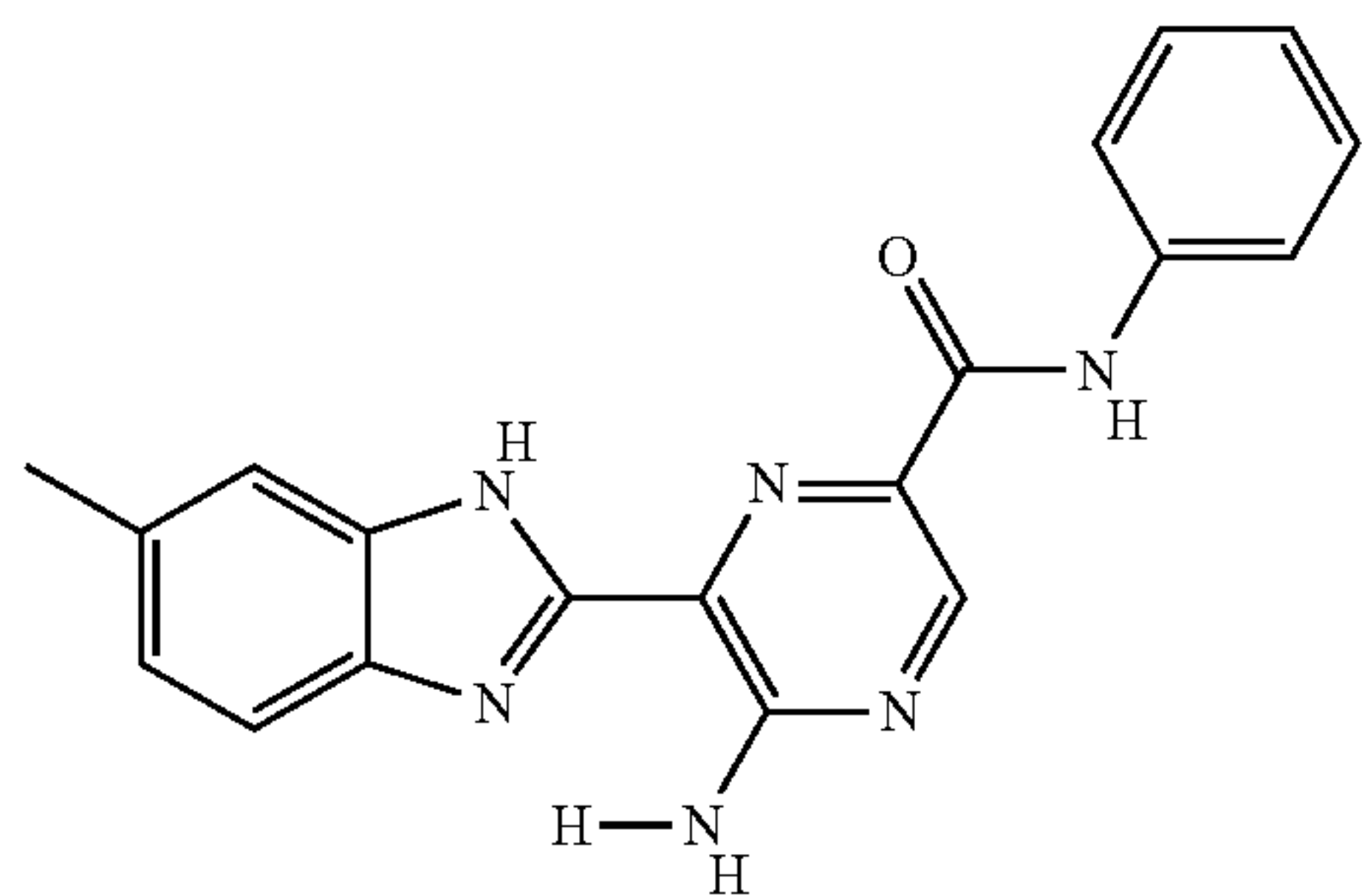
II-41
