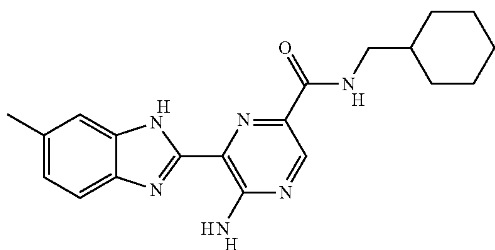
II-63
