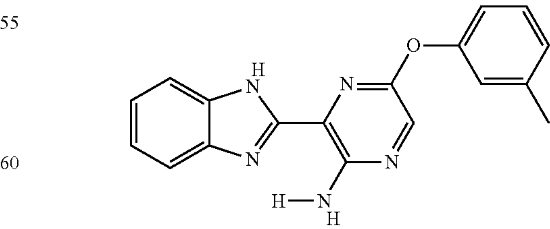
II-10
