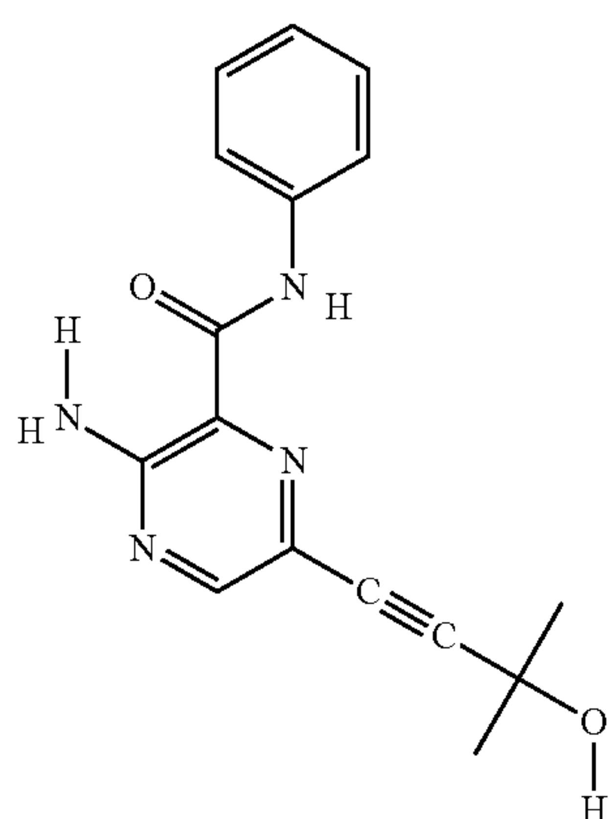
II-81
