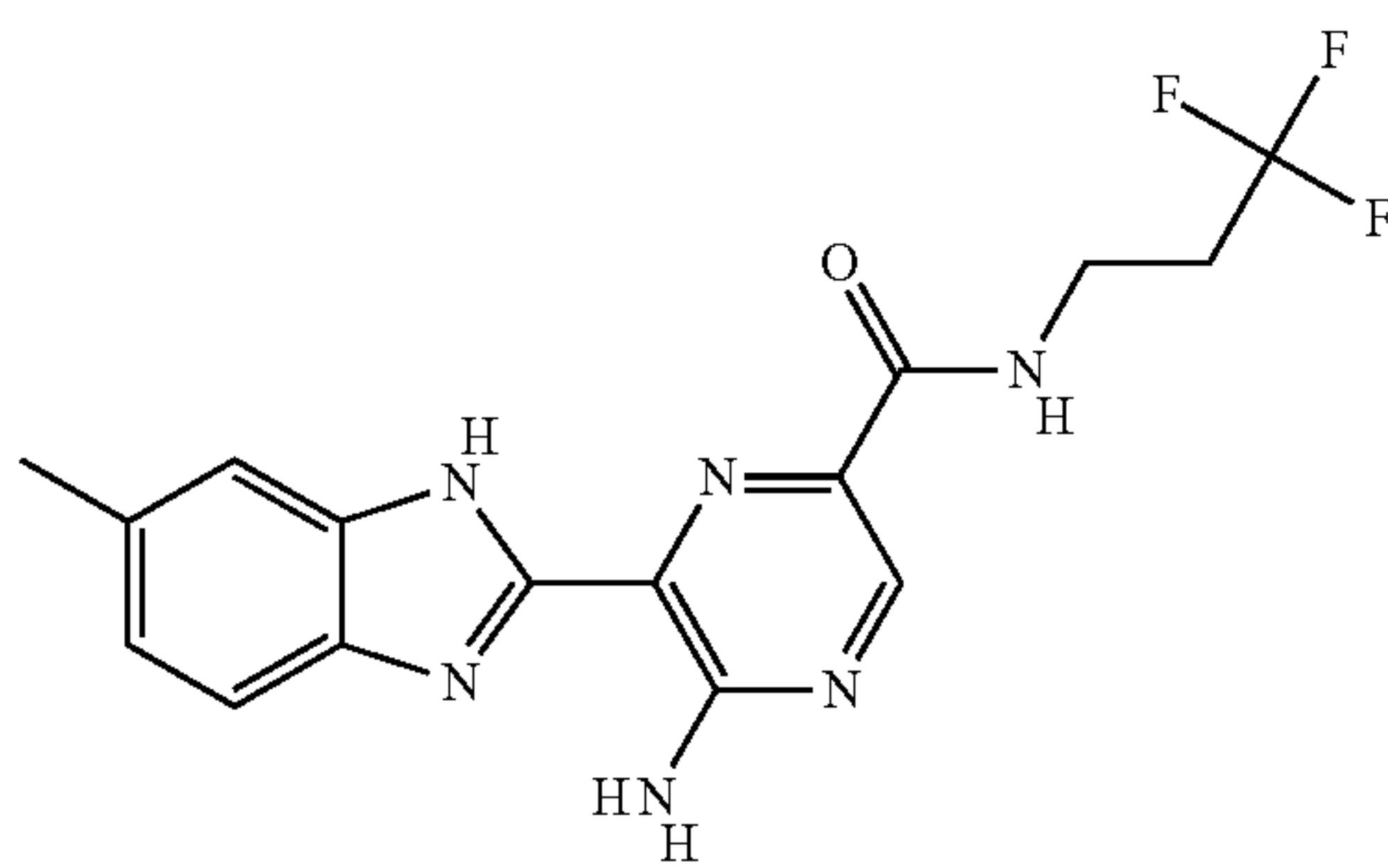
II-73
