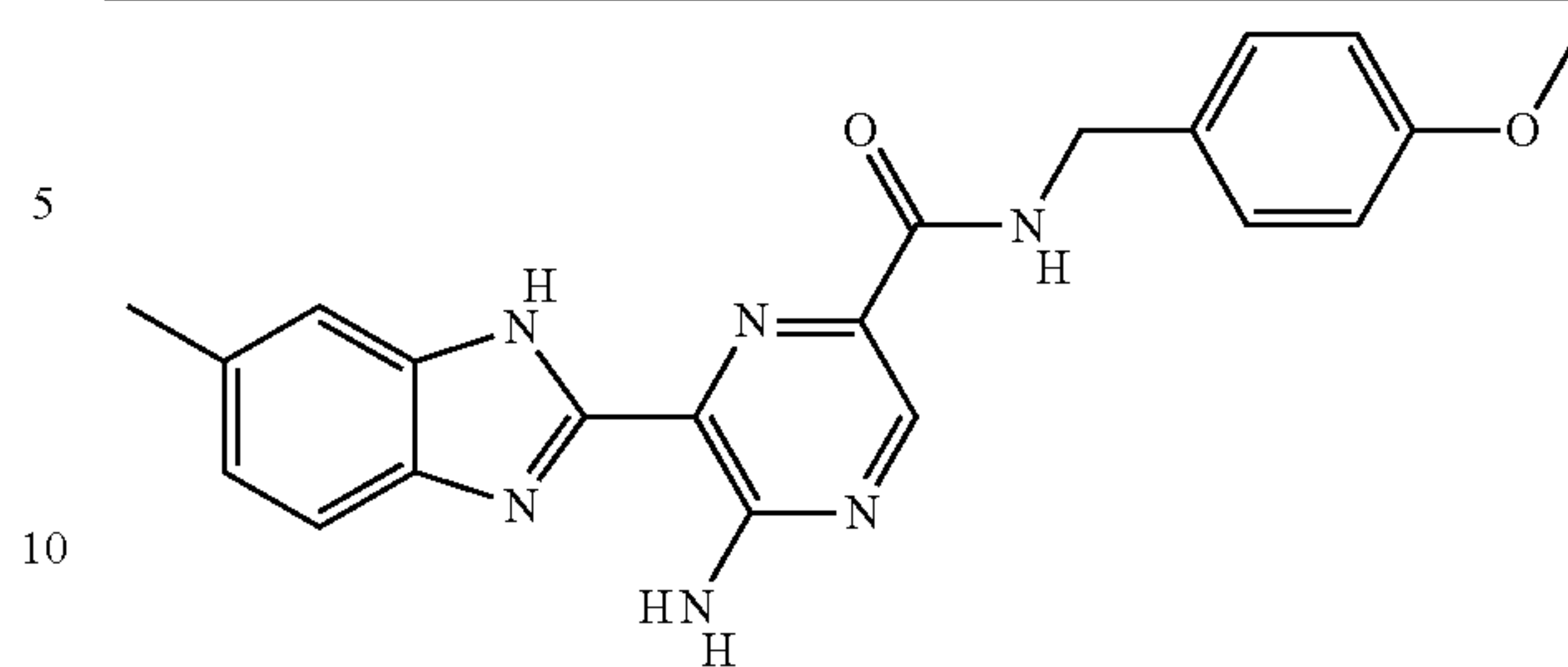
II-65
