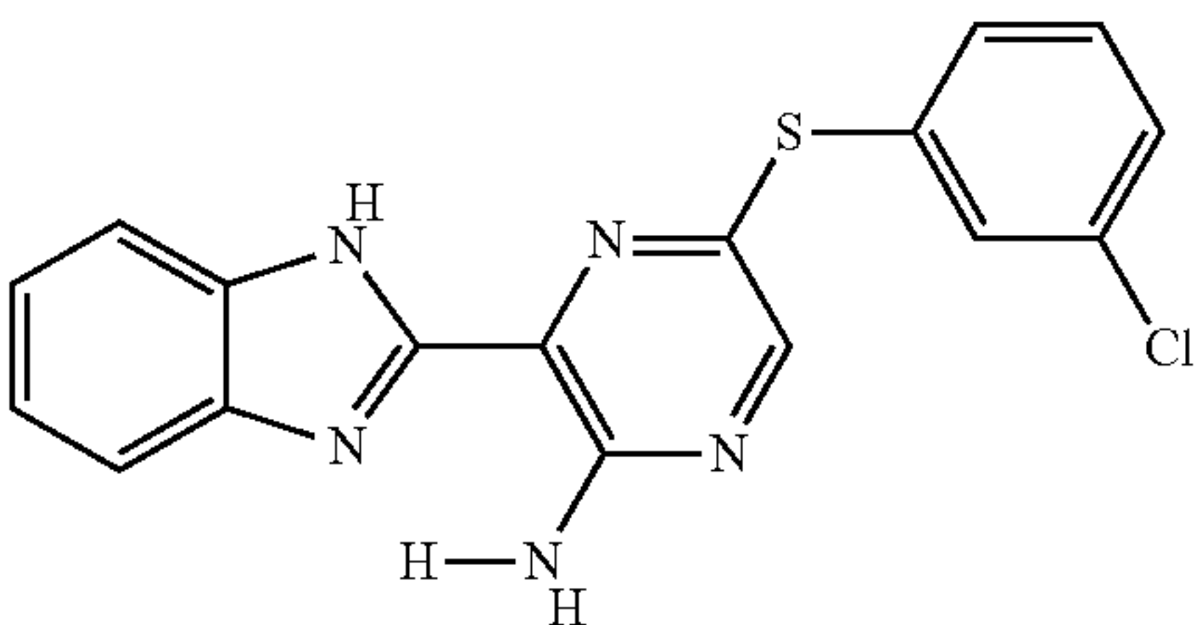
II-39
