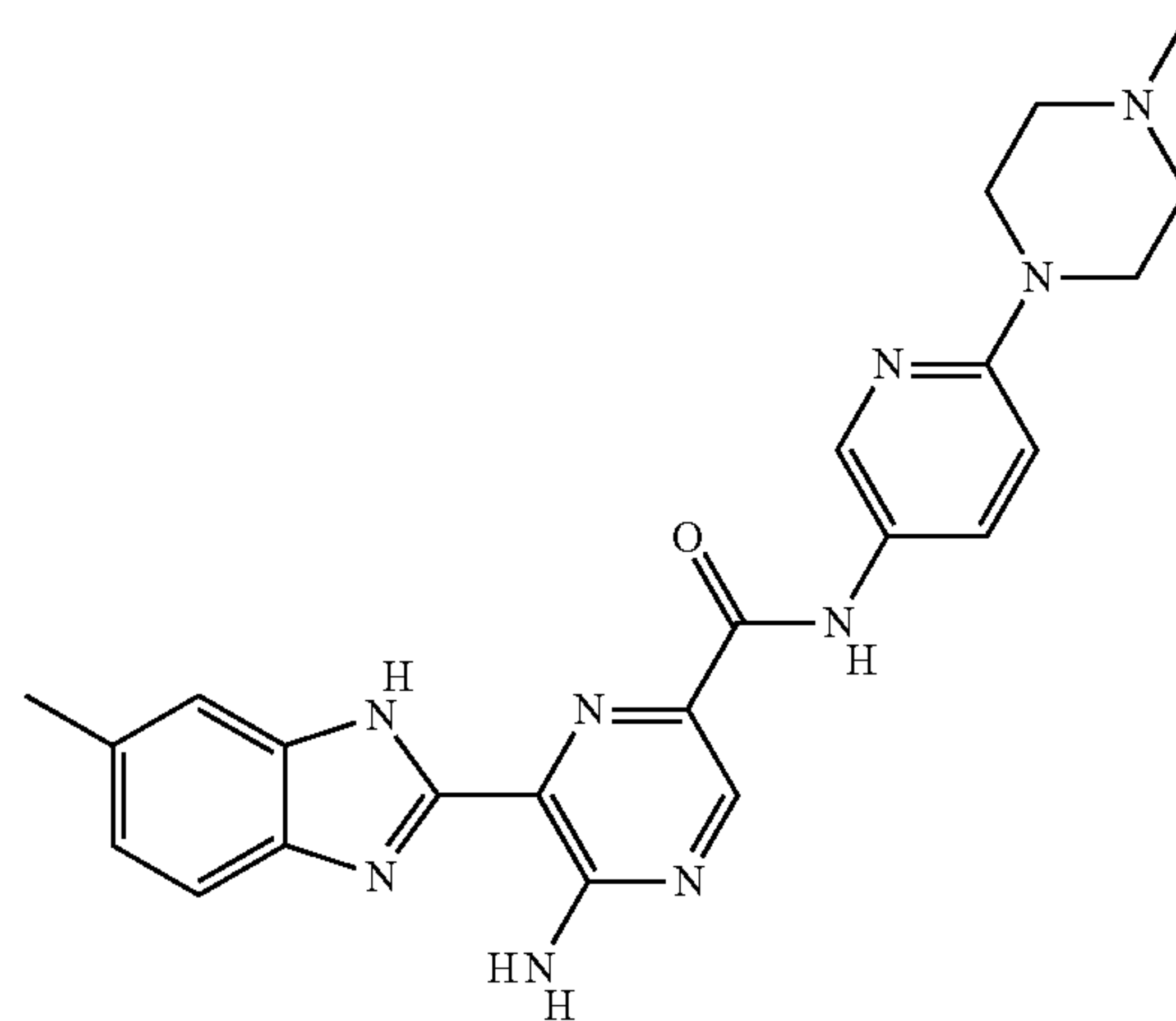
II-45
