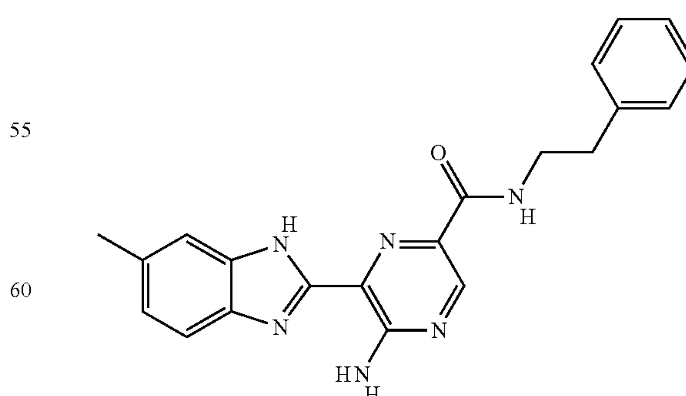
II-69
