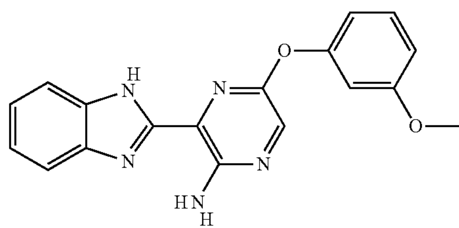
II-15
