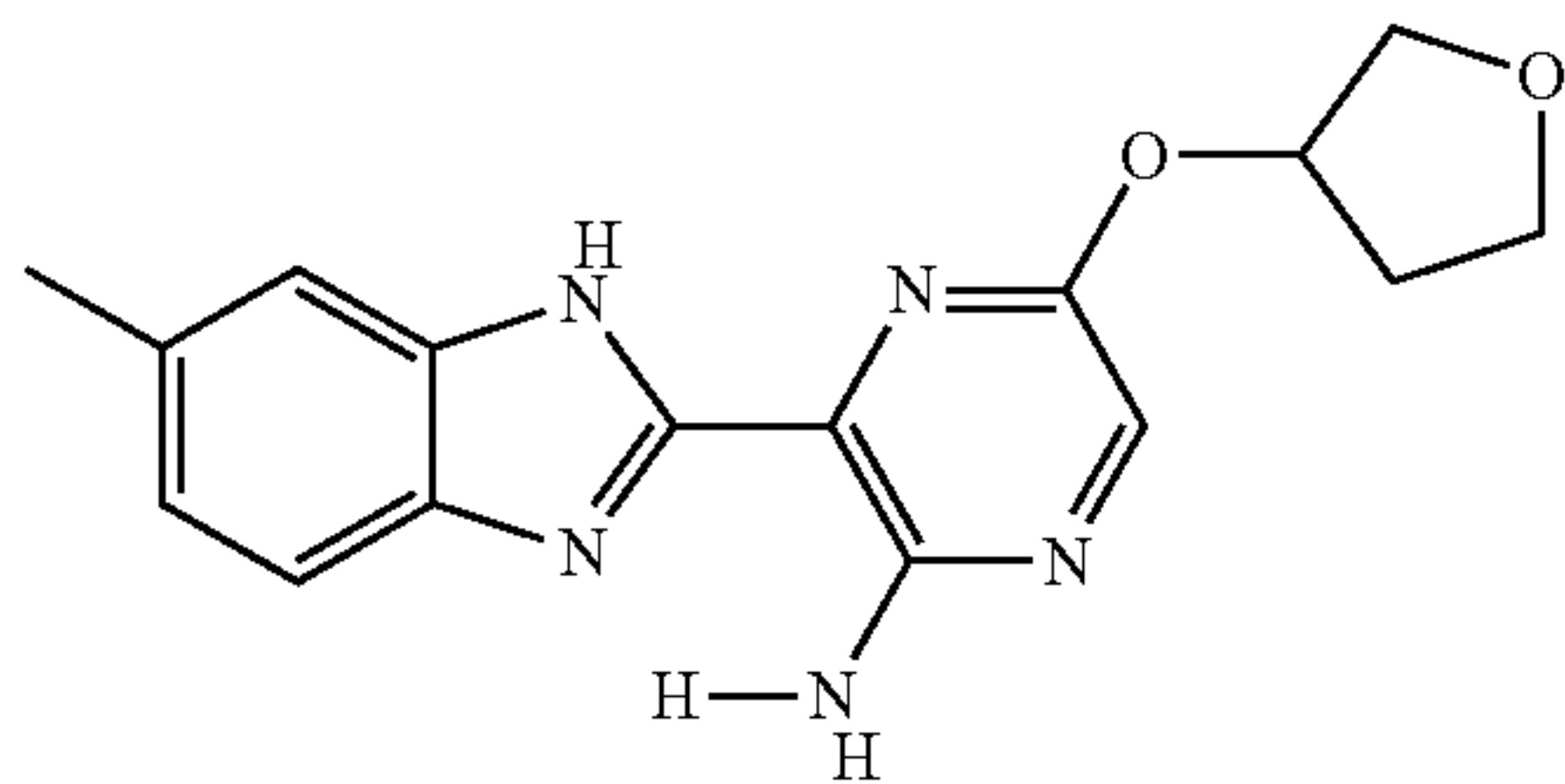
II-32
