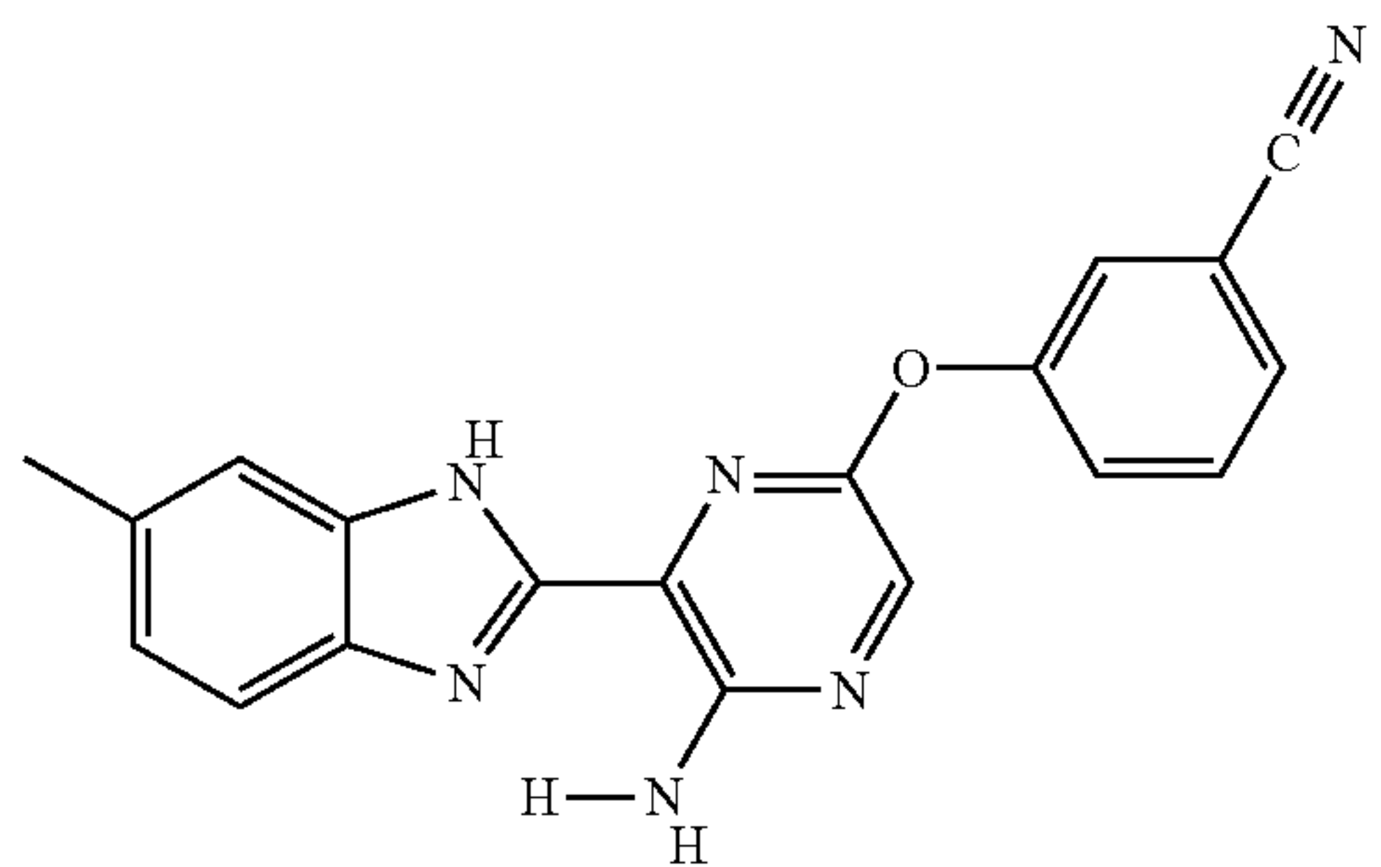
II-31
