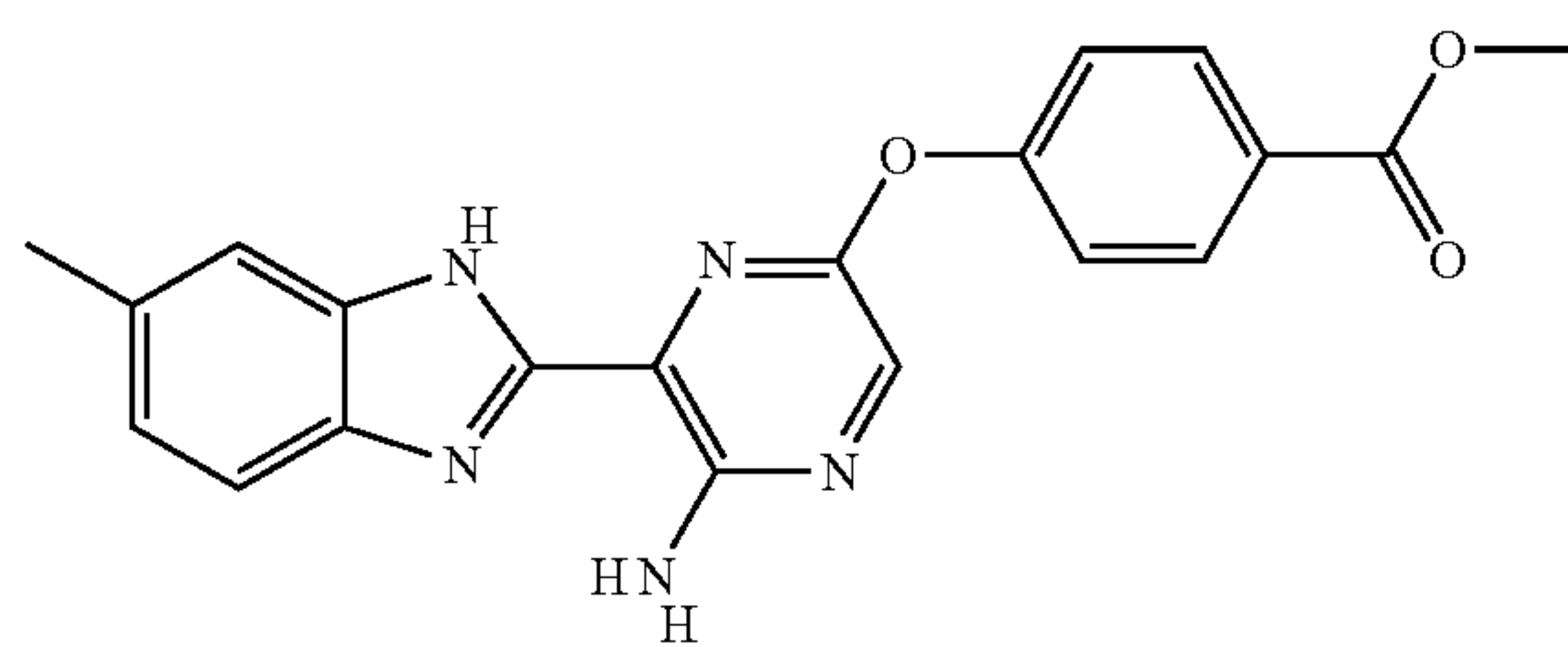
II-25
