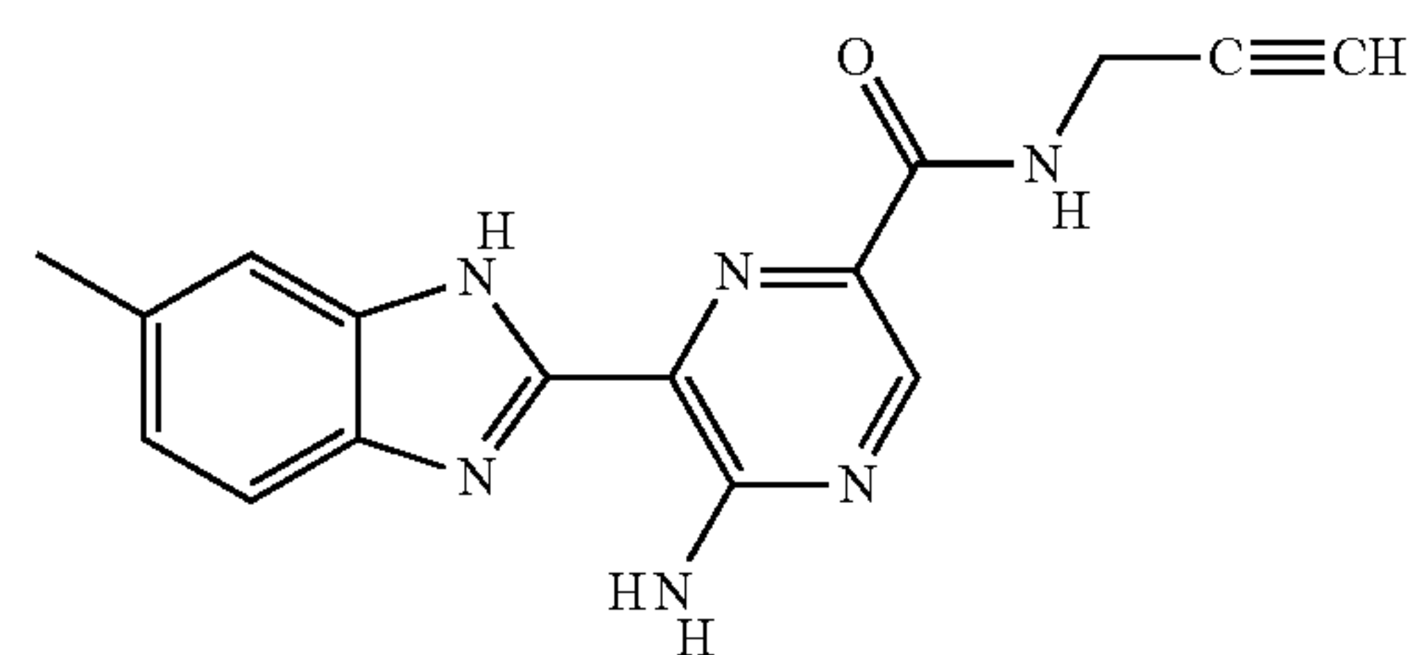
II-54
