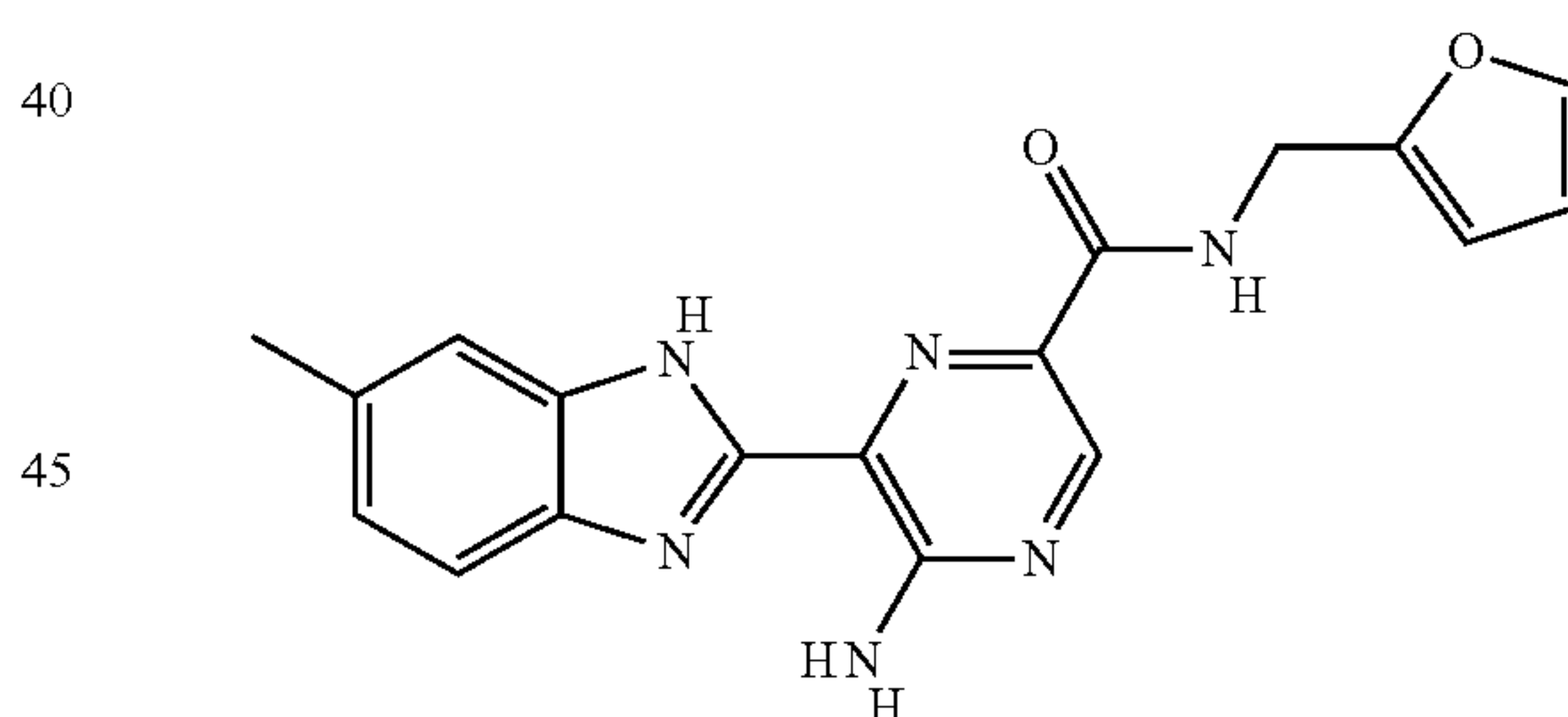
II-68
