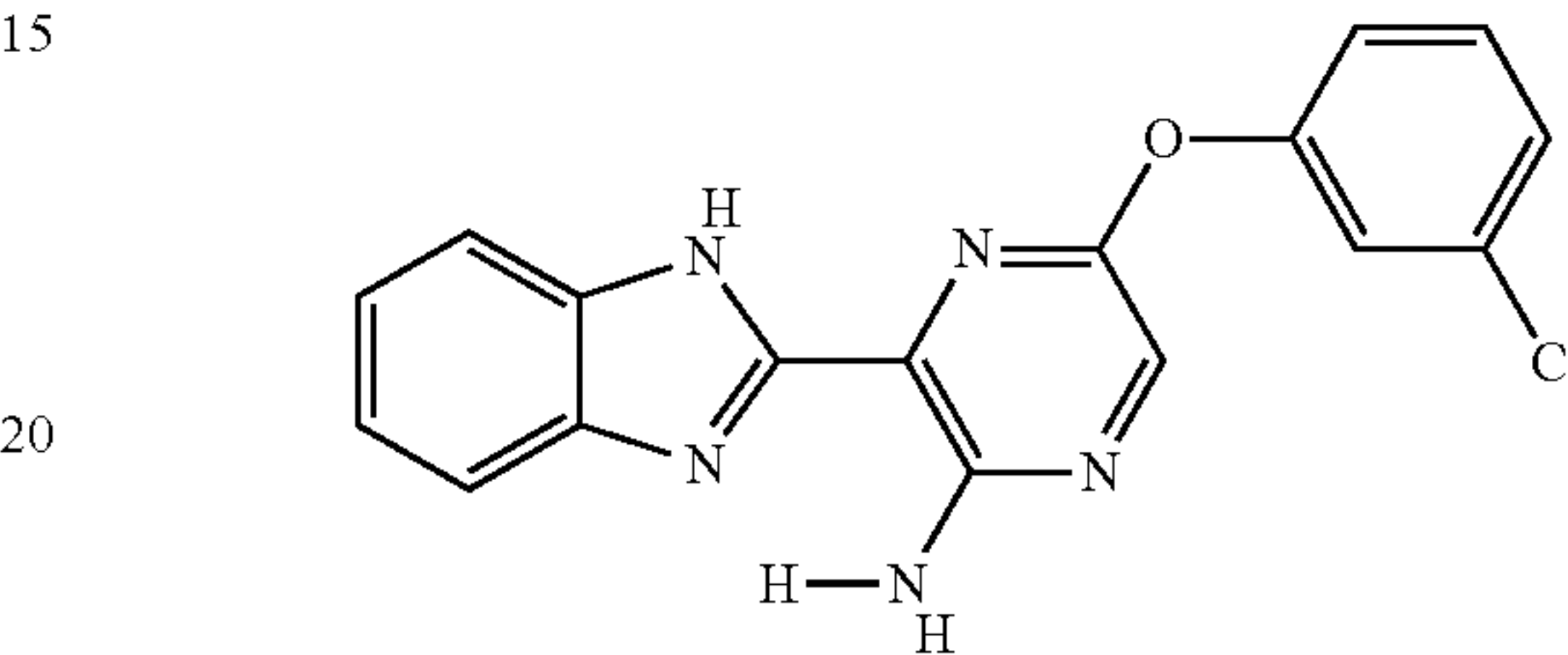
II-7
