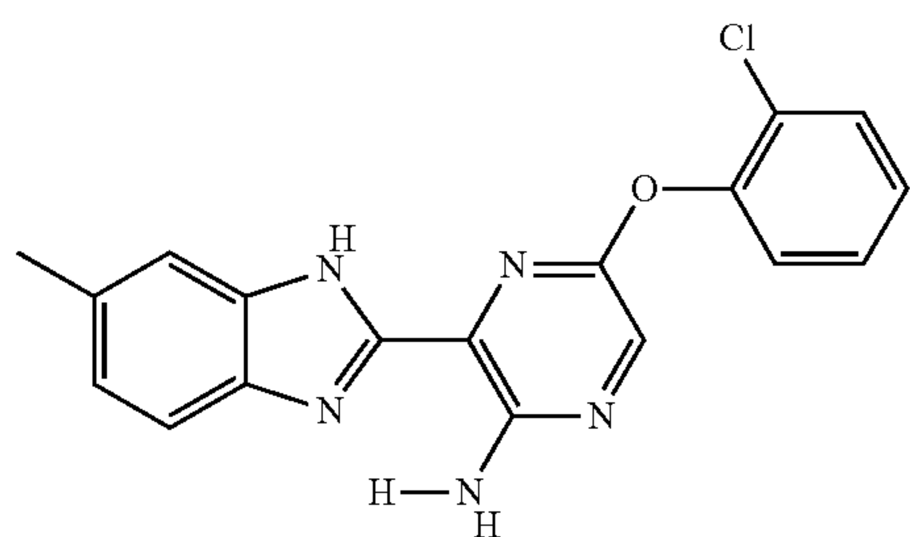
II-21
