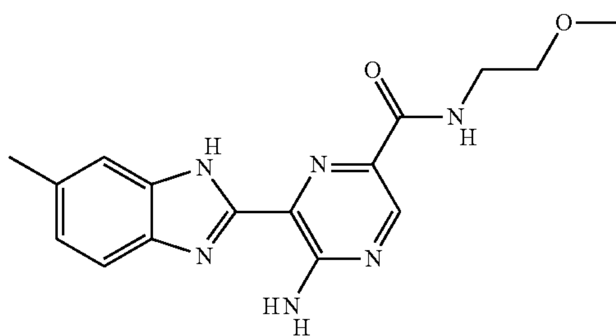
II-71
