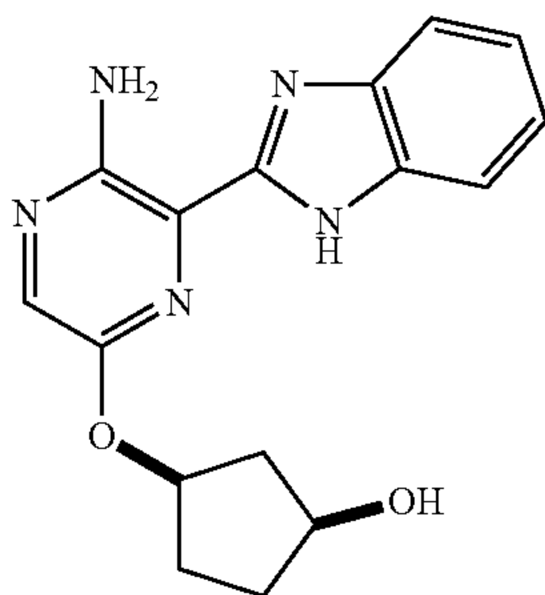
II-35
