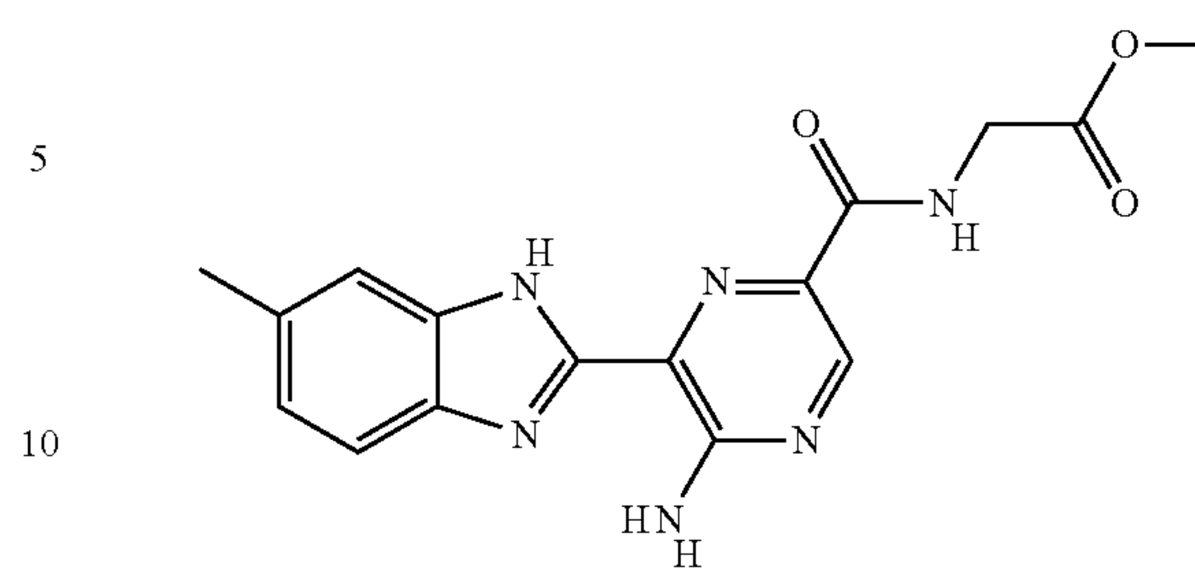
II-55
