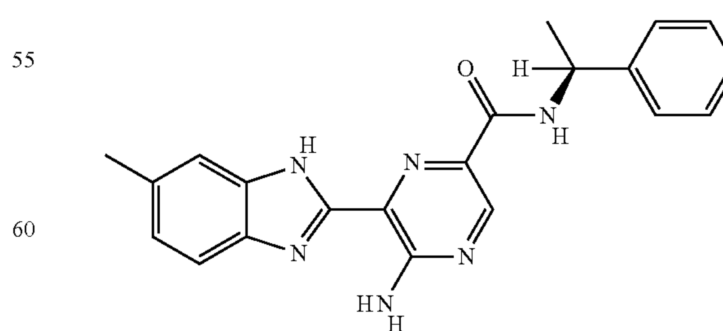
II-59
