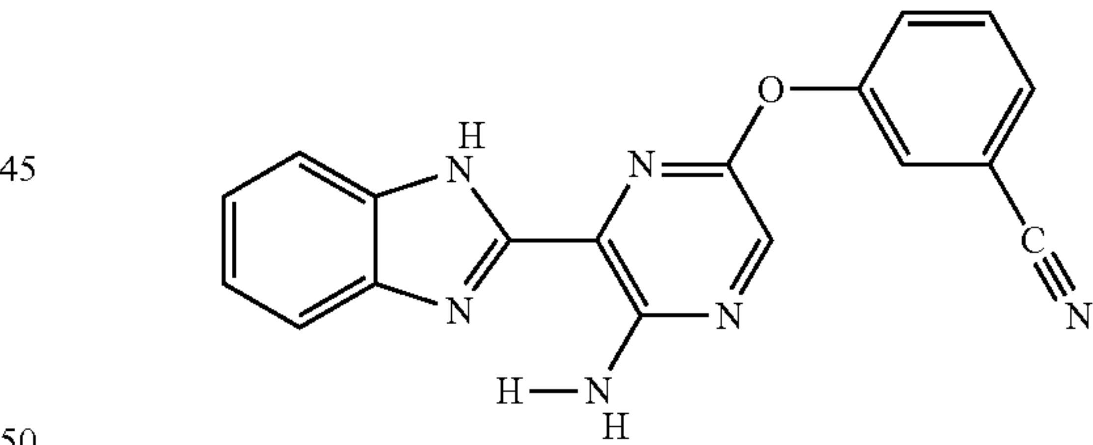
II-9
