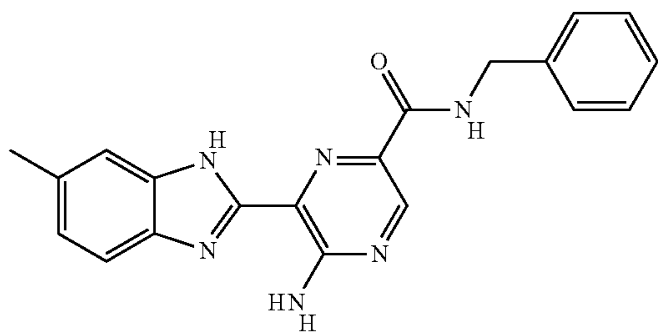
II-43
