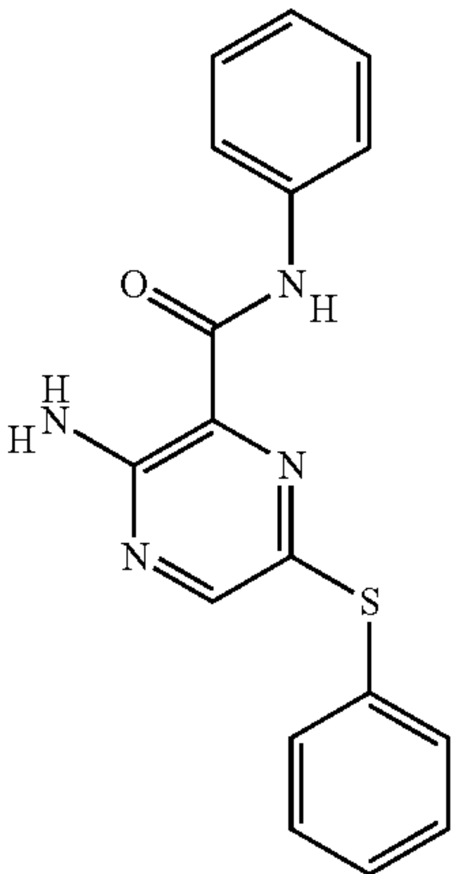
II-37
