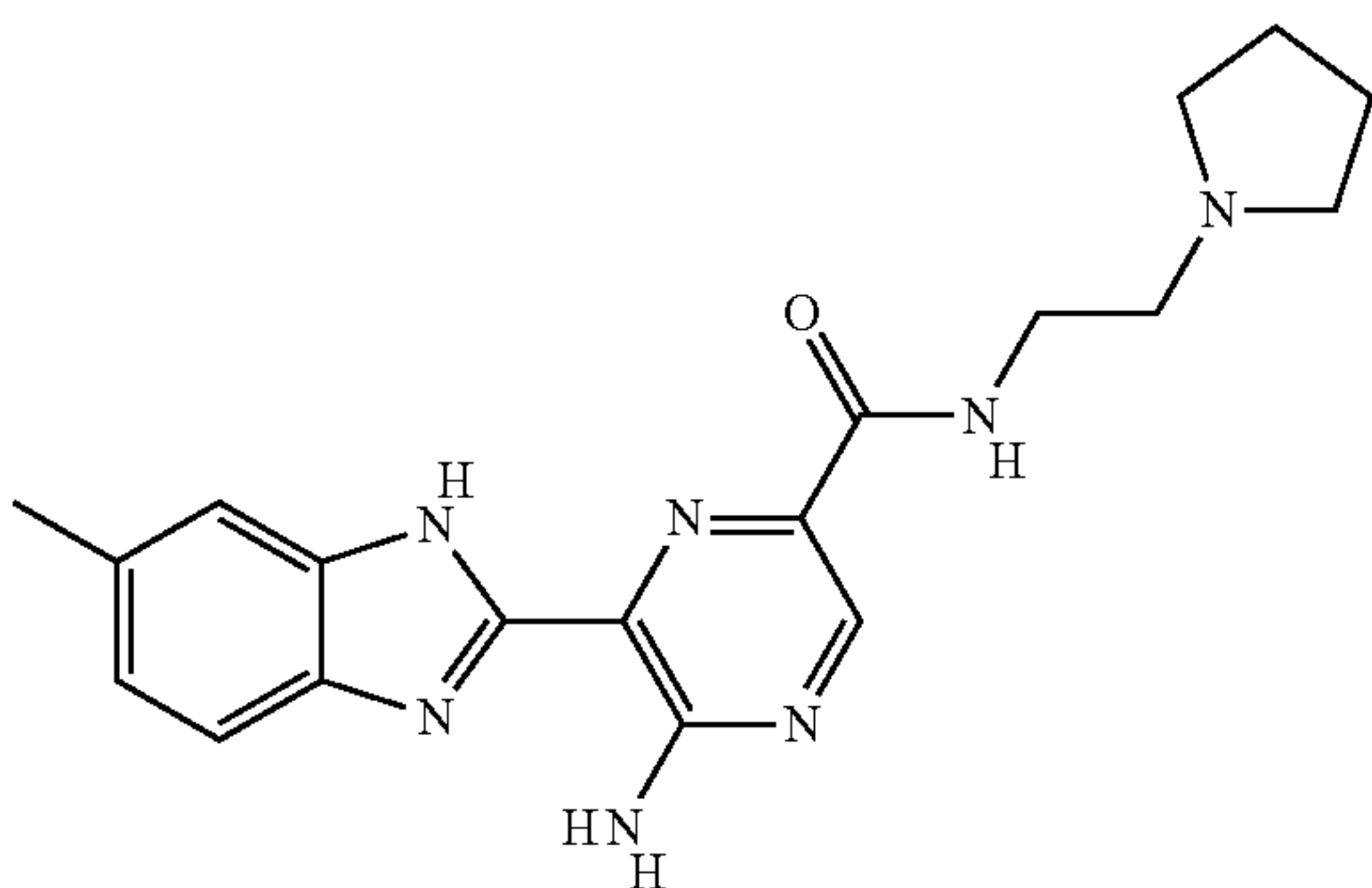
II-51
