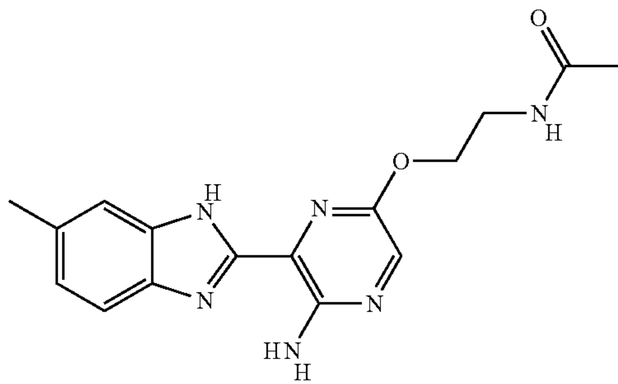
II-34
