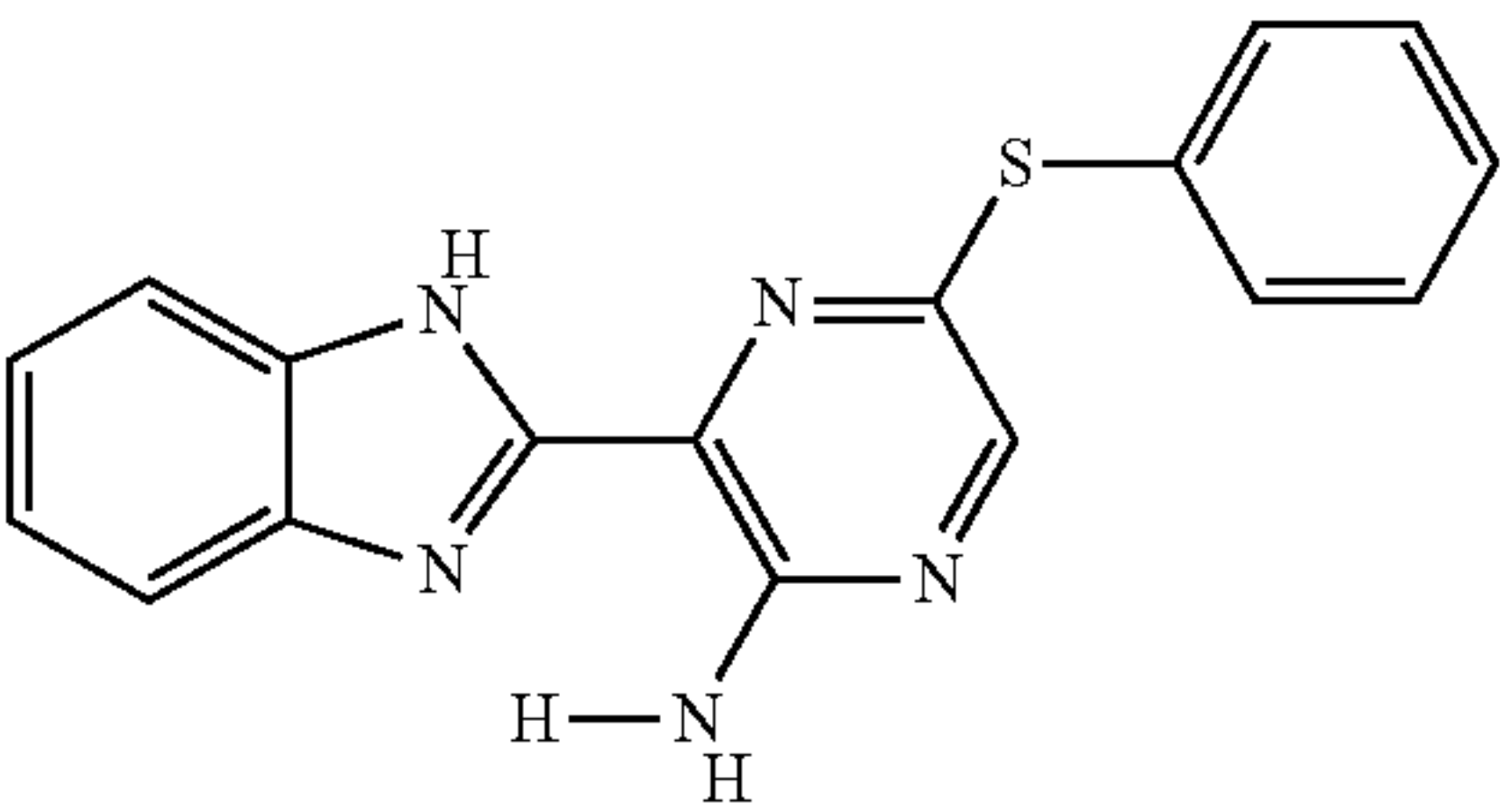
II-38
