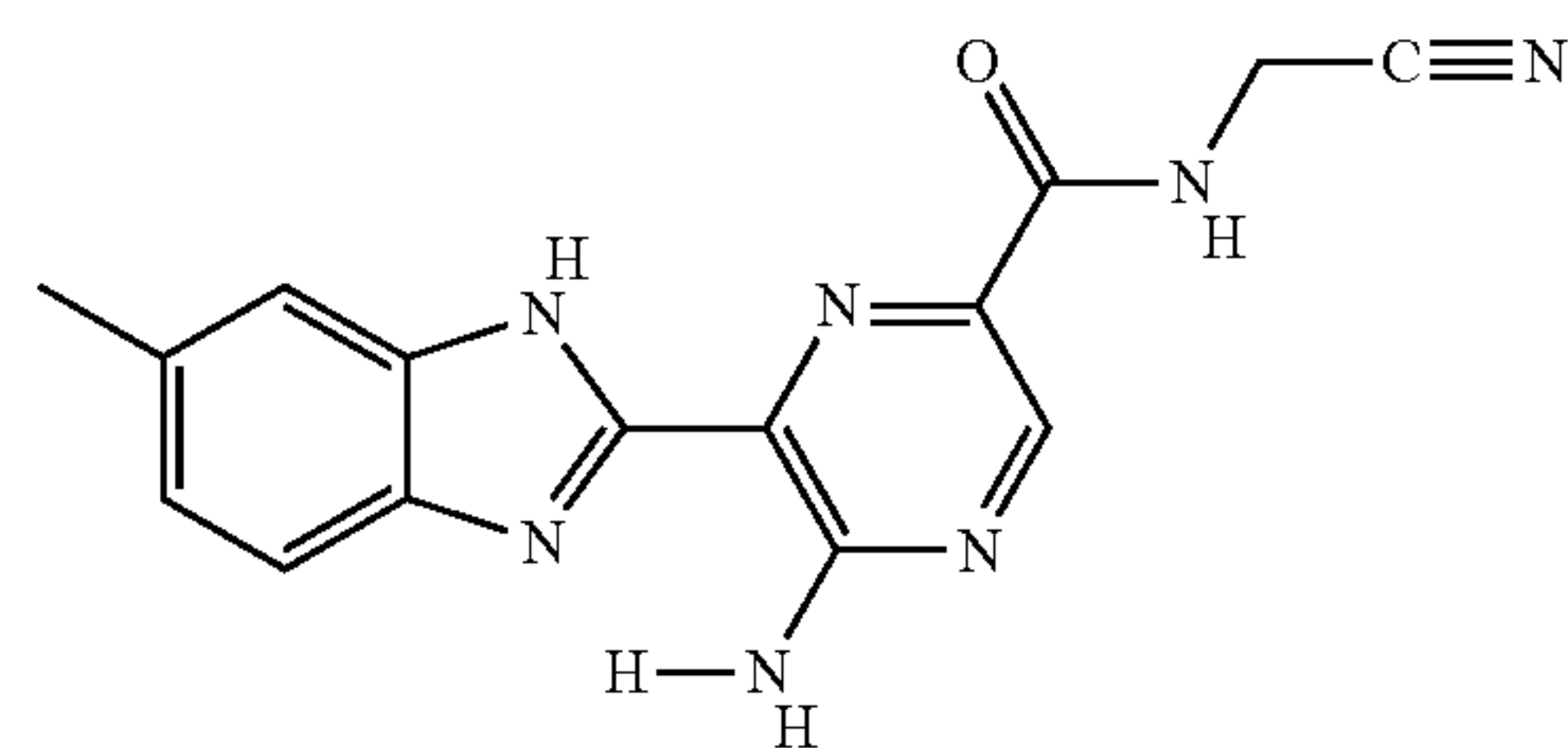
II-48
