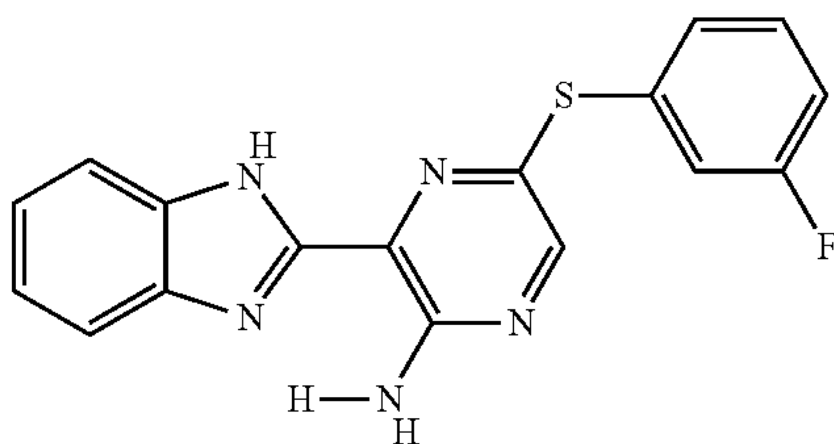
II-40
