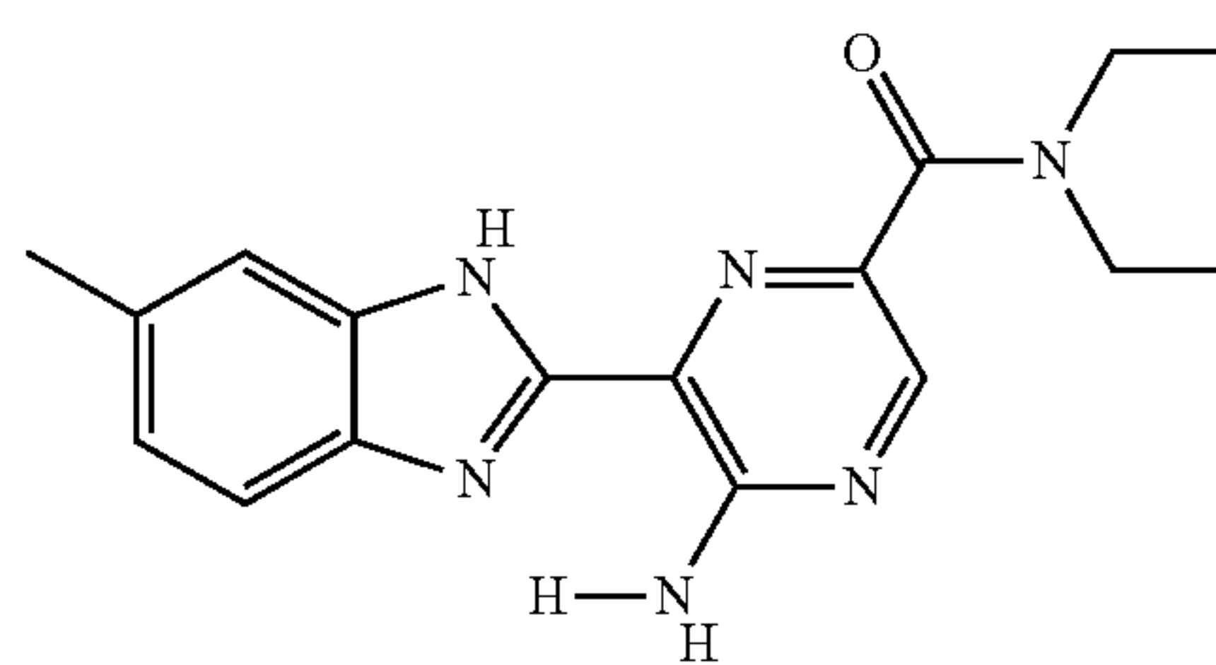
II-46
