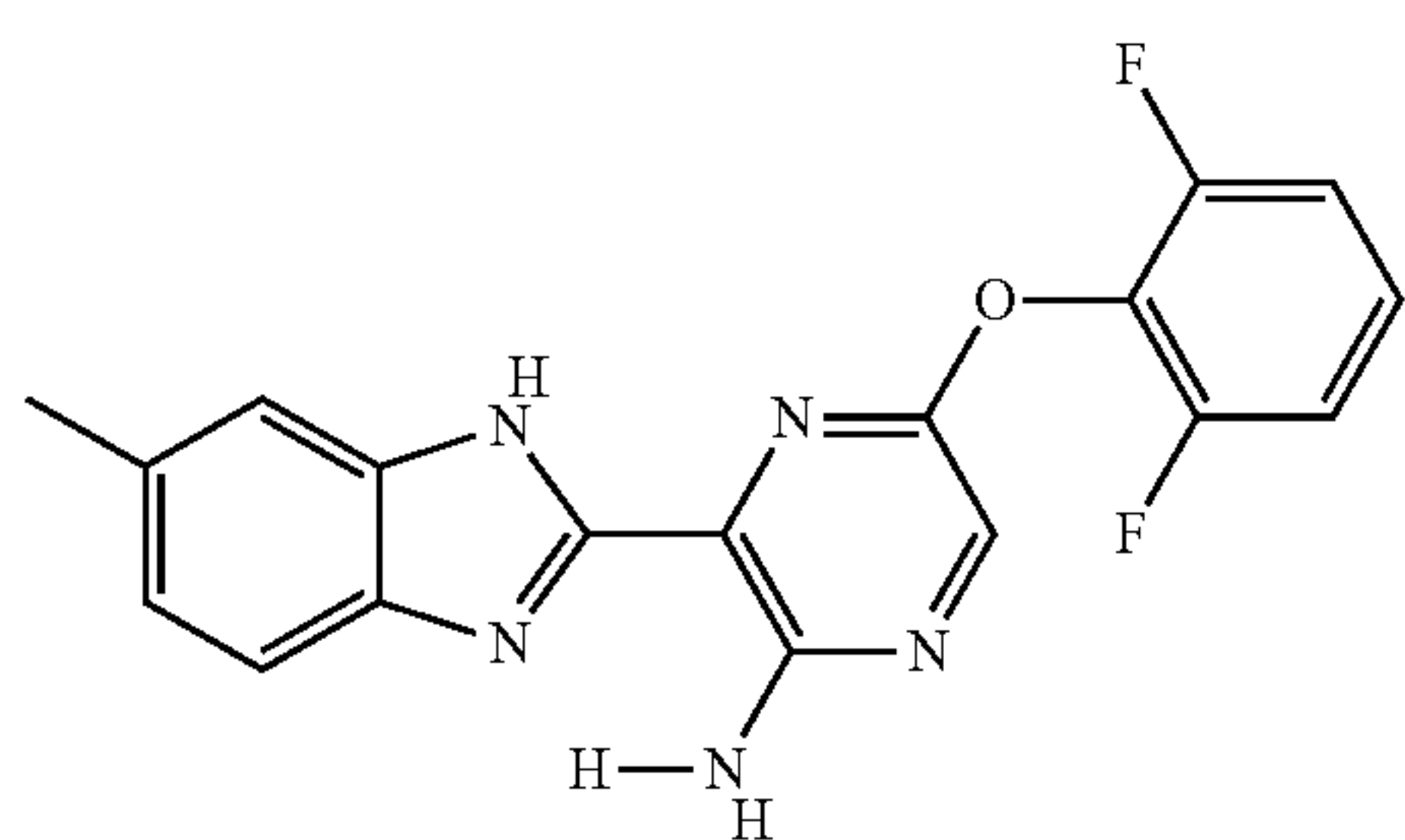
II-22
