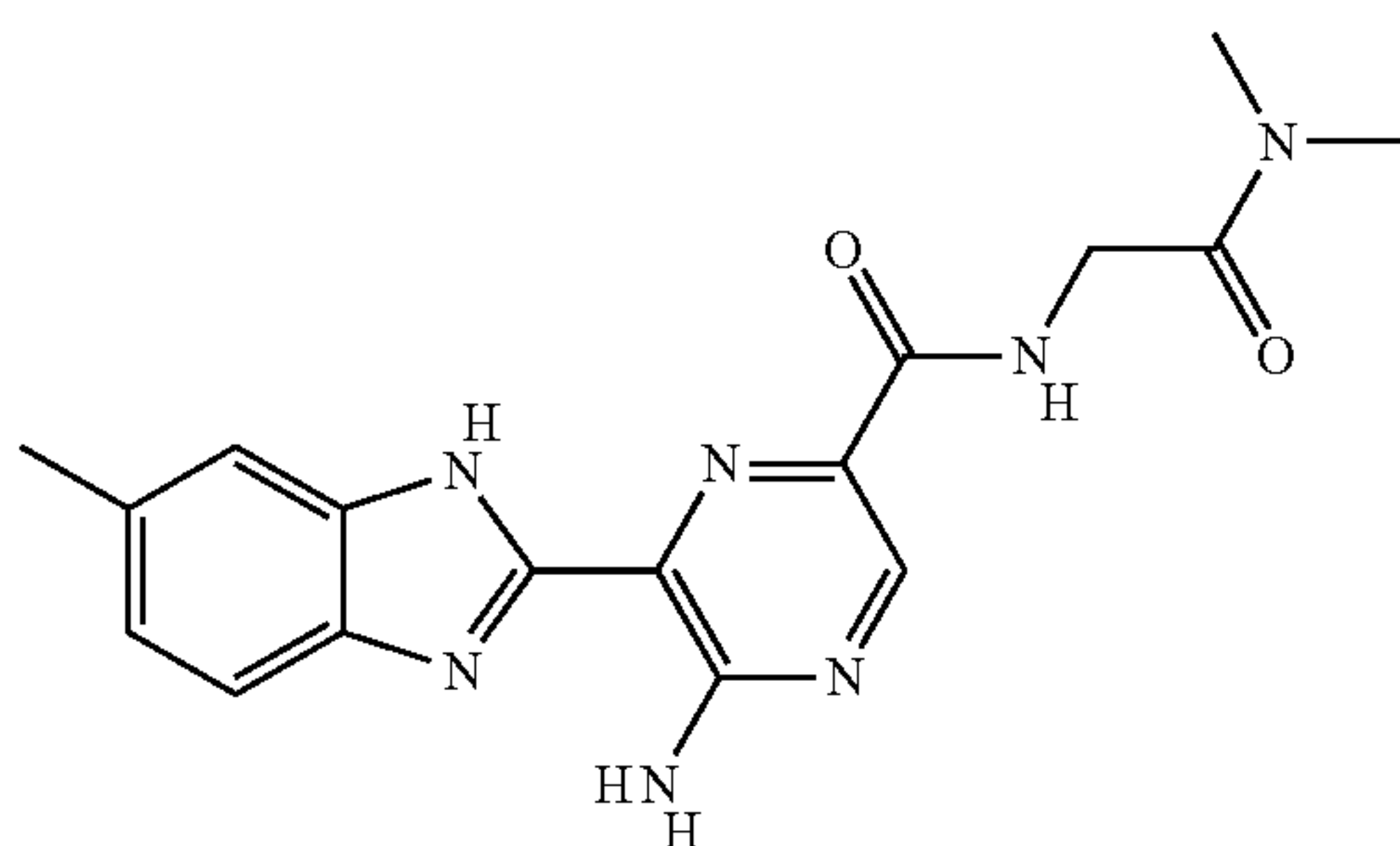
II-61
