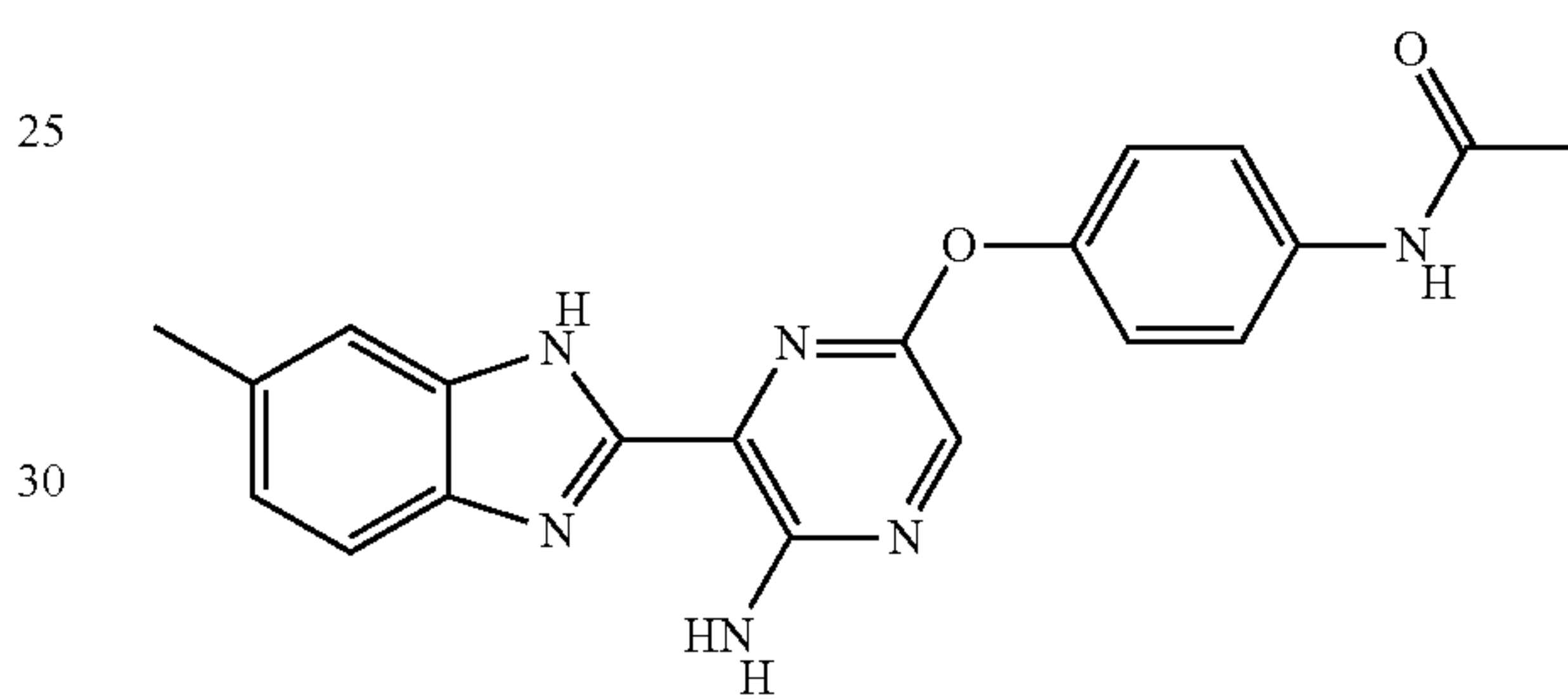
II-18
