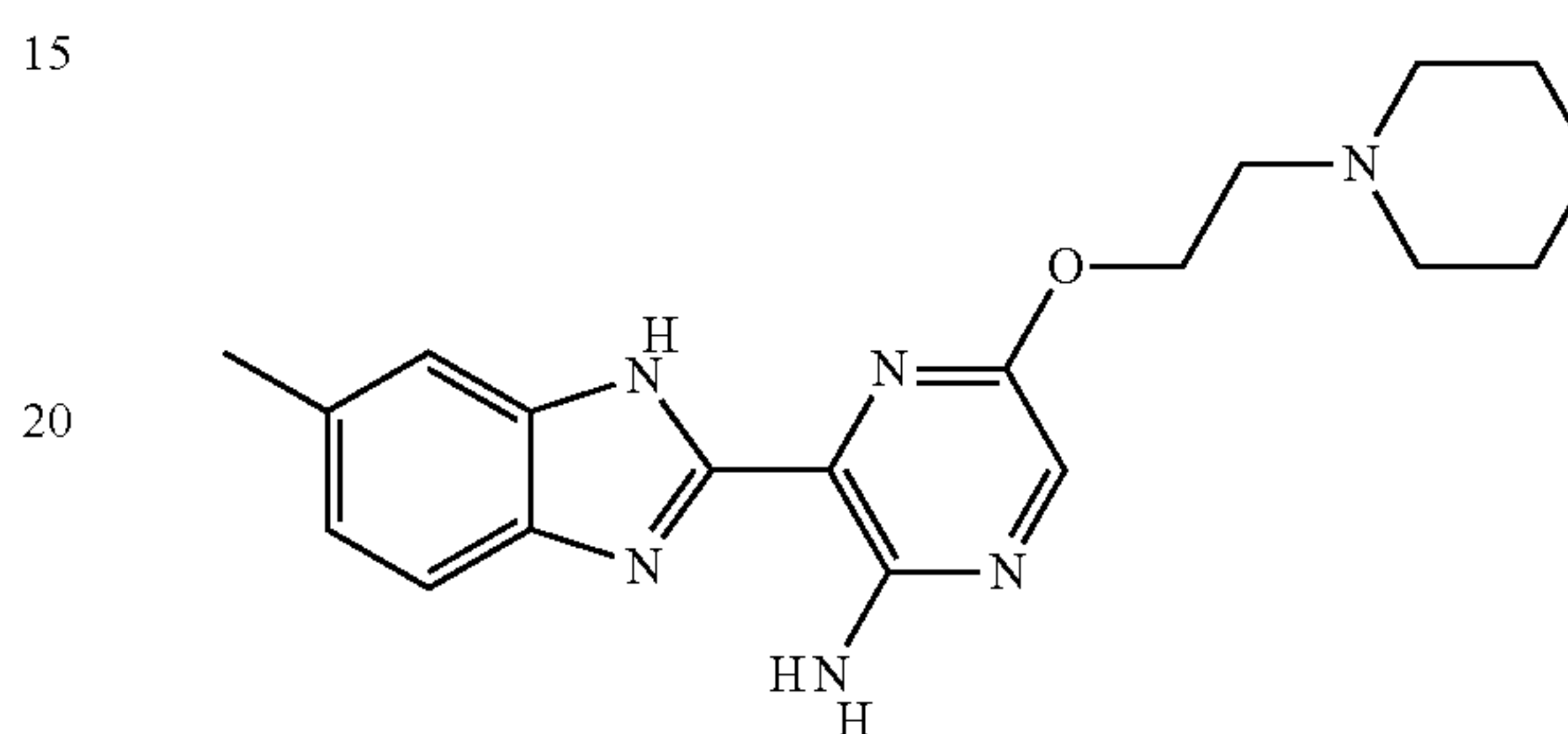
II-27
