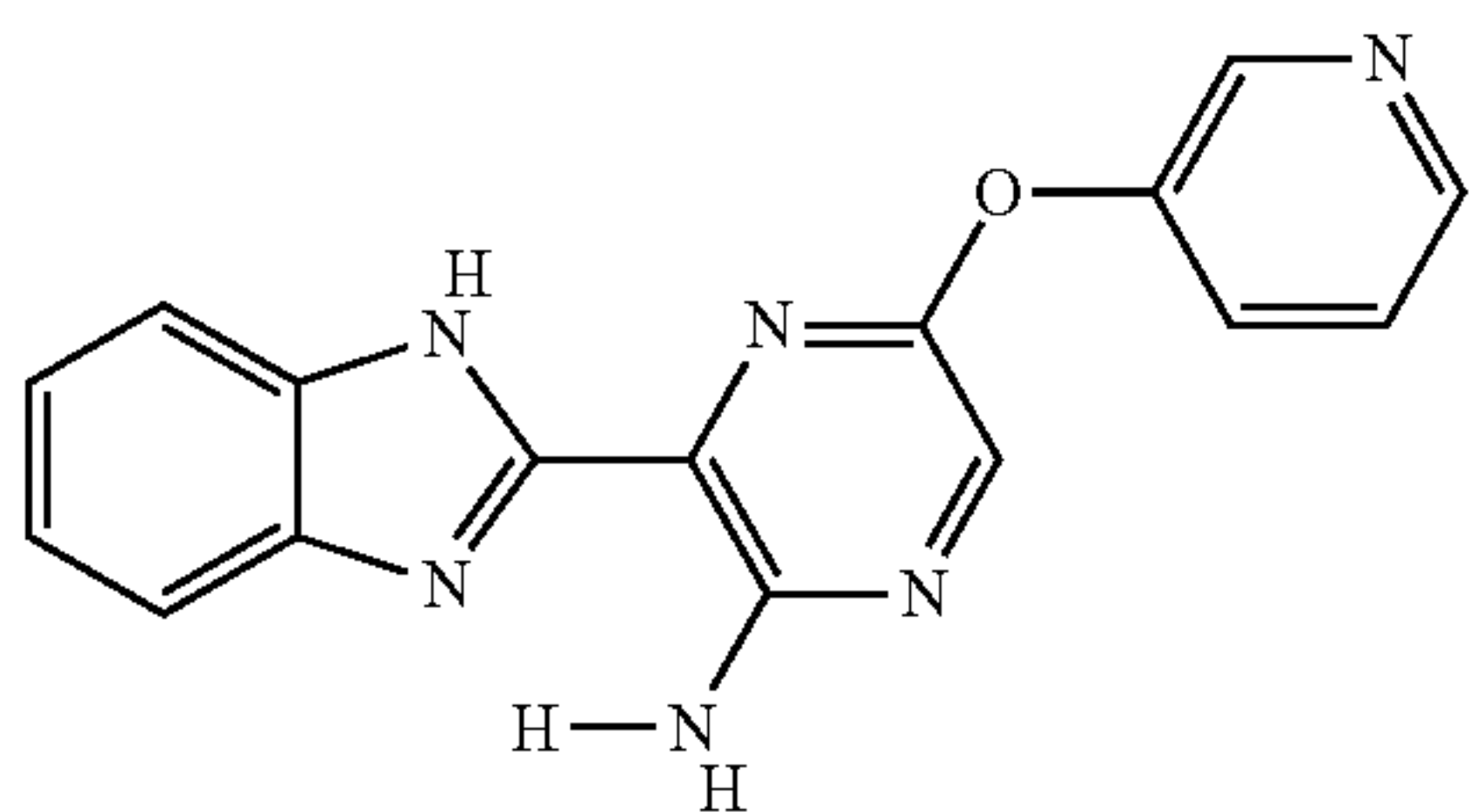
II-12
