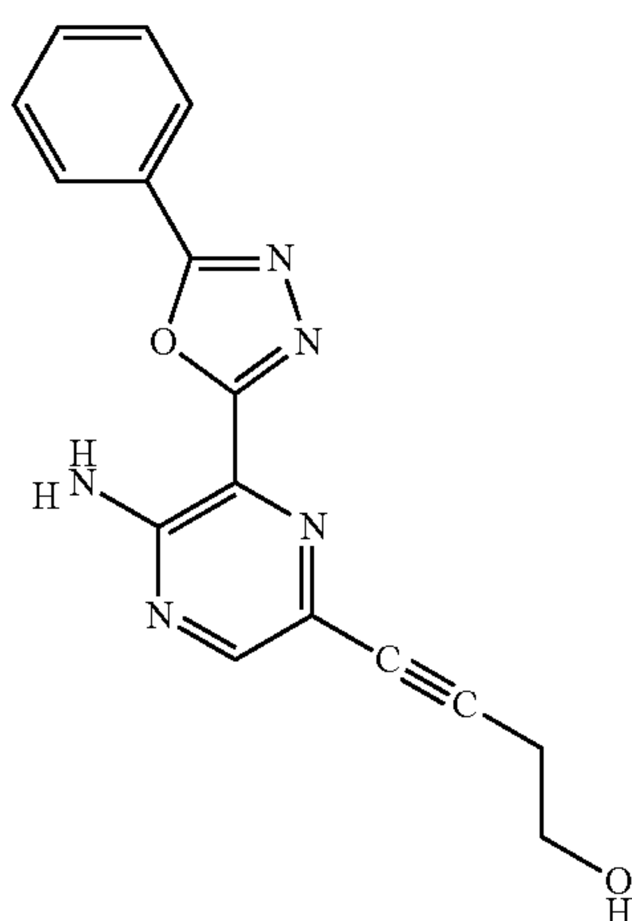
II-89
