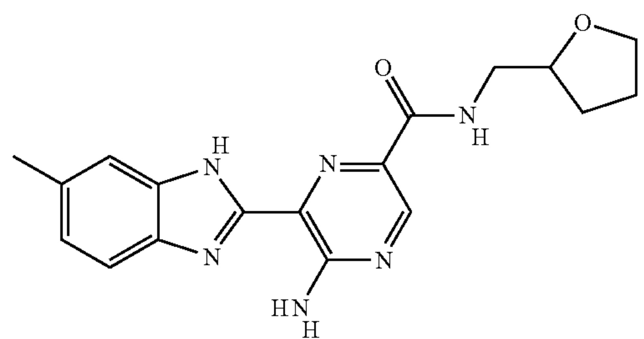
II-52
