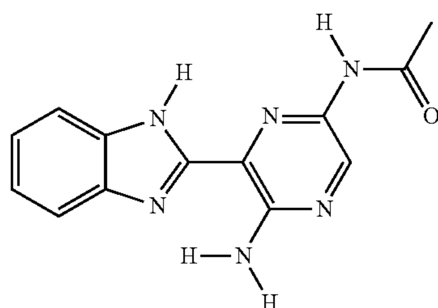
II-91
