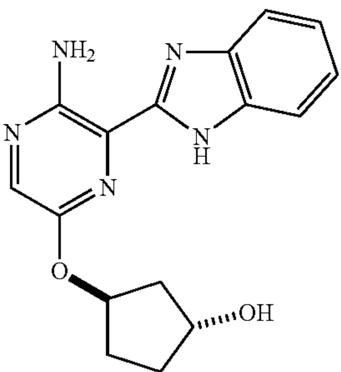
II-36
