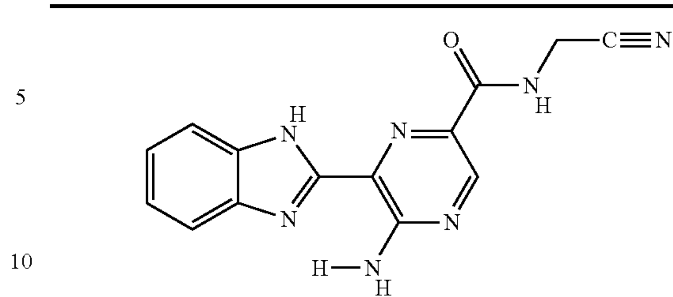
II-75
