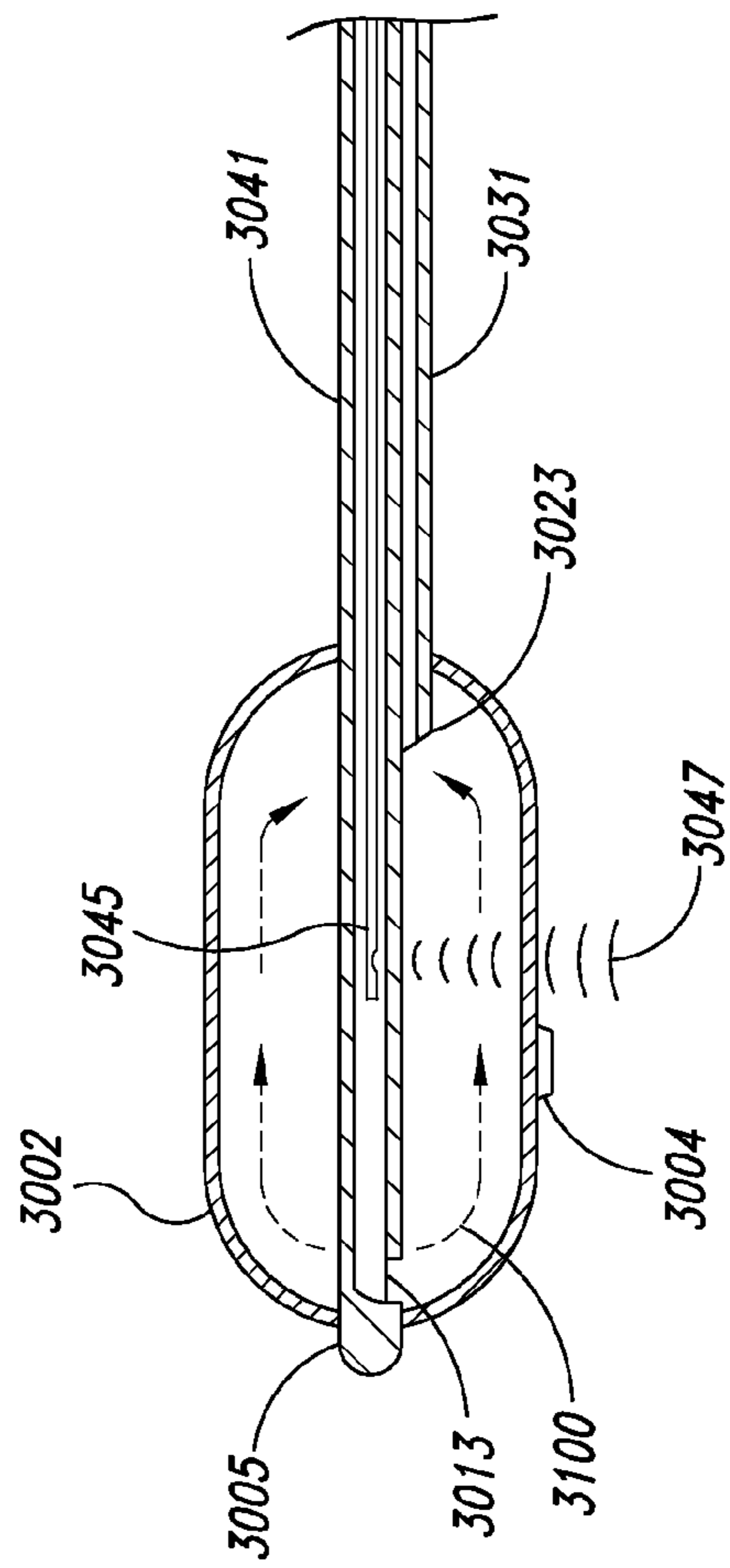
FIG. 20B
