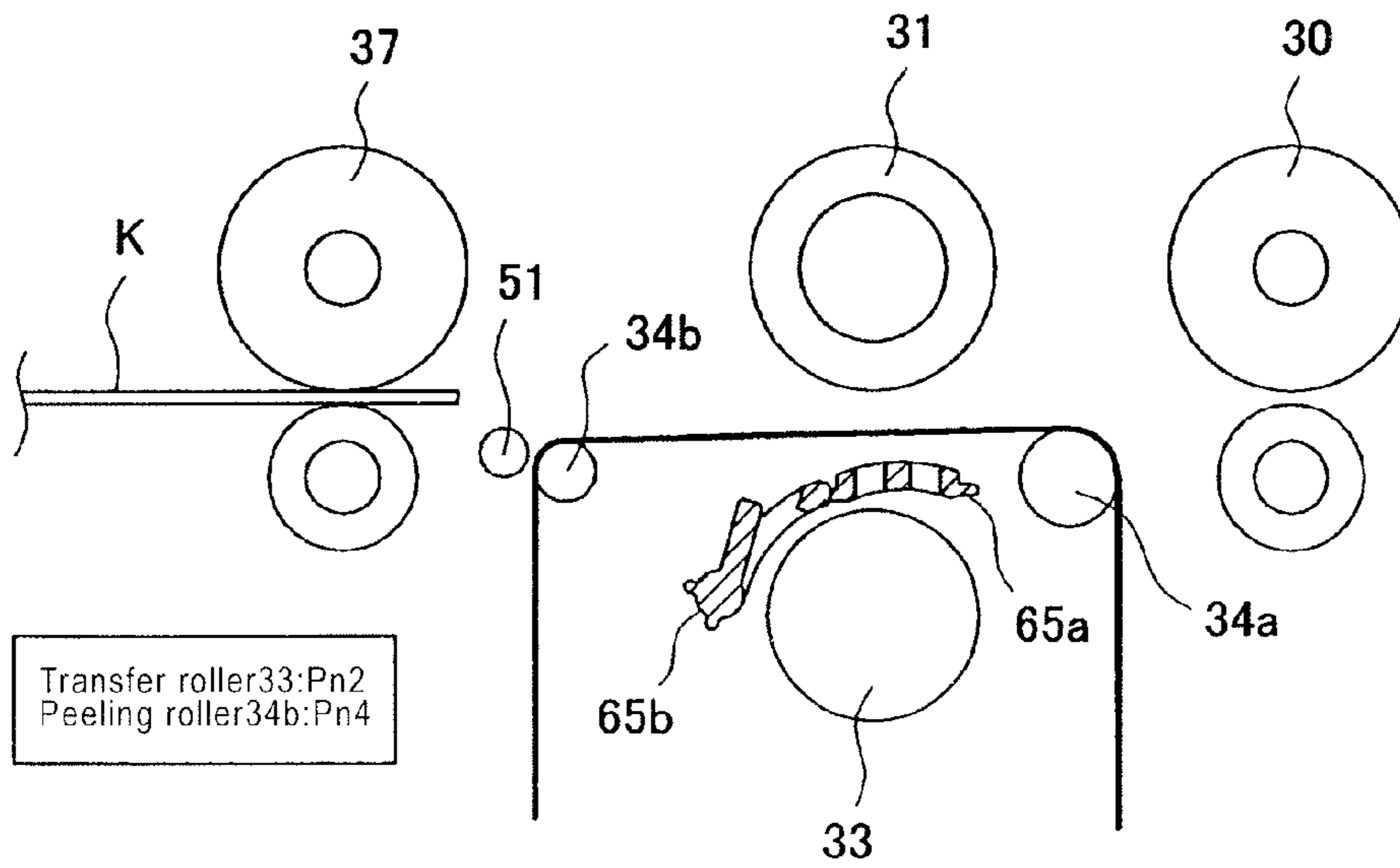
FIG. 4B
