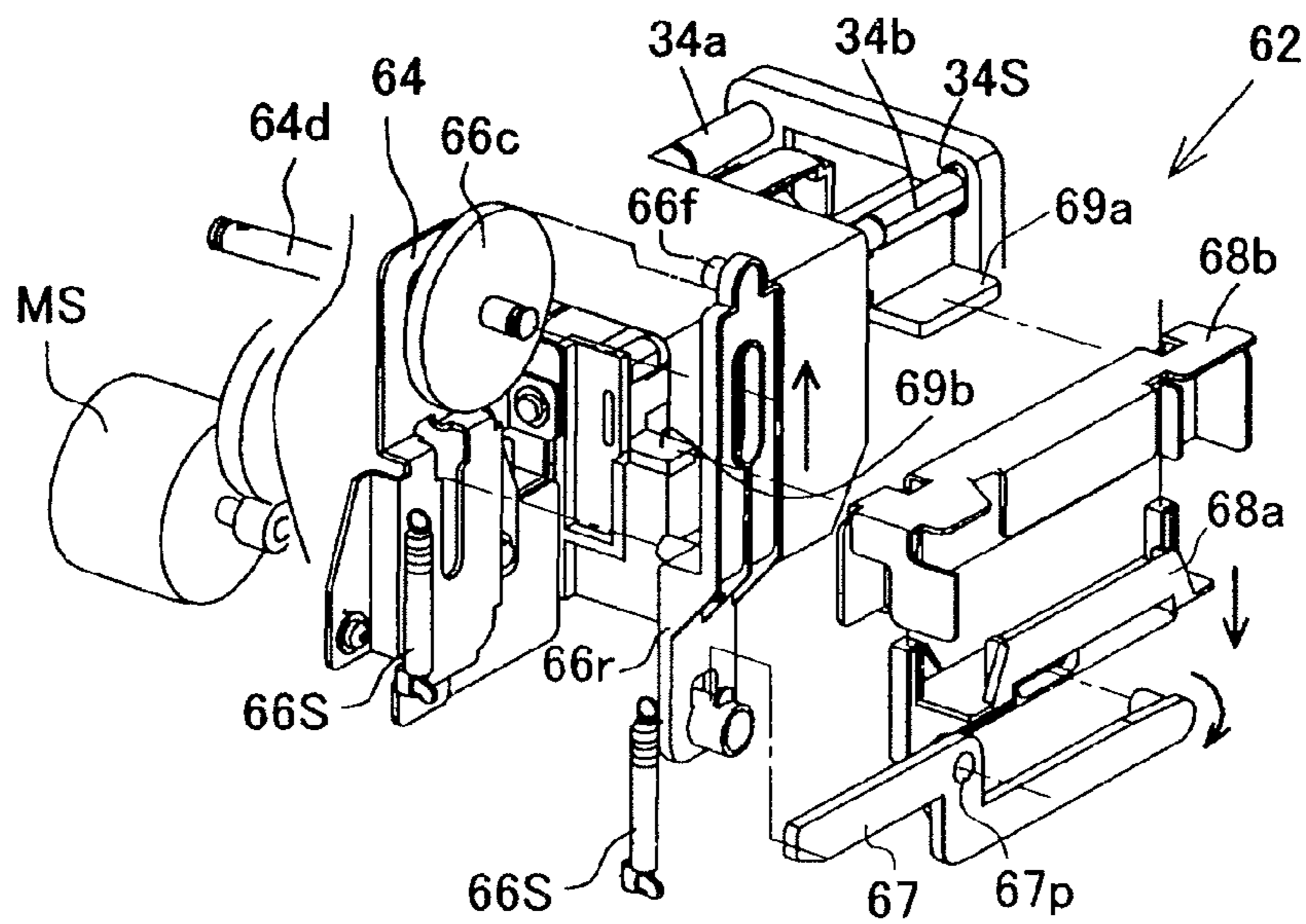
FIG. 8B
