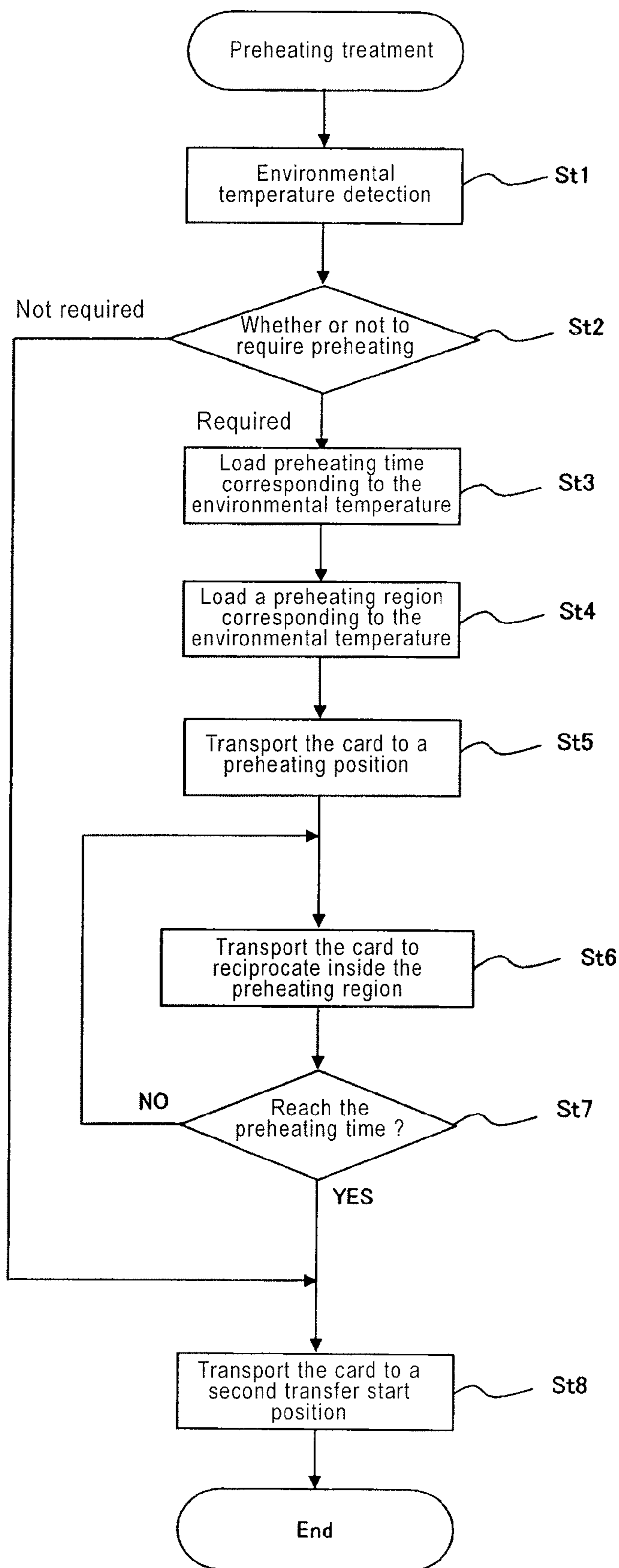
FIG. 14
