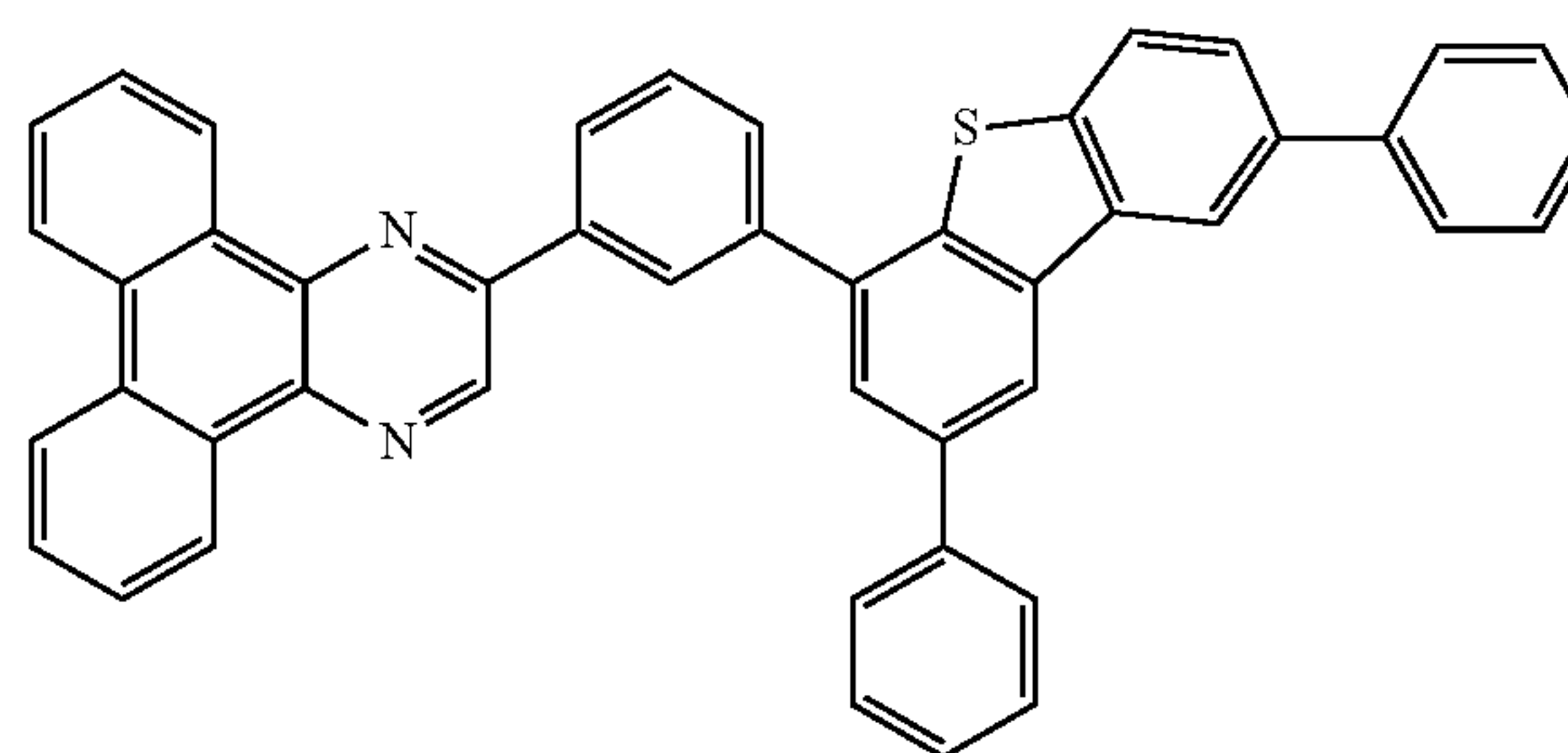
2mDBTPDBq-III
