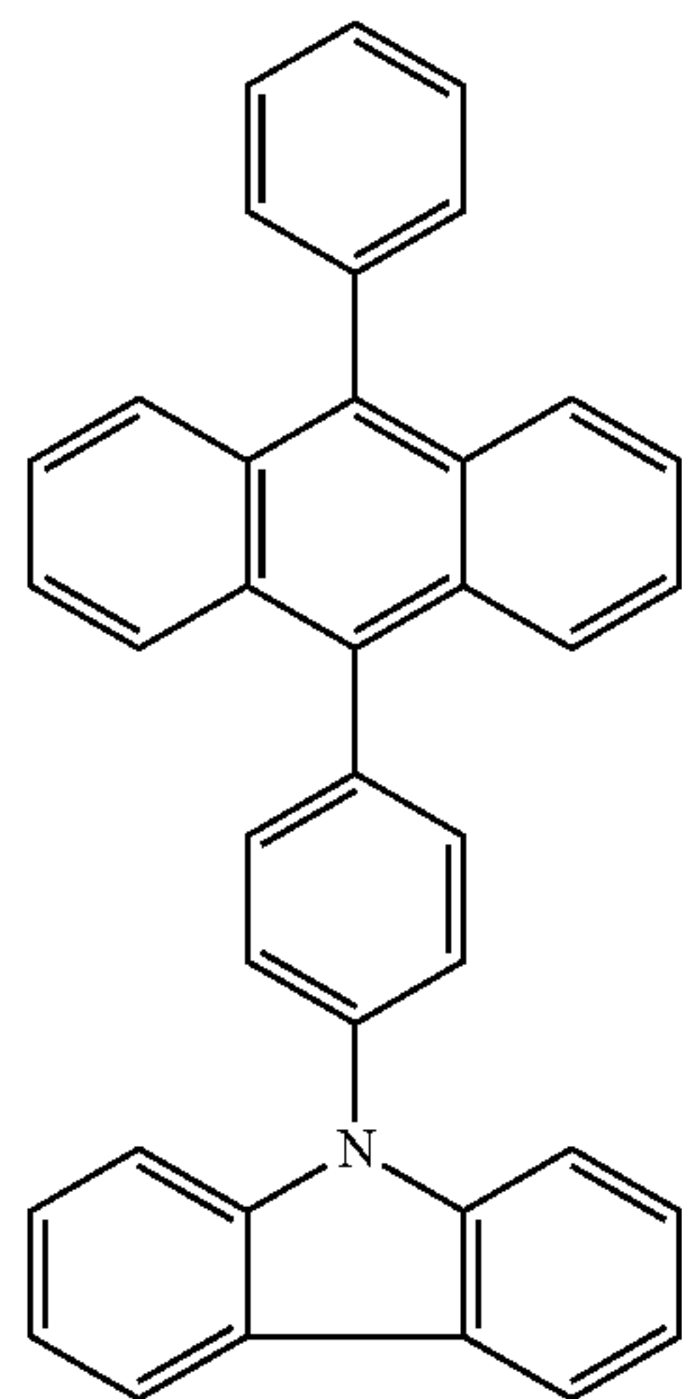
PCzPA
