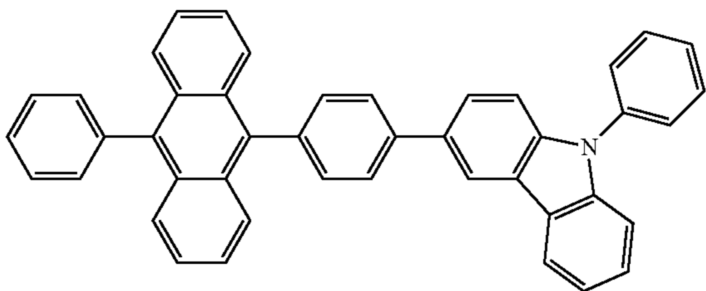
PCzPA
