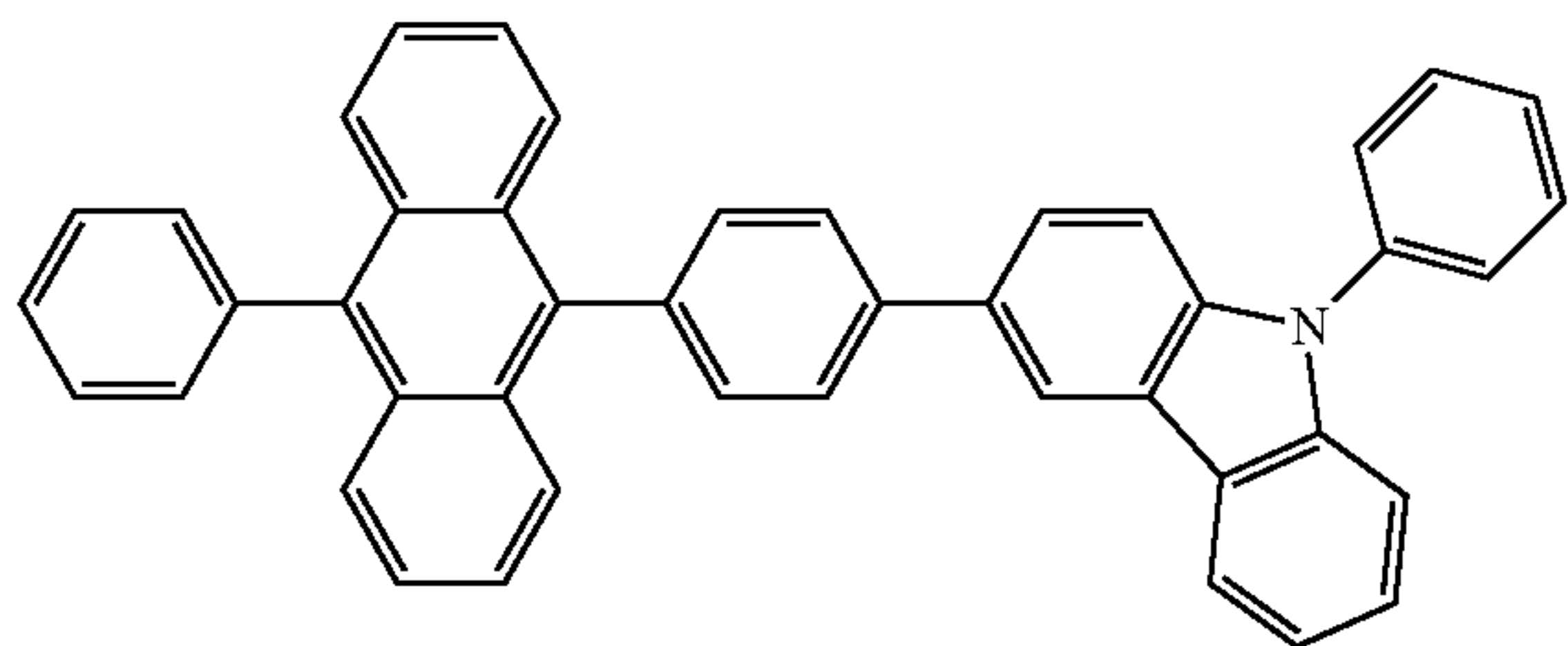
PCzPA
